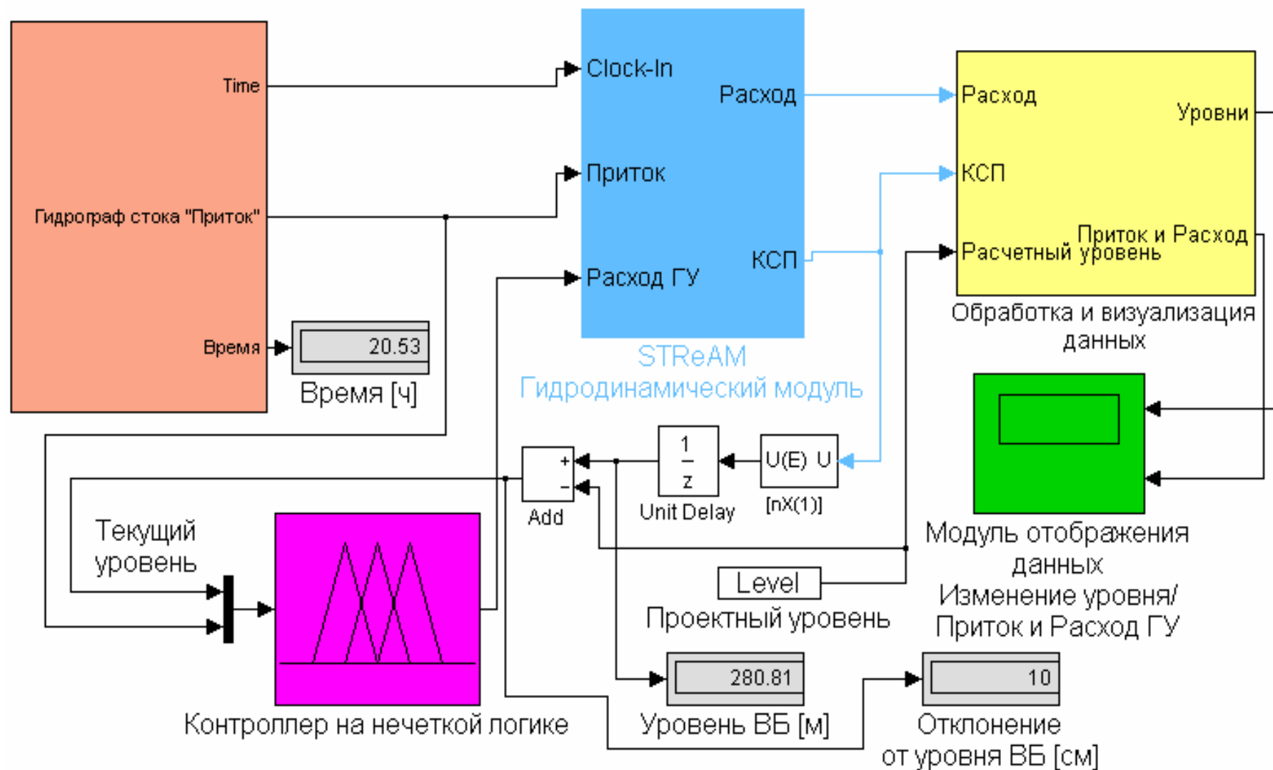
Рисунок 2 - Компьютерная модель регулирования
