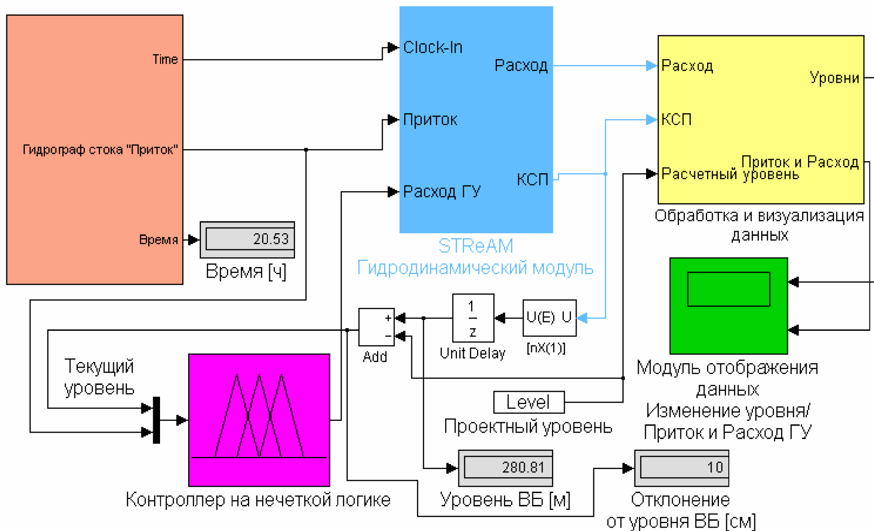
Рисунок 2 - Компьютерная модель регулирования
