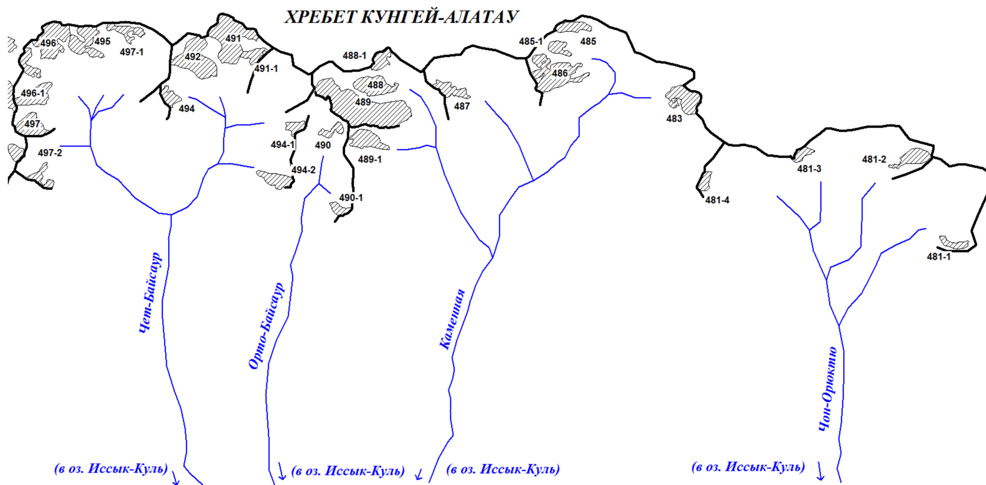
Рис. 44. Схема расположения ледников в бассейнах рек Чон-Орюктя, Каменная, Орто-Байсаур и Чет-Байсаур. Условные обозначения см. на рис. 26.
