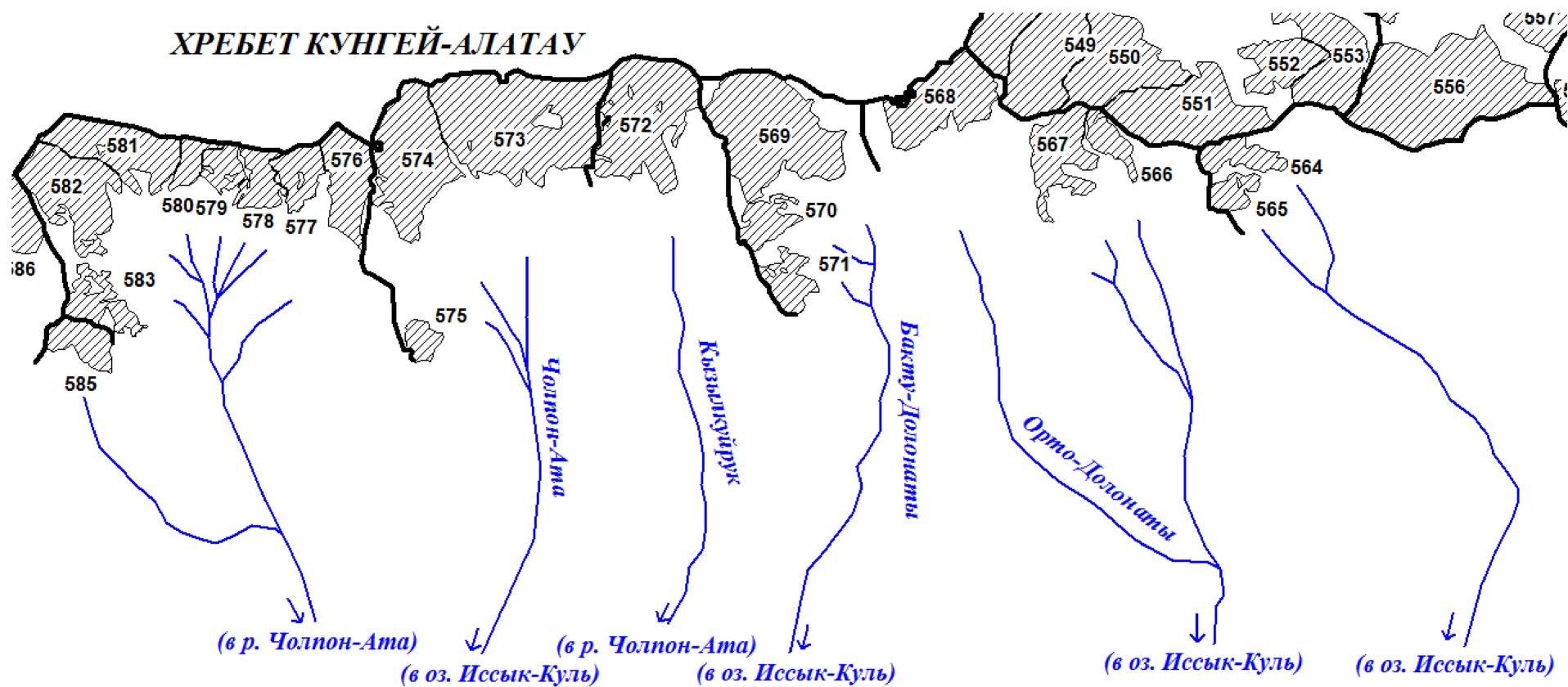
Рис. 47. Схема расположения ледников в бассейнах рек Орто-Долонаты, Бакту-Долонаты и Чолпон-Ата. Условные обозначения см. на рис. 26.
