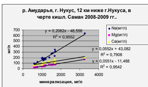
Рисунок 3 – Графики зависимости содержания главных ионов ( \text{Ca}^{2+} , \text{Mg}^{2+} , \text{Na}^{+} , \text{HCO}_3^{-} , \text{Cl}^{-} , \text{SO}_4^{2-} ) от величины минерализации на различных створах р. Амударья
