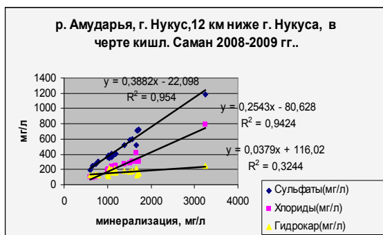
Рисунок 3 – Графики зависимости содержания главных ионов ( \text{Ca}^{2+} , \text{Mg}^{2+} , \text{Na}^{+} , \text{HCO}_3^{-} , \text{Cl}^{-} , \text{SO}_4^{2-} ) от величины минерализации на различных створах р. Амударья
