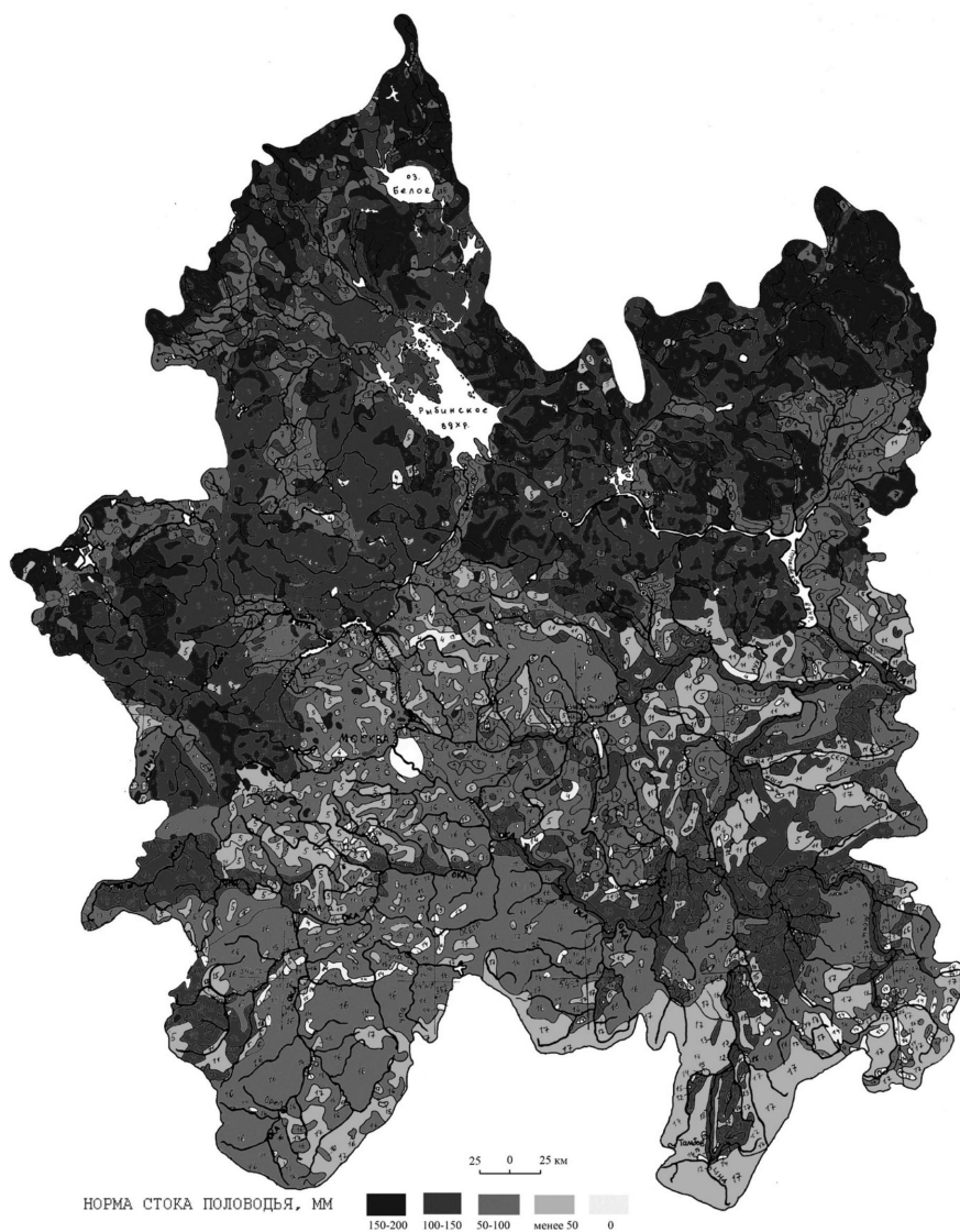
Рис. Средний многолетний сток половодья в основных ландшафтных комплексах бассейнов рек Оки и Верхней Волги, мм
