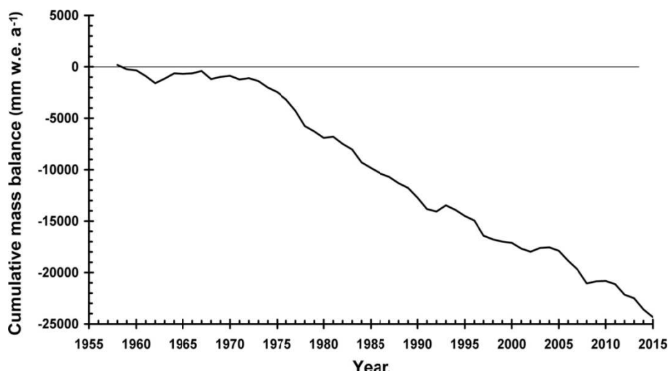
Рисунок 1– Кумулятивная кривая баланса массы ледника Туйыксу за 1957–2015 гг.
