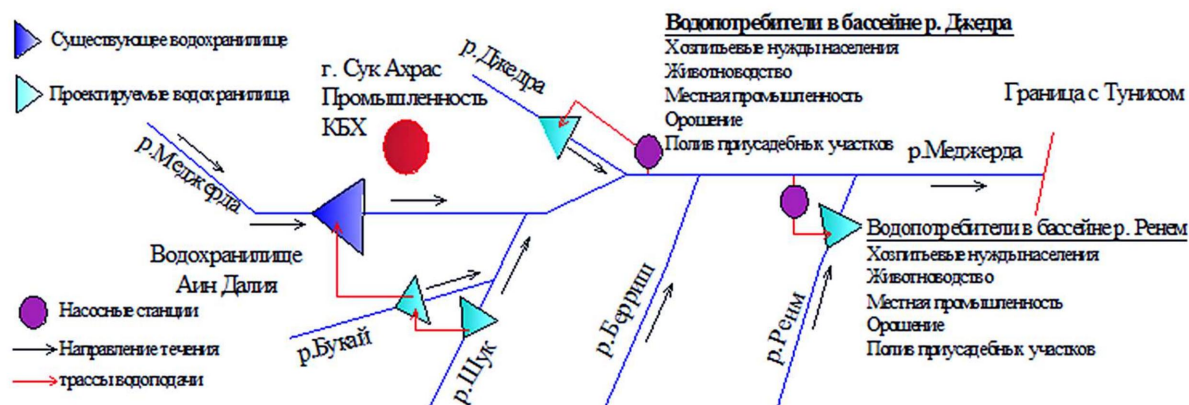
Рис. 2. Размещение водопотребителей по территории бассейна и возможные схемы дотации части стока в регулирующие водохранилища
