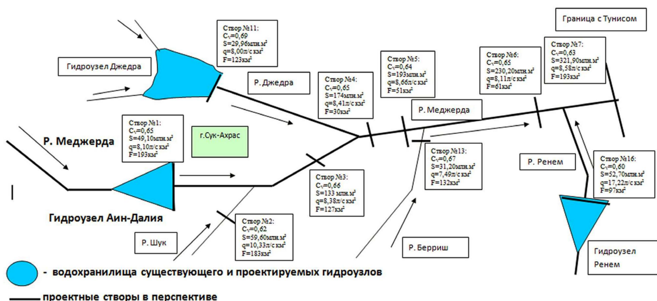
Рис. 1. Основные гидрологические характеристики реки Меджерды
