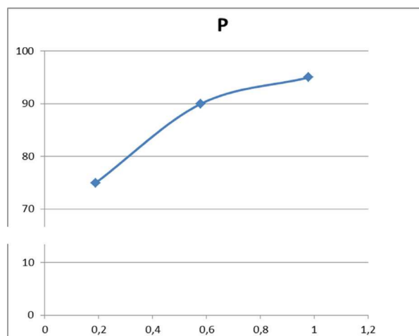
Рис. 6. Сечение номограмм при \alpha = 0,8 ; C_v = 0,4
