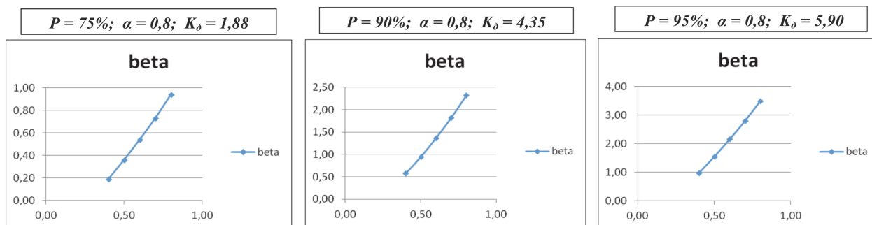
Рис. 4. Ветви традиционных номограмм при фиксированных значениях отдачи
