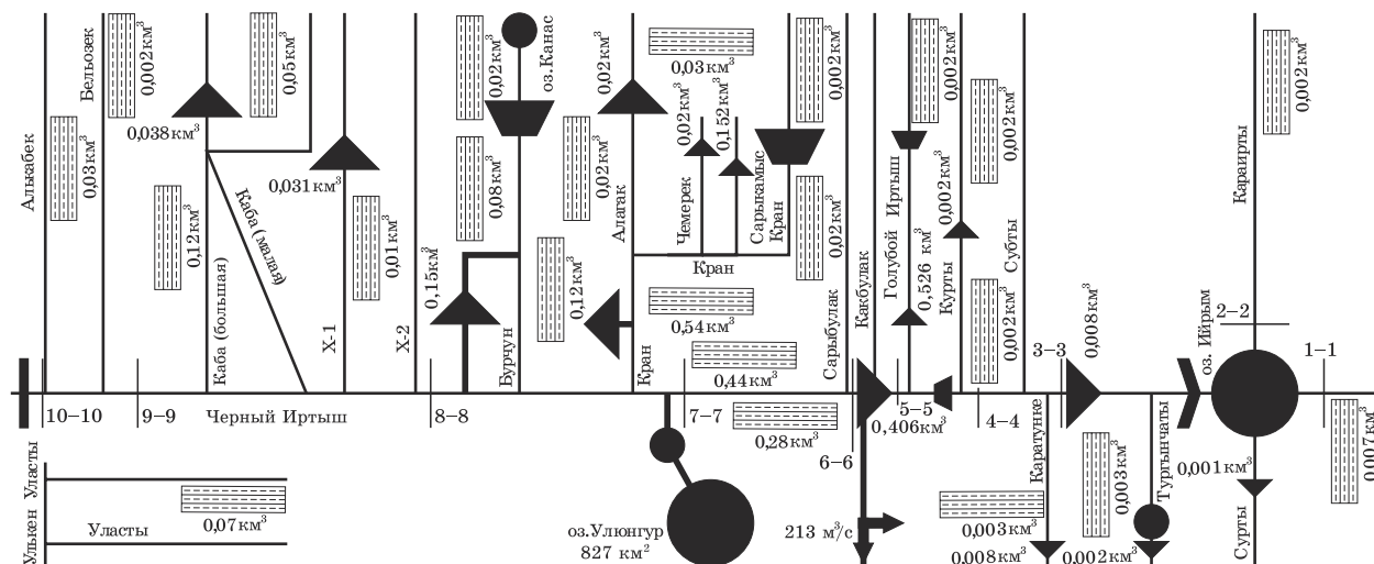
Рис. 1. Водохозяйственный комплекс реки Черный Иртыш: — — реки; ● — озера; ▲ — водохранилища; 0,15 км 3 — объем водохранилищ; ▨ — орошаемые земли; 0,01 км 3 — объем воды, забираемый на орошение; — — каналы; р. Черный Иртыш — название рек, озер; ◀ — строящиеся гидроузлы, каналы; ■ — граница между Китаем и Казахстаном; } — плотина; | 00 — створ и номер створа
