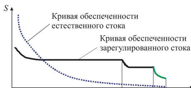
Рис. 3. Кривые обеспеченности естественного и зарегулированного стоков
