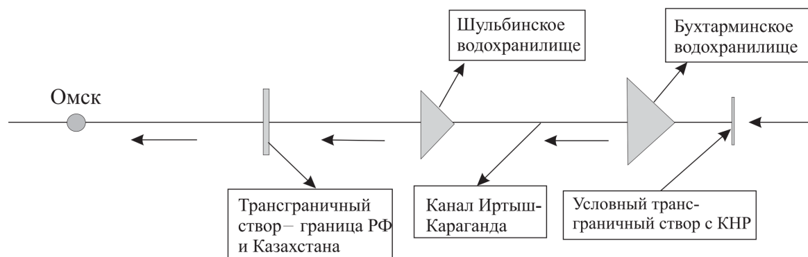
Рис. 1. Водохозяйственная система среднего Иртыша
