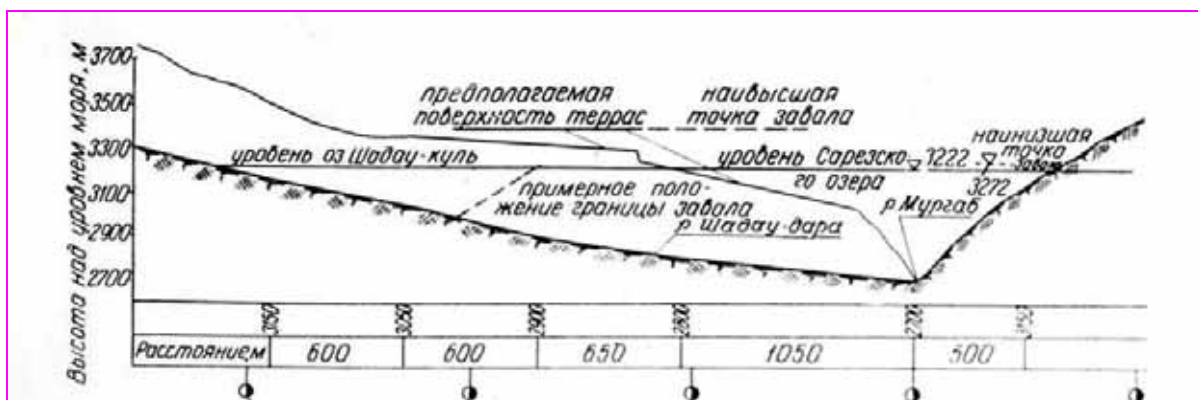
Рис. 7. Совмещенные поперечные профили на левом берегу. Значительная масса обвала легла на конус выноса р. Шатаудара впереди террас
