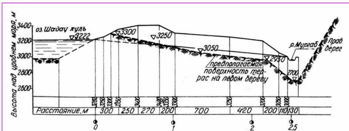
Рис. 9. Поперечный профиль через завал от озера Шатаукуль до р. Мургаб
