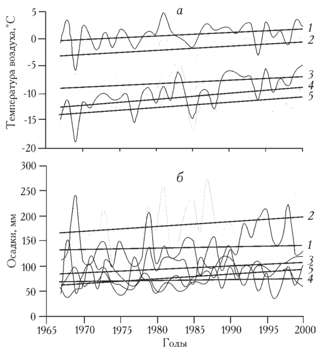
Рис. 1. Изменение средней температуры воздуха (а) и сумм осадков (б) за холодный период (ноябрь—март), 1966—2000 гг., по данным метеостанций Арыс (1), Алматы (2), Урalsк (3), Семипалатинск (4), Петропавловск (5)
