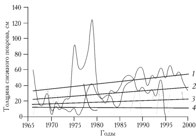
Рис. 3. Толщина снежного покрова в первую декаду марта, измеренная по постоянным рейкам (1966—2000 гг.) на метеостанциях Петропавловск (1), Уральск (2), Семипалатинск (3), Алматы (4)
