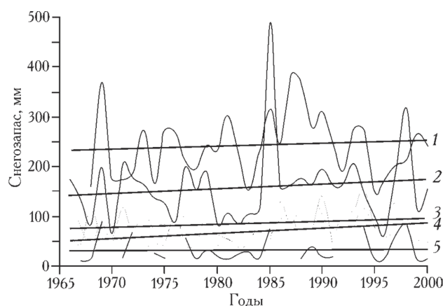
Рис. 4. Многолетние изменения средних из максимальных снеговодосодержаний (1966—2000 гг.) по данным метеостанций Большое Алма-тинское озеро (1), Кокпекты (2), Петропавловск (3), Уральск (4), Арыс (5)
