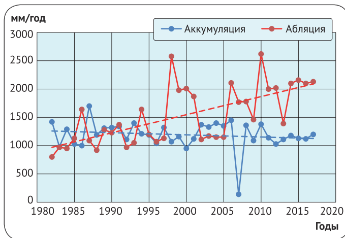
Рис. 5. Аккумуляция и абляция ледника Гарабаши. Источник: Ледники и климат Эльбруса. М.; СПб., 2020.
