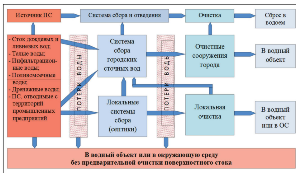
Рисунки 2. – Схематичное изображение системы сбора, отвода и очистки сточных вод и поверхностного стока
