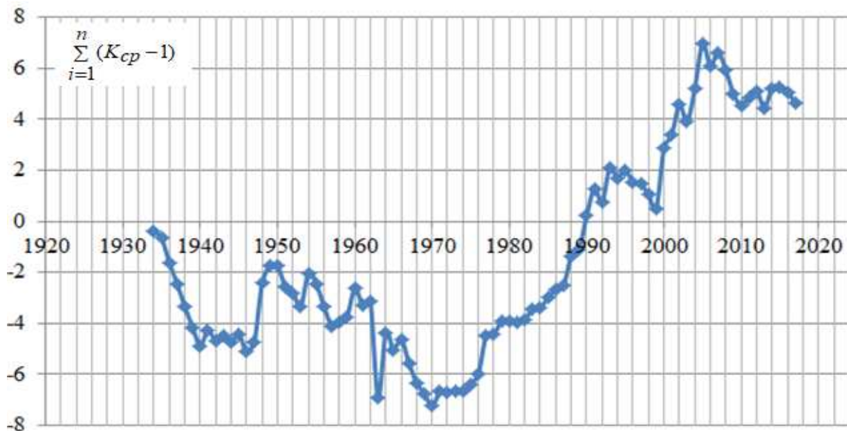
Рисунок 2 – Разностная интегральная кривая расходов воды реки Тобыл (гидрологический пост Гришкина)
