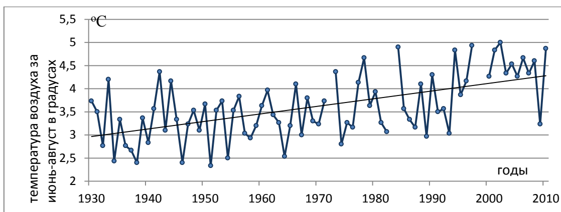
Рис. 18. Изменение средней температуры воздуха за июнь-август по метеостанции Тянь-Шань
