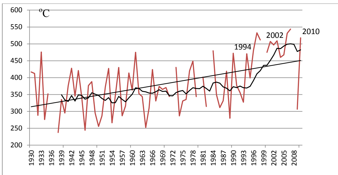
Рис.11 Сумма положительных температур на метеостанции Тянь-Шань
