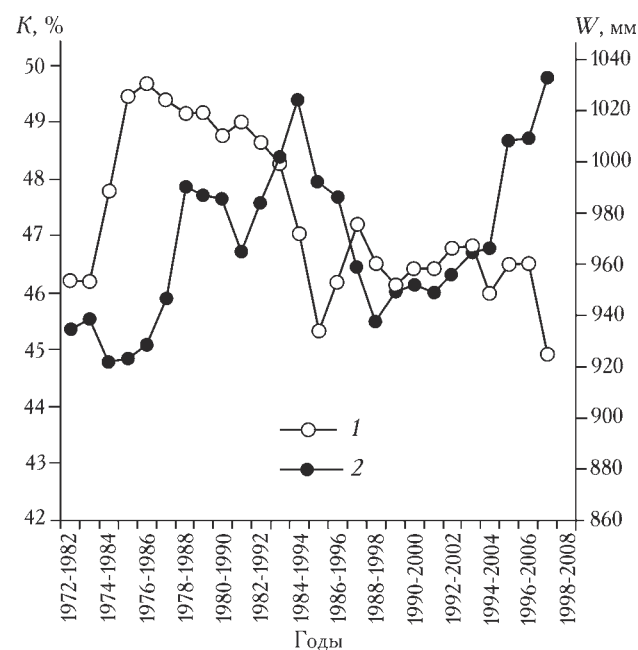
Рис. 1. Изменения скользящих по десятилетиям средних значений индекса континентальности K (1) и суммарного количества осадков W (2) за балансовый год для ледника Туяксу за 1972—2006 гг.
