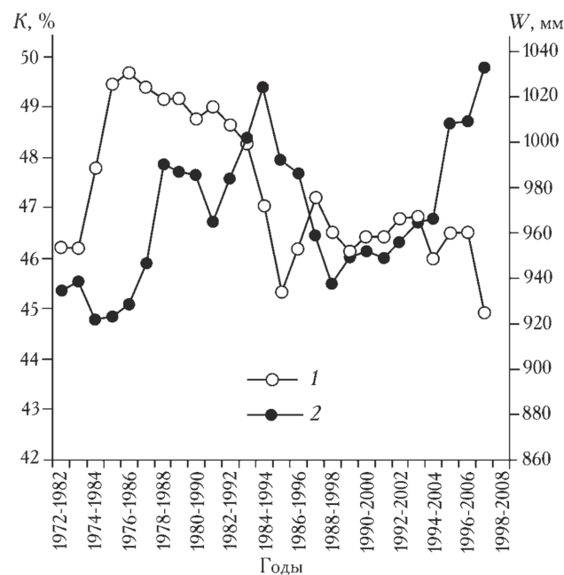
Рис. 1. Изменения десятилетних средних значений индекса континентальности K (1) и суммарного количества осадков W (2) за десятилетия для ледника Туяксу за 1972—2006 гг.
