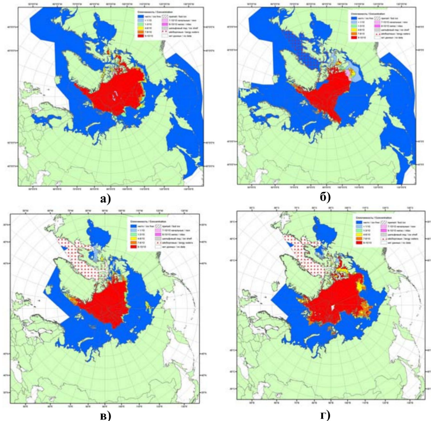
Рис. 2. Ледовая обстановка в годы наименьшей ледовитости на российских арктических морях в середине сентября: 2005 г. (а), 2007 г. (б), 2012 г. (в), 2014 г. (г).
