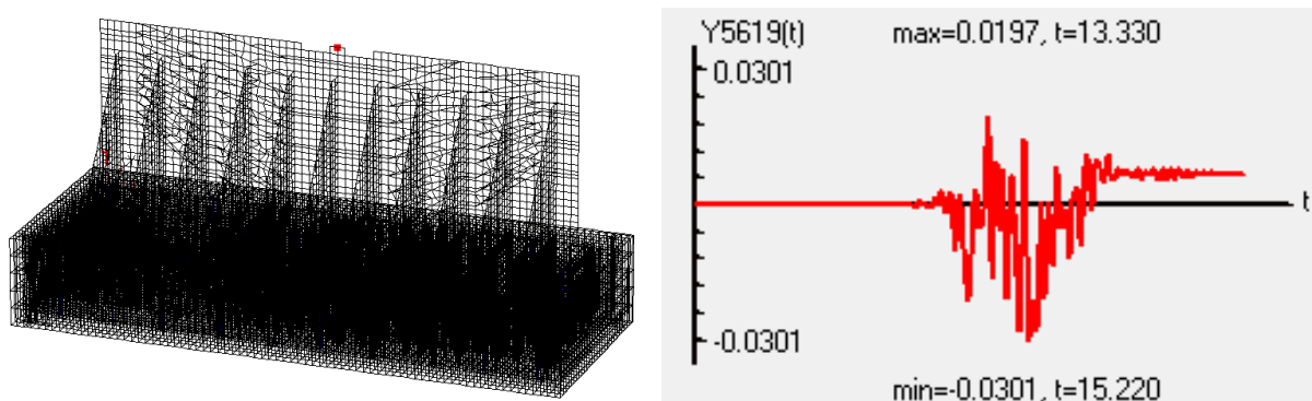
Рисунок 7 – Перемещение конструкции
