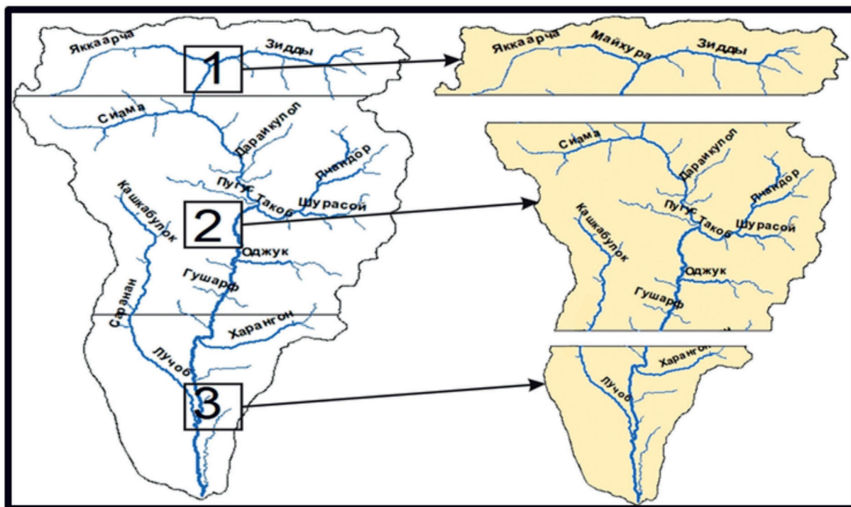
Рис. 5. Схема деления на 3 участка (района) бассейна реки Варзоб
