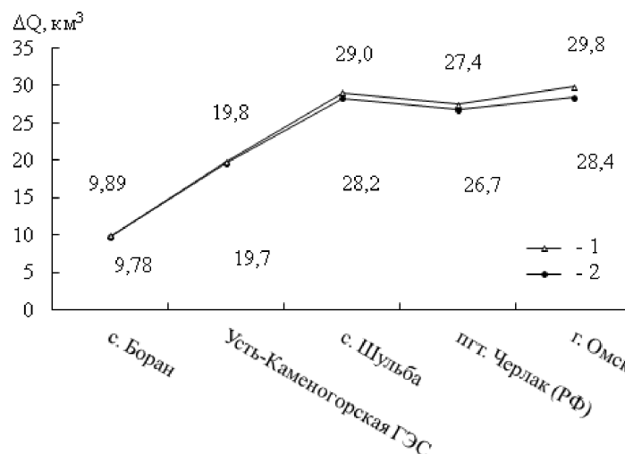
Рис. 2. График изменения среднемноголетней нормы стока рассчитанной за период 1931...1973 гг. (1) и нормы стока (из [2]) (2) по длине р. Ертис.
