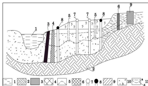
Рис. 9. Комплексный барьер с двухсторонним поступлением загрязняющих веществ к водозаборам хозяйственно-питьевых вод одновременно от реки и с водосбора. 1 – водоем с загрязненной водой, 2 – водопор. барьеры: 3 – биохимический, 4 – природно-техногенный, 5 – гидродинамический, 6 – искусственный геохимический, 7 – водозаборные скважины, 8 – дренажные скважины, 9 – источник загрязнения, 10 – аллювиальный горизонт, 11 – УГВ (а – статический, б – динамический).
