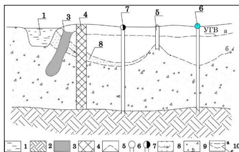
Рис. 7. Схема комплексного барьера с временным дренажем (разрез): 1 – водоем с загрязненной водой, 2 – водопор. барьеры: 3 – стихийный биохимический, 4 – природно-техногенный, 5 – гидродинамический, 6 – водозаборные скважины, 7 – дренажные скважины, 8 – потоки загрязненных вод, 9 – водоносный горизонт, 10 – УГВ: а – статический, б – динамический.
