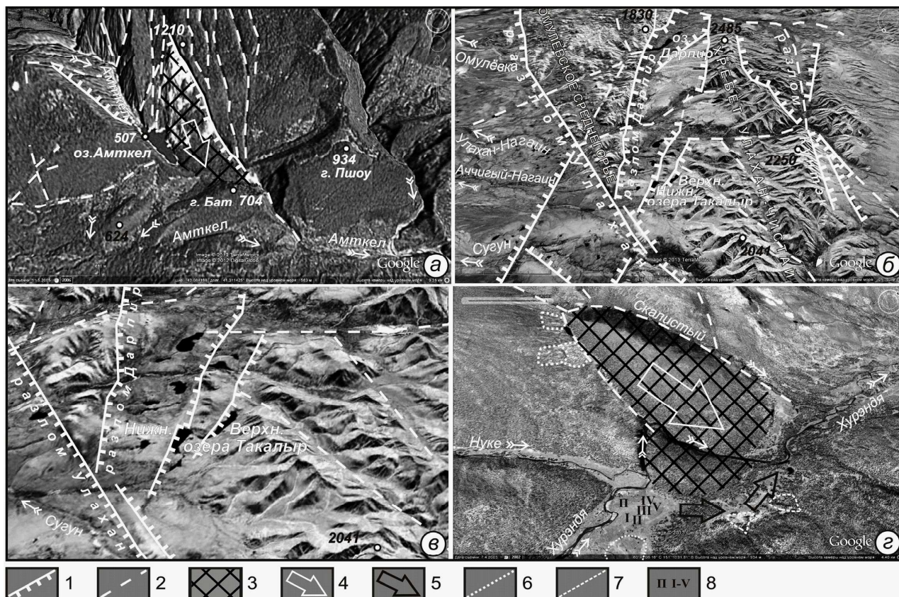
Рис. 3. Тектонические и сейсмотектонические запруды горных долин: а – оз. Амткел в Абхазии; б, в – озёр Дарпир и Такалыр в горах Черского; г – долины р. Хуронда в Северном Приохотье. 1 – сбросовые и взбросовые уступы, местами со сдвиговой составляющей; 2 – разломы без заметной вертикальной составляющей, в том числе и раздвиговые; 3 – блоки горных пород, сместившиеся по вертикали и горизонтали; 4 – направления горизонтального смещения блоков; 5 – брошенный участок долины р. Хуронда; 6 – контуры малых (объемами < 1 млн м 3 ) оползней; 7 – контуры пролювиально-селевых конусов выноса; 8 – поймы и надпойменные террасы на месте бывшего подпрудного озера пра-Нукэ, сформировавшиеся за счет вреза р. Хуронда при спуске её вод через раскрывающуюся и промываемую расщелину
