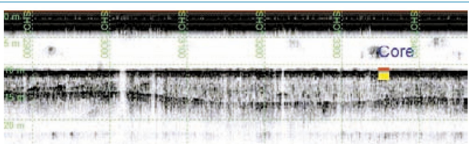
Рис. 6. Сплошное распространение илов в центральной части водохранилища: core – положение точки опробования грунтовой трубкой; цветные слои сверху вниз – ил, торф и подстилающий слой озерно-аллювиальных песков; горизонтальные линии проведены через 5 м. Fig. 6. The silts continuous distribution in the reservoir central part; core is the location of the ground pipe sampling point; colored layers downword are silt, peat and underlying layer of lacustrine/alluvial sands; horizontal lines with the 5 m interval.
