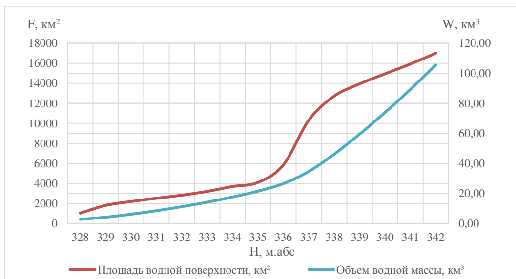
Рисунок 2. График зависимости параметров озера от уровня воды
