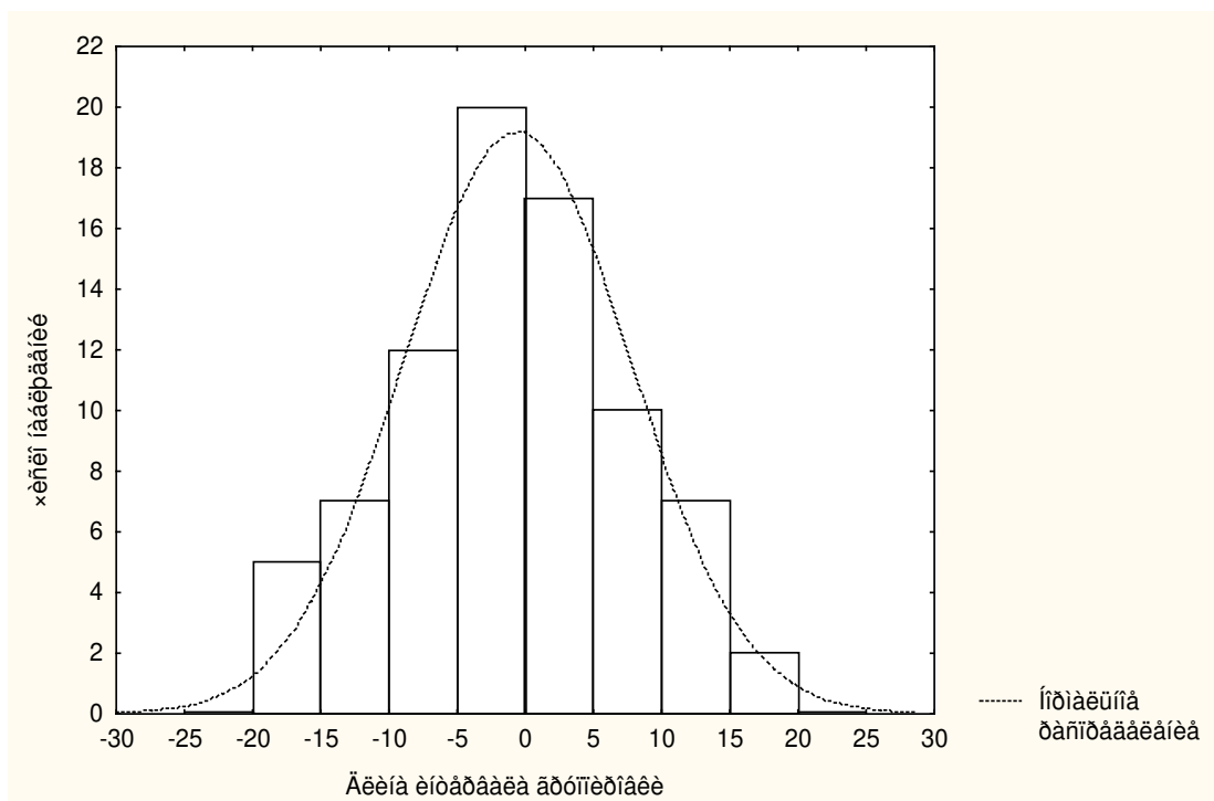
Рис. 8. Гистограмма сглаженных значений годовых приращений УМК с нормальной наложенной плотностью распределения.
