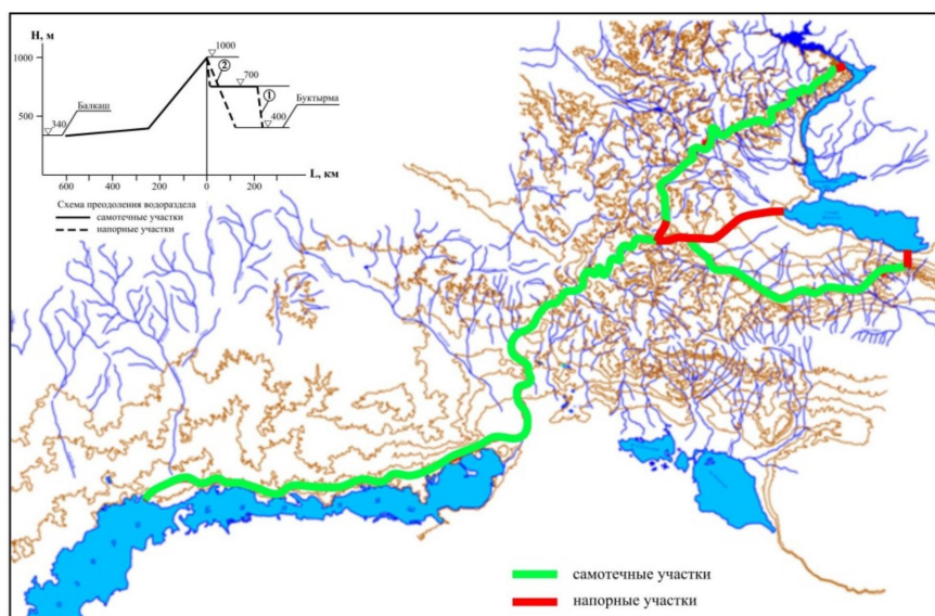
Рисунок 13 – Переброска стока р. Ертис в озеро Балкаш
