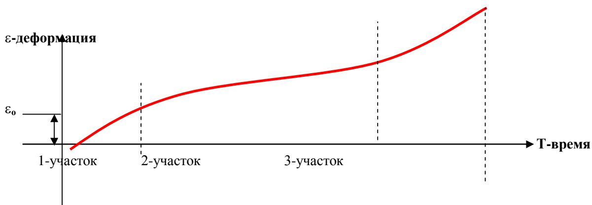
Рис.1. Кривая ползучести материалов
