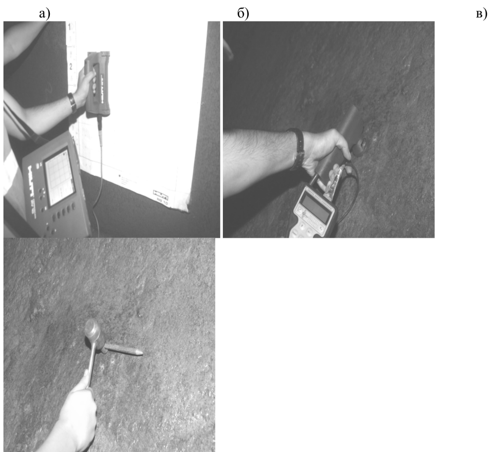
Рис. 3. Оценка прочности обделки камеры гидроагрегата №3 а - обнаружение и анализ арматуры с использованием портативной системы (Ferroskan FS 10); б - проверка прочности методом ударным импульсом ИПС-МГ4.03; в - проверка прочности ударным способом молотком Кашикарова
