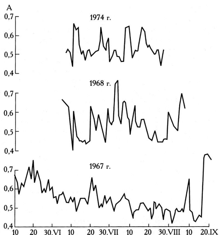
Рис. 1. Изменение альбедо поверхности в фирновой зоне ледника Марух в теплые периоды 1967, 1968 и 1974 гг
