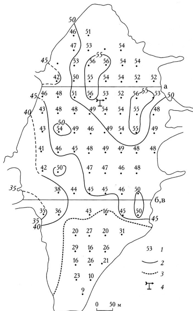
Рис. 2. Распределение альbedo на леднике Обручева 20 июля 1976 г. 1 — величина альbedo, %; 2 — изолинии альbedo; 3 — граница сезонного снега; 4 — метеоплощадка; а, б, в — профили учащенной альбедосъемки
