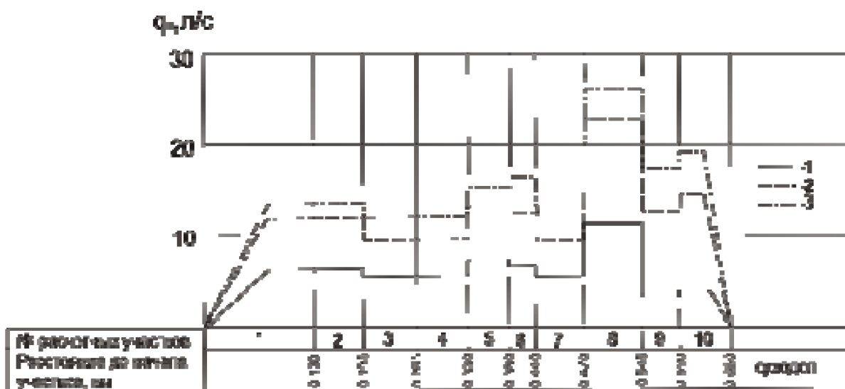
Рисунок Н.2.3.3 - Эпюры интенсивности притока болотных вод к дорожной трассе
