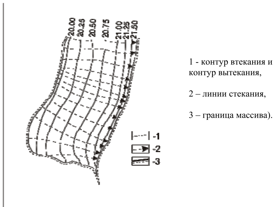
Рисунок Н.2.2.1 - План в горизонталях (мБС) и сетка линий стекания болотного массива с транзитным стоком, представленного осоково-сфагновым, облесённым берёзой и сосной микроландшафтом
