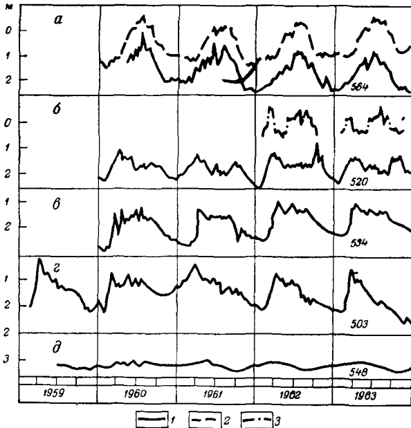
Рис. 49. Графики изменения уровня грунтовых вод долины среднего течения р. Амударьи
