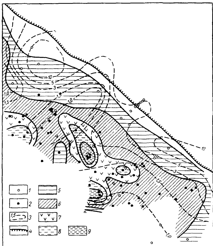
Рис. 56. Схема снижения уровня подземных вод на участке водозабора Ашхабадского конуса выноса
