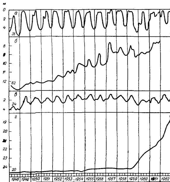
Рис. 50. Графики изменения уровня грунтовых вод Мургабского оазиса а — искусственный гидрологический режим грунтовых вод с глубиной залегания уровня до 5 м; б — искусственный гидрологический режим с глубиной залегания уровня более 5 м; в — ирригационный режим с глубиной залегания уровня до 5 м, г — ирригационный режим с глубиной залегания уровня более 10 м. Цифры на кривых — номера наблюдательных скважин
