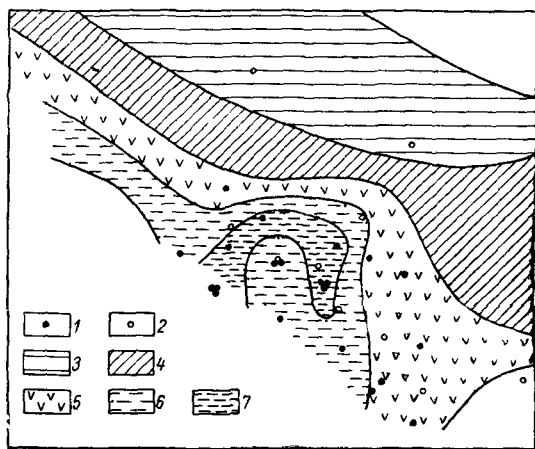
Рис 58 Схема снижения уровня подземных вод на участке водозабора Алтыябского конуса выноса
