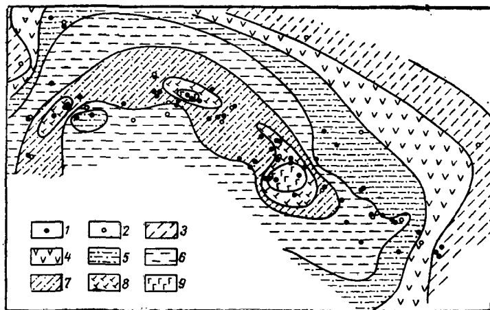
Рис. 57. Схема снижения уровня подземных вод на участке водозабора Фирюзинского конуса выноса
