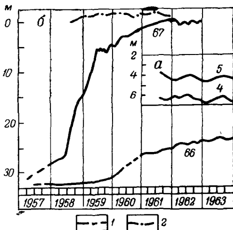
Рис. 52. Графики изменения уровня грунтовых вод в зоне влияния Каракумского канала а — циклический преимущественно компенсированный режим грунтовых вод, б — положительно декомпенсированный режим грунтовых вод.
