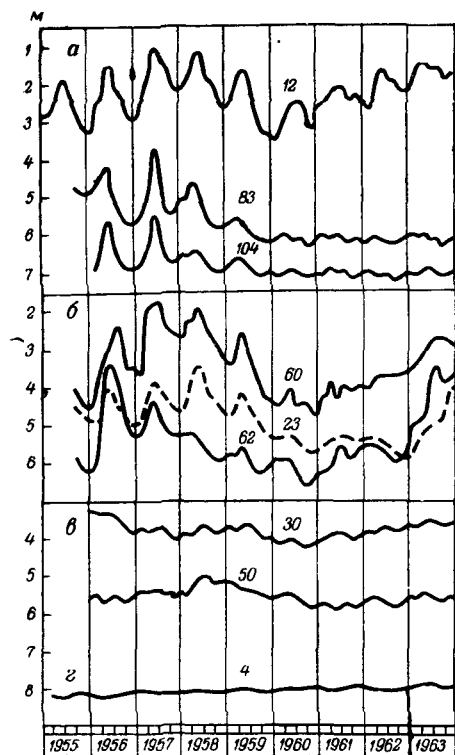
Рис. 51. Графики изменения уровня грунтовых вод Тедженского оазиса
