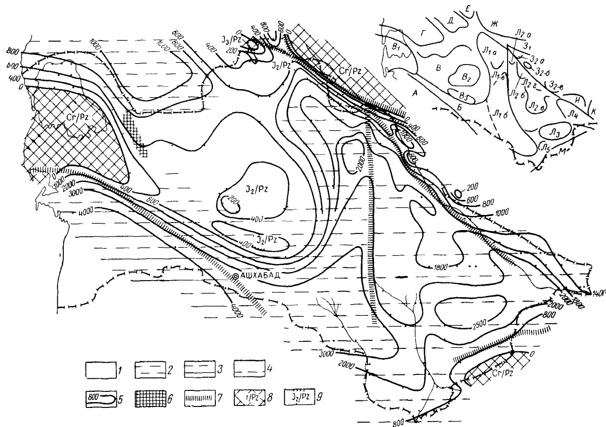
Рис. 6 Схема распространения литологических комплексов и структурных элементов ранне- и среднеюрского времени
