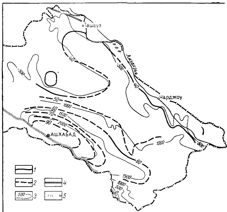
Рис. 39. Схематическая карта геонизотерм Каракумского артезианского бассейна по кровле водоносного комплекса верхнемеловых отложений 1 — геонизотермы достоверные, 2 — геонизотермы предполагаемые; 3 — стратонизогипсы кровли водоносного комплекса, 4 — тектонические нарушения, 5 — граница альпийской геосинклинальной области
