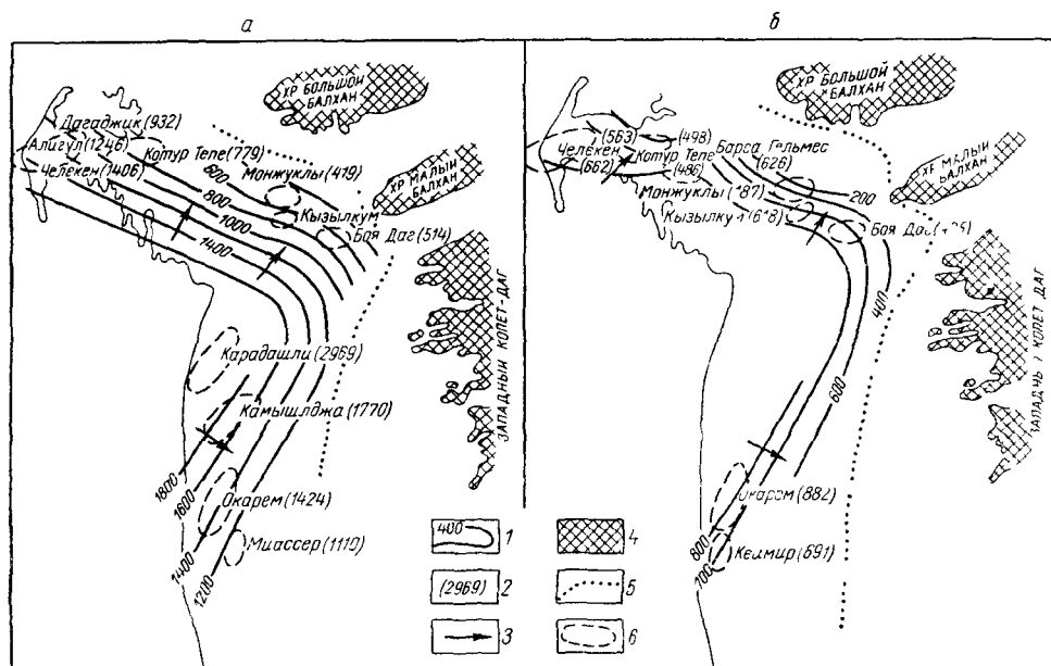
Рис 26 Схемы гидроизопьез нижней (а) и верхней (б) частей разреза водоносного комплекса среднеплиоценовых отложений (по В. В. Колодию, 1966)
