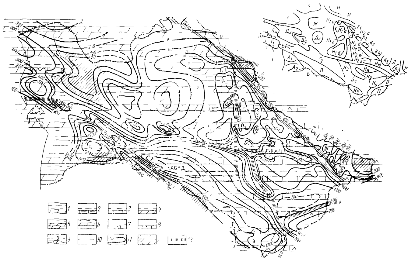
Рис 10. Схема распространения литологических комплексов и структурных элементов датского и раннеолигоценового времени
