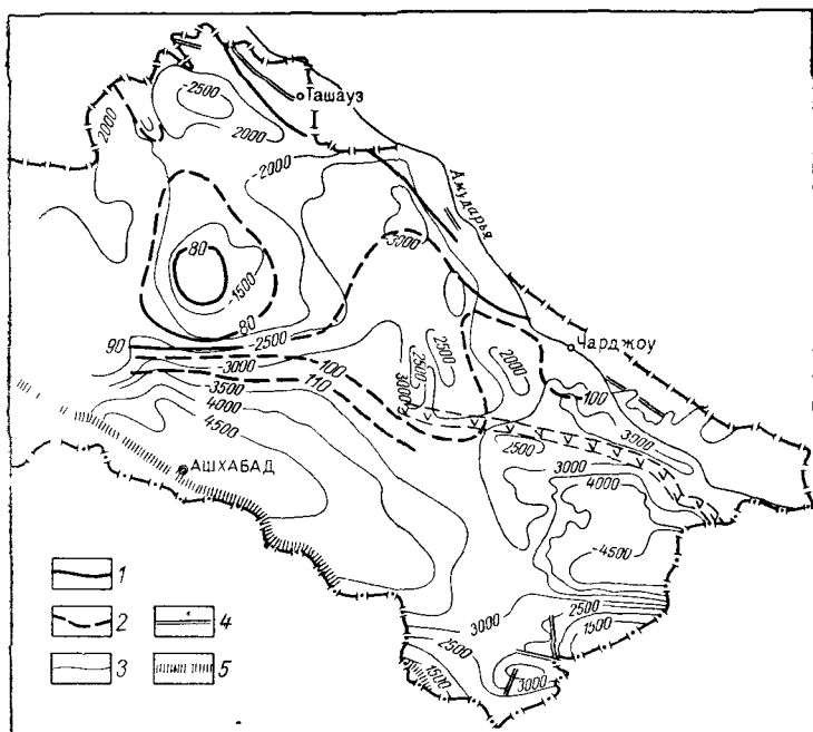
рис. 40. Схематическая карта геозотерм Каракумского артезианского бассейна по кровле водоносного комплекса юрских отложений 1 — геозотермы достоверные, 2 — геозотермы предполагаемые, 3 — стратонизогипсы водоносного комплекса, 4 — тектонические нарушения, 5 — граница альпийской геосинклинальной области
