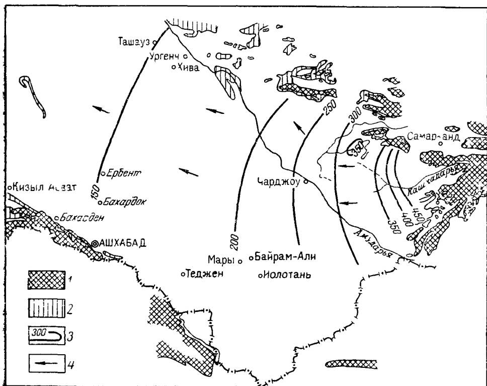
Рис 33 Схематическая карта гидроизопьез водоносного комплекса верхнемеловых отложений Каракумского артезианского бассейна
