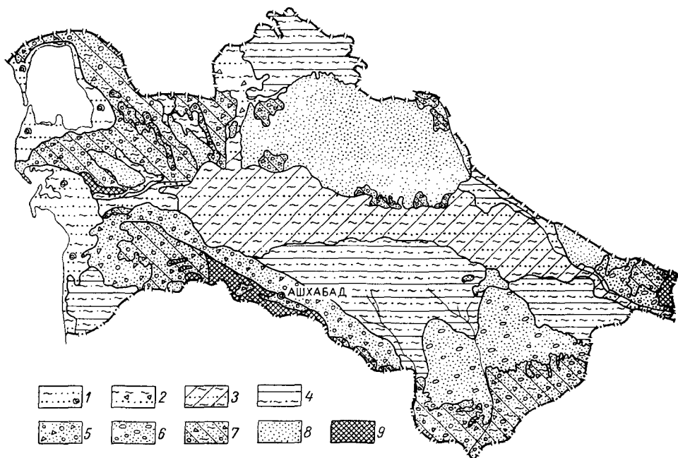
Рис. 12. Схема генетических типов четвертичных отложений (по Г. Бердыеву, 1965)
