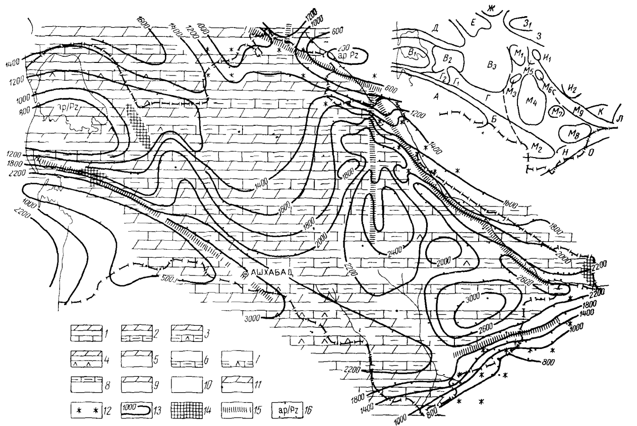
Рис 9 Схема распространения литологических комплексов и структурных элементов мелового периода
