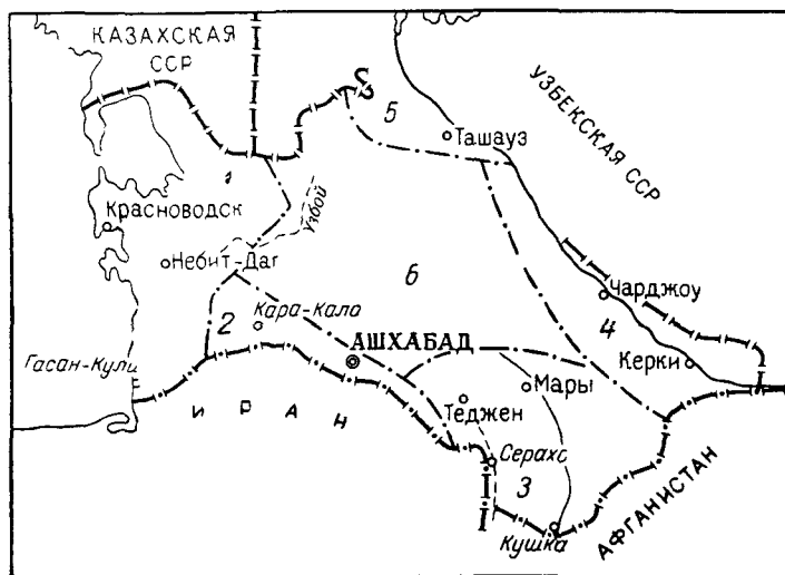
Рис. 1. Карта основных народнохозяйственных районов Туркменской ССР (по В. Б. Жмуйда)
