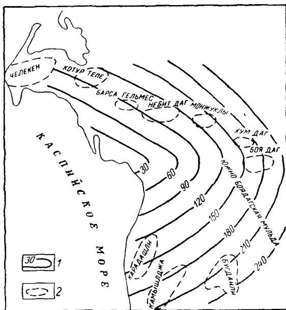
Рис. 24. Схема минерализации подземных вод апшеронских отложений (составил А. Акмамедов) 1 — изогалы минерализации, г/л, 2 — геологические структуры
