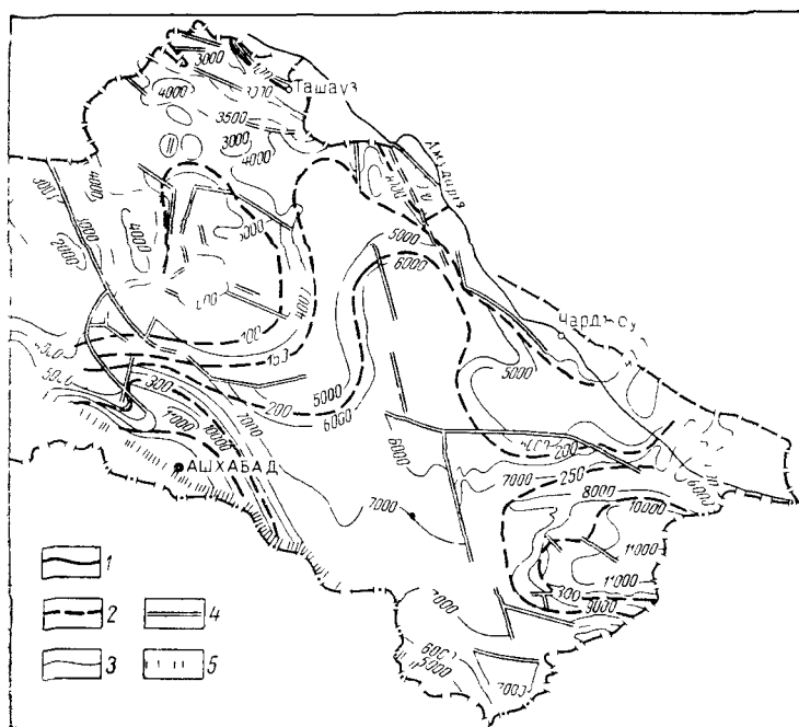
рис. 41. Схематическая карта геозотерм Каракумского артезианского бассейна по кровле складчатого фундамента 1 — геозотермы достоверные, 2 — геозотермы предполагаемые, 3 — стратонизогипсы водоносного комплекса, 4 — тектонические нарушения, 5 — границы геосинклинальной области
