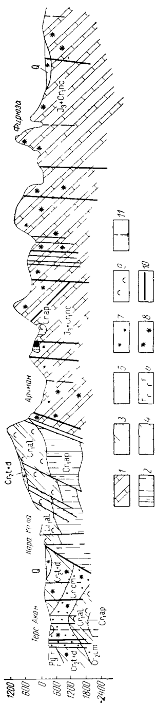
Рис. 29. Схематический гидрогеологический разрез через Копет-Даг
