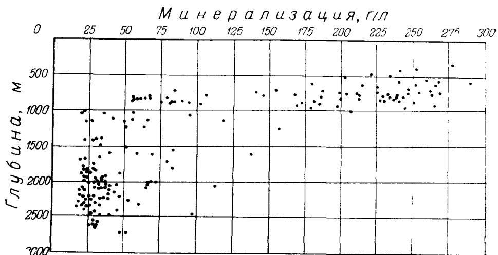
Рис. 21. Зависимость минерализации подземных вод Челекена от глубины залегания
