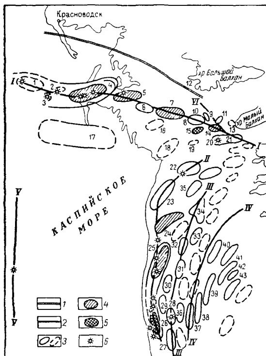
Рис 19. Схема расположения глубинных разломов и локальных структур в Западно-Туркменской впадине (по Н. С. Бескровному и др., 1963)
