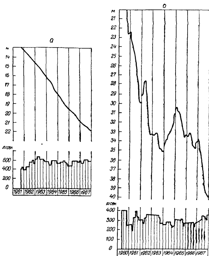
Рис. 46. Графики изменения уровня воды в районе развития искусственного дренирования или эксплуатации подземных вод а — режим искусственного дренирования или эксплуатации подземных вод по скв. 366, б — то же, по скв. 561
