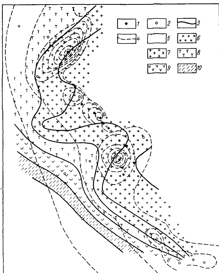
Рис. 61. Схема минерализации подземных вод в районе Джебельского водозабора
