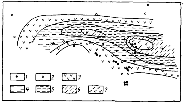
Рис. 59. Схема снижения уровня подземных вод на участке Секиязьского конуса выноса
