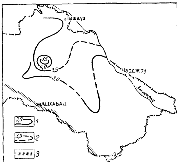
Рис. 42. Схематическая карта геотермического градиента осадочной толщи Каракумского артезианского бассейна 1 — изолинии геотермического градиента достоверные; 2 — изолинии градиента предполагаемые; 3 — граница альпийской геосинклинальной области
