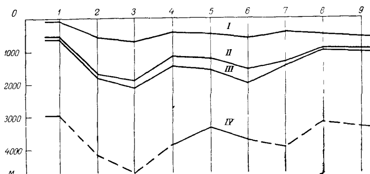
Рис. 20. Распределение мощностей плиоценовых отложений в Юго-Западной Туркмении
