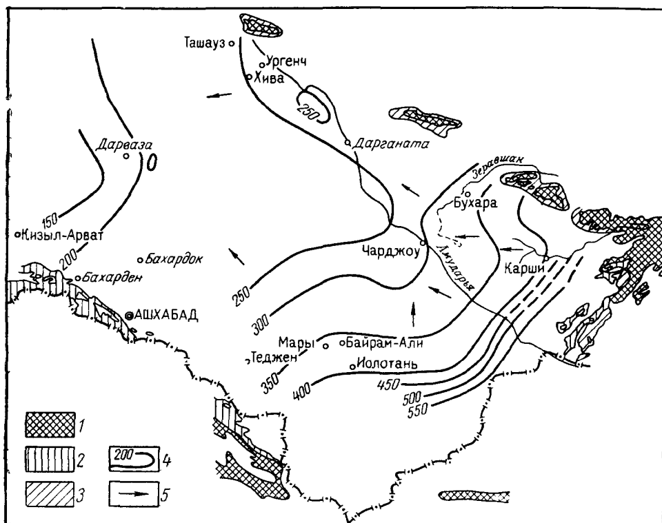
Рис. 32. Схематическая карта гидроизопьез водоносного комплекса нижнемеловых отложений Каракумского артезианского бассейна
