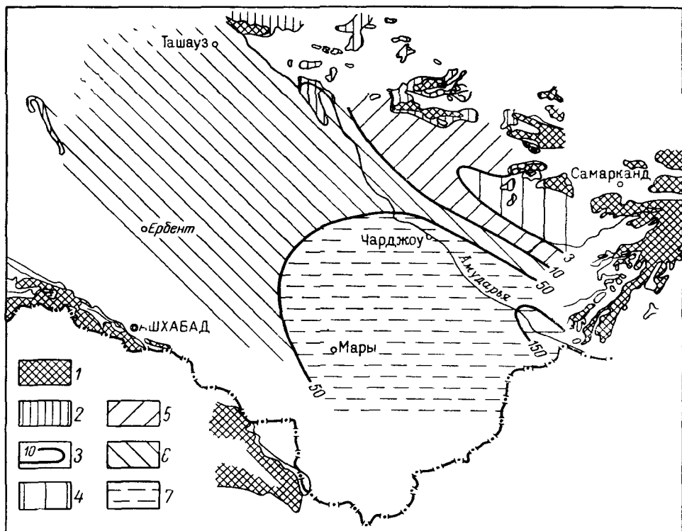
Рис. 36. Схематическая гидрохимическая карта водоносного комплекса верхнемеловых отложений Каракумского артезианского бассейна
