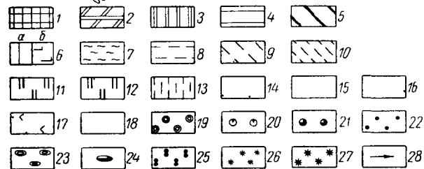
1 — водоносный комплекс верхнепалеозойских и триасовых отложений 2 — водоносный комплекс нижних и среднеюрских отложений 3 — водоносный комплекс верхних юрских отложений, 4 — водоносный комплекс отложений неомока 5 — водоносный комплекс айсиклинских и сеноманских отложений, тогда а — водопроницаемая и безводная (сдренированная) туркских сеноманских и датских отложений б — водоупорная туркских сеноманских и датских отложений, в — водоупорная толща палеогена 6 — водоносный комплекс средние и верхнемiocеновые отложений, 9 — водопроницаемые и безводные (сдренированные) средние и верхнемiocеновые отложения 10 — водоносный комплекс верхнего миоцена — нижнего плицена 11 — водоносный комплекс акчагыльских отложений 12 — водопроницаемые и безводные (сдренированные) акчагыльские отложения 13 — водоносный комплекс апшеронских отложений 14 — водоносный комплекс нижние и средние четвертичных отложений (каракумская свита) 15 — водоносный комплекс пролювиальных чегвертинных отложений 16 — водоносный комплекс хазарских и хвалынских отложений, 17 — водопроницаемые, но безводные (сдренированные) хвалынские отложения 18 — водоносный горизонт морских новокаспийских отложений Минерализация подземных вод 19 — воды хлоридные натриевые разной минерализации 20 — воды хлоридные натриевые (10–30 г/л) 21 — воды хлоридные натриевые (50–150 г/л) 22 — воды хлоридные натриевые (более 150 г/л) 23 — воды хлоридно сульфатные натриевые разной минерализации, 24 — воды хлоридно сульфатные натриевые (2–34 г/л), 25 — воды хлоридно сульфатные натриевые (50–150 г/л) 26 — воды хлоридно сульфатные натриево-магниевого (более 150 г/л), 27 — воды смешанного состава (до 1 г/л) 28 — направление движения подземных вод первого от поверхности земли водоносного комплекса
