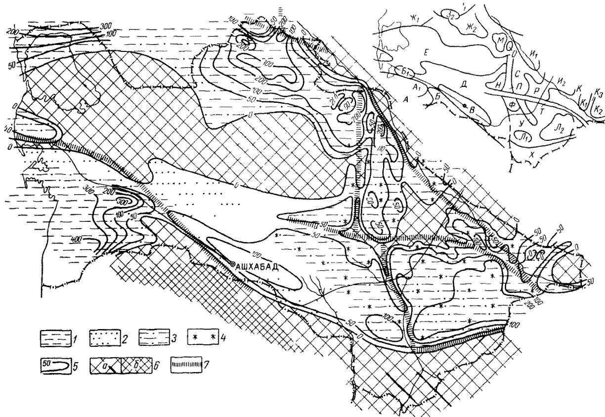
Рис. 11. Схема распространения литологических комплексов и структурных элементов среднеолигоценового и раннемиоценового времени
