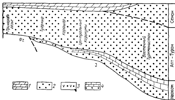
Рис. 8 Соотношение литологических комплексов мелового периода 1 — глинисто-карбонатный, 2 — терригенный, 3 — сульфатно карбонатно терригенный, 4 — карбонатно терригенный
