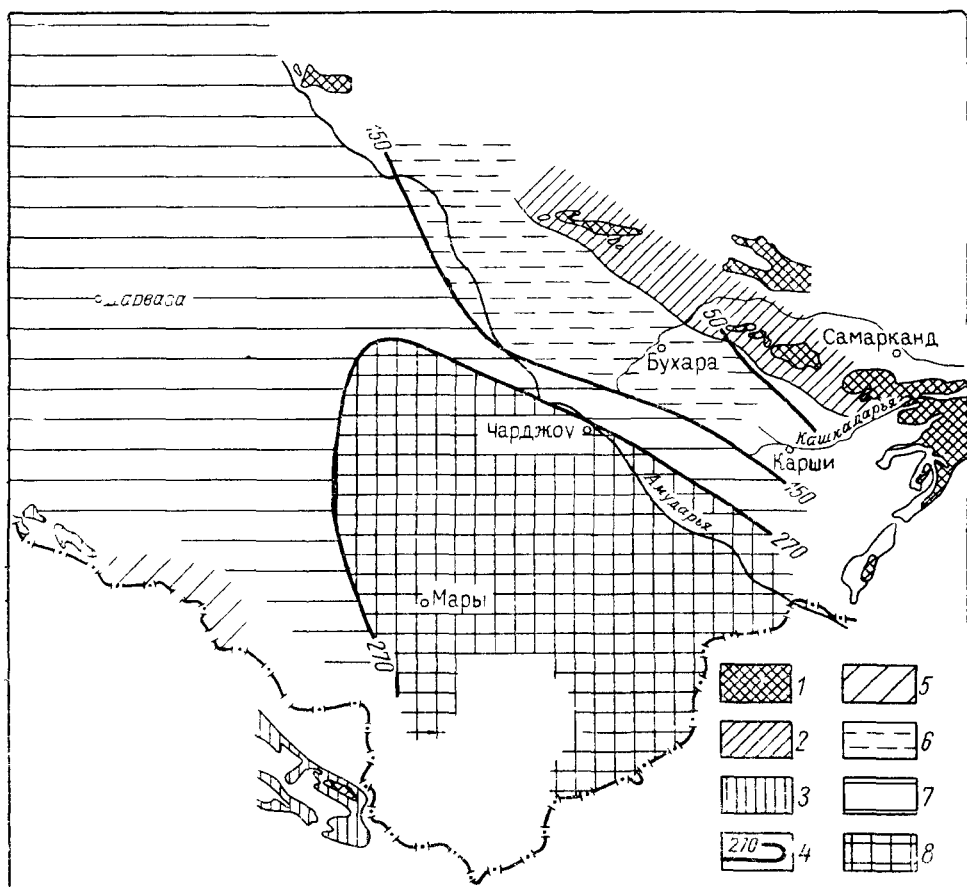
Рис 34. Схематическая гидрохимическая карта водоносного комплекса юрских отложений Каракумского артезианского бассейна
