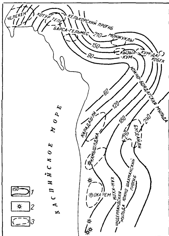
Рис. 23. Схема минерализации подземных вод верхней части разреза среднеплиоценовых отложений (составил А. Акмамедов)
