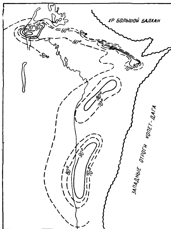
Рис. 27. Схема геонизотерм Западно-Туркменского артезианского бассейна на глубине 2000 м ниже уровня моря (по С. С. Джибути, 1962)
