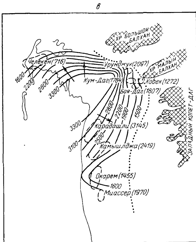
Рис. 25. Схемы гидродинамической обстановки нижней части разреза среднеплиоценовых отложений на начало ачкагыльского (а), апшеронского (б) и бакинского (в) времени
