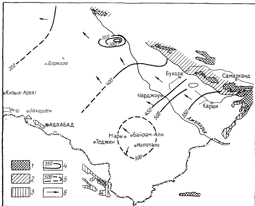
Рис. 31. Схематическая карта гидроизопьез водоносного комплекса юрских отложений Каракумского артезианского бассейна
