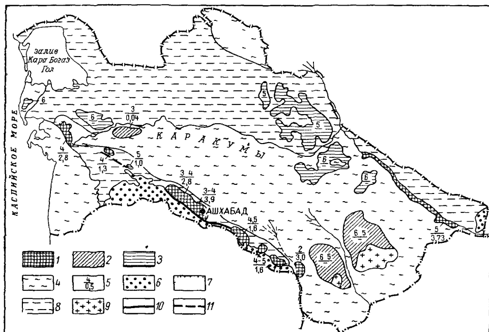
Рис. 53. Схематическая карта прогнозных эксплуатационных запасов пресных и слабосолоноватых подземных вод Туркменской ССР (составила Р. Н. Клышникова)
