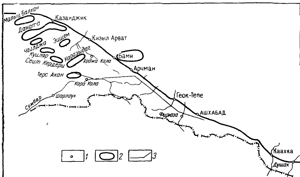
Рис 28 Схематическая карта фактического материала по складчатой области Копет-Дага (составил А. В. Кудельский)
