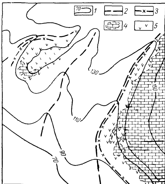
Рис 44 Схема пьезометрической поверхности водоносного комплекса верхнеюрских известняков (по В. Н. Озябкину)
