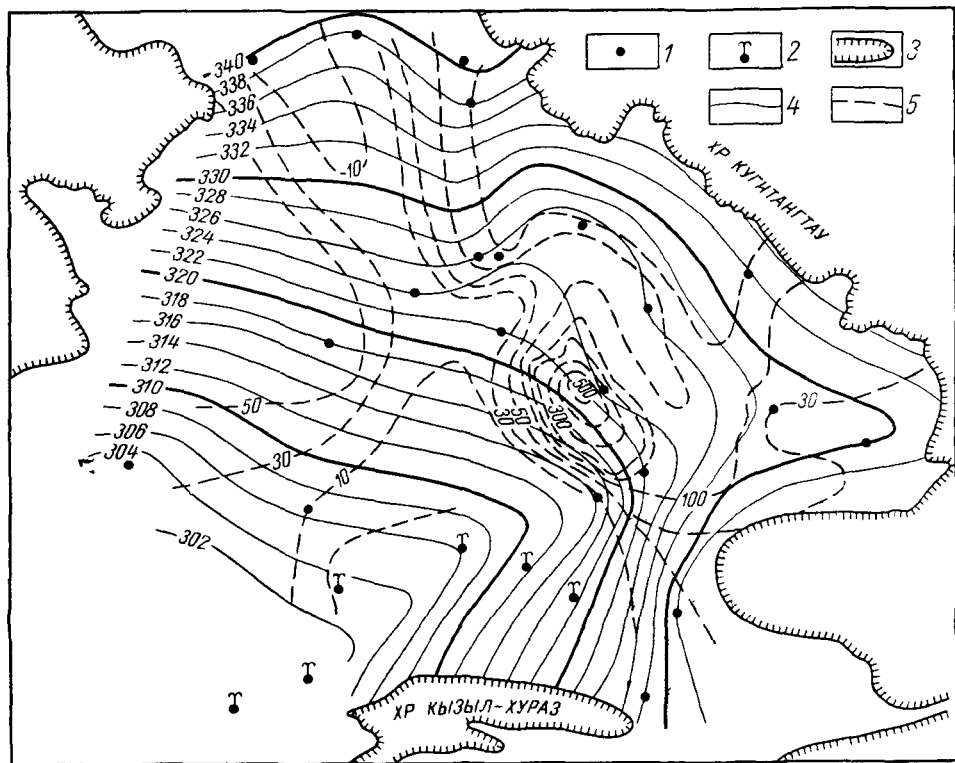
Рис 45. Карта гидроизогипс и скоростей движения вод карлюкского водоносного горизонта в гравийно-галечных отложениях (по В. Н. Озябину)
