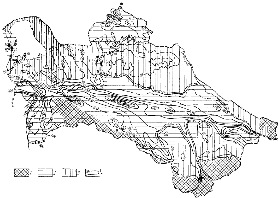
Рис. 13. Схема распределения мощностей четвертичных отложений (по Г. Бердыеву, 1965)
