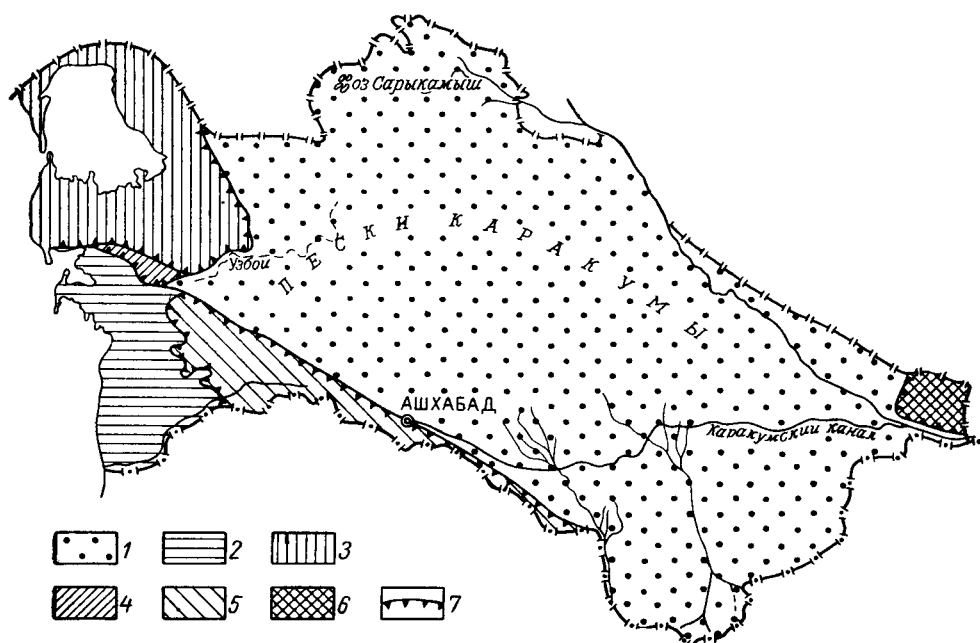
Рис. 16. Схема гидрогеологического районирования территории Туркменской ССР
