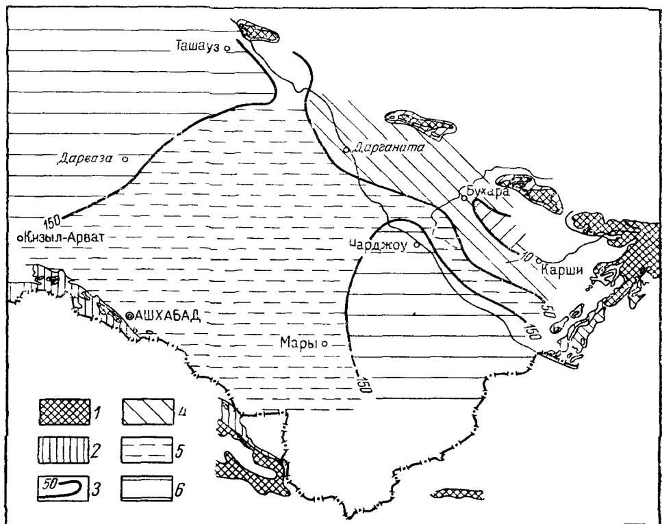
Рис. 35. Схематическая гидрохимическая карта водоносного комплекса нижнемеловых отложений Каракумского артезианского бассейна
