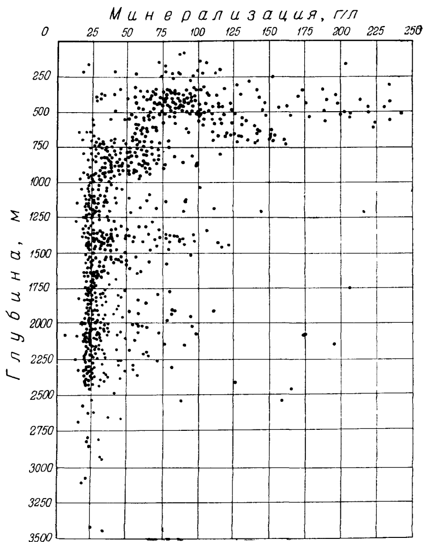
Рис. 22. Зависимость минерализации подземных вод Небит-Дага от глубины залегания
