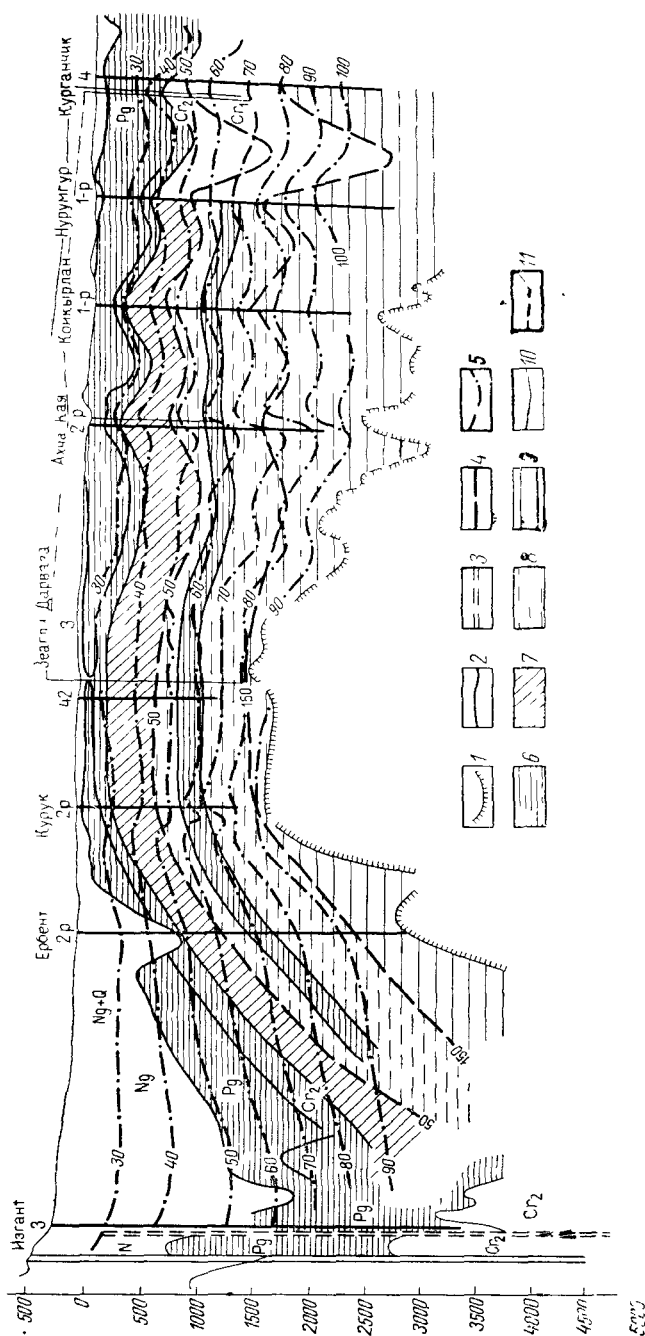
Рис. 37. Гидрогеологический разрез по линии Тахтакаирский вал — Колет-Дог 1 — поверхность фундамента; 2 — стратиграфические границы; 3 — тектонические нарушения; 4 — изоминеры; 5 — изотермы; 6 — водоупорная толща; 7 — зоны распространения 7 — подземных вод с минерализацией от 10 до 50 мг/л; 8 — слабых рассолов с минерализацией подземных вод от 50 до 150 г/л; 9 — крепких рассолов с минерализацией подземных вод от 150 до 270 г/л; 10 — линия падения напора приведенных напоров водоносного комплекса юрских отложений; 11 — линия падения напора приведенных напоров нижнемелового водоносного комплекса
