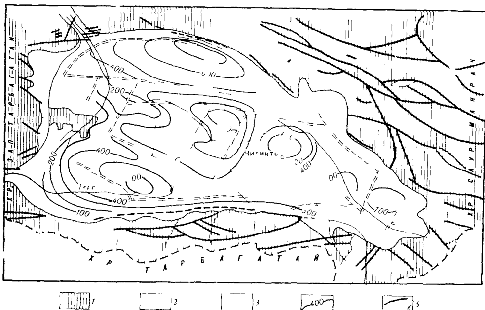
Рис. 24 Структурная схема Чиликтинского артезианского бассейна (составлена по материалам И. В. Климовской)
