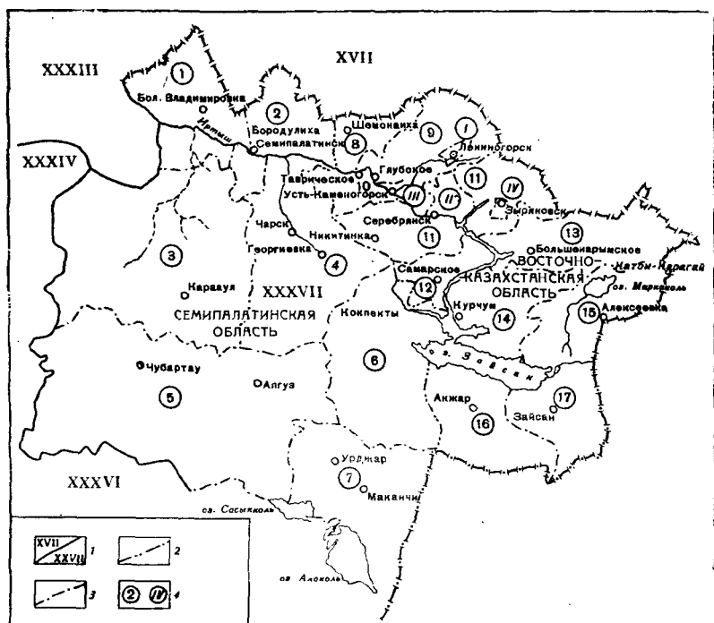
Рис. 1. Обзорная карта Восточного Казахстана (составил В. И. Белянин)
