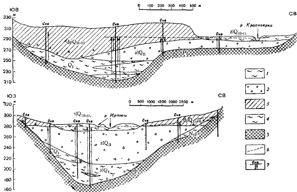
Рис. 21 Гидрогеологические разрезы долины р. Красноярки выше ст. Предгорное и долины р. Иртыша у г. Усть-Каменогорска (составил В. И. Белянин)
