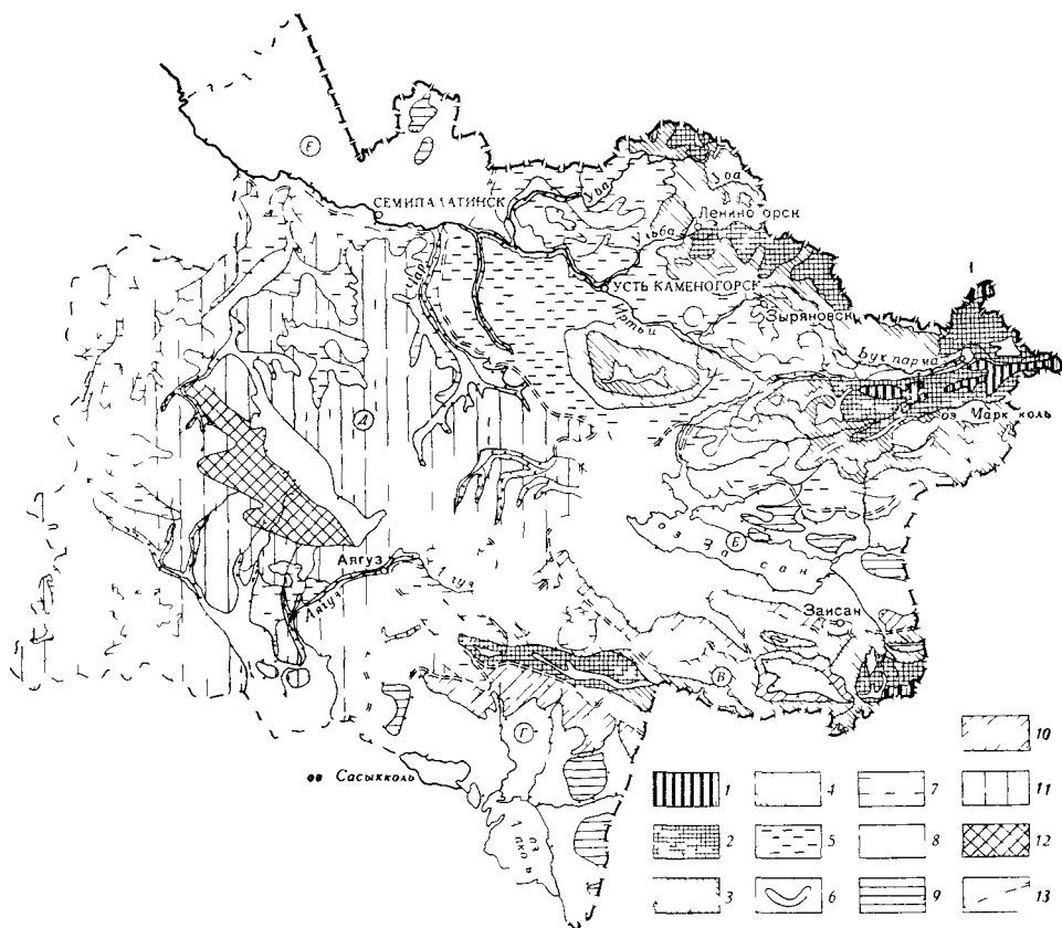
Рис. 2. Схема геоморфологического районирования Восточного Казахстана (составил В. С. Ерофеев)
