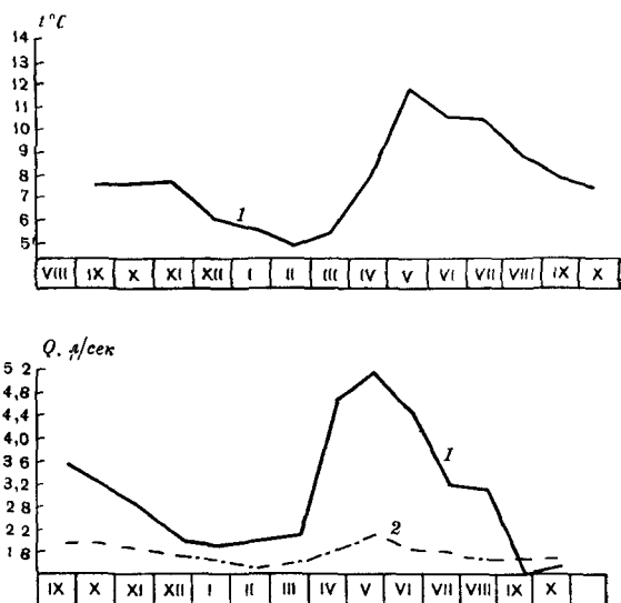
Рис 34 График колебаний температуры и расходов грунтовых трещинных вод по родникам из осадочных пород палеозоя в центральной части Калбинского хребта (составила Г. Х. Казовская) 1 — родник № 5, 2 — родник № 15
