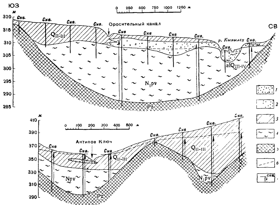
Рис. 22 Гидрогеологические разрезы долины р. Кызылсу в створе с Чалобай и р. долины Антипова ключа к западу от пос. Белоусовка (составил В. И. Белянин)
