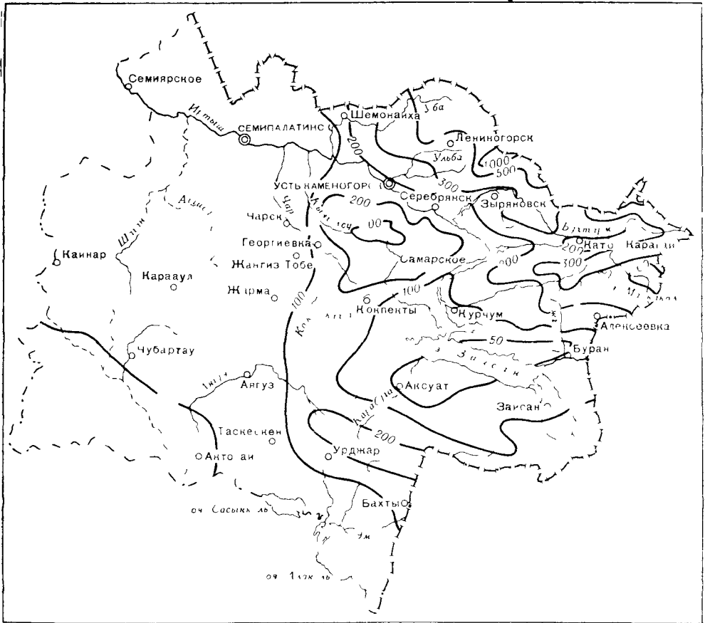
Рис. 11 Карта распределения твердых осадков в изотиниях стоя воды в мм (по Р. И. Гальперину)
