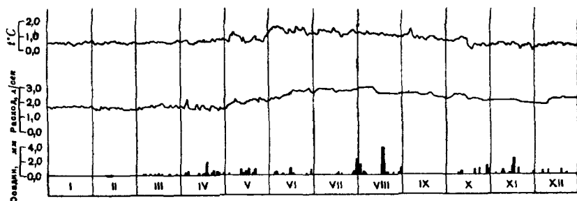
Рис. 33 Совмещенные графики колебаний количества осадков, расходов и температуры грунтовых трещинных вод из палеозойских гранитов в центральной части Калбинского хребта (составила Г. Х. Казовская)
