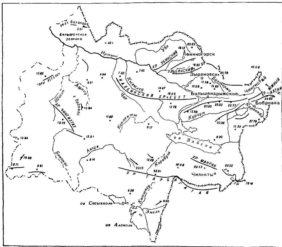
Рис. 3 Орографическая схема Восточного Казахстана (составила Т. Г. Егорова)
