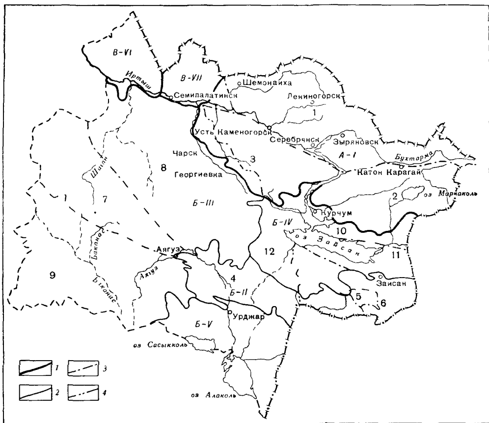
Рис. 18. Схема гидрогеологического районирования Восточного Казахстана (составлена Б. Е. Антыпко)
