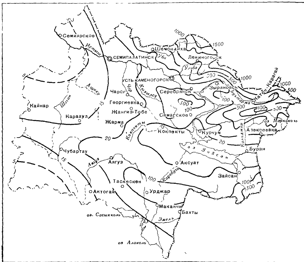
Рис. 12 Карта среднегодового поверхностного стока в изолиниях слоя воды в мм (по И. С. Соседову и З. Т. Беркалиеву)
