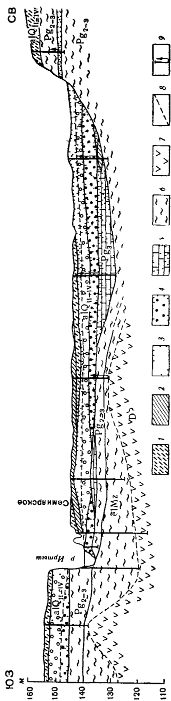
Рис 29 Геологический разрез долины р Иртыша в районе сел Семирское—Майское (составил С М Мухамеджанов) 1 — супеси пылеватые, 2 — суглинки, 3 — песок изредка гравелистый, 4 — гравийно-галечные отложения, 5 — гравийно-галечные отложения, 6 — глина плотная, иногда с лигнитом, 7 — кварцевые порфиры и порфиры, 8 — уровень грунтовых вод, 9 — палеометрические уровни по скважинам
