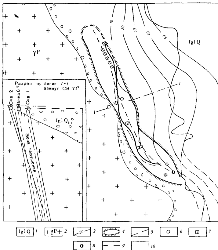
Рис 38 Схематическая гидрогеологическая карта участка выходов Рахмановских ключей (составил В. И. Белянин)
