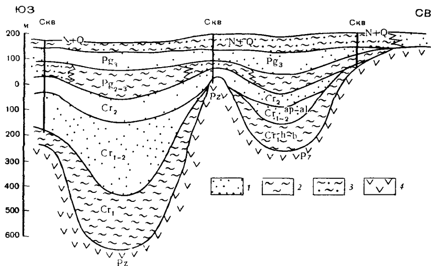
Рис. 30 Схематический геолого-гидрогеологический разрез Иртышского артезианского бассейна по линии I—I (составила Б. Е. Антипко)
