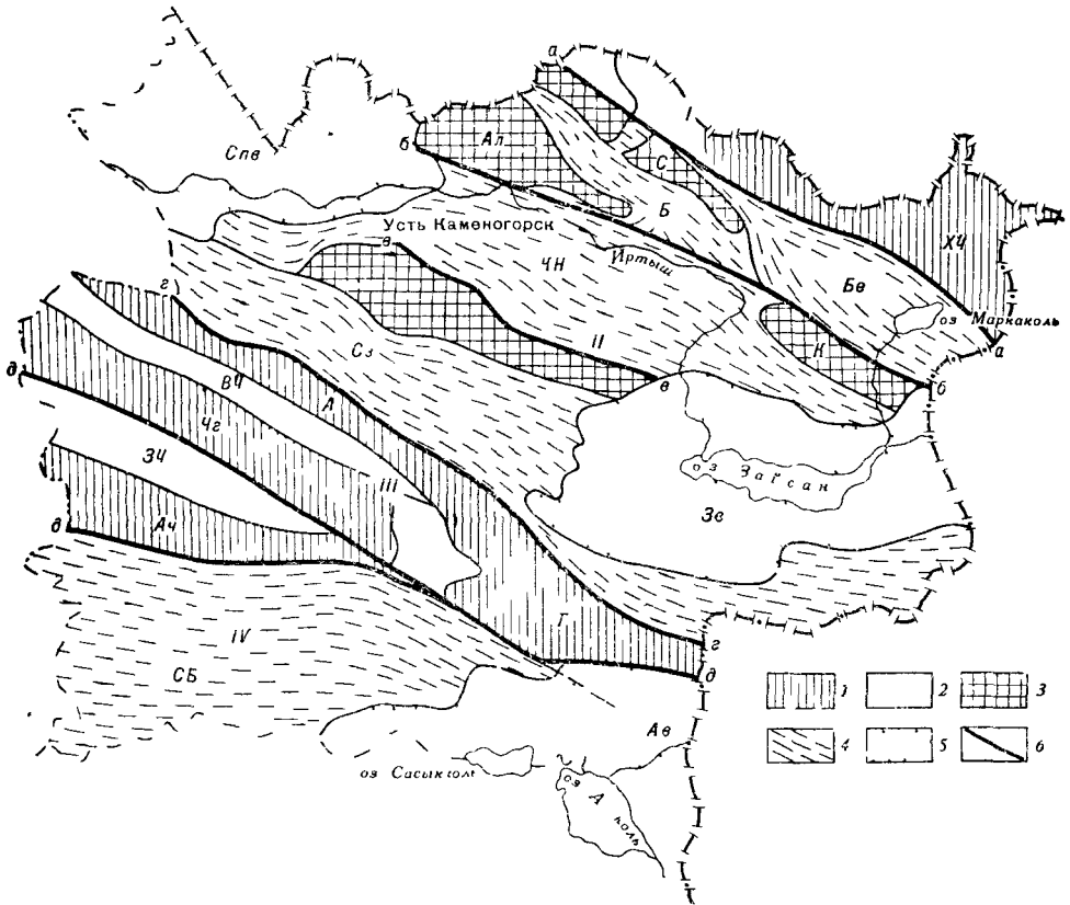
Рис. 15. Схема основных структур палеозоя Восточного Казахстана (составил В. С. Ерофеев по материалам Н. А. Афоничева, Р. А. Борюкаева, П. Ф. Иванкина, В. П. Нехорошева, Г. Ф. Яковлева).
