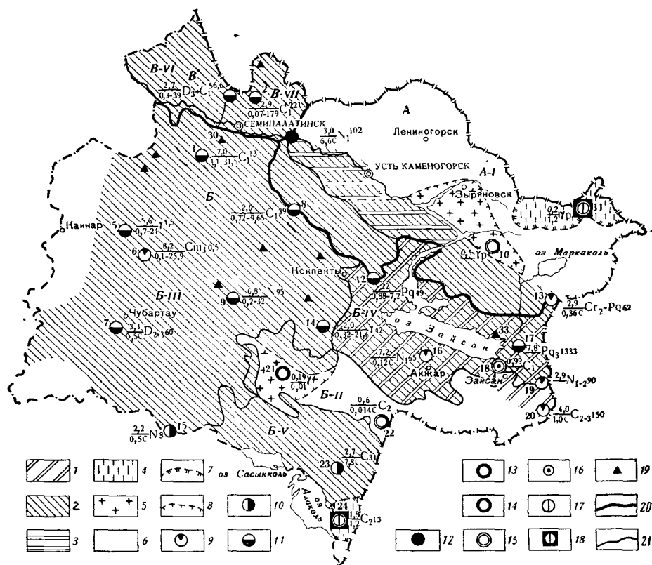
Рис. 37. Схематическая карта распространения минеральных вод и лечебных грязей Восточного Казахстана (составила А. Б. Авдеева)
