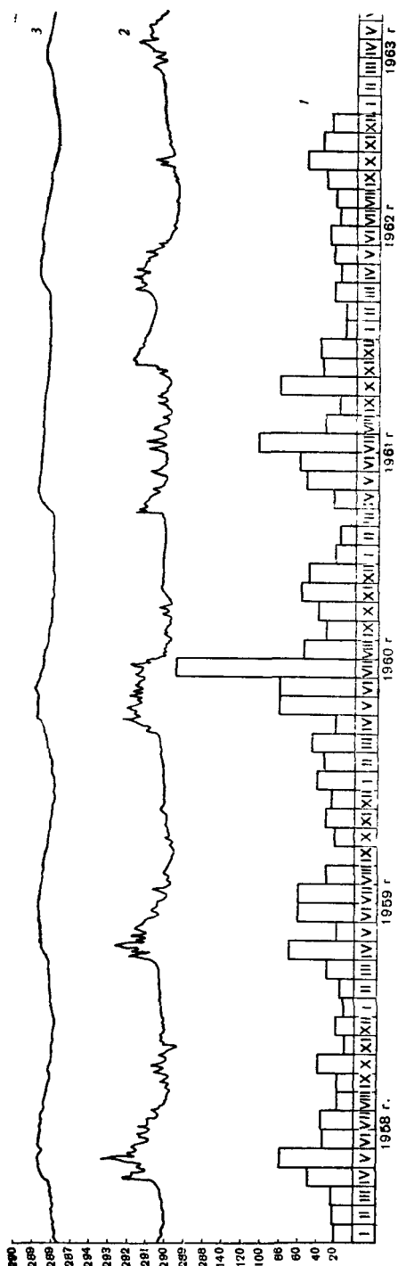
Рис. 36 Совмещенные графики колебаний количества атмосферных осадков, уровня грунтовых вод и поверхностного водотока р. Убы (составила Г. Х. Казовская) 1 — среднемесячное количество атмосферных осадков в мм, 2 — уровень воды в р. Убе, 3 — уровень грунтовых вод по скважине в долине реки
