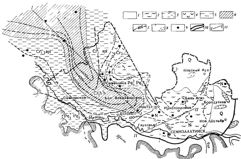
Рис 28 Схематическая карта отложений, залегающих на складчатом палеозойском фундаменте в пределах Ишим Иртышского артезианского бассейна (составила Б. Е. Антыпко)
