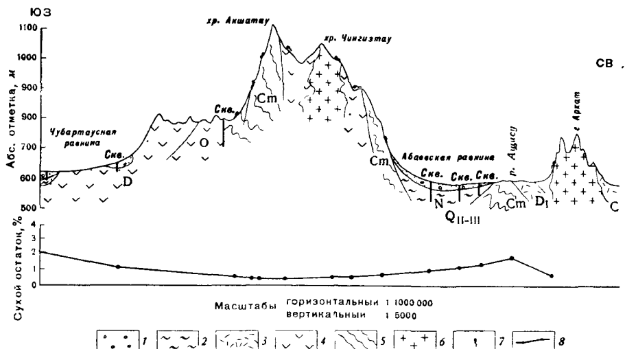
Рис. 26. Геолого-гидрогеологический разрез через Чингизский хребет (Чингиз-Жарминско-Балхашский район) (составил Ф. К. Кабиев)
