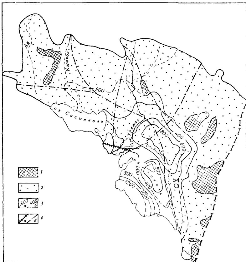
Рис. 27. Тектоническая схема Алакольского артезианского бассейна (составил С. М. Мухамеджанов)
