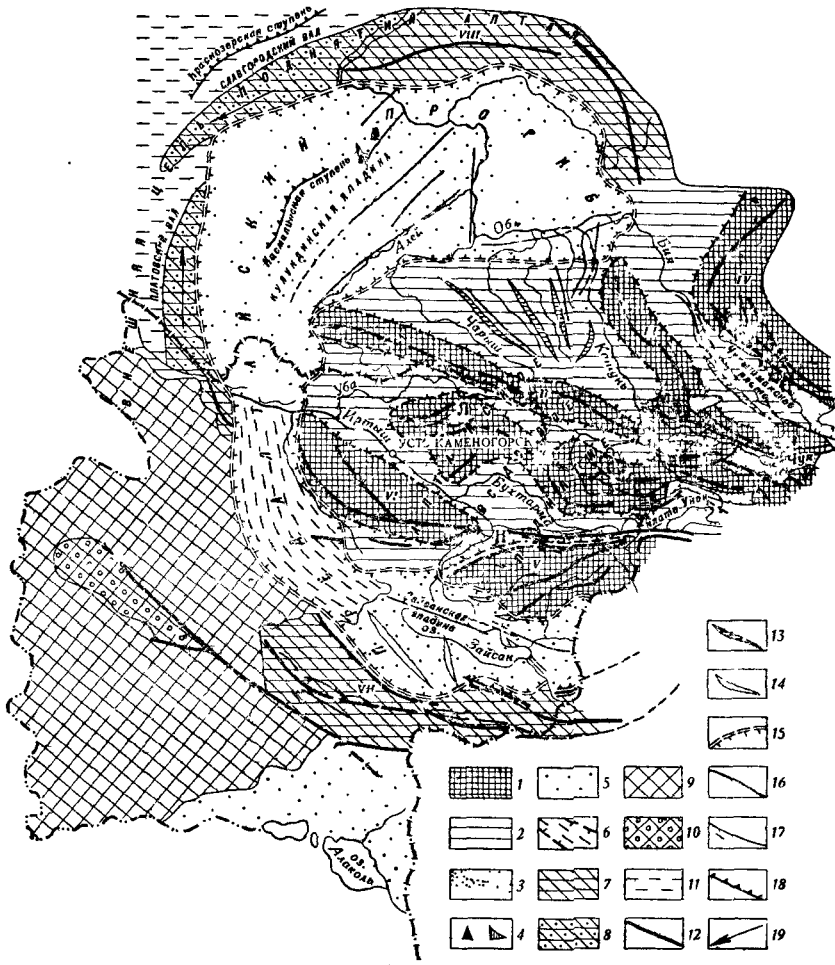
Рис. 16. Схема альпийской тектонической структуры Алтая (составил В. С. Ерофеев)
