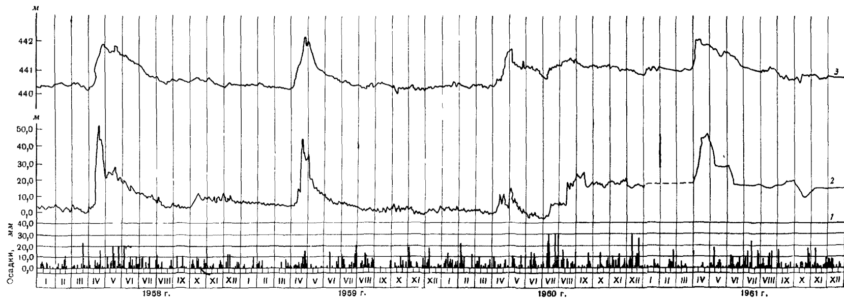
Рис 35. Совмещенные графики колебаний количества атмосферных осадков, уровней грунтовых вод и поверхностного водотока р Березовки (составила Г. Х. Казовская)
