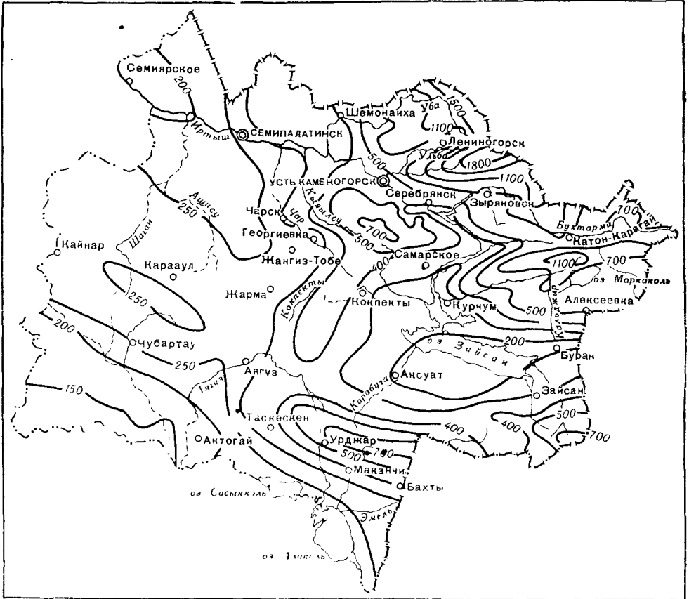
Рис. 10. Карта распределения годовых сумм осадков в изолиниях слоя воды в мм (по И. С. Соседову и Р. И. Гальперину)
