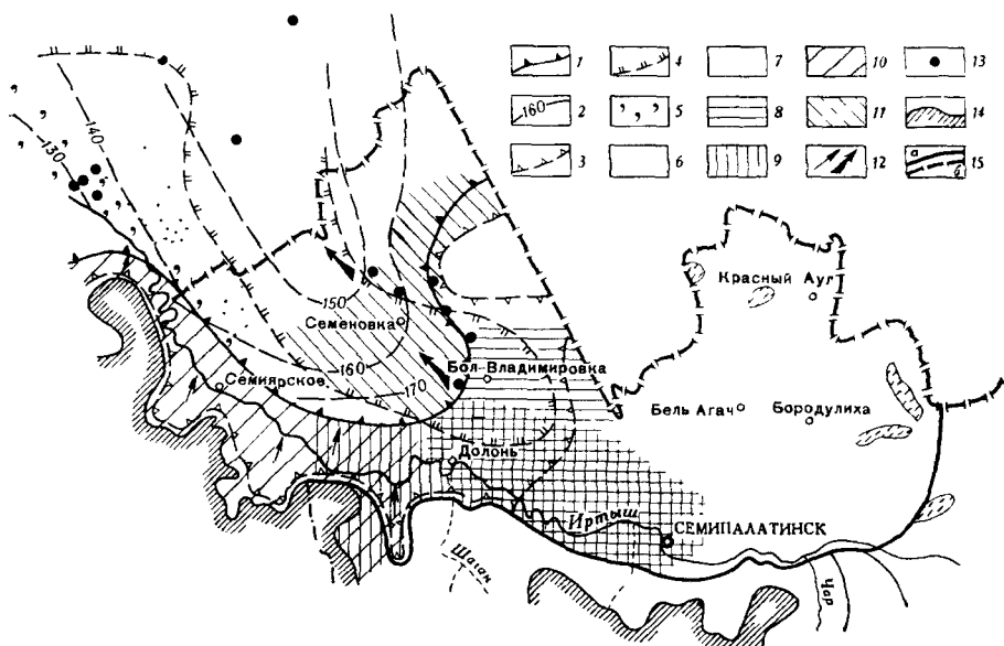
Рис 31. Схематическая гидрогеологическая карта водоносного комплекса нерасчлененных меловых отложений Иртышского артезианского бассейна (составила Б. Е. Антыпко)
