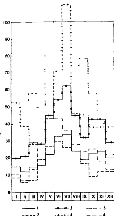
Рис. 9 Сопоставление внутригодового распределения осадков по постам на блюдений (составил И. В. Токарев) 1 — Семипалатинск 2 — Аксуат 3 — Усть-Каменогорск 4 — Маркаколь 5 — Лениногорск 6 — Зайсан
