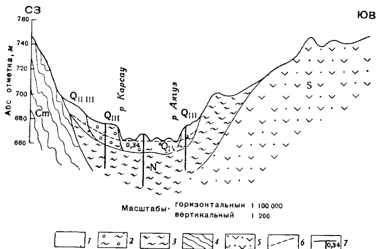
Рис 25 Геолого-гидрогеологический разрез р. Аягуз выше г. Аягуз (Чингиз-Жарминско-Балхашский район) (составил Ф. К. Кабиев)
