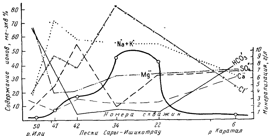
Рис. 51. Гидрохимический профиль между речью Или и Каратаем (составила С. В. Шорина)
