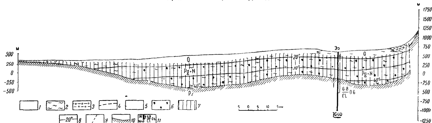
Рис. 66. Гидрогеотермический разрез через Восточно-Чуйскую и Западно-Чуйскую впадины по линии IV—IV (составили О. М. Дырдин и Г. Р. Алещенко)
