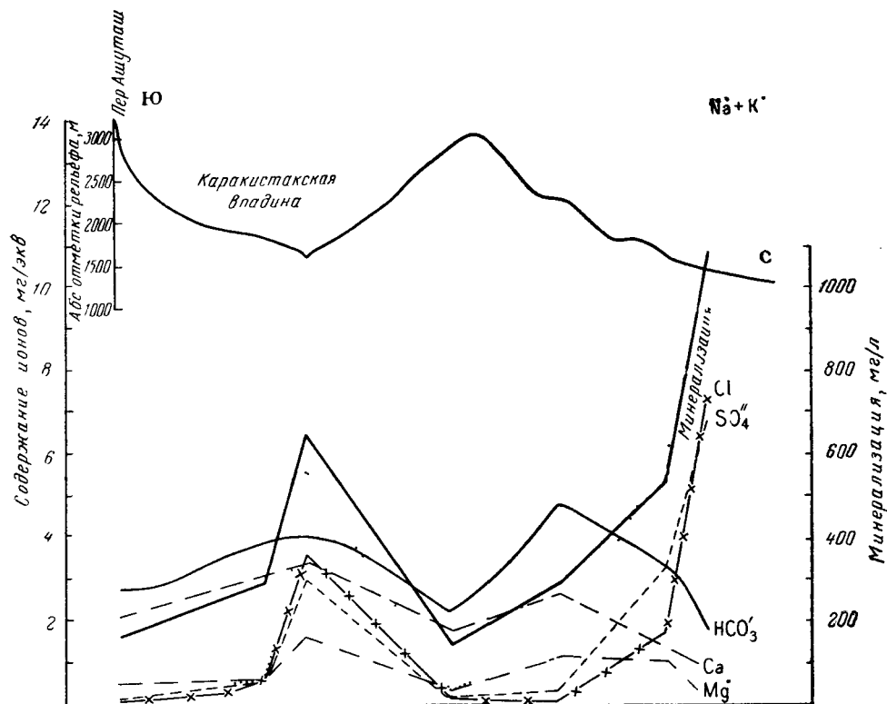
Рис 33 Схематический гидрохимический разрез по Киргизскому хребту (составила А А Мухоряпова)
