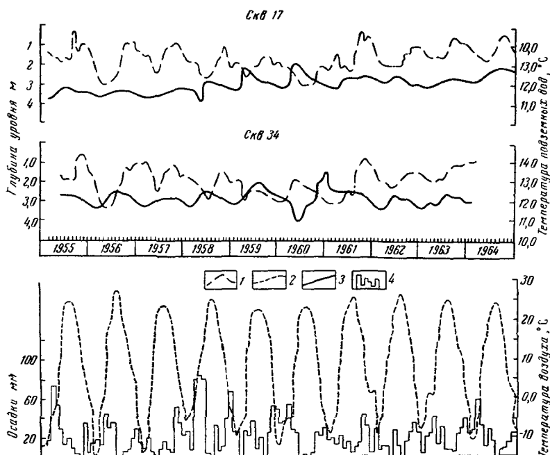
Рис. 83 График изменения уровня и температуры подземных вод междуречья Чу—Курагаты (составили Е. Н. Алексин и А. Ж. Джакелов)
