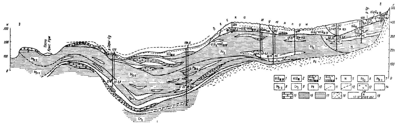
Рис 26. Схематический гидрогеологический разрез вдоль Западно-Чуйского артезианского бассейна (составили Н. Ф. Федин, И. Б. Даденкова)
