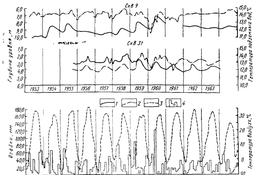
Рис. 82. График колебаний уровня и температуры грунтовых вод правобережья долины р. Чу в ее средней части (составили Е. Н. Алексини и А. К. Джаkelов) 1 — температура подземных вод; 2 — температура воздуха; 3 — уровень грунтовых вод; 4 — месячная сумма атмосферных осадков
