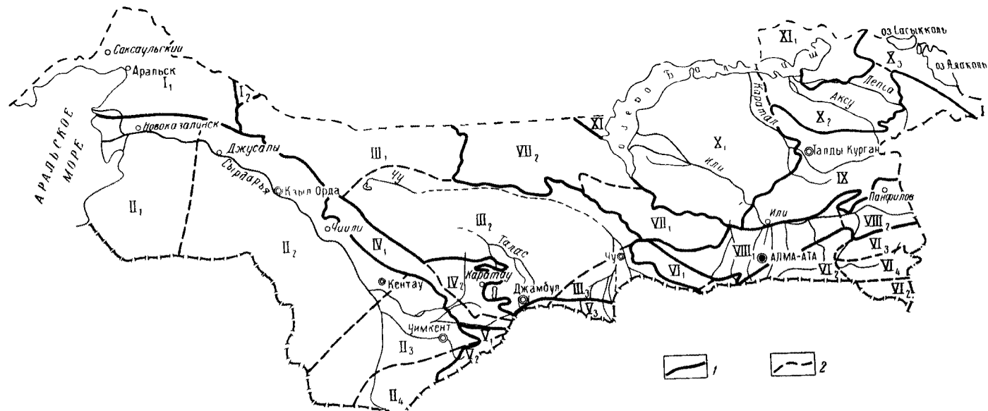
Рис. 14. Схема гидрогеологического районирования территории Южного Казахстана (составил В И Дмитриевский)
