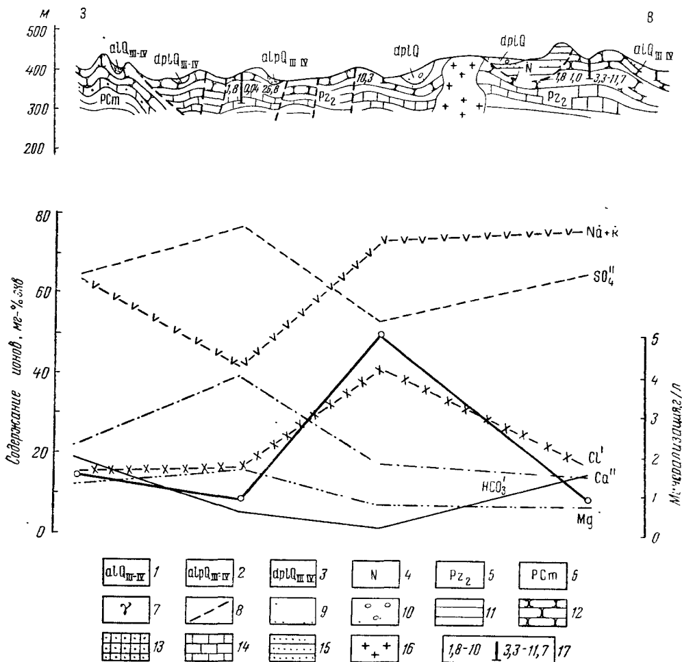
Рис. 53. Схематический геолого-гидрогеологический разрез вкострости долины временных водотоков (составил А. А. Толмачева)
