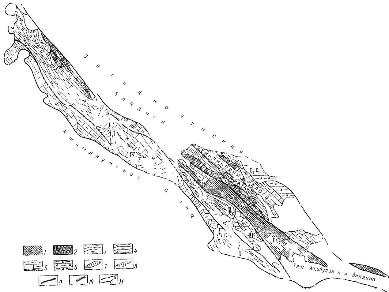
Рис 29 Схема структурно-тектонического строения Каратауской системы бассейнов трещинных вод (составила Г. А. Калмыкова по материалам А. Г. Новикова, Ф. Е. Снницына и др.)
