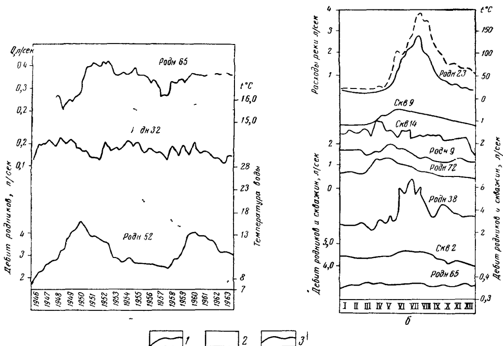
Рис. 73 График изменения режима грунтовых и напорных вод (составил А. Г. Голубь)
