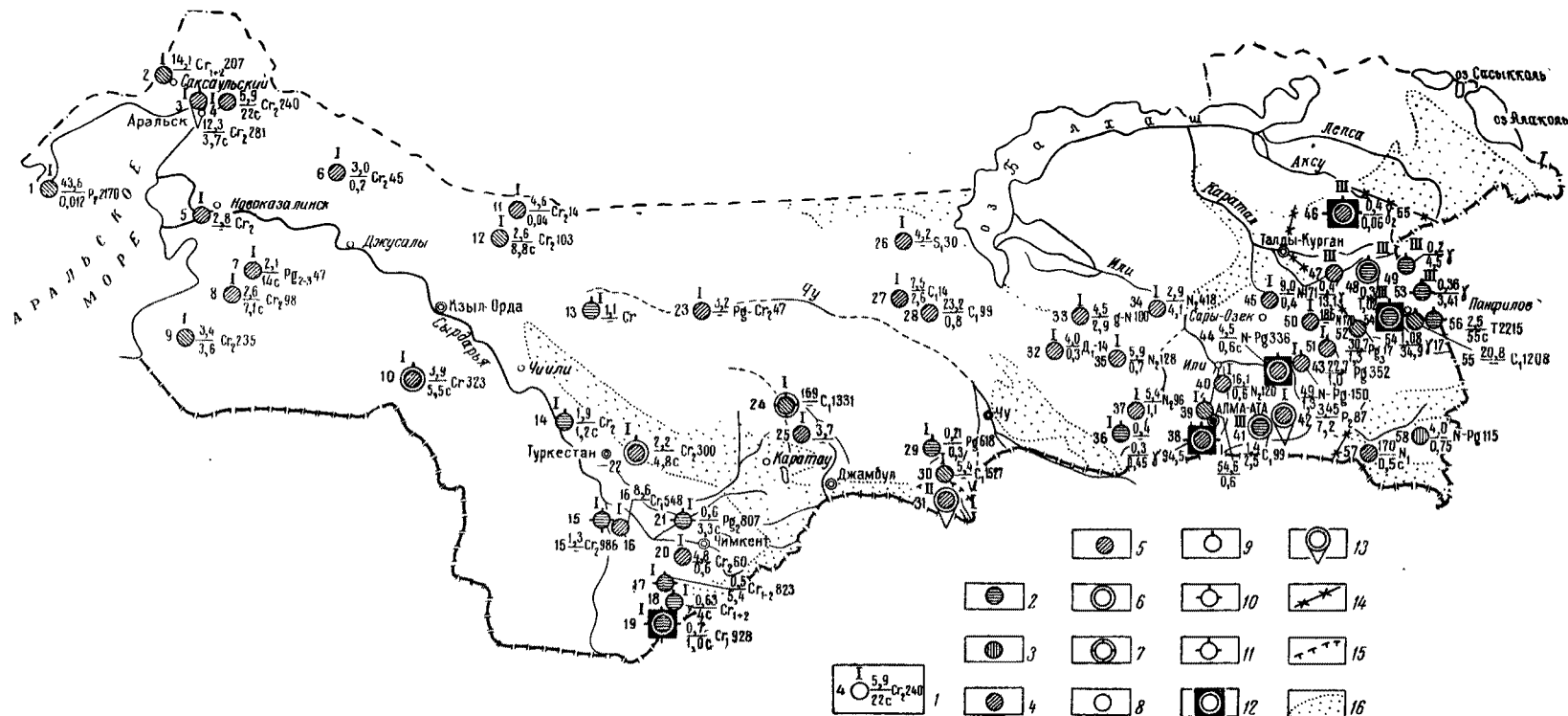
Рис. 70. Схематическая карта распространения минеральных вод на территории Южного Казахстана (составила А. Б. Авдеева)
