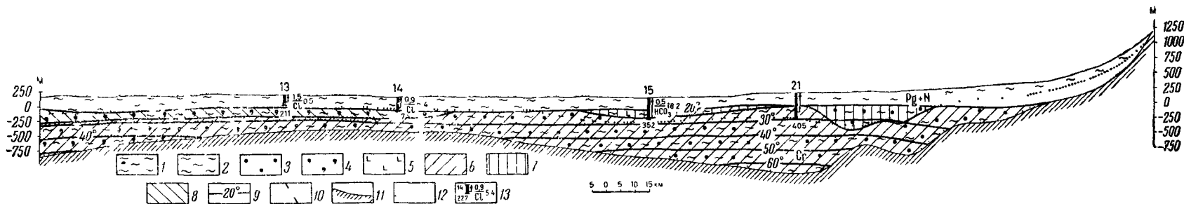
Рис. 65. Гидрогеотермический разрез через Сарысуйскую и Западно-Чуйскую впадины по линии III—III (составил Г. Р. Алещенко)
