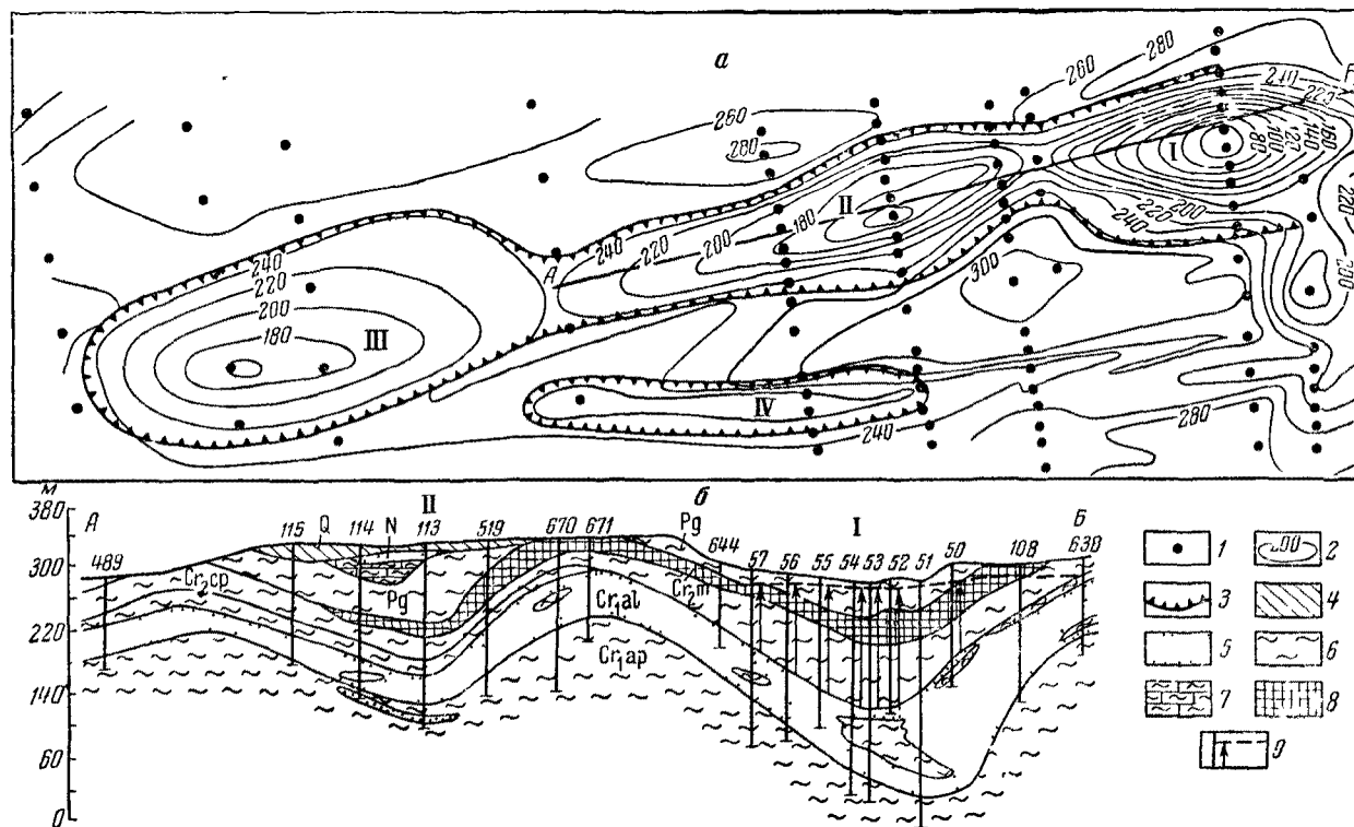
Рис 79 Схема муьды (а) (Сарбласской — I—II—III и Новоукраинской IV) и геологический профиль (б) по линии А—Б
