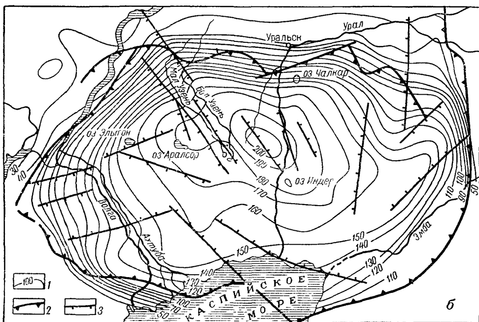
Рис. 70. Схематическая геотермическая карта Прикаспийской впадины а — на абс. отметке — 3000 м; б — по поверхности подсолевых отложений (по А. А. Алексину и Е. А. Дьяконовой, 1967) 1 — изотермы; 2 — борт Прикаспийской впадины; 3 — градиенты силы тяжести
