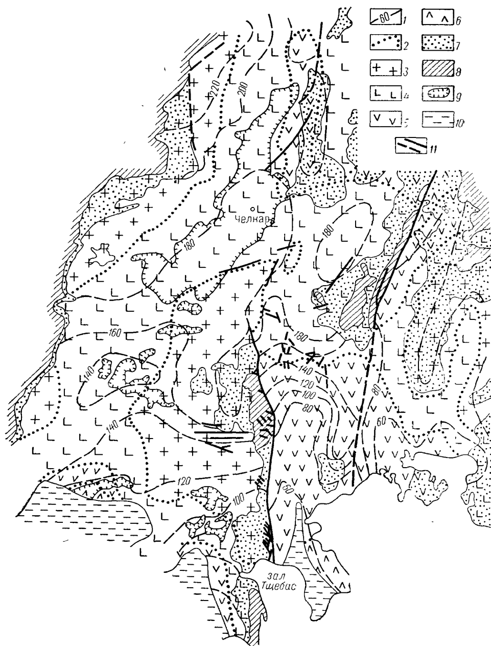
Рис. 42. Схематическая карта гидроизопьез и химического состава подземных вод верхнеэоценовых отложений Северного Приаралья. (Составили Г. Т. Давидович и Л. М. Онищенко)
