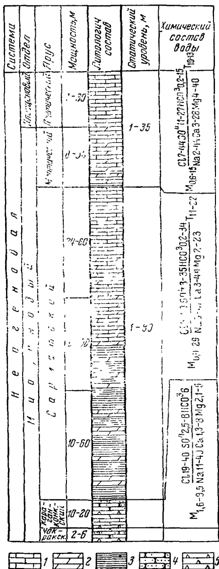
Рис. 47. Гидрогеологический разрез неогеновых отложений Южного Мангышлака. (Составили В. Б. Коллаков, Г. Н. Абдразакова):
