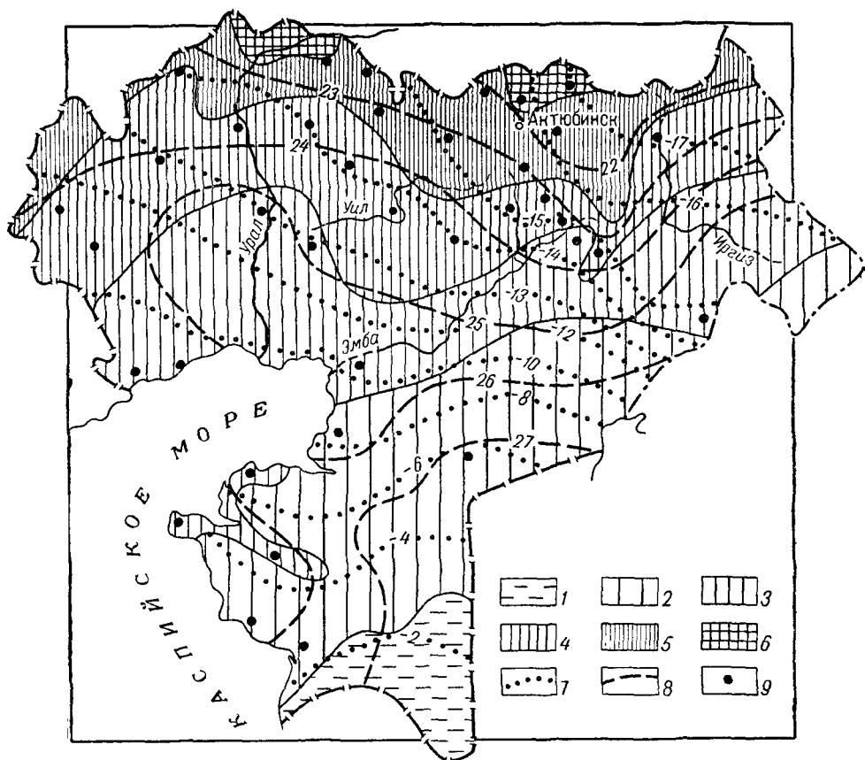
Рис. 7. Схематическая карта основных климатических показателей (составил Ж. С. Садыков)
