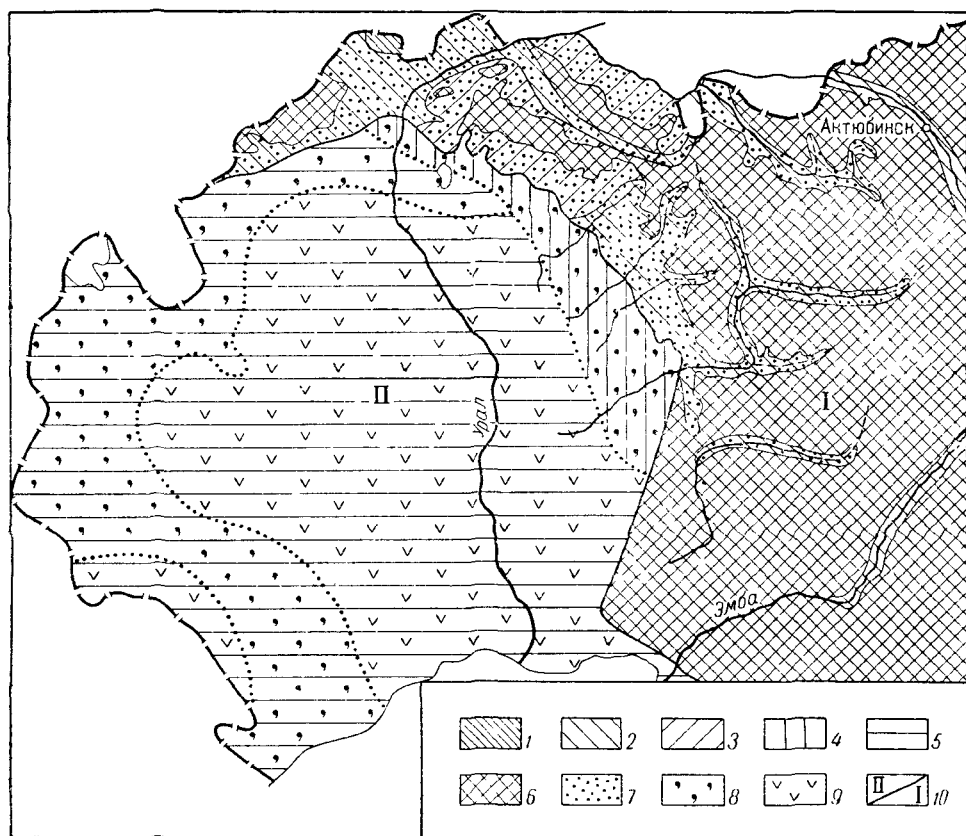
Рис. 34. Схематическая гидрогеологическая карта верхнеплиоценовых отложений Прикаспийской впадины. (Составила Г. В. Брянская)
