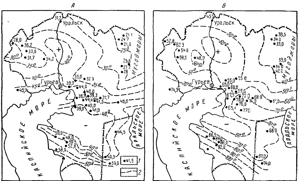
Рис. 71. Схематические геотермические карты Арало-Каспийского региона для глубин А — 1000 м; Б — 2000 м (Составлены Ж. С. Сыдыковым по материалам В. Б. Колпакова, В. Н. Корценштейна, И. Б. Дальяна, Д. А. Джангирияца, Ж. С. Садыхова и др.) 1 — скважины, в которых проведены глубинные размеры температуры воды, °С, 2 — изотермы, °С
