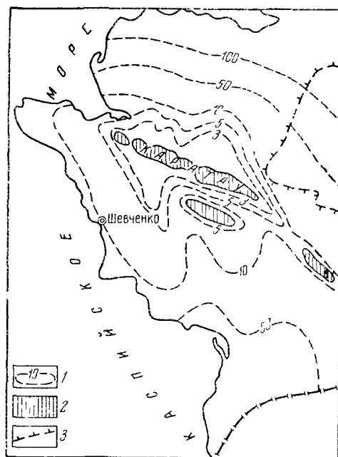
Рис. 51. Схематическая карта минерализации подземных вод сеноман-альбского водоносного комплекса. (Составили В. Б. Колпаков, А. К. Кугешев, Ж. С. Садыков):
