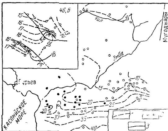
Рис. 72. Схематическая карта гидроизотерм сеноман-альбского водоносного комплекса Эмбенского района и солянокупольной структуры Ушкан. (Составил В. Б. Колпаков)
