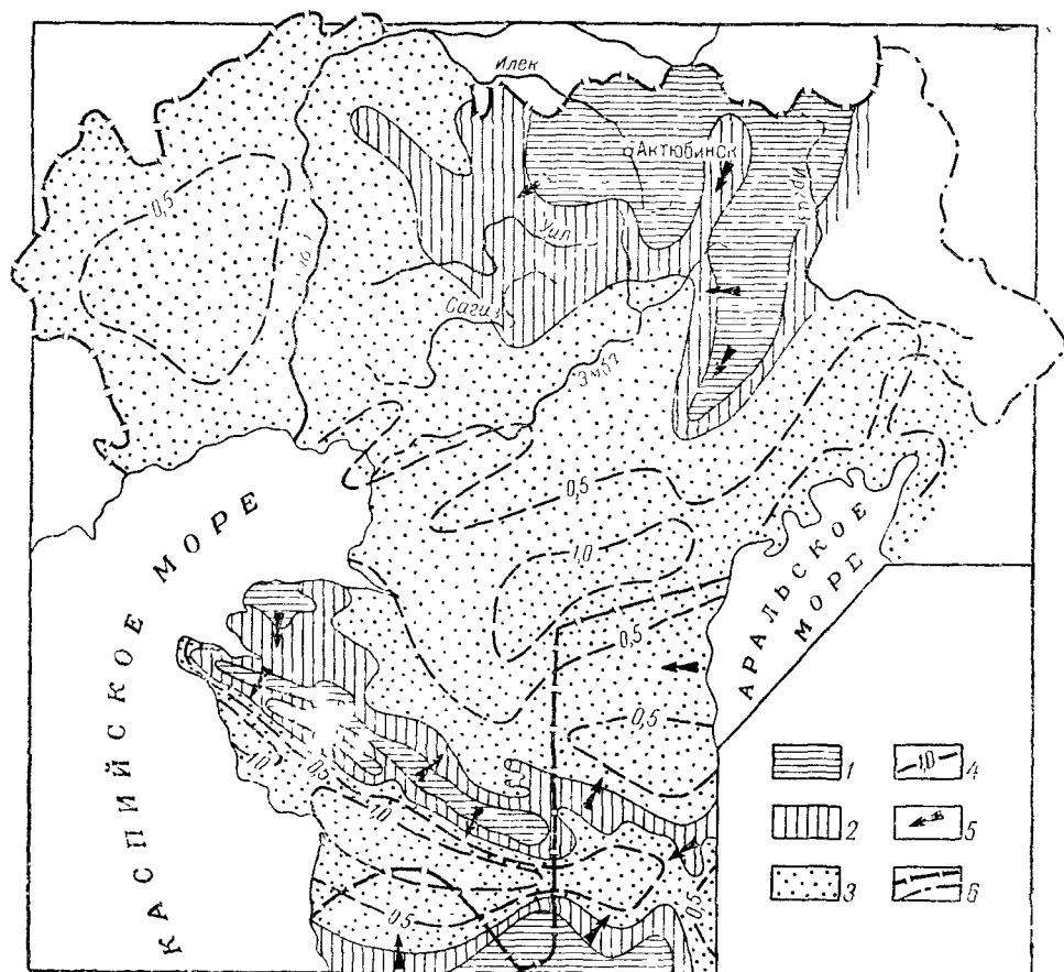
Рис. 58. Палеогидрогеологическая схема юрских отложений. (Составил Ж. С. Садыков)
