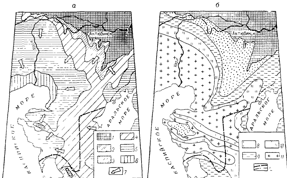
Рис. 62 Схематические карты положения пьезометрической поверхности (а) и градиента минерализации (б) подземных вод нижнемеловых отложений Западного Казахстана (составил Ж. С. Сыдыков)
