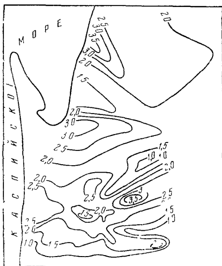
Рис 48. Изолинии минерализации подземных вод карстового бассейна долины Кетык, г/л (Составили В. Б. Колпаков, Г. Н. Абдразакова)
