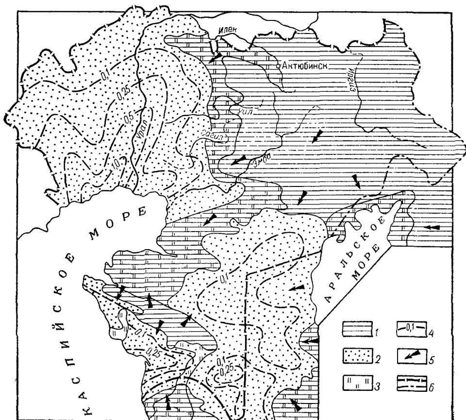
Рис. 61. Палеогидрогеологическая схема среднеплиоценовых отложений (составил Ж. С. Сыдыков)
