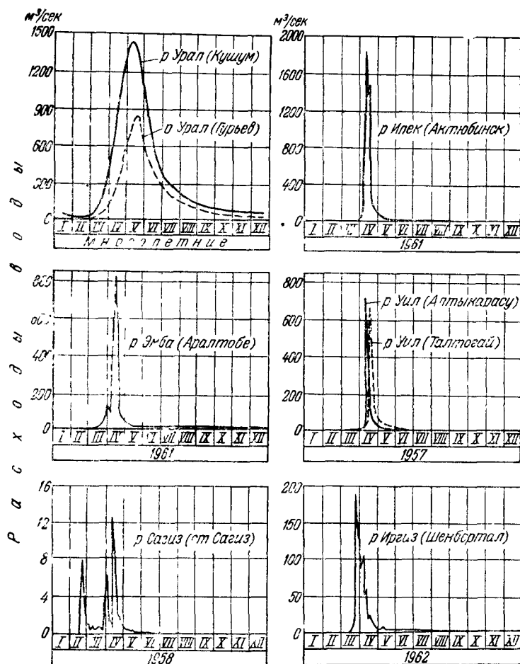
Рис. 8. Гидрографы основных рек Западного Казахстана
