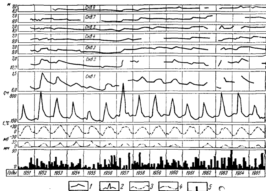
Рис. 55. Изменение уровня грунтовых вод и метеогидрологических факторов на Чапаевском балансовом участке. (Составил Н. И. Гордиенко) 1 — уровень грунтовых вод (м); 2 — уровень воды в р. Урале (см); 3 — температура воздуха (°C); 4 — дефицит насыщения воздуха (мм); 5 — атмосферные осадки (мм)
