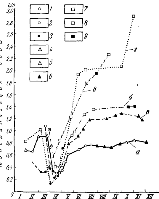
Рис. 10. Изменение минерализации воды основных рек Западного Казахстана в течение года (по Ж. С. Садыкову)
