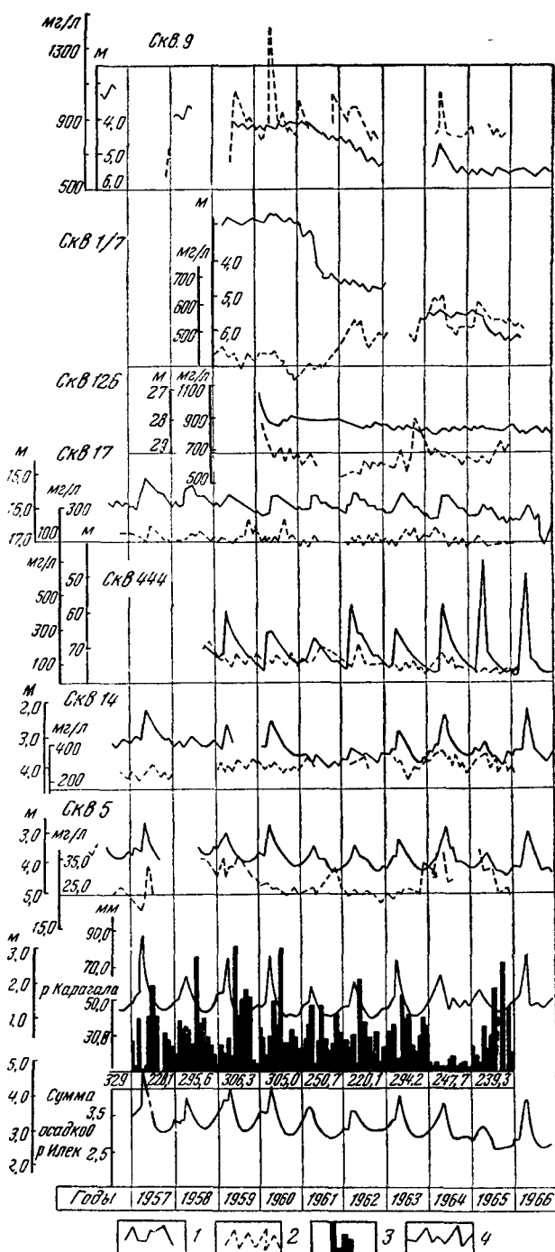
Рис. 57. Изменение атмосферных осадков и гидрогеологических показателей. (Составили Ю. В. Архидьконских, Н. М. Васильева)
