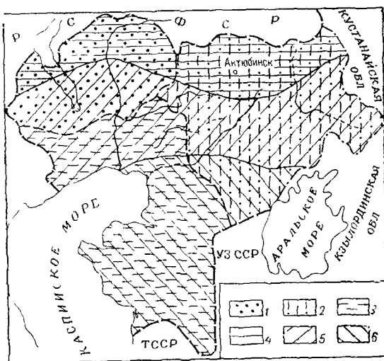
Рис. 1. Обзорная карта Западного Казахстана: Административные области: 1 — Уральская, 2 — Актюбинская, 3 — Гурьевская. Природно-климатические зоны: 4 — степная; 5 — полупустынная; 6 — пустынная.
