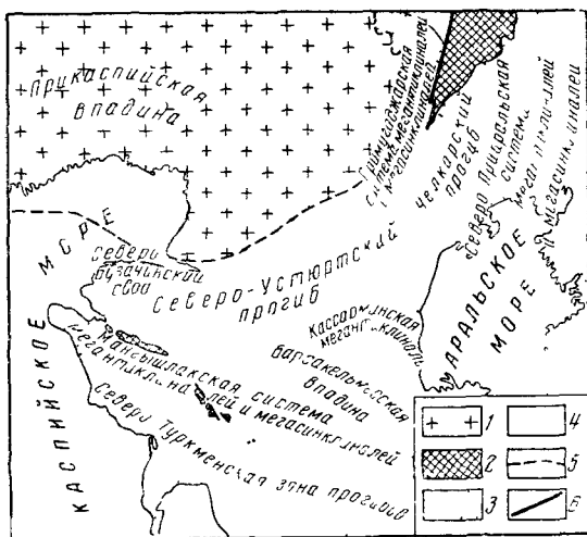
Рис. 28 Основные структурные элементы Западно-Казахстанской части Туранской плиты (По В. С. Журавлеву, Р. Г. Гарешкову)
