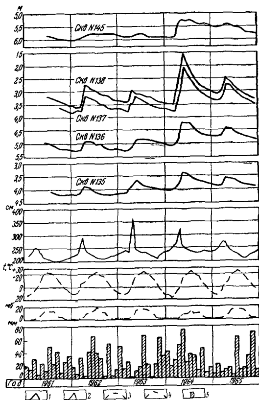
Рис 56 Изменение уровня грунтовых вод и метеогидрологических факторов на Казахском балансовом участке (Составил Н. И. Гордиенко)
