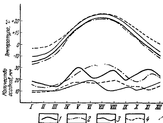
Рис. 6. Изменение средних многолетних месячных температур воздуха (1881—1960 гг.) и количества осадков (1891—1945 гг.)
