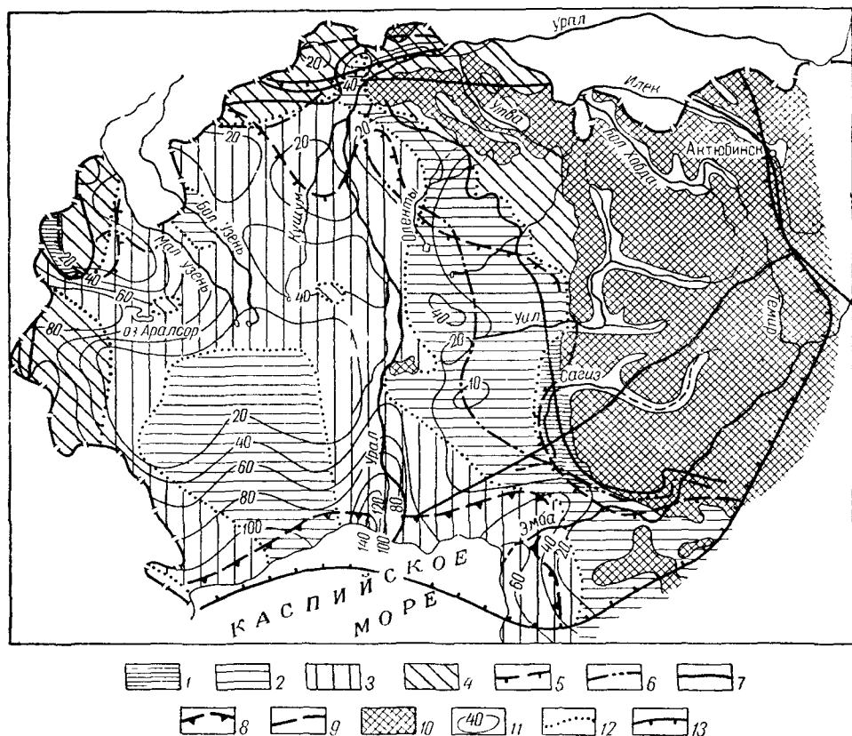
Рис. 32. Схематическая гидрогеологическая карта четвертичных отложений каспийских трансгрессий. (Составил М. П. Распопов)
