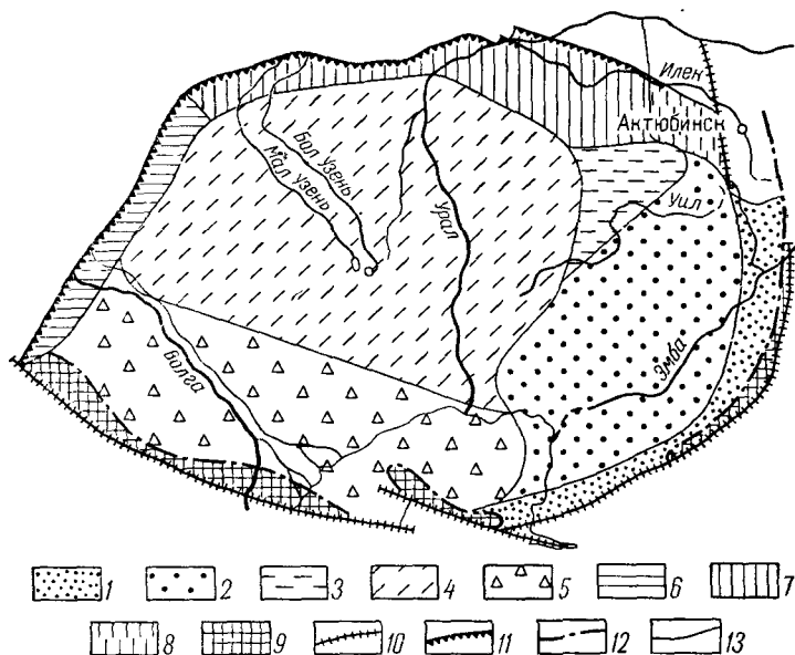
Рис. 26. Схема расположения структурных зон Прикаспийской впадины (по В. С. Журавлеву):
