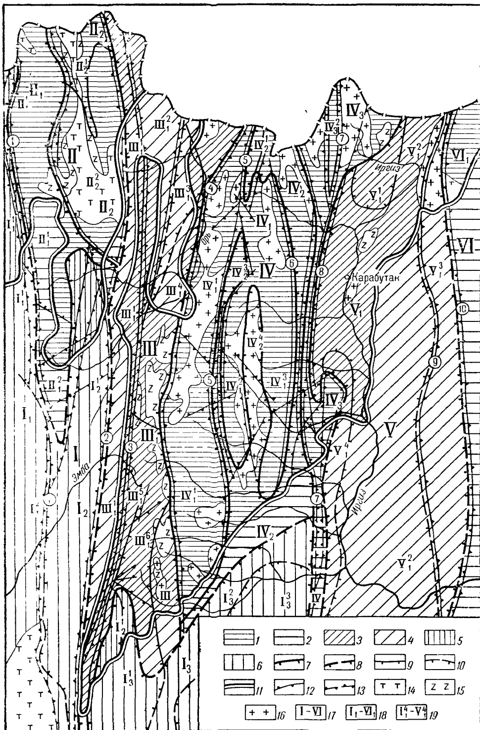
Рис. 27. Схематическая тектоническая карта южной оконечности Урала. (Составил П. Л. Смольяников)
