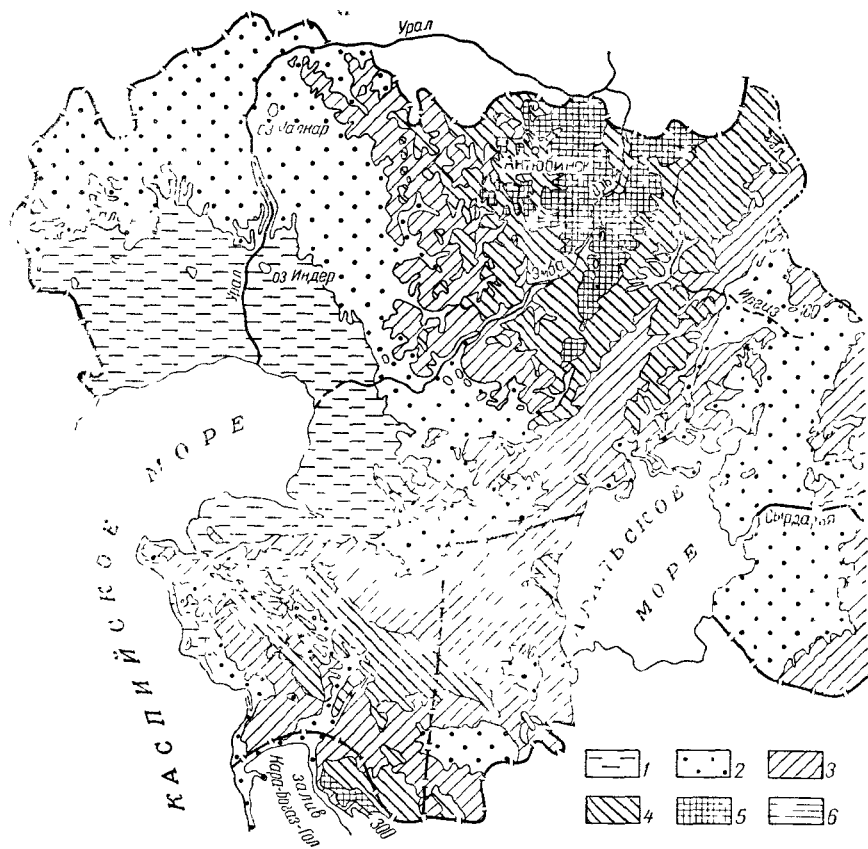
Рис. 2. Гипсометрическая карта Западного Казахстана (составила А. А. Гуськова):
