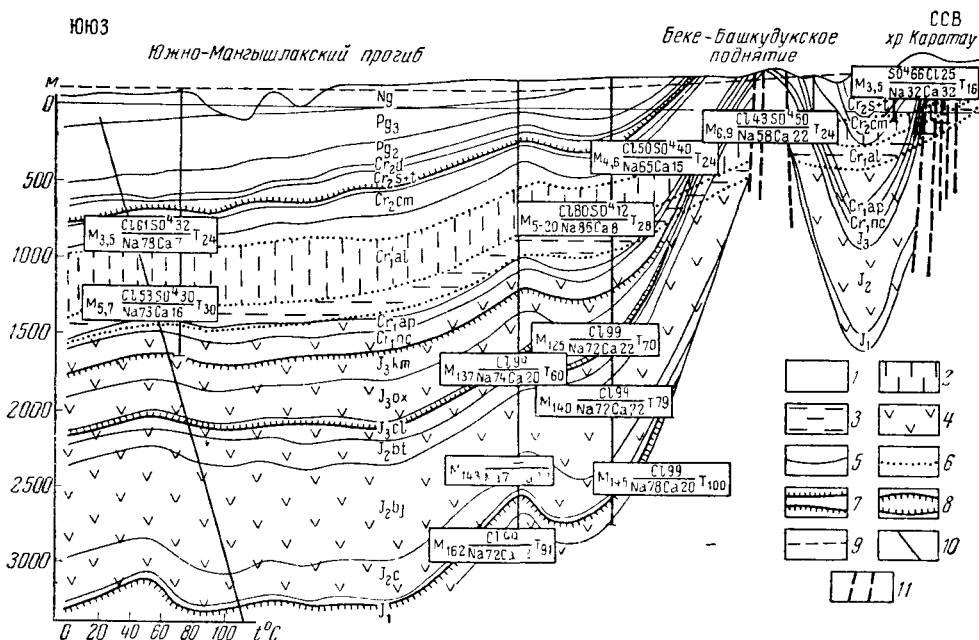
Рис. 50. Гидрогеологический профиль Южно-Мангышлакского артезианского бассейна по направлению Каратау-Юг. (Составили В. Б. Коллаков, Г. Н. Абдразакова)
