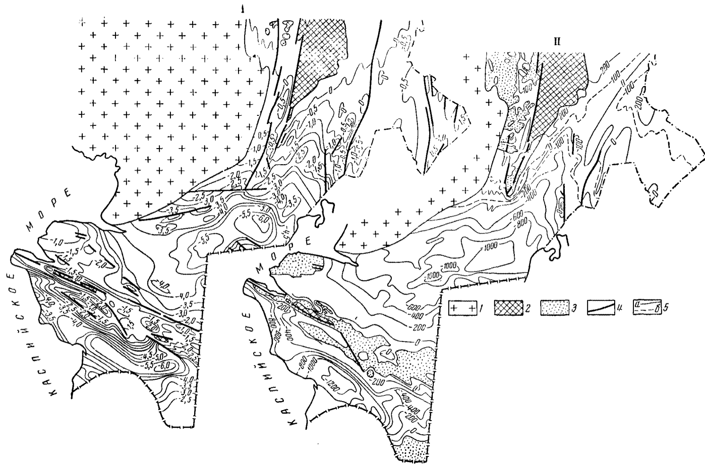
Рис. 29. Структурные карты поверхности фундамента (I) и кровли меловых отложений (II) западно-казахстанской части Туранской плиты (по В. С. Журавлеву, Р. Г. Гарецкому)
