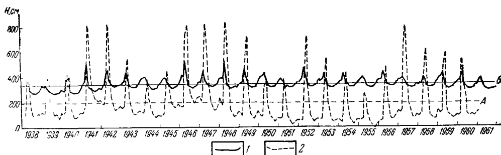
Рис. 9. Колебание уровней воды р. Урала у пос. Кушум — 1 и р. Илека у гор. Актюбинска — 2
