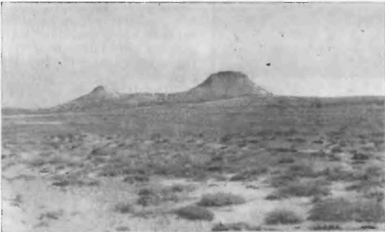
Рис 4 Денудационный останец на Тургайской равнине, плоская вершина бронирована железистыми песчаниками верхнего олигоцена. Останец сложен алевролитами и глинами среднего олигоцена, прилегающая равнина — глинами чеганской свиты (Фото Р А Сегедина)
