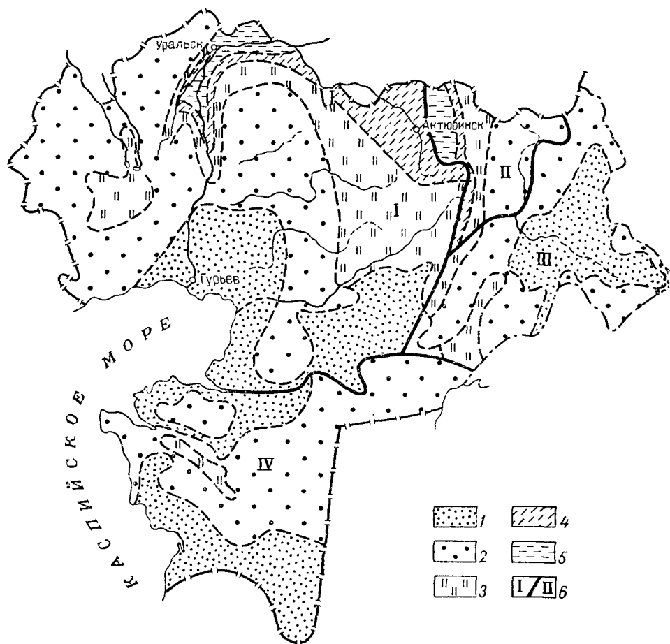
Рис. 63. Схематическая карта среднегодового слоя питания подземных вод Западного Казахстана. (Составил Ж. С. Сыдыков)
