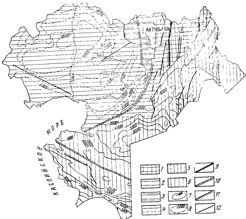
Рис. 25. Тектоническая схема Западного Казахстана
