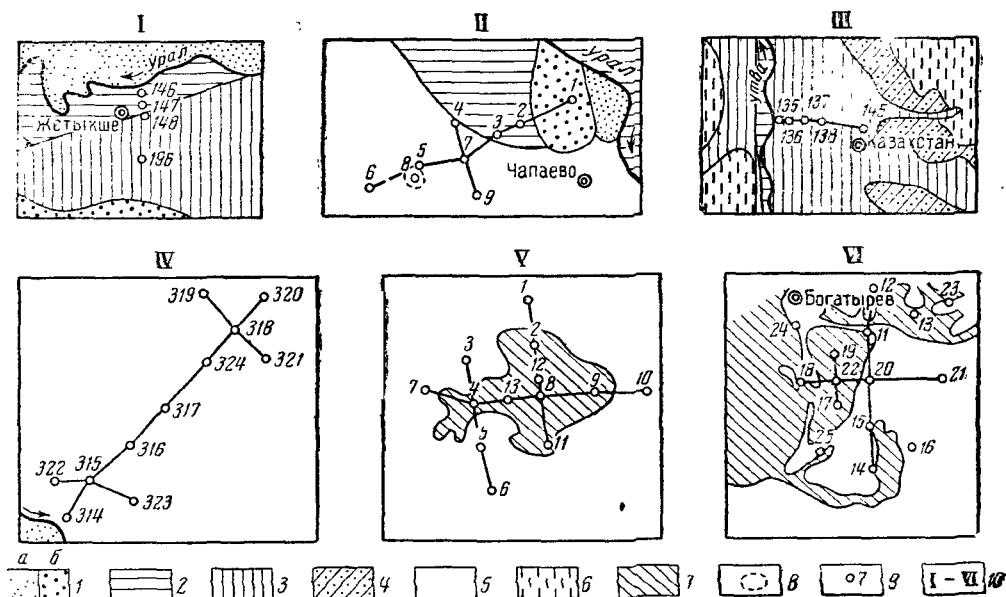
Рис. 53. Схема расположения наблюдательной сети на балаисовых участках северной части Прикаспия. (Составил А. В. Сотников, Н. И. Гордиенко)
