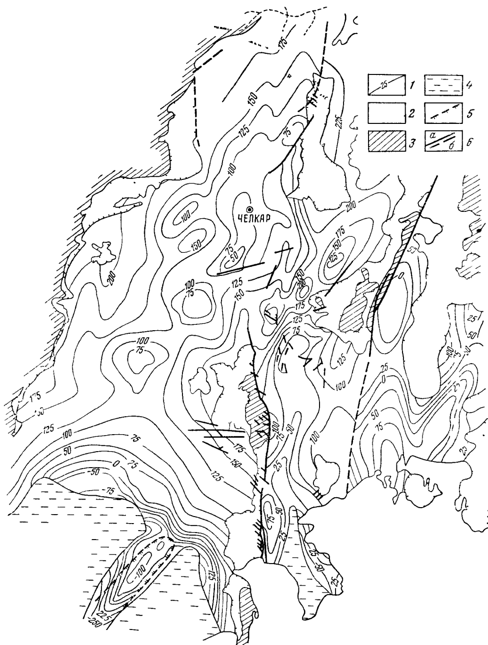
Рис. 43 Схематическая карта глубин залегания кровли песчаной фации верхнеэоценовых отложений Северного Приаралья (Составили Г. Т. Давидович и Л. М. Онищенко) 1 — изогипсы кровли песчаной фации отложений, через 25 м, 2 — участки выхода песчаных отложений на дневную поверхность, 3 — участки, на которых отсутствуют песчаные фации, 4 — участки, на которых наблюдаются песчаные фации, 5 — участок, на котором отсутствуют подземные воды в верхнеэоценовых отложениях, 6 — линии тектонических нарушений (а — установленные и б — предполагаемые)
