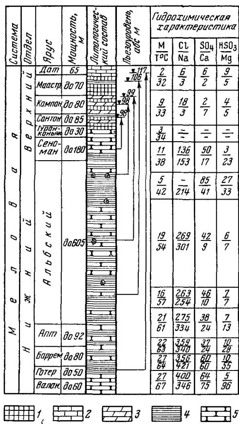
Рис 49 Гидрогеологический разрез чехловых отложений Мангышлака (Составил В. Б. Колпаков)
