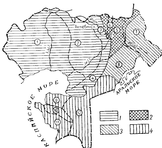
Рис 31. Схема гидрогеологического районирования Западного Казахстана (по А. В. Сотникову, Ж. С. Сыдыкову)
