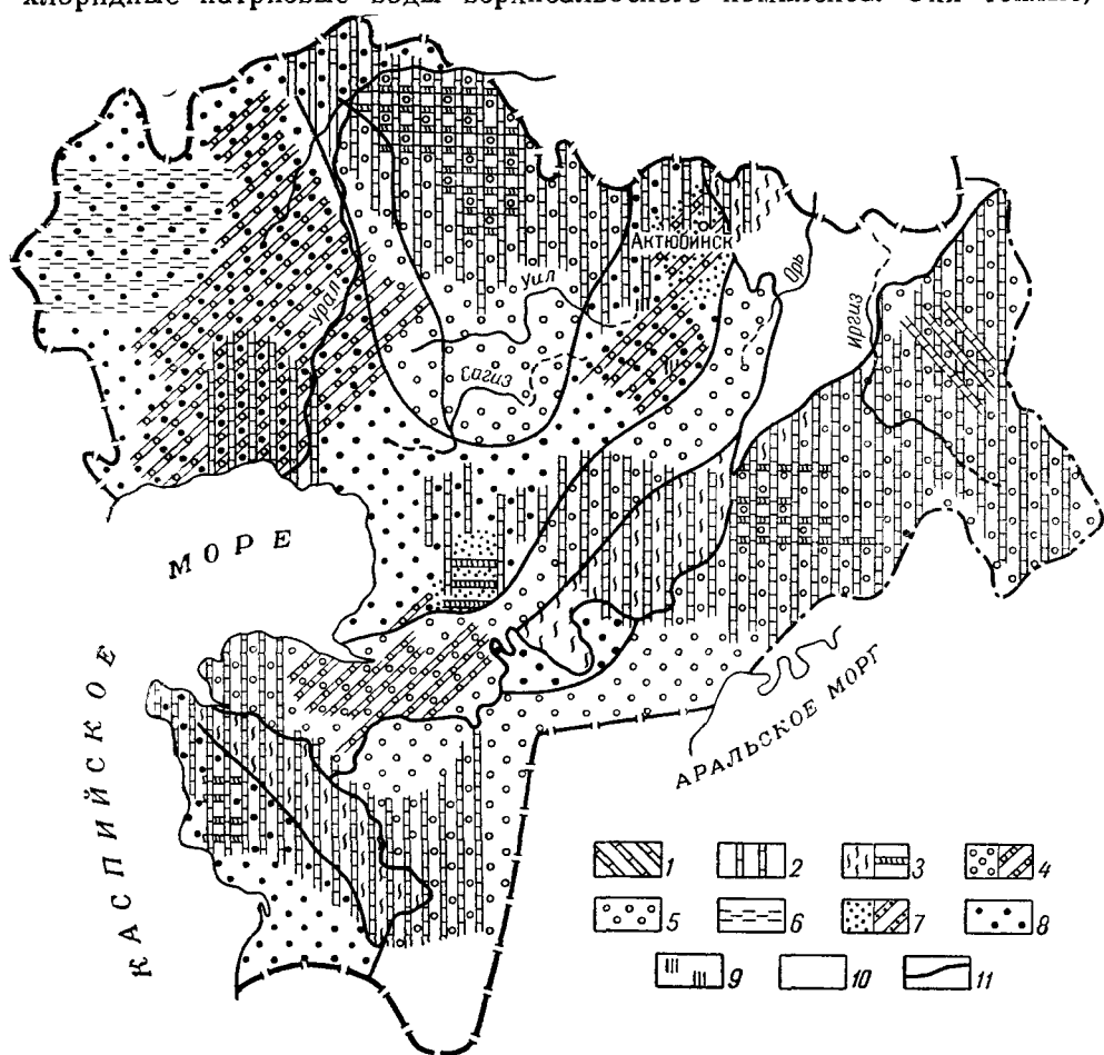
Рис. 75. Схематическая карта распространения минеральных лечебных вод Западного Казахстана. (Составила А. Б. Авдеева)
