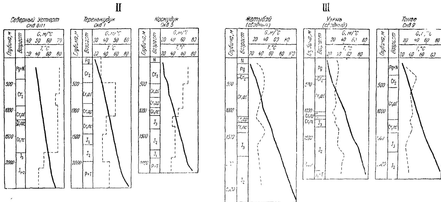
Рис. 69. Геотермическая характеристика разрезов опорных пунктов I — Прикаспийской впадины; II — Устюрта; III — Южного Мангышлака 1 — температура, °C; 2 — геометрическая ступень, M/°C
