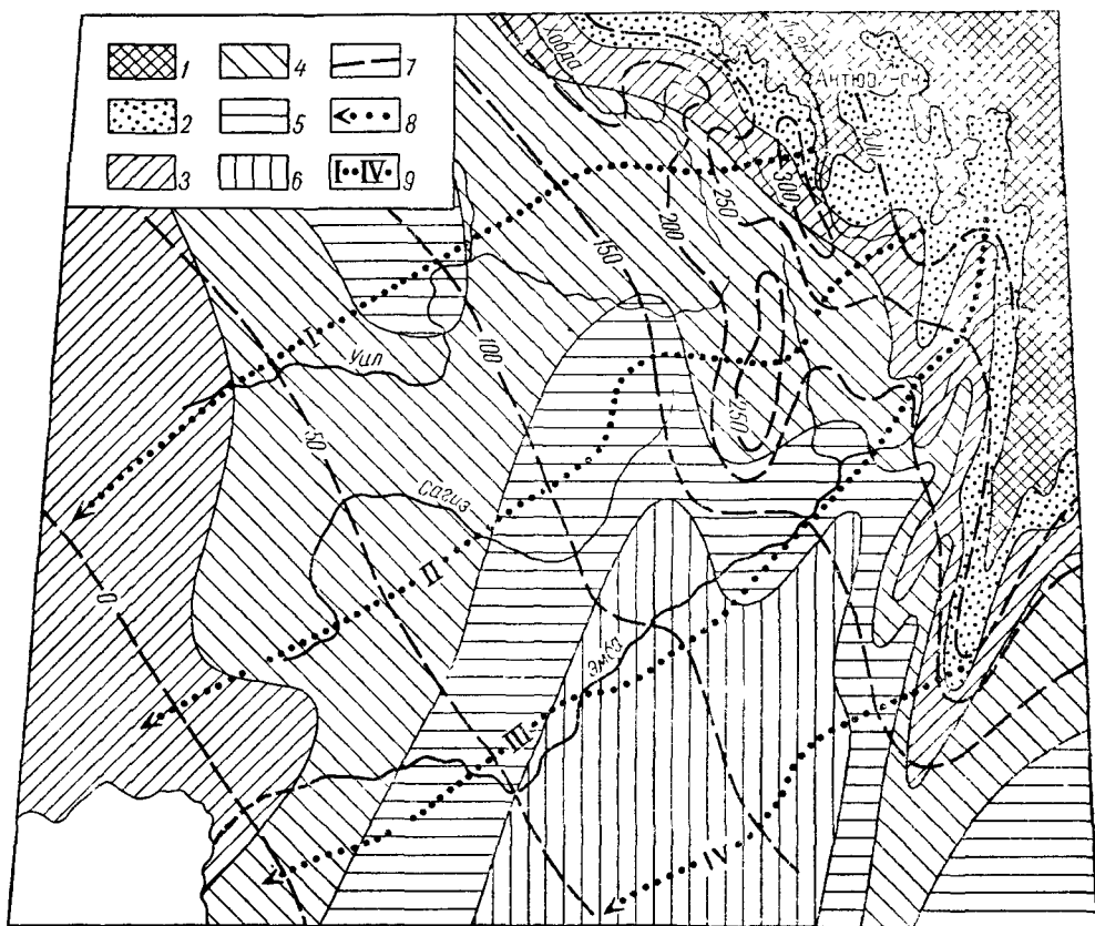
Рис. 35. Схематическая карта гидронизопьез и мощностей сеноман-альбского водоносного комплекса восточной части Прикаспийской впадины (составил Ж. С. Садыков)
