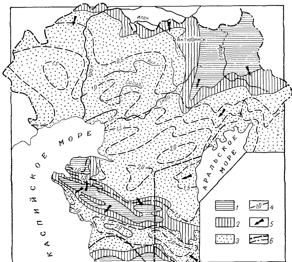
Рис. 59. Палеогидрогеологическая схема меловых отложений. (Составил Ж. С. Сыдыков)
