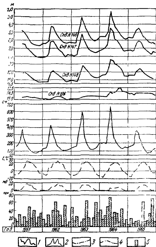
Рис. 54. Изменение уровня грунтовых вод и метеогидрологических факторов на Жетыкшинском балансовом участке. (Составил Н. И. Гордненко)
