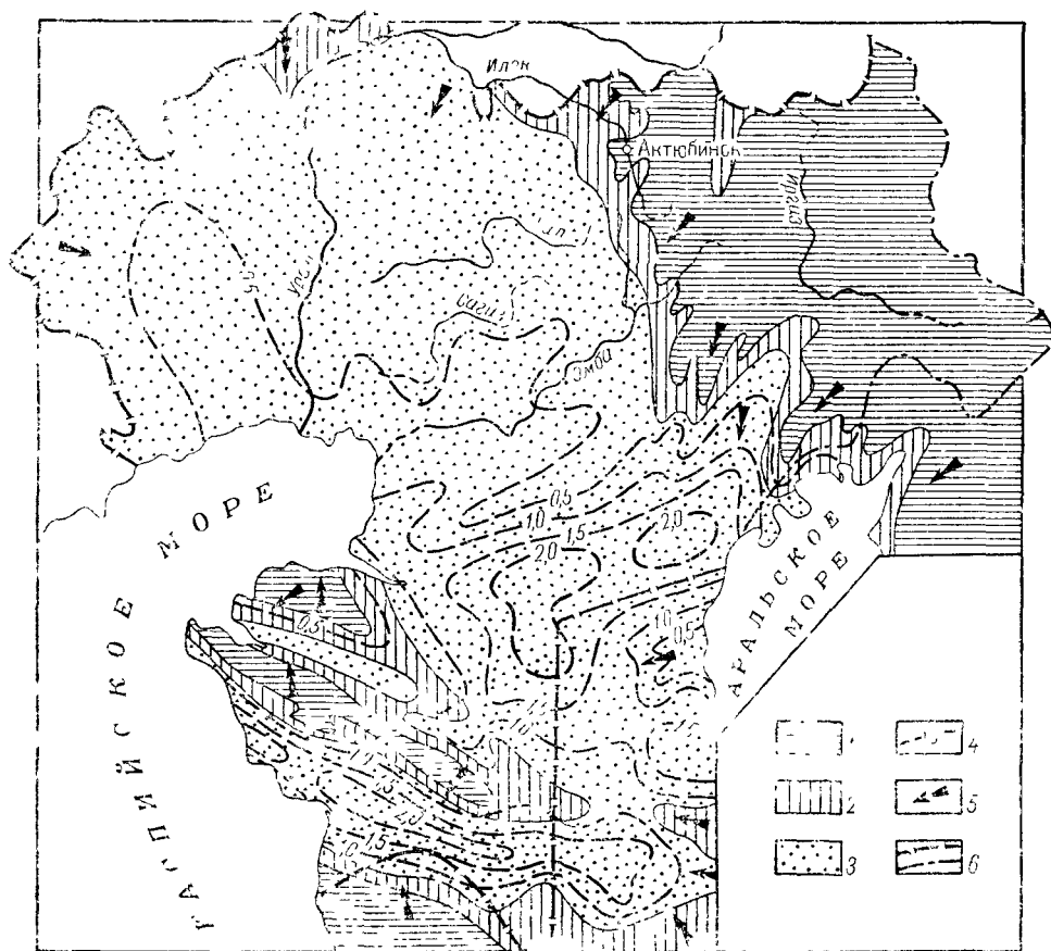
Рис. 60. Палеогидрогеологическая схема нижнемиоценовых отложений.
