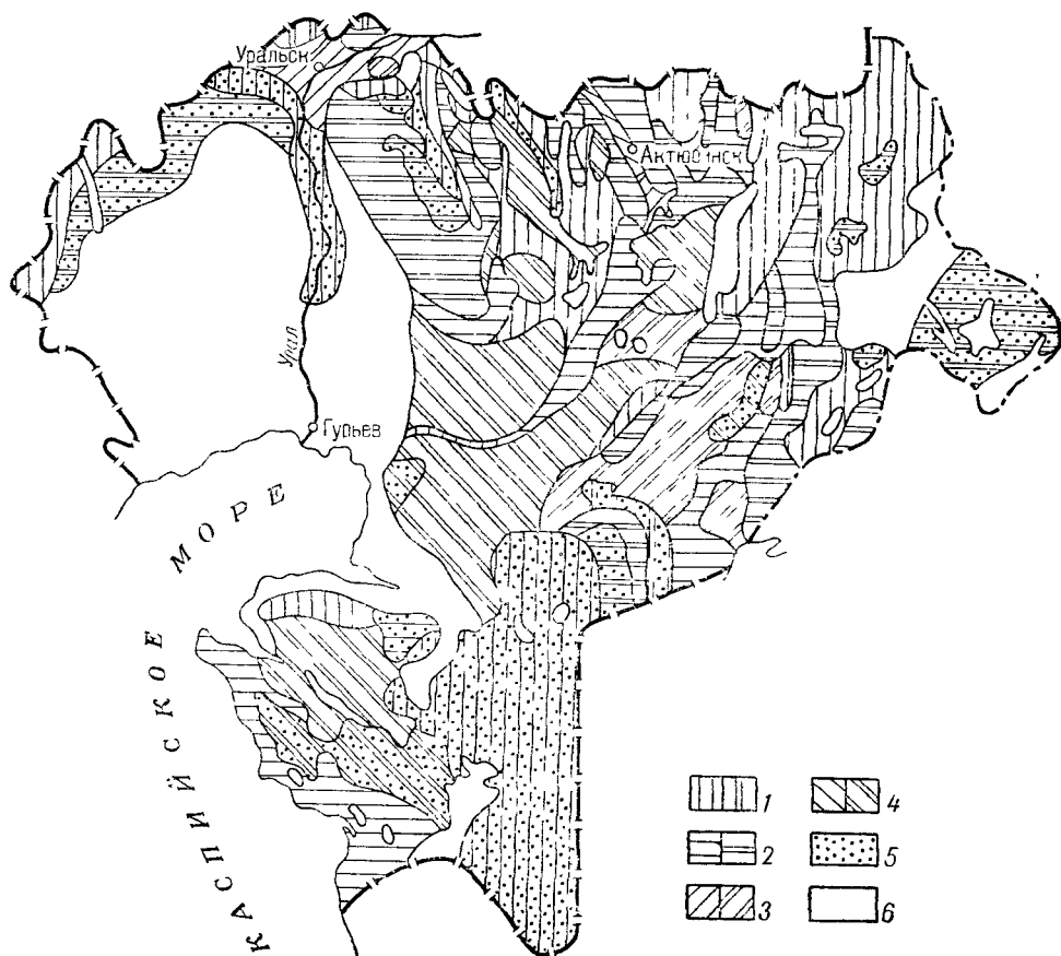
Рис. 64. Возможная производительность расчетных водозаборов с минерализацией подземных вод до 3 г/л
