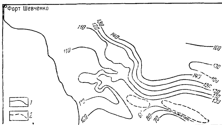
Рис. 52. Схематическая карта гидроизопьез сеноман-альбского водоносного комплекса Южно-Мангышлакского артезианского бассейна. (Составили В. Б. Колпаков, И. Ф. Головатый):
