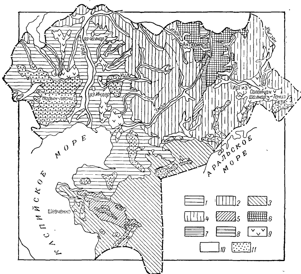
Рис. 30. Схематическая геоморфологическая карта Западного Казахстана. (Составили Н. Э. Зейберлих, М. В. Проницева)
