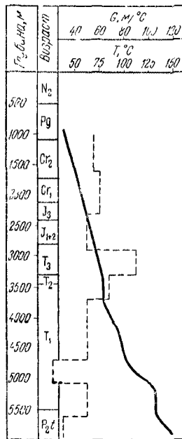
Аралсор СКВ СТ 1
