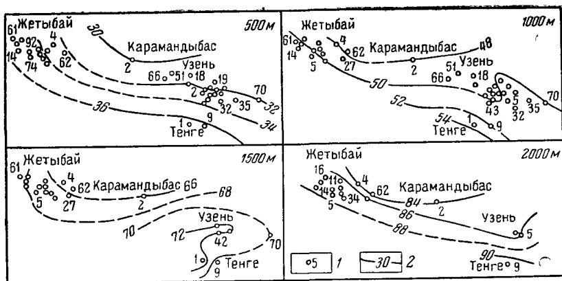
Рис. 73. Схема распределения температуры на различных глубинах в северной части Южно-Мангышлакского артезианского бассейна (по В. Н. Корценштейну, 1967)
