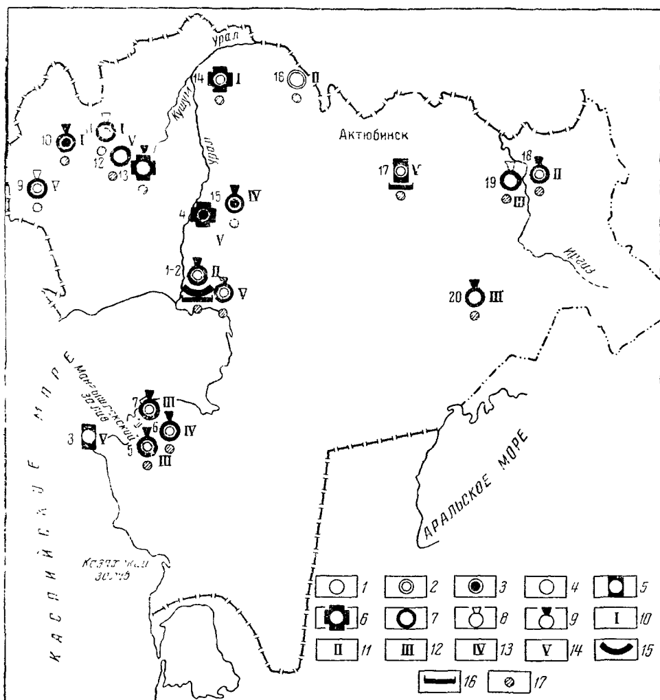
Рис. 76. Схематическая карта минеральных лечебных грязей Западного Казахстана. (Составил М. Н. Гончаров)
