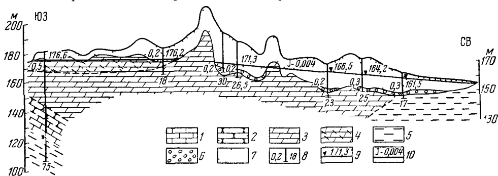
Рис 46 Гидрогеологический разрез песчаного массива Саускан (Составила И. М. Суслова)
