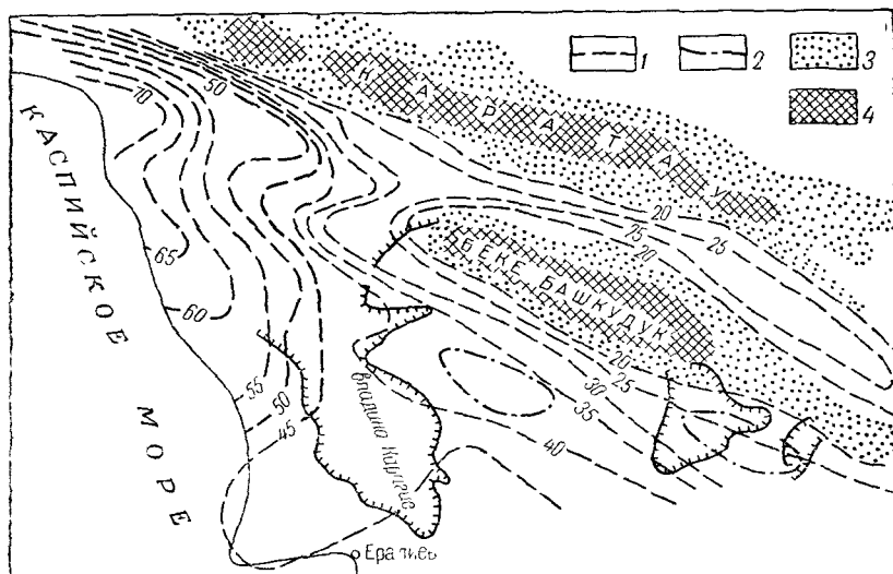
Рис. 74. Схематическая карта гидронизотерм верхнеальбского водоносного комплекса Южно-Мангышлакского артезианского бассейна (составил В. Б. Колпаков)
