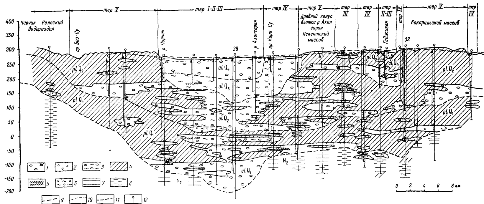
Рис 35. Схематический геолого-гидрогеологический разрез через низовья долины Чирчика и Ахангарана (в створе селений Чиназ — Солдатское — Новоалексеевское). 1 — галечники, 2 — гравий, 3 — галечники с примесью глинистых частиц, 4 — суглинки песчаные и пылеватые, 5 — конгломераты на смешанном цементе, 6 — пески аркозовые с гравием, 7 — глины, 8 — алевролиты глинистые, 9 — пьезометрический уровень подземных вод, 10 — уровень грунтовых вод, 11 — контур возрастных комплексов отложений, 12 — скважины разведочные (слева показан интервал установки фильтра и величина напора водоносного горизонта — стрелкой).
