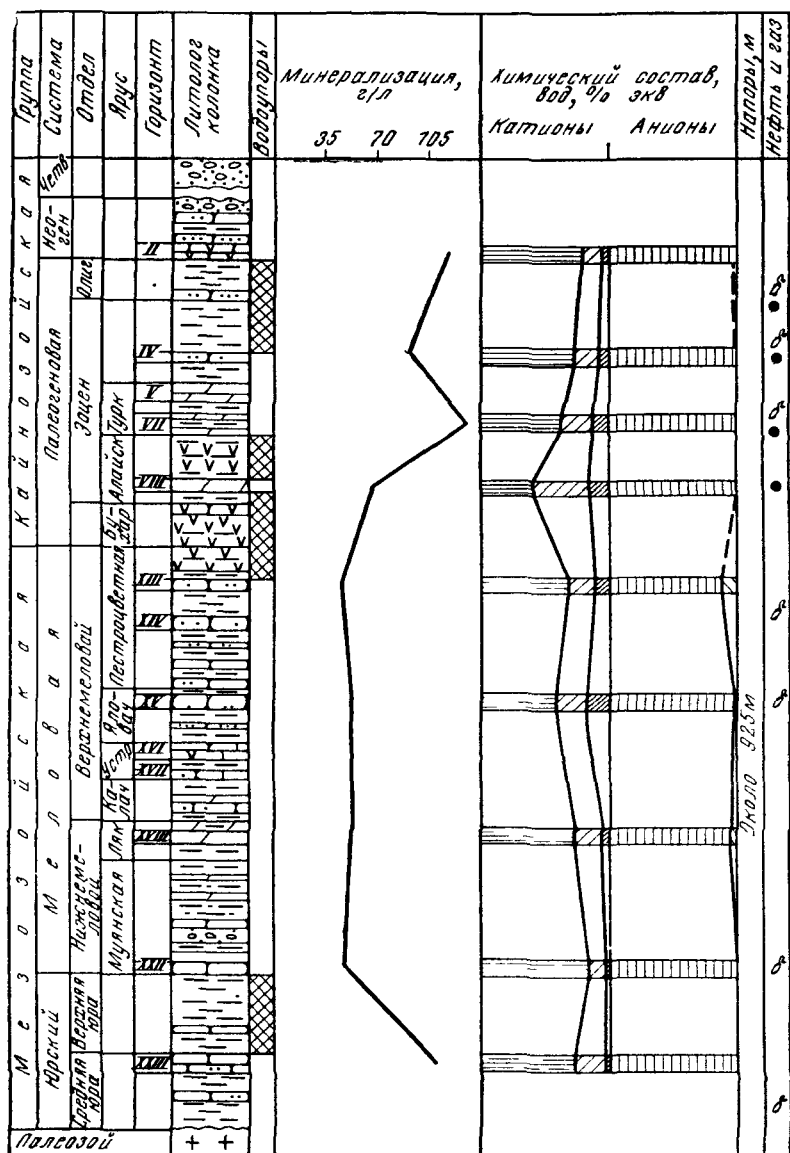
Рис. 78. Гидрогеологический разрез Северо-Сухского газонефтяного месторождения. Условные обозначения те же, что и на рис. 76
