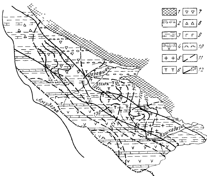
Рис. 47 Схематическая гидрохимическая карта водоносного комплекса неоконгломератских отложений
