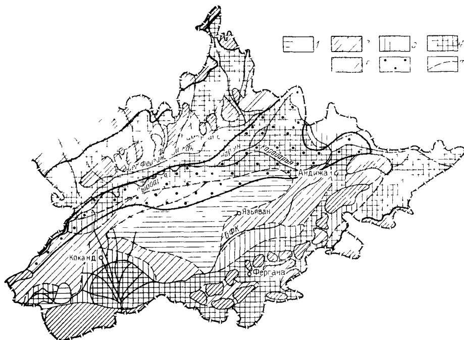
Рис. 31. Схема водопроводимости верхней стометровой толщи водоносных четвертичных отложений Ферганского артезианского бассейна. Водопроводимость ( кп ) в м/сутки: 1 — до 100, 2 — от 100 до 500; 3 — от 500 до 1000, 4 — более 1000, 5 — не изученные участки (адыры и горы), 6 — Нарын-Карадарья Сырдарьинский аллювиальный поток подземных вод, 7 — границы участков с разной водопроводимостью
