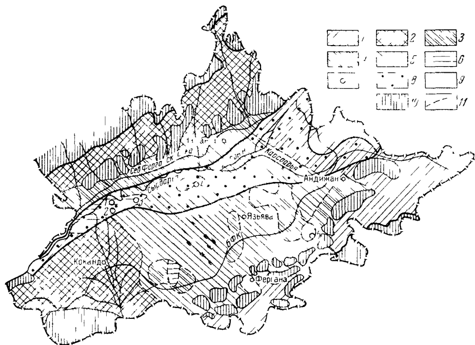
Рис 32. Гидрохимическая схема эксплуатируемых водоносных горизонтов среднечетвертичных (ташкентских) отложений Ферганского артезианского бассейна. Воды гидрокарбонатно-сульфатные 1 — плотный остаток 0,5 г/л Воды сульфатно-гидрокарбонатные 2 — плотный остаток до 0,5 г/л, 3 — плотный остаток 0,5—1 г/л, 4 — плотный остаток 1—2,5 г/л Воды сульфатно-гидрокарбонатные и гидрокарбонатно-сульфатные 5 — плотный остаток до 0,5 г/л Воды сульфатные с повышенным содержанием хлоридов 6 — плотный остаток 0,5—1 г/л 7 — вычленившиеся участки хлоридных и хлоридно-сульфатных вод плотный остаток 1—2 г/л, 8 — Нарын Карадарья Сырдарьинский аллювиальный поток подземных вод 9 — пролювиальные (подгорно-верные) потоки подземных вод, 10 — площади, где среднечетвертичные водоносные горизонты отсутствуют или не эксплуатируются, 11 — границы гидрохимических полей
