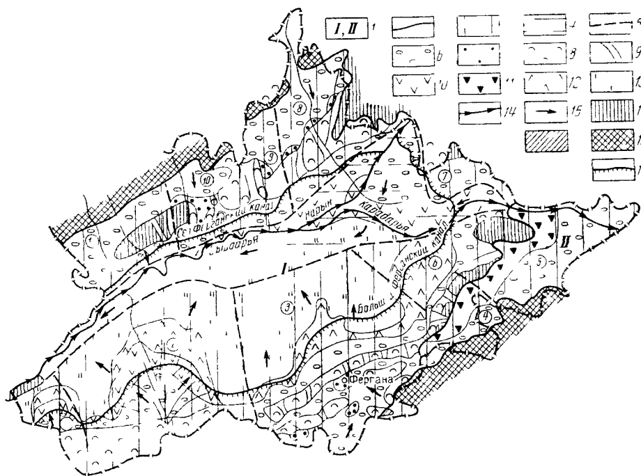
Рис. 30. Схема гидрогеологического районирования четвертичных водоносных комплексов Ферганского артезианского бассейна. Составил В. А. Гейц.
