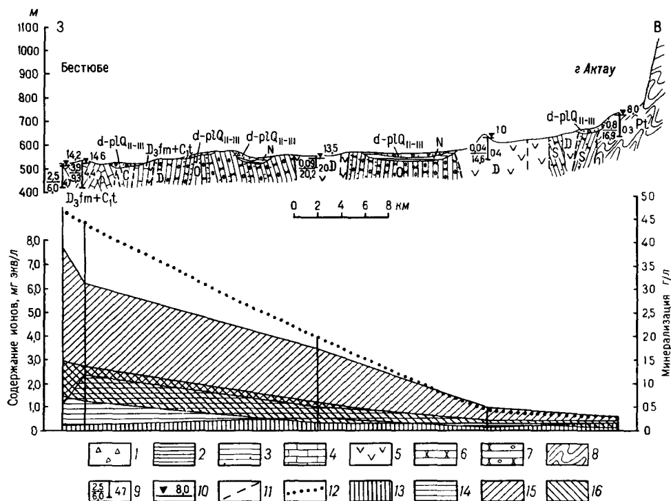
Рис 43 Гидрогеологический разрез и гидрохимический профиль восточного крыла Джайльминской синклинали по линии Бестюбе-Актау (составил Л. Я. Тененбаум) 1 — воды спорадического распространения делювиально-пролювиальных средне-верхнечетвертичных отложений ( dplQ_{II-III} ). Супеси и суглинки с линзами песков; 2 — водоупорные пестроцветные неогеновые глины (N); 3 — водоносный комплекс осадочных каменноугольных отложений (C) Аргиллиты, пересланяющиеся с алевролитами и песчанками; 4 — водоносный комплекс карбонатных фаменских и турнейских отложений ( D_3fm-C_1t ) Известняки; 5 — подземные воды зоны открытой трещиноватости эффузивных девонских пород (D) Порфириды, альбитофиры, туфы; 6 — водоносный комплекс осадочных силурийских отложений (S) Песчаники и алевролиты; 7 — водоносный комплекс осадочных ордовикских отложений (O) Песчаники с прослоями конгломератов и алевролитов; 8 — подземные воды зоны открытой трещиноватости метаморфических протерозойских пород (Pt) Кварциты и метаморфические сланцы; 9 — скважины слева в числителе — дебит (л/сек), в знаменателе — понижение (м), справа — минерализация воды (г/л); 10 — уровень подземных вод; 11 — тектонические нарушения, на гидрохимическом профиле 12 — линия общей минерализации воды (г/л); содержание ионов (мг.экв/л) 13 — HCO_3^- , 14 — SO_4^{2-} , 15 — Cl^- , 16 — Mg^{2+} Содержание Ca^{2+} откладывается от нуля графика
