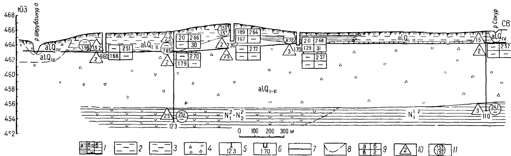
Рис 68 Инженерно-геологический разрез междуречья Шерубайнуры и Сокура (составила Л А Лебедь по материалам И С Русакова)
