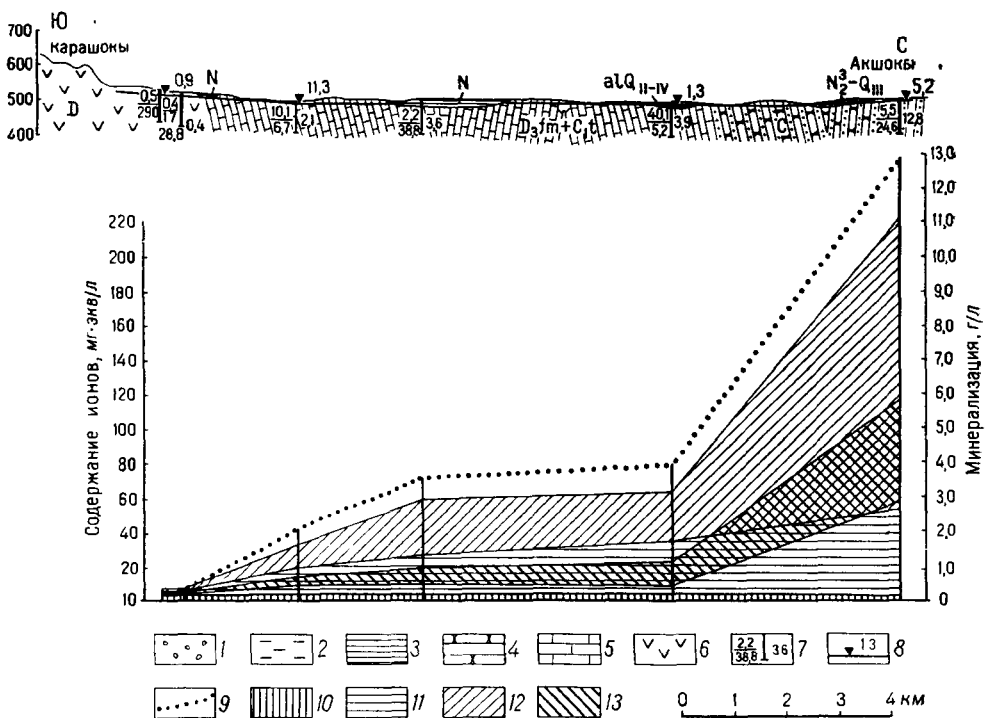
Рис. 42 Гидрогеологический разрез и гидрохимический профиль центральной части Джанлыминской синклинали по линии Карашоки-Акшоки (составил Л. Я. Тененбаум) 1 — водоносный горизонт аллювиальных среднечетвертичных—современных отложений (alQ II-IV ) Пески с гравием, супеси; 2 — воды спорадического распространения делювиально-пролювиальных верхнеплиоценовых — верхнечетвертичных отложений (N 2 2 —Q III ). Супеси и суглинки с линзами песков; 3 — водоупорные нестроцветные неогеновые глины (N); 4 — водоносный комплекс осадочных каменноугольных отложений (C). Аргиллиты, алевролиты, песчаники; 5 — водоносный комплекс карбонатных фаменских и турийских отложений (D 3fm —C it ) Известняки, 6 — подземные воды зоны открытой трещиноватости эффузивных девонских пород (D) Порфириты, альбитофиры, туфы; 7 — скважины: слева в числителе — дебит (л/сек), в знаменателе — понижение (м), справа — минерализация воды (г/л); 8 — уровень подземных вод; на гидрохимическом профиле: 9 — линия общей минерализации воды (г/л); 10 — содержание ионов (мг·экв/л), 11 — HCO 3 - ; 12 — Cl - ; 13 — Mg 2+ . Содержание Ca 2+ откладывается от нуля графика
