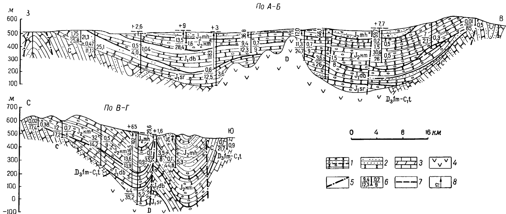
Рис. 33. Гидрогеологические разрезы Карагандинского артезианского бассейна по линиям А—Б и В—Г (составили И. М. Детцель, Н. С. Евтюхина)
