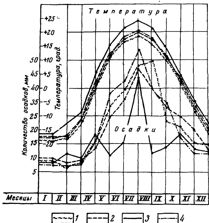
Рис 4. График изменения средних месячных температур воздуха и количества осадков за период с 1945 по 1958 г. Данные станций 1 — в Петропавловске, 2 — в Кустаная, 3 — в Тургае, 4 — в Целинограде
