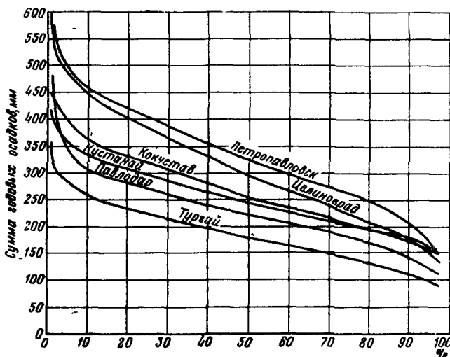
Рис. 7. График обеспеченности атмосферными осадками (по О. А. Дроздову)
