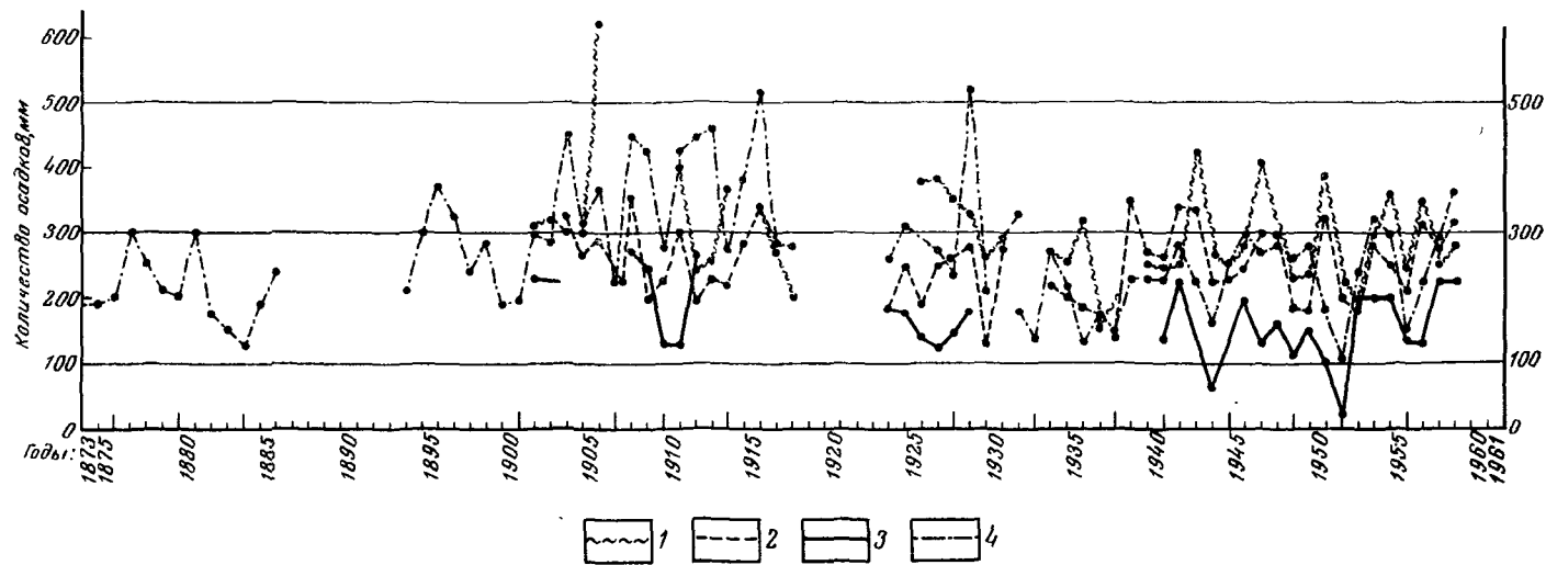
Рис. 6. График изменений суммы годовых осадков Данные метеостанций: 1 — в Петропавловске; 2 — в Кустане; 3 — в Тургае; 4 — в Целинограде
