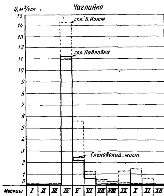
Рис. 9. Средние месячные расходы рек за многолетний период
