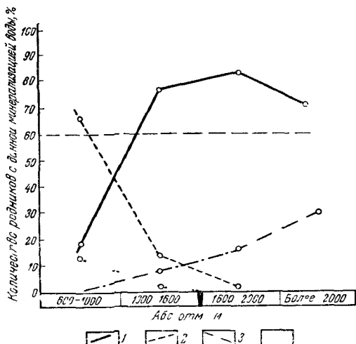
Рис. 41. Распределение родников с различной минерализацией воды по ярусам рельефа
