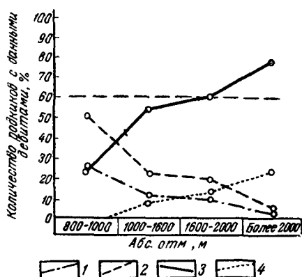
Рис. 40. Распределение родников с разными дебитами по ярусам рельефа
