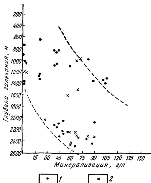
Рис. 48. Зависимость минерализации вод юрско-нижнемелового комплекса от глубины залегания пласта 1 — структуры центральной части, 2 — структуры восточной части
