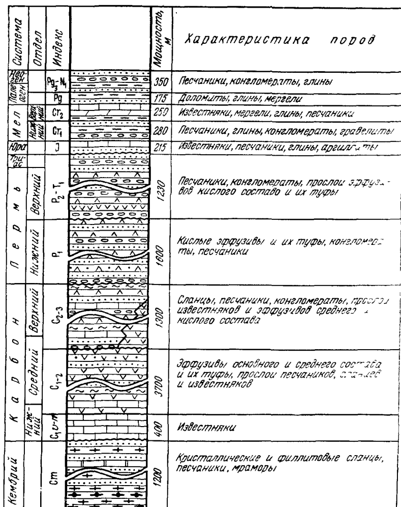
Рис. 17. Сводная стратиграфическая колонка пород Южно-Гиссарской зоны
