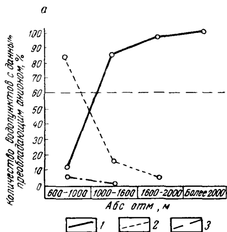
Рис. 42. Распределение вод с различными преобладающими анионами (а) и катионами (б) по ярусам рельефа
