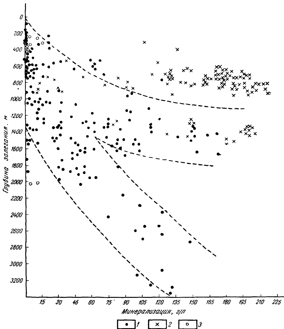
Рис. 47. Зависимость минерализации вод верхнемеловых — палеогеновых отложений южной периферии Каракчикум-Каныбадамского бассейна от глубины залегания 1 — центральная часть; 2 — восточная часть, 3 — западная часть
