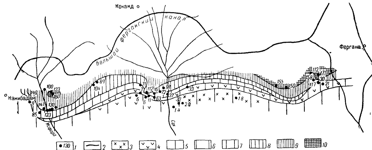
Рис. 33. Схематическая гидрохимическая карта вод II пласта палеогеновых отложений:
