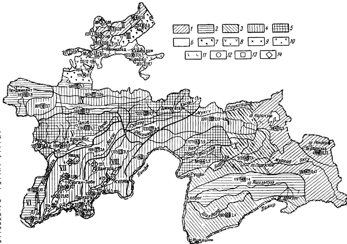
Рис. 64. Схематическая карта ресурсов подземных вод
