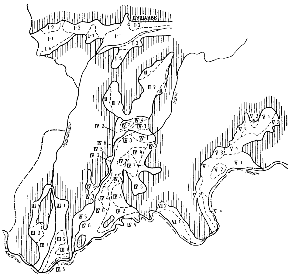
Рис. 82. Схема гидрогеолого-мелиоративного районирования орошаемых земель Южного Таджикистана. Условные знаки см. на рис. 81
