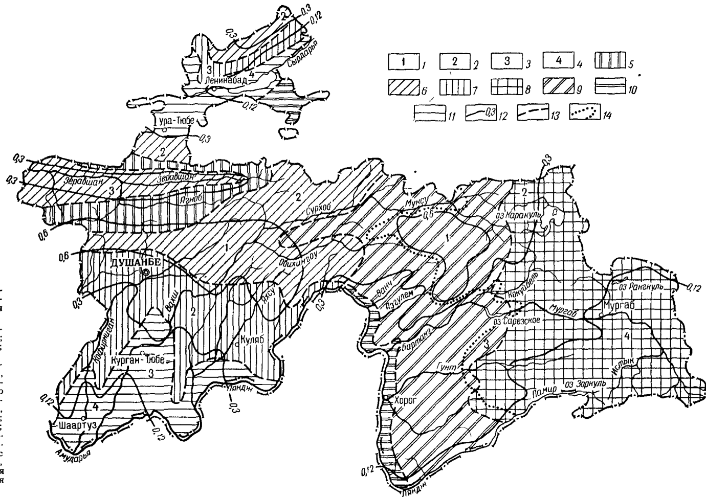
Рис. 11. Схема климатического районирования. Климатические зоны увлажнения (по Н. Н. Иванову):
