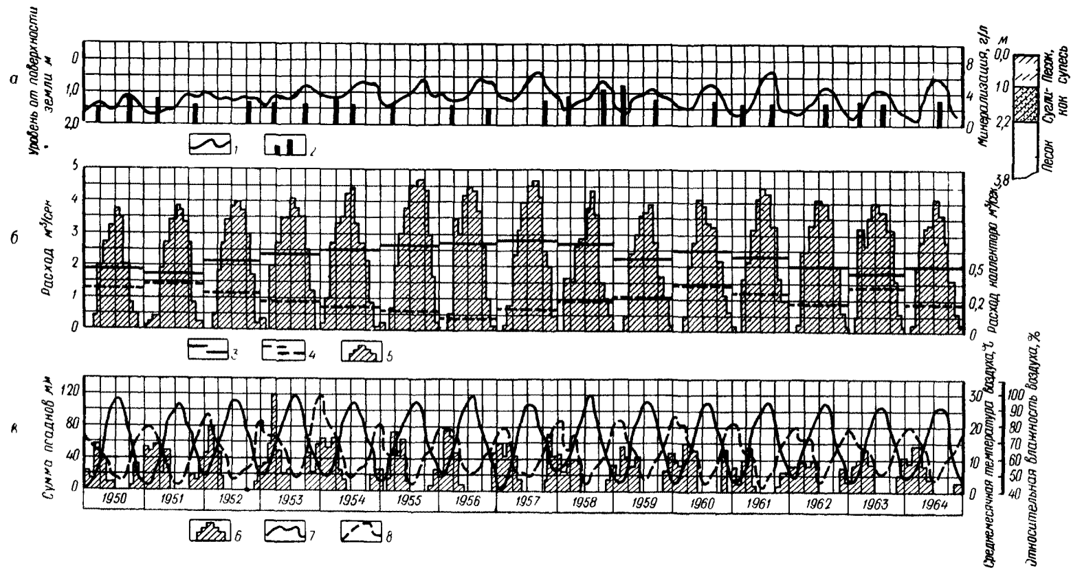
Рис 78 Режим уровня грунтовых вод и изменение их минерализации для естественно слабодренированных площадей третьей террасы р Вахи в сопоставлении с водоподачей на орошение и климатическими факторами а — орошаемые земли левобережья в 250 м от коллектора В Д II и в 250 м от канала «Ветка переключения» (скв 56) б — канал «Ветка переключения» в метеорологические данные 1 — уровень от поверхности земли, м 2 — минерализация грунтовых вод, г/л 3 — кривая среднеговегационного расхода канала «Ветка переключения», м³/сек 4 — кривая среднегодового расхода коллектора В Д II, м³/сек 5 — водоподача на орошение, м³/сек 6 — осадки, мм 7 — температура воздуха, °C 8 — относительная влажность воздуха, %
