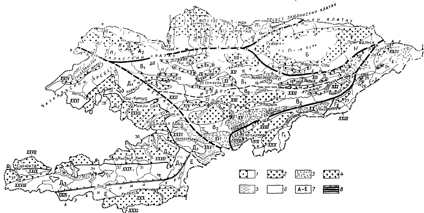
Рис. 10. Схема гидрогеологического районирования Киргизской ССР:
