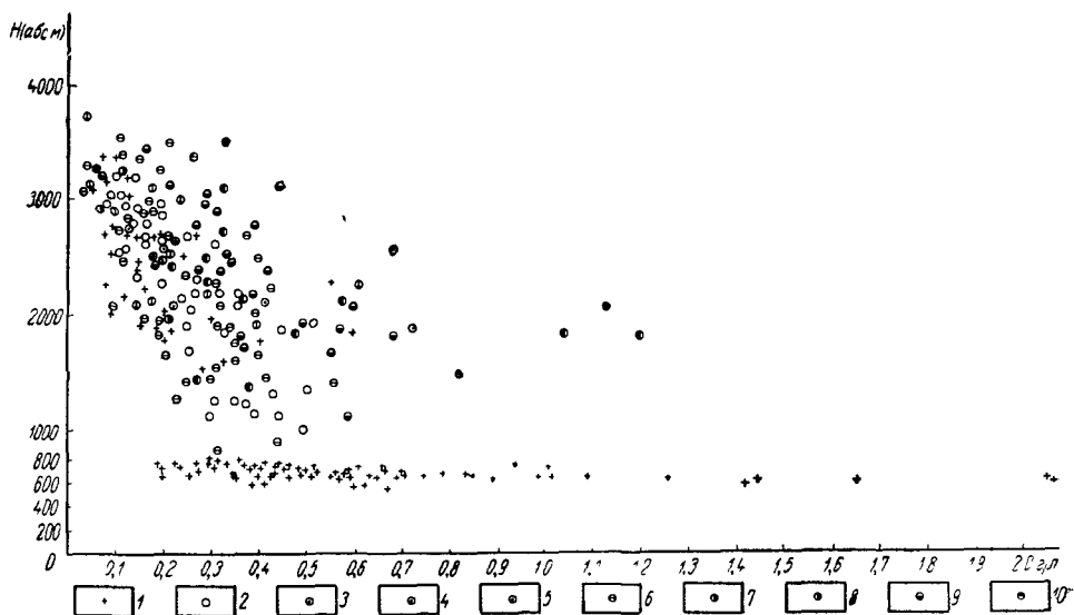
Рис. 24 Изменение величины общей минерализации грунтовых вод с изменением абсолютной высоты (для Чуйского бассейна подземного стока) 1 — в четвертичных отложениях, 2 — в известняках нижнего карбона, 3 — в сланцах верхнего протозоя, 4 — в молассах палеоген-неогена, 5 — в порфиритах и сланцах ордовика, 6 — в гранитоидах палеозоя, 7 — в песчаниках и сланцах девона, 8 — в сланцах силура, 9 — в сланцах, гранулитях и гнейсах кембрия, 10 — в конгломератах неоген-древнетчетвертичного времени
