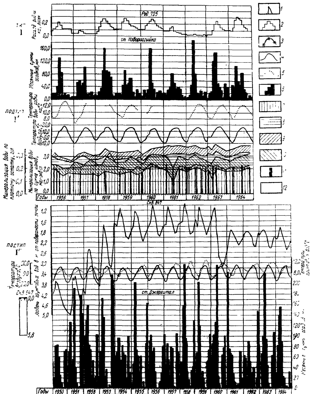
Графики климатического типа (I) режима подземных вод
