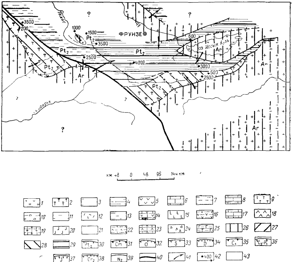
Рис. 30. Палеогидрогеологические схемы Тянь-Шаня (по Е. И. Лагутину, 1966)
