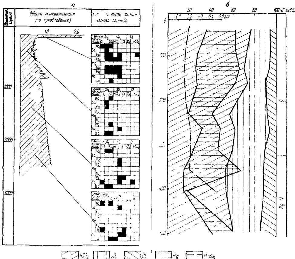
Рис 23 Вертикальная гидрохимическая зональность внутренней части Чуйского бассейна подземного стока а — в целом для бассейна, б — для района Саргоу
