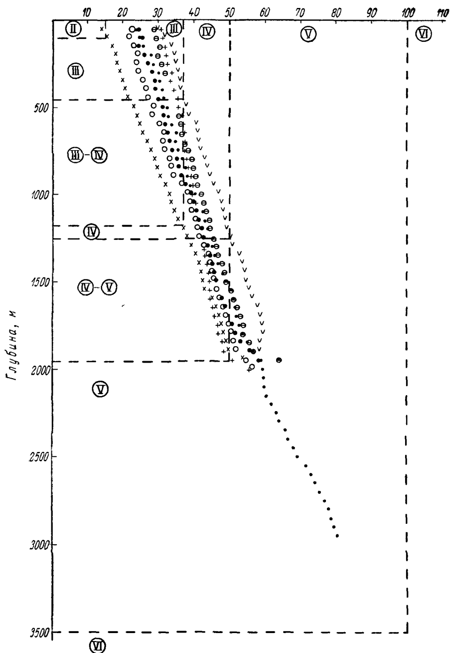
Рис. 29. Зависимость температуры подземных вод от глубины их залегания ный Избаскент (сле II-VI — номера
