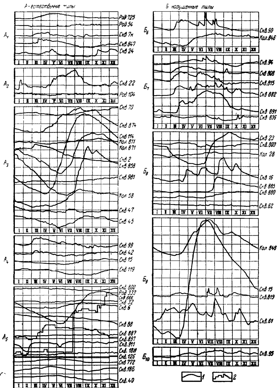
Рис. 16. Сводные графики генетических типов режима подземных вод Киргизской ССР. Масштабы вертикальные: колебаний уровня — в одном делении шкалы 1 м расхода 0,4 л/сек.
