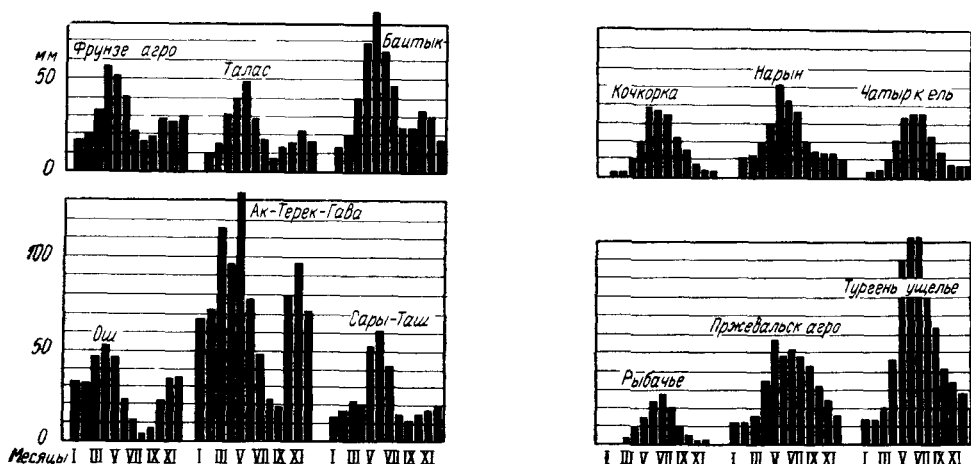
Рис. 4 Годовой ход осадков (по З. А. Рязанцевой, 1962)
