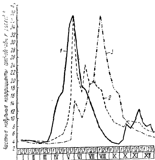
Рис. 3. Гидрографы рек Киргизской ССР для основных типов питания (по М. Н. Большакову, 1962).
