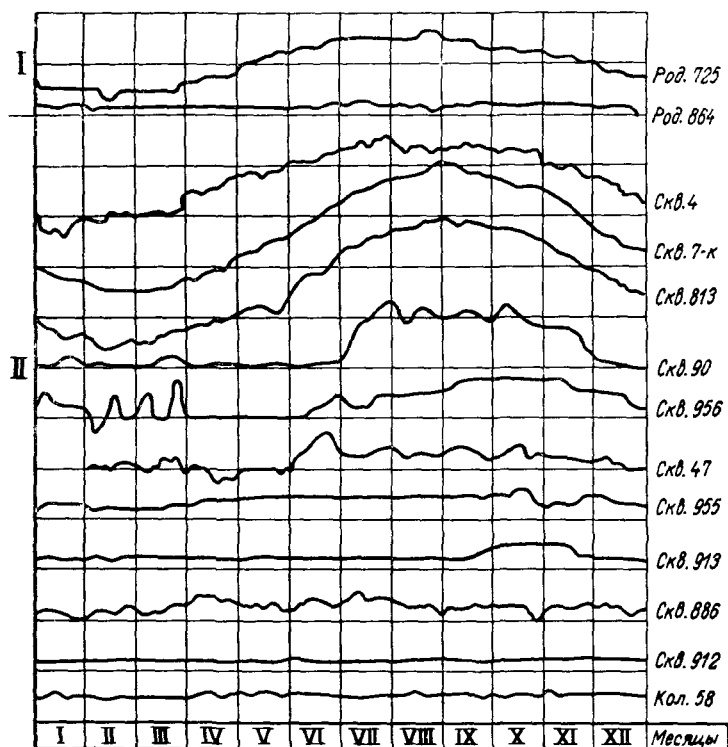
Рис. 20. Графики сезонных изменений температуры грунтовых вод в Чуйском бассейне в зависимости от глубины их залегания.
