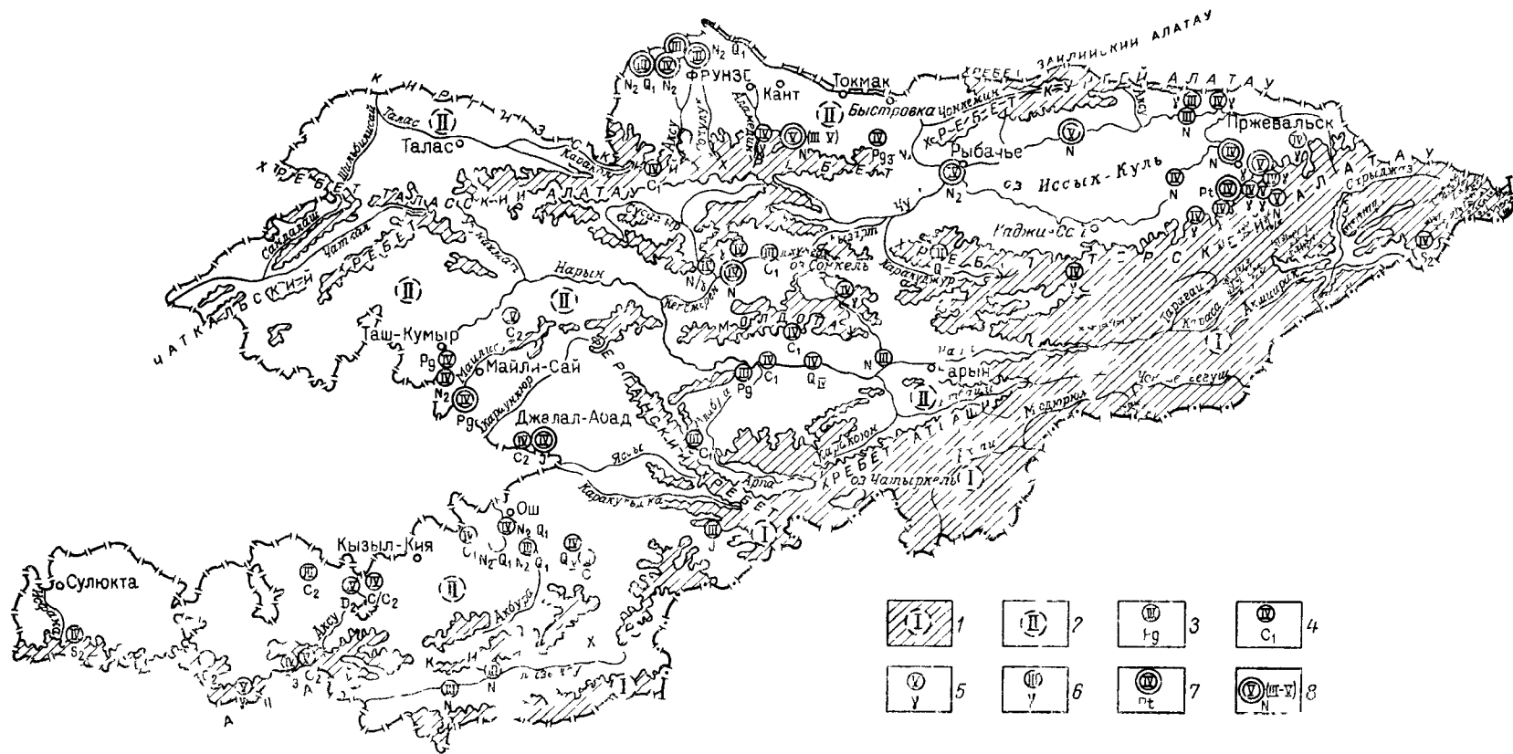
Рис. 26 Схема распространения вертикальных гидротермических зон Киргизской ССР
