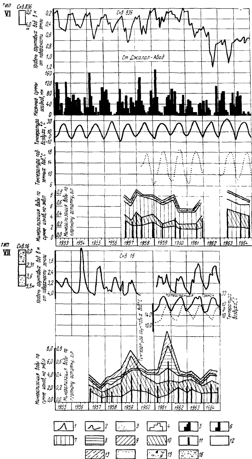
Рис. 18. Графики ирригационного (V), ирригационно-климатического (VI), ирригационно-гидрогеологического (VII) и ирригационно-гидрологического (VIII) типов режима подземных вод. V тип. Кол. 846—Кугартская впадина, третья терраса р. Кугарт; скв. 90—Чуйская впадина, северо-западная часть пролювиально-аллювиальной равнины; VI тип. Скв. 836—Ферганская впадина; VII тип. Скв. 16—Чуйская впадина, вторая левобережная терраса р. Чу. VIII тип. Кол. 848—долина р. Караункюр. Среднемесячные значения: 1—уровня, 2—температуры воздуха, 3—температуры грунтовых вод, 4—расхода рек; 5—месячная сумма осадков; 6—водоподача на орошение; инградиенты химического состава подземных вод: 7— \text{HCO}_3 , 8— \text{SO}_4 , 9— \text{Cl} , 10— \text{Mg} ; 11—плотный остаток; 12—суглинок, 13—супесь, 14—песок, 15—гравийно-галечник, 16—галечник
