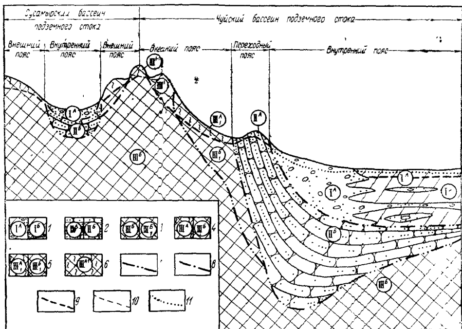
Рис. 21. Принципиальная схема вертикальной гидродинамической зональности подземных вод на примере Чуйского и Сусамырского бассейнов подземного стока. Внутренние и переходные части: 1 — гидродинамический этаж поровых вод — с гидродинамическими зонами безнапорных вод (IА) и напорных вод (IБ); 2 — гидродинамический этаж порово-трещинных вод с гидродинамическими зонами безнапорных (грунтовых) вод (IIА) и высоконапорных вод (IIБ), 3 — гидродинамическая зона высоконапорных вод этажа трещинных вод (IIIБ) и подэтажа пластово-трещинных вод (IIIБ), 4 — гидродинамический этаж трещинных вод с гидродинамическими зонами безнапорных (интенсивной трещиноватости) вод (IIIА) и высоконапорных вод глубокой циркуляции (IIIБ); 5 — гидродинамический подэтаж пластово-трещинных вод с гидродинамическими зонами безнапорных вод открытой трещиноватости (IIIА) и высоконапорных вод глубокой циркуляции (IIIБ); 6 — слабо изученная в гидрогеологическом отношении гидродинамическая подзона многолетнемерзлых пород (IIIА-1). Границы: 7 — гидродинамических этажей, 8 — подэтажей, 9 — зон, 10 — подзон, 11 — уровень грунтовых вод
