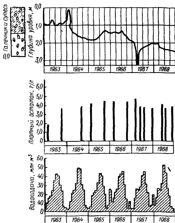
Рис. 72. Режим уровня и изменение минерализации грунтовых вод нижней части конуса выноса р. Исфара (скв. 37) в сопоставлении с водоподачей на орошение
