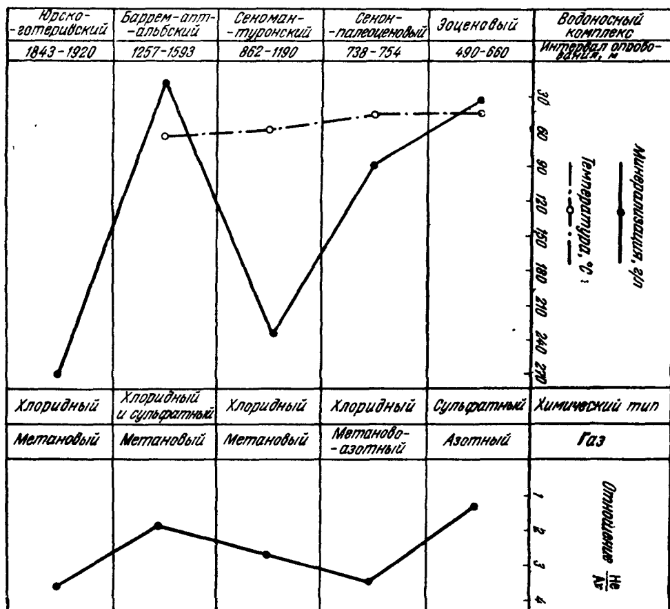
Рис. 50. Характеристика пластовых вод структуры Любоб
