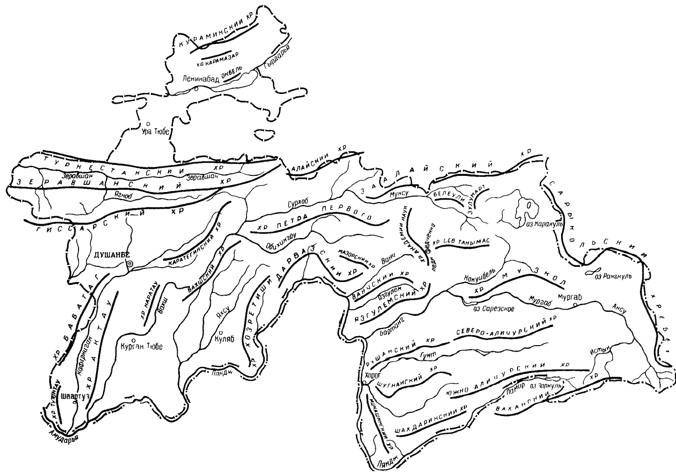
Рис. 2. Орогидрографическая схема
