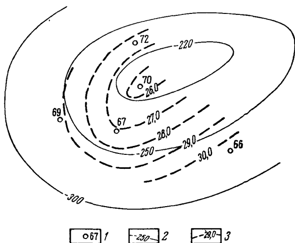
Рис. 70. Схема изменения геотермической ступени неогеновых отложений на площади Шаамбары, масштаб 1 : 25 000:
