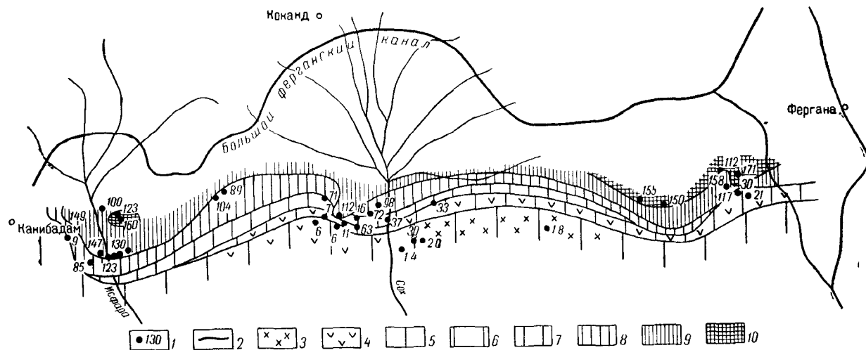
Рис. 33. Схематическая гидрохимическая карта вод II пласта палеогеновых отложений: 1 — скважина, цифра — минерализация, 2 — южная граница распространения вод хлоридного кальцевого типа; 3 — воды гидрокарбонатного натриевого типа; 4 — воды сульфатного натриевого типа. Минерализация вод, г/л: 5 — 1—10, 6 — 10—35; 7 — 35—75; 8 — 75—100, 9 — 100—150, 10 — >150
