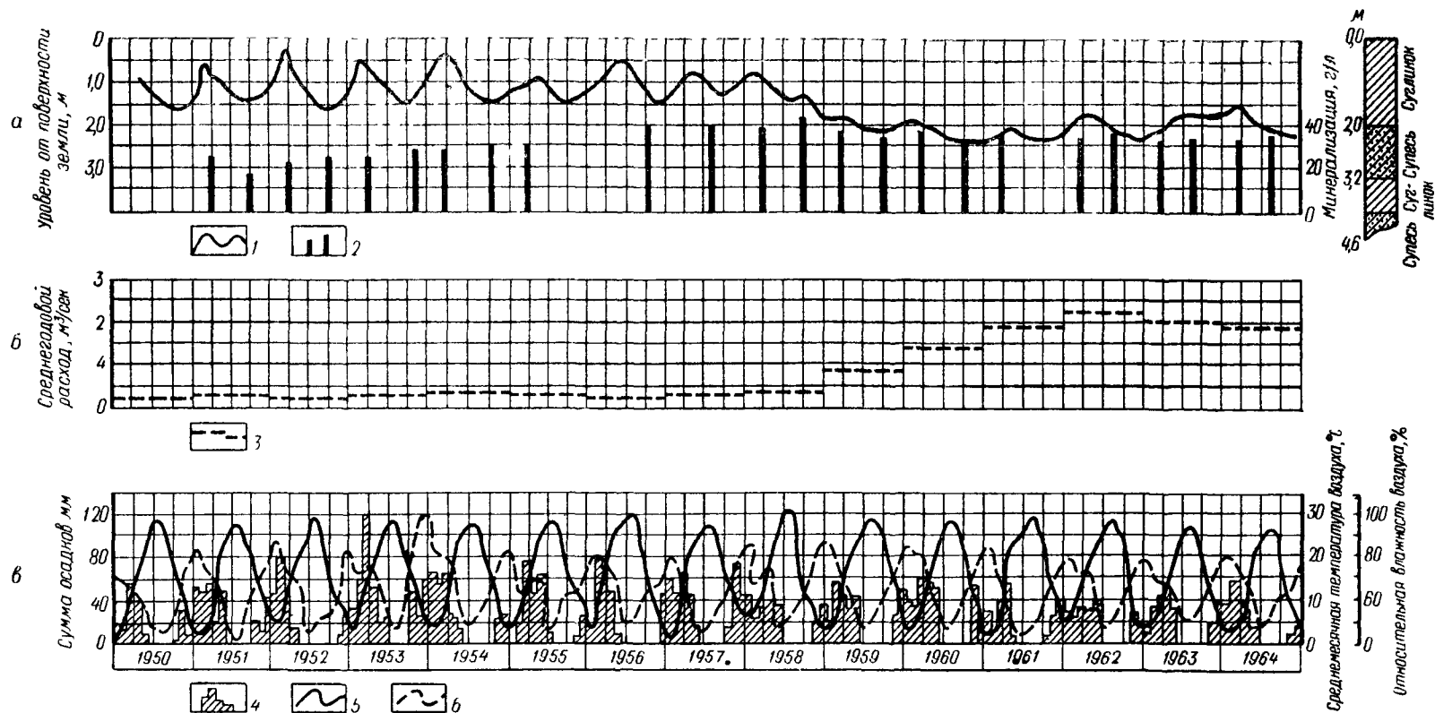
Рис. 80. Режим уровня грунтовых вод и изменение их минерализации для естественно дренируемых площадей третьей террасы р. Вахш в сопоставлении с климатическими факторами и коллекторно-дренажным стоком: а — солончаки Карагайского понижения в 500 м от Центрального сброса и в 350 м от коллектора В-7 (скв. 188); б — коллектор В-7; в — метеорологические данные 1 — уровень от поверхности земли, м, 2 — минерализация грунтовых вод, г/л; 3 — кривая среднегодового расхода коллектора В-7, м³/сек, 4 — осадки, мм; 5 — температура воздуха, °С, 6 — относительная влажность, %
