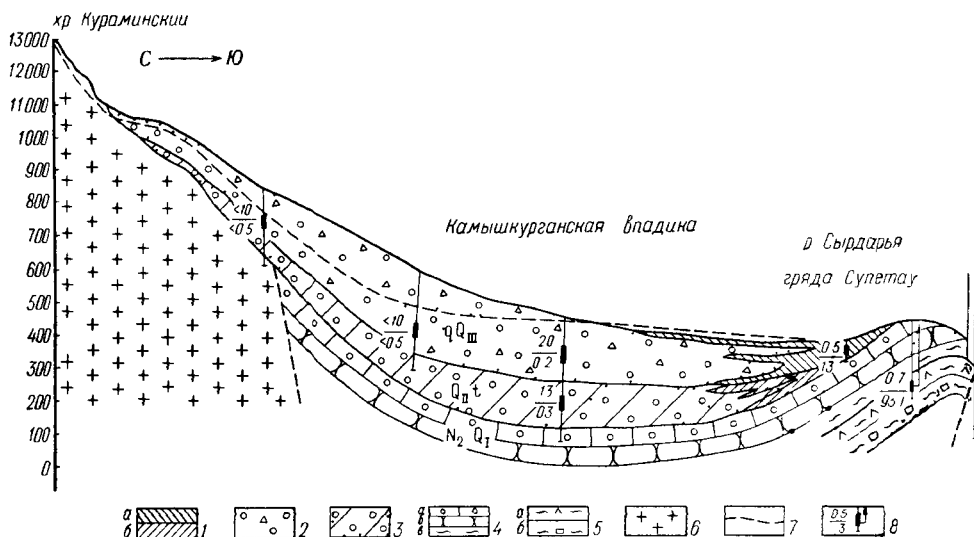
Рис 29 Схематический гидрогеологический разрез Камышкурганской впадины
