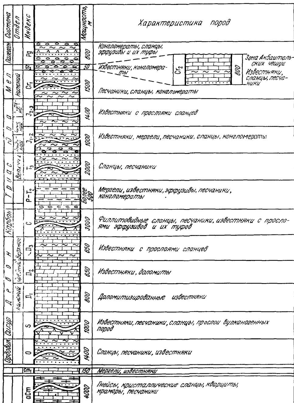
Рис. 20. Сводная стратиграфическая колонка пород зоны Центрального Памира
