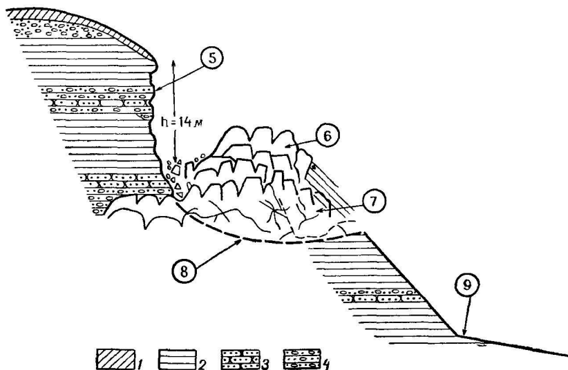
Рис. 86. Инсеквентный деплясивный оползень на северных склонах предгорий Зеравшанского хребта:
