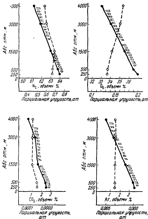
Рис. 58. Зависимость содержания компонентов воздуха, способных раствориться в воде на различной высоте (расчетные величины)
