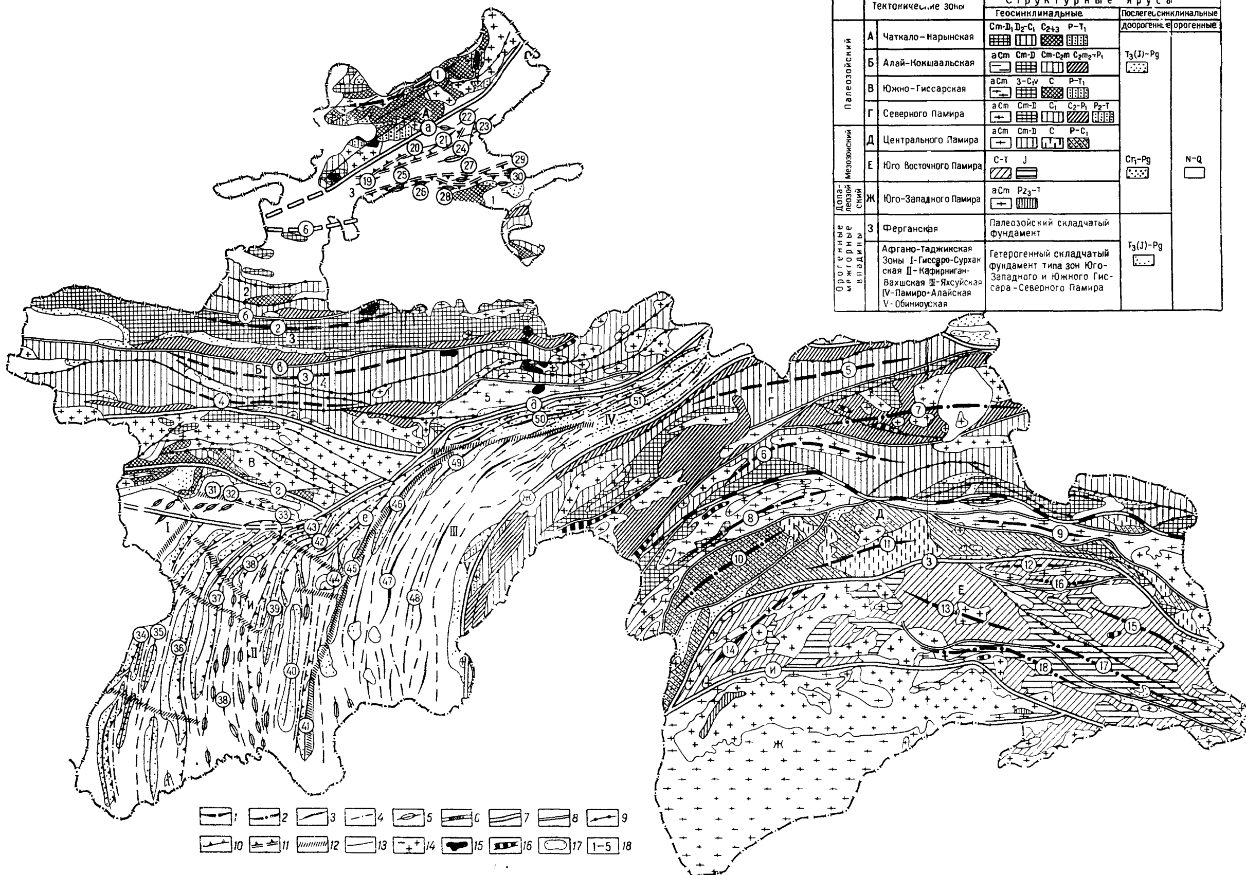
Рис. 12. Тектоническая схема территории Таджикской ССР. Составил Я. А. Беккер, по Б. П. Бархатову (Памир), П. Д. Виноградову, М. М. Кухтикову, А. П. Марковскому, Д. П. Резвому, Н. М. Синицину, П. К. Чихачеву
