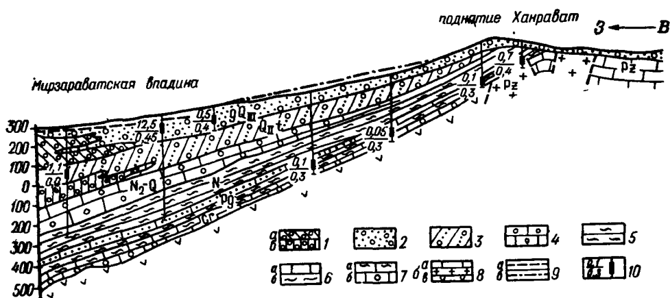
Рис. 24. Гидрогеологический разрез Мирзаватской впадины
