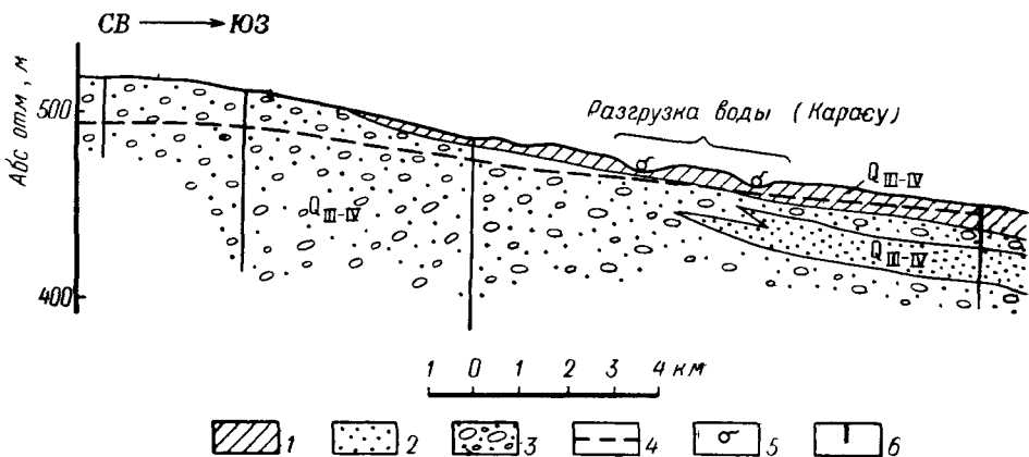
Рис. 37. Продольный гидрогеологический профиль через Пянджский конус выноса: 1 — суглинки, 2 — пески; 3 — галечники, 4 — уровень подземных вод со свободной поверхностью, 5 — родник; 6 — скважина
