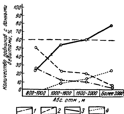
Рис. 40. Распределение родников с разными дебитами по ярусам рельефа Фоновые дебиты, л/сек 1 — <0,01, 2 — 0,01—0,1; 3 — 0,1—1 4 — >1
