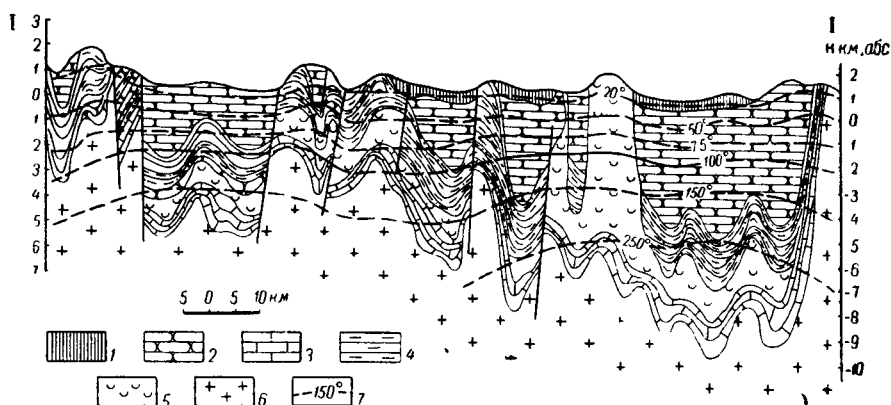
Рис. 69. Схематический геотермический разрез по линии I—I (см. рис. 68)
