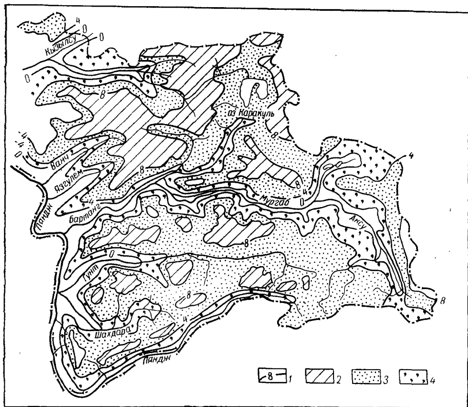
Рис. 88. Схематическая карта распространения многолетней мерзлоты (по Я. Я. Сердюку): 7 — изотермы многолетних среднегодовых температур; 2 — районы повсеместного распространения многолетнемерзлых пород; 3 — районы спорадического распространения многолетнемерзлых пород; 4 — районы деградации многолетнемерзлых пород
