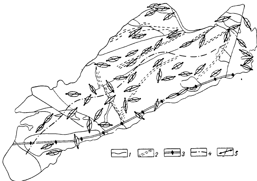
Рис. 25. Основные направления максимально приоткрытых трещин магматических пород верхнего палеозоя (Северо-Таджикский регион, горы Моголтау):
