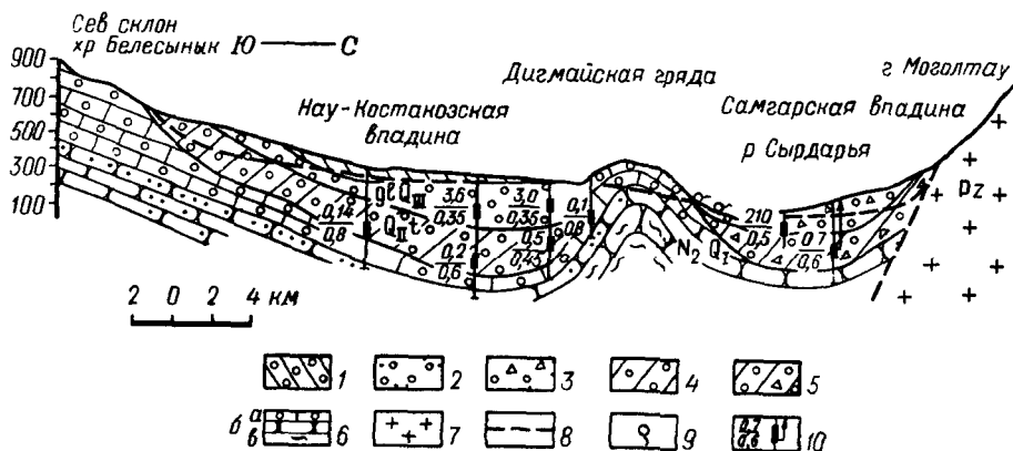
Рис 28 Схематический гидрогеологический разрез Нау-Костакоской и Самгарской впадин
