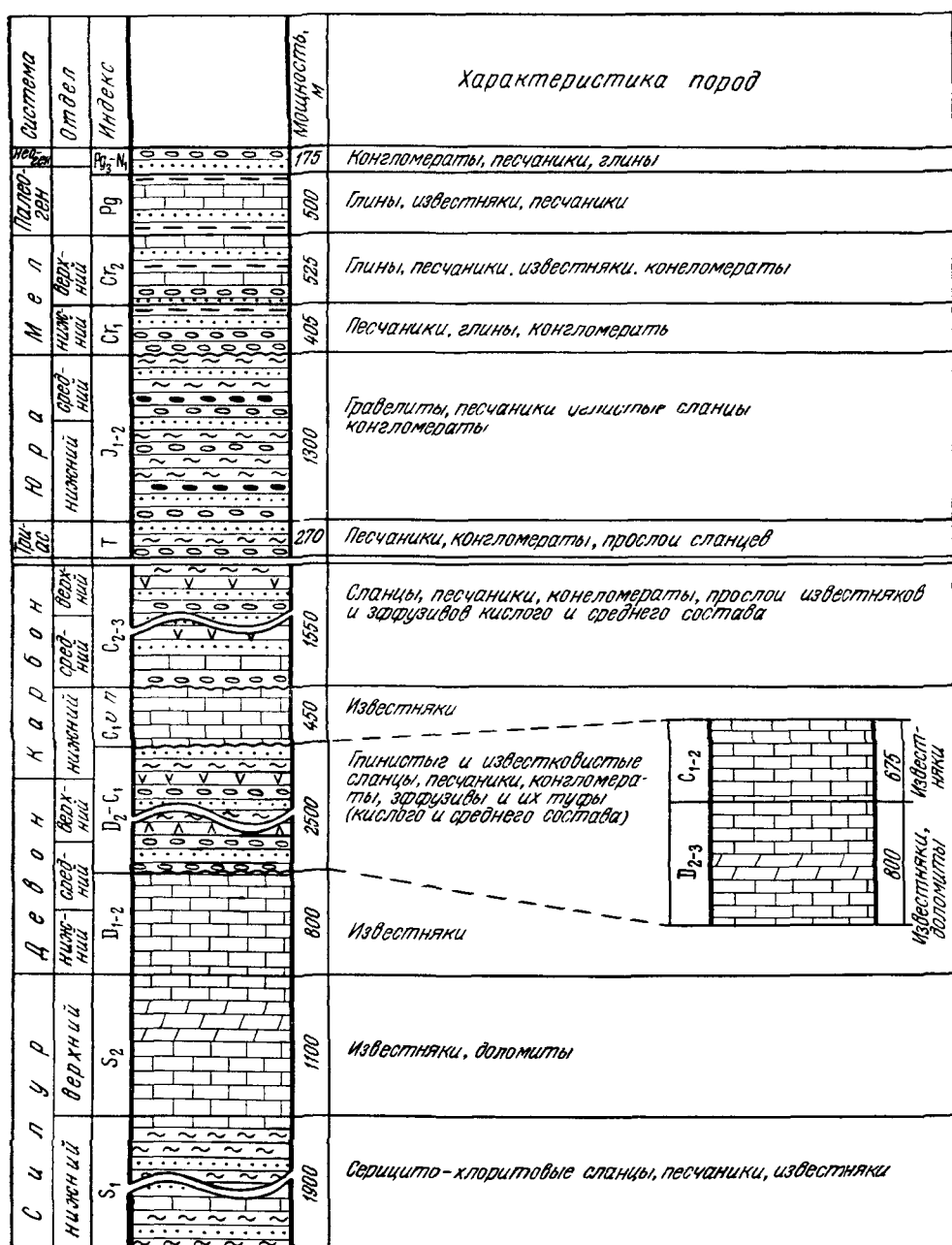
Рис. 16. Сводная стратиграфическая колонка пород Зеравшано-Гиссарской подзоны
