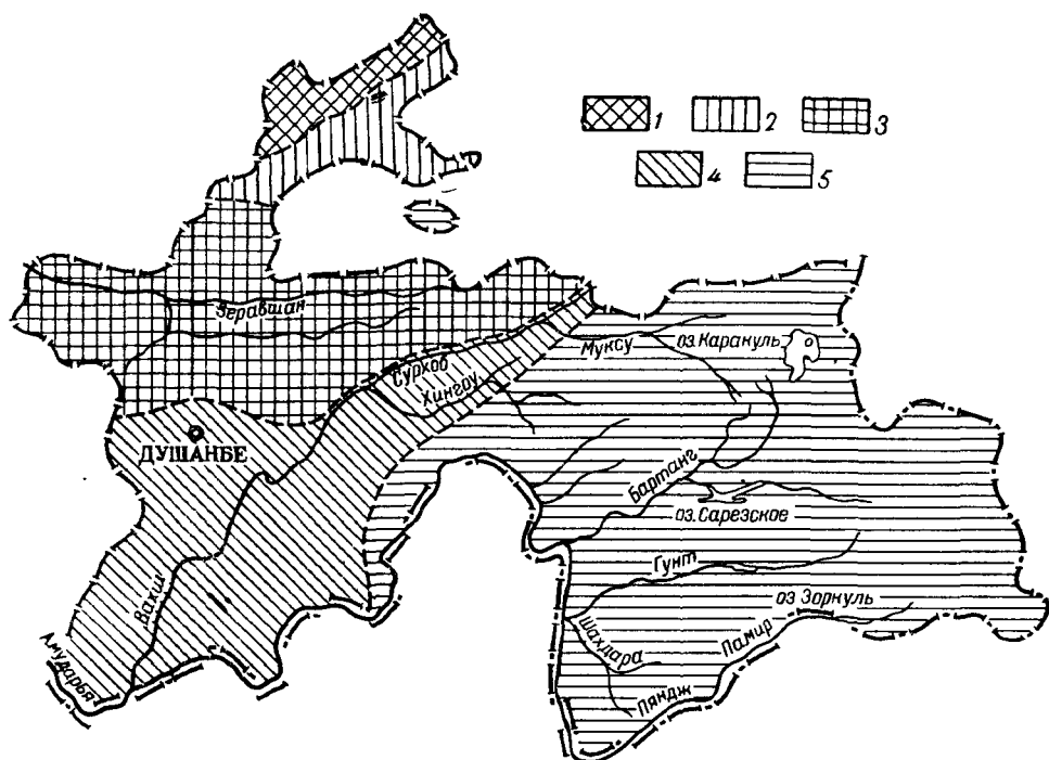
Рис. 1. Схема основных районов Таджикистана
