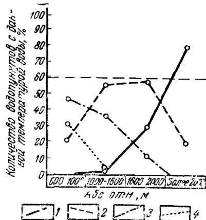
Рис. 43. Распределение родников с различной температурой воды по ярусам рельефа
