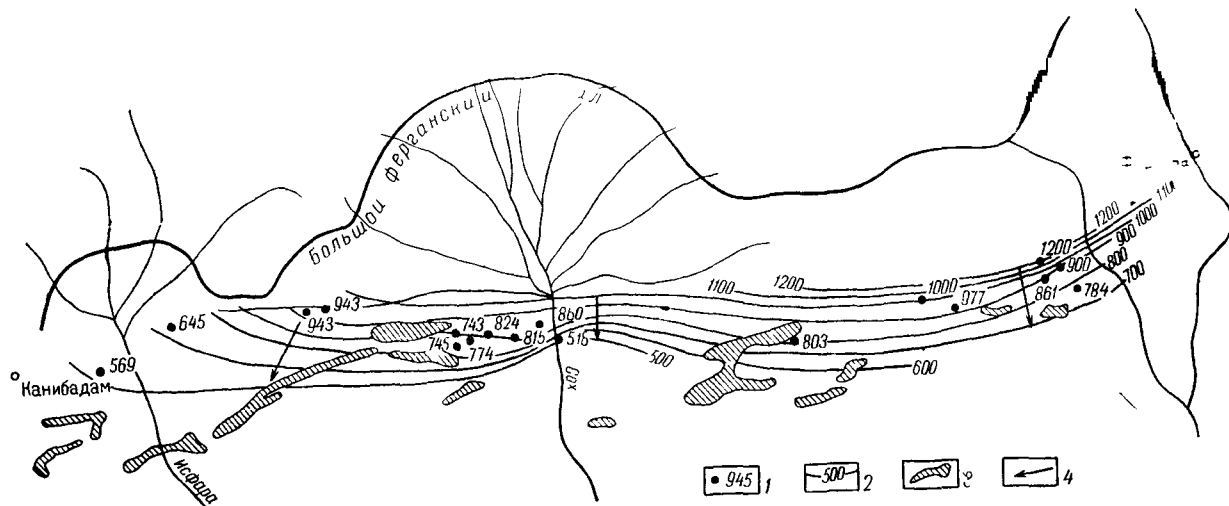
Рис. 32. Схематическая карта приведенных напоров вод у подошвы II пласта: 1 — скважина, цифра — приведенный напор; 2 — изолинии приведенных напоров; 3 — выходы палеогеновых пород; 4 — предполагаемое направление движения подземных вод
