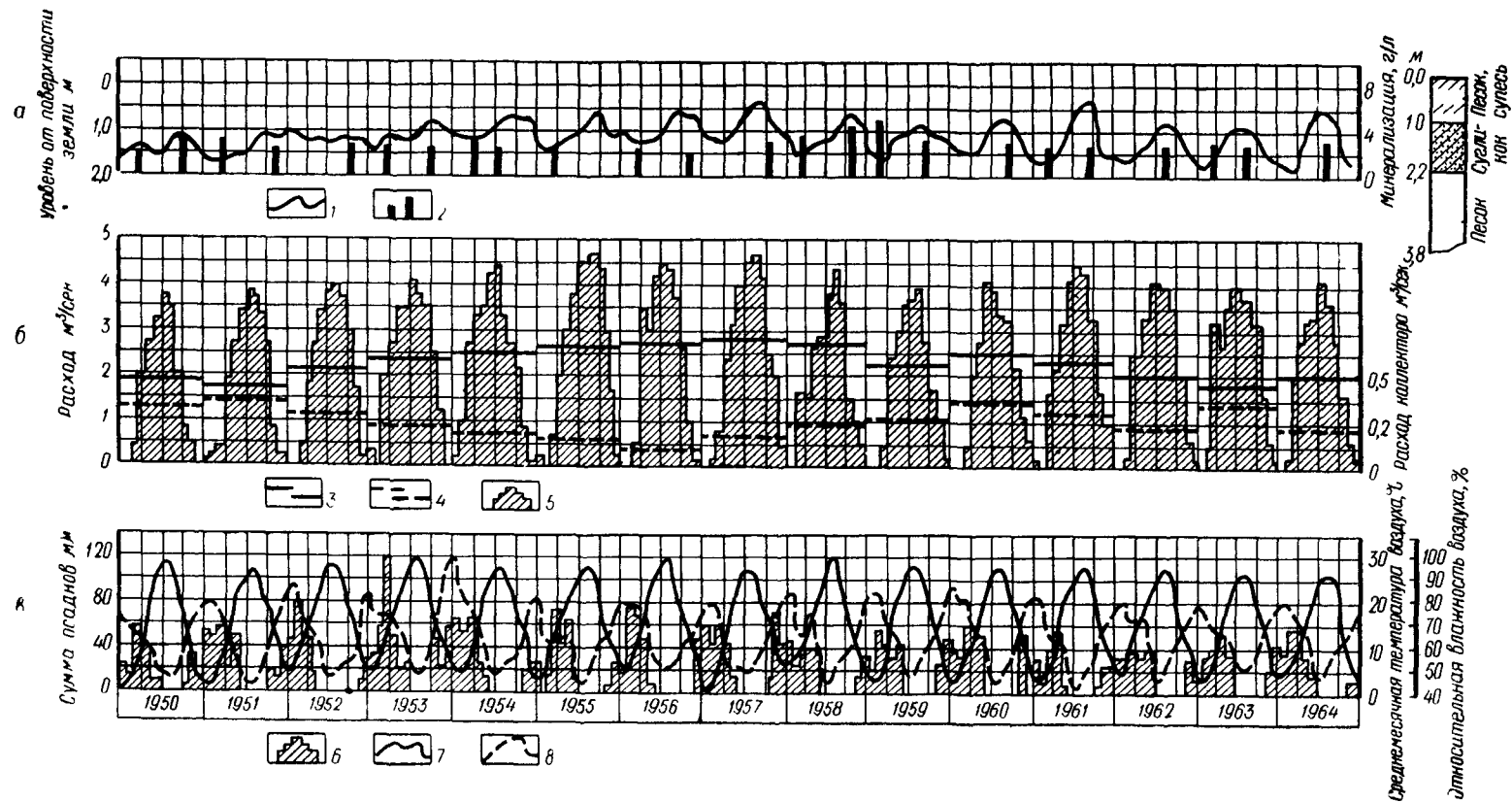
Рис 78 Режим уровня грунтовых вод и изменение их минерализации для естественно слабодренированных площадей третьей террасы р Вахш в сопоставлении с водоподачей на орошение и климатическими факторами
