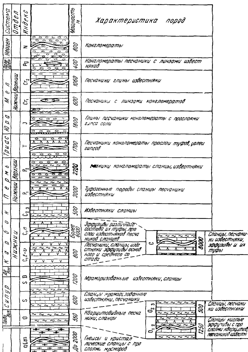
Рис 19 Сводная стратиграфическая колонка пород зоны Северного Памира
