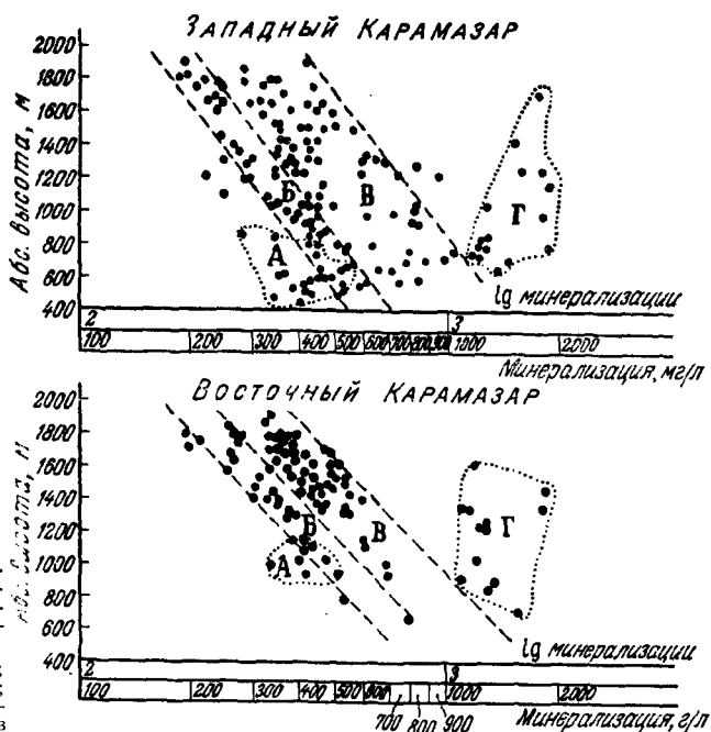
Рис. 26. Зависимость минерализации воды от гипсометрического положения водопункта (Северо-Таджикский регион):
