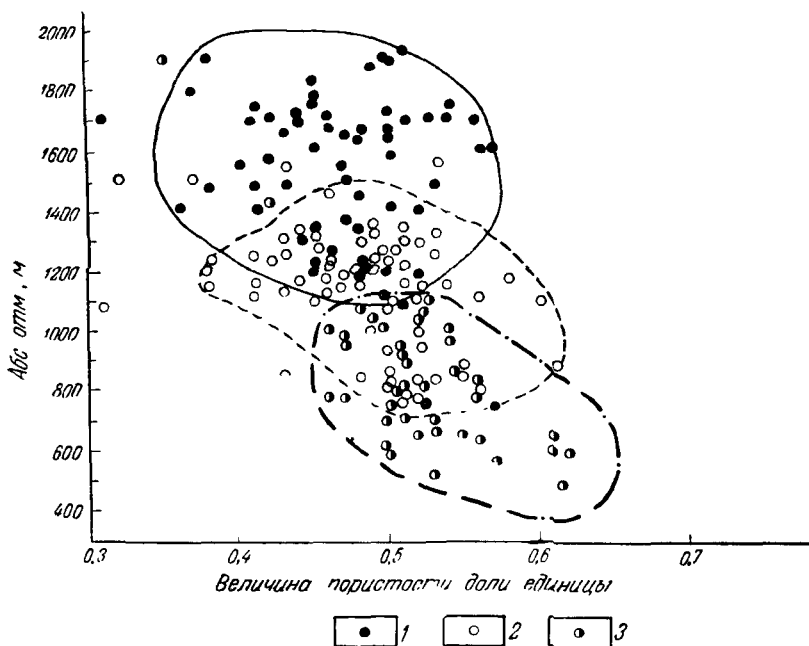
Рис. 38. Зависимость пористости лёссовидных пород от гипсометрии 1 — Q^1_{II} ; 2 — Q^2_{II} ; 3 — Q^3_{II}
