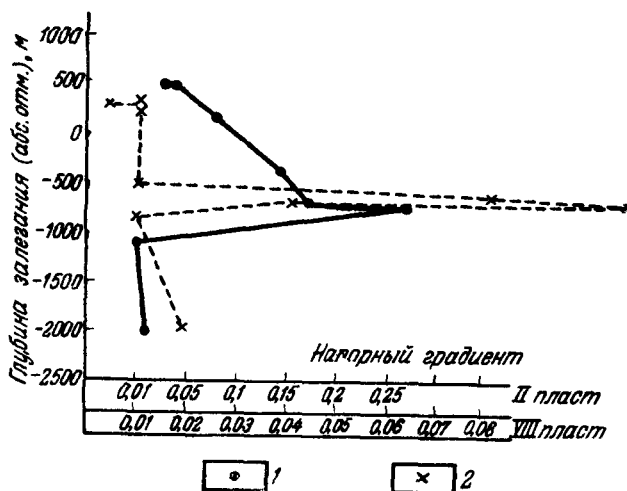
Рис. 34. Изменение напорного градиента в зависимости от глубины залегания водоносного горизонта Напорный градиент: 1 — II пласта; 2 — VIII пласта
