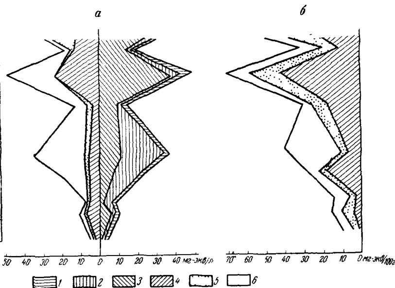
Рис. 56. Сопоставление содержания катионов в водных вытяжках и в поглощенном состоянии (породы глубоких частей разреза структуры Андыген) а — состав водных вытяжек, б — состав поглощенных катионов 1 — \text{HCO}_3 , 2 — \text{SO}_4 , 3 — \text{Cl} , 4 — \text{Na} , 5 — \text{Mg} , 6 — \text{Ca}
