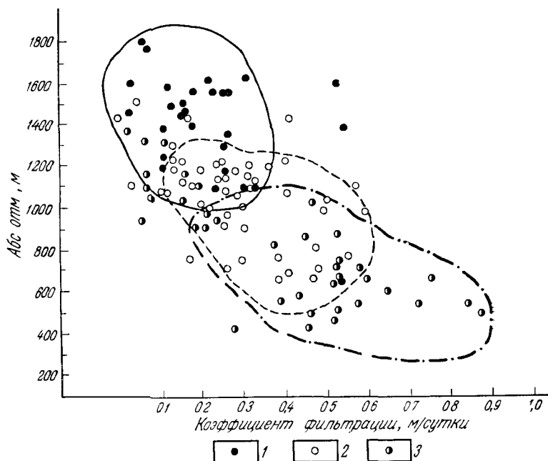
Рис 39 Зависимость коэффициента фильтрации лессовидных пород от гипсометрии 1 — Q^I_{II} 2 — Q^2_{II} 3 — Q^3_{II}
