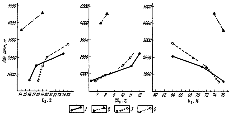
Рис 61. Зависимость средневзвешенных содержаний компонентов растворенных газов подземных вод от гипсометрического положения водопункта
