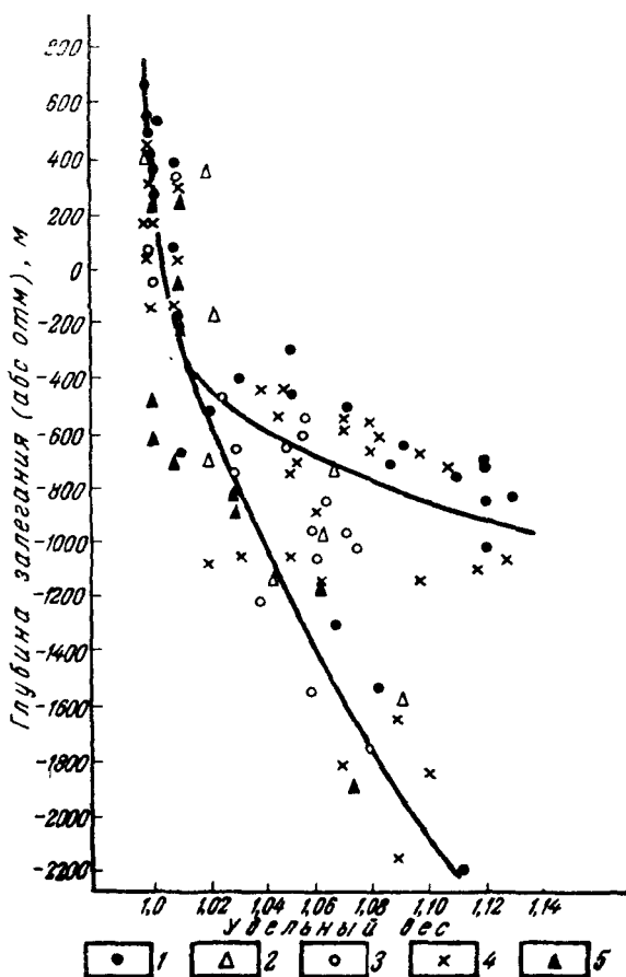
Рис. 31. Изменение удельного веса подземных вод палеогена в зависимости от глубины залегания водоносного горизонта
