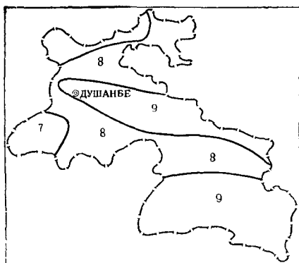
Рис. 83. Схема сейсмического районирования Таджикистана (цифрами показана балльность)
