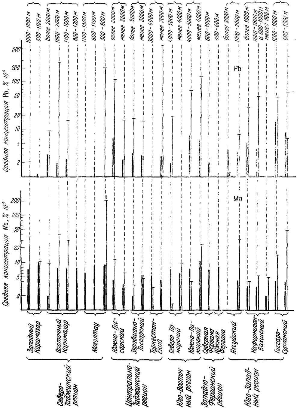
Рис. 57. Изменение средних концентраций свинца и молибдена в подземных водах на различных гипсометрических уровнях 1 — средняя фоновая концентрация; 2 — средняя аномальная концентрация
