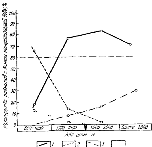
Рис. 41. Распределение родников с различной минерализацией воды по ярусам рельефа Фоновая минерализация, г/л 1 — <0,1 2 — 0,1—1, 3 — 1—3, 4 — >3
