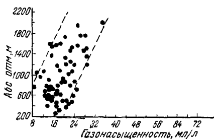
Рис. 60. Зависимость основных параметров газового состава от гипсометрического положения водопункта
