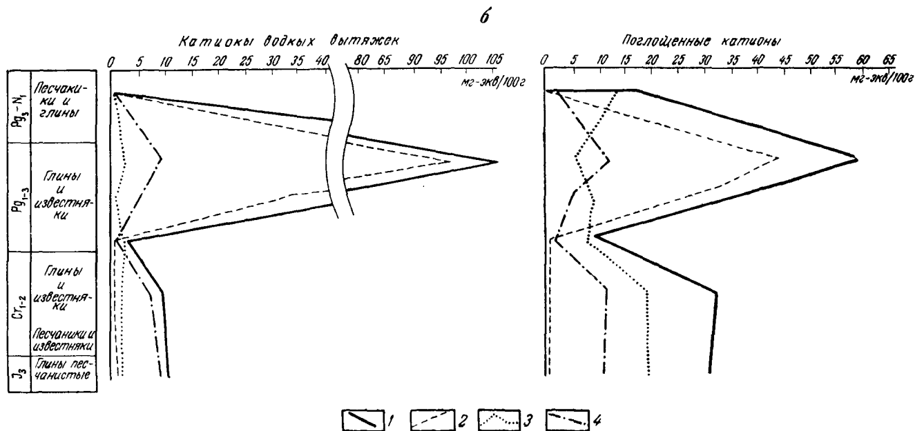
Рис. 53. Сопоставление содержания катионов в водных вытяжках и в поглощенном состоянии (кора выветривания в разных климатических зонах)
