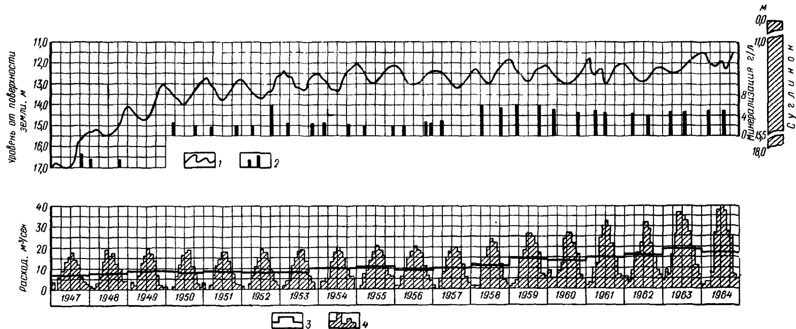
Рис. 75. Режим уровня грунтовых вод и изменение их минерализации для естественно дренированных площадей четвертой террасы р. Вахи в сопоставлении с водоподачей на орошение. Орошаемые земли левого бережья находятся в 30 м от канала Кумсангыр (скв. 24):
