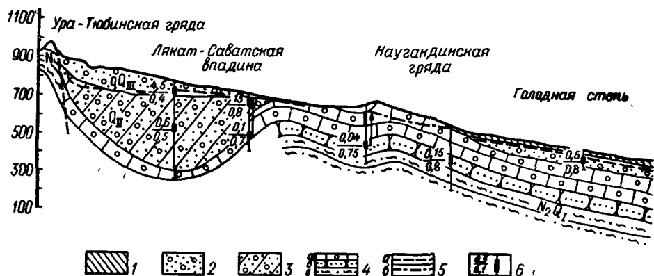
Рис. 30. Схематический гидрогеологический разрез Лякат-Саватской впадины
