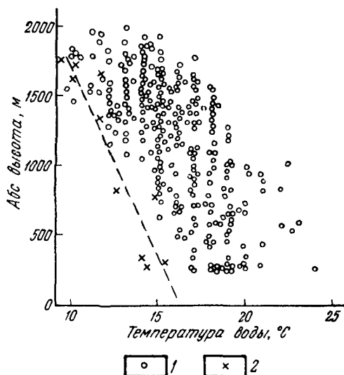
Рис. 27. Зависимость температуры воды от гипсометрического положения водопункта (Северо-Таджикский регион):
