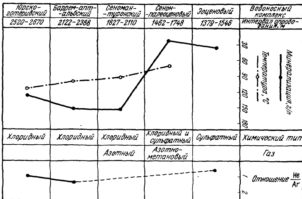
Рис. 51. Характеристика пластовых вод структуры Шаамбары
