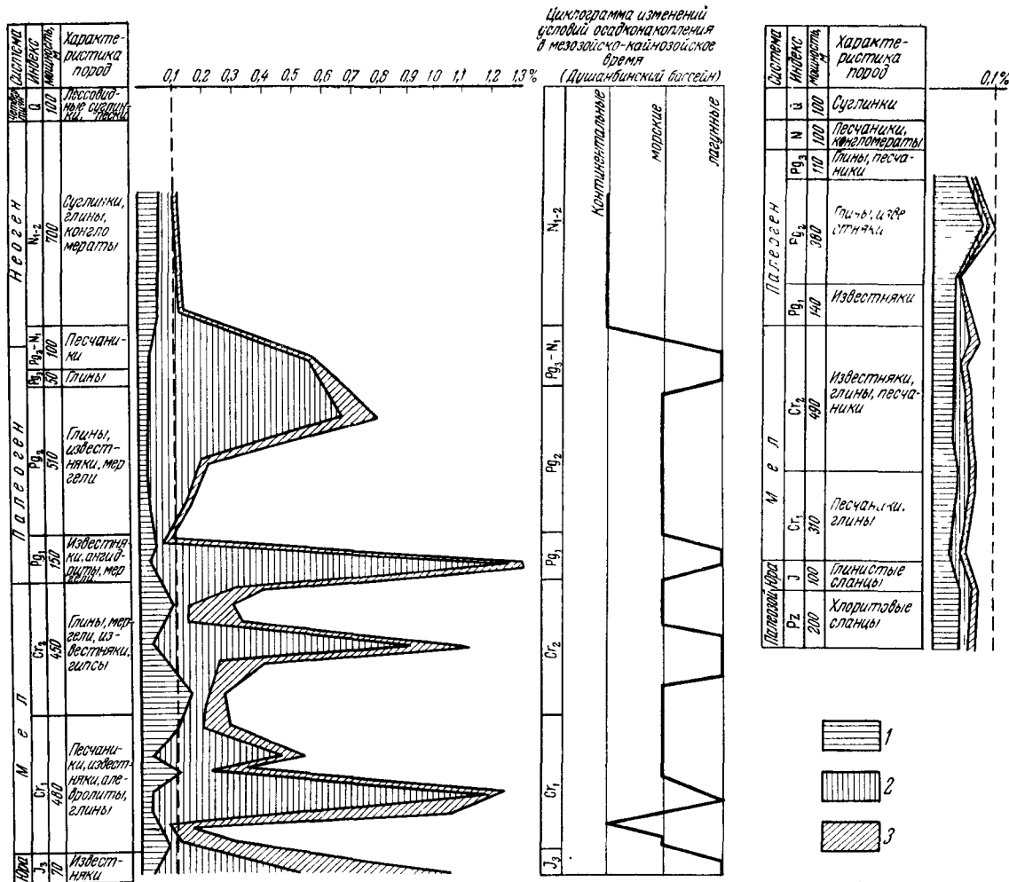
Рис. 54. Эпюры засоленности до-четвертичных пород коры выветривания и глубоких частей разреза Душанбинского артезианского бассейна
