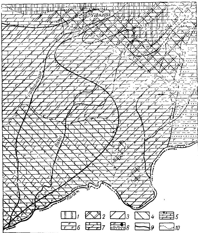
Рис. 45. Схема распространения различных типов бухарских отложений и приуроченных к ним подземных вод с различной минерализацией
