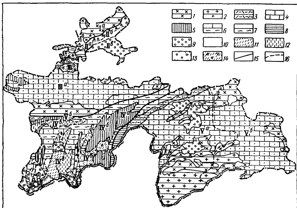
Рис. 89. Схема инженерно-геологического районирования Таджикистана:
