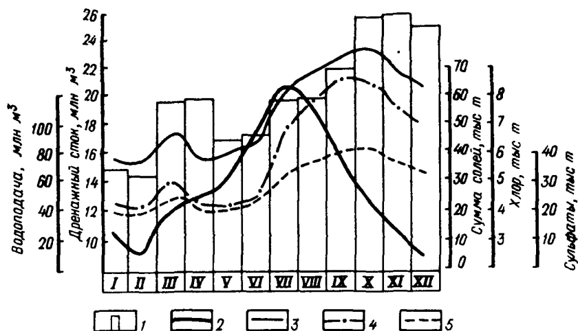
Рис. 73. Вынос солей дренажными водами с левобережья Кайраккумского водохранилища: 1 — дренажный сток, 2 — водоподача на орошение, 3 — сумма солей, 4 — хлор-ион, 5 — сульфат-ион
