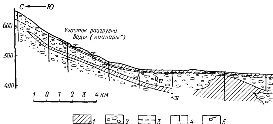
Рис 36 Продольный гидрогеологический профиль через долину реки Яхсу.
