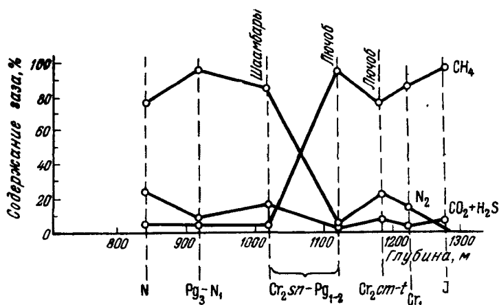
Рис. 62. Изменение газового состава подземных вод Душанбинского артезианского бассейна с глубиной
