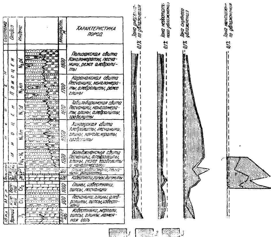
Рис. 44. Эпюры засоленности дочетвертичных пород в разных климатических зонах Гипотетические соли: 1 — гидрокарбонатные; 2 — сульфатные; 3 — хлоридные
