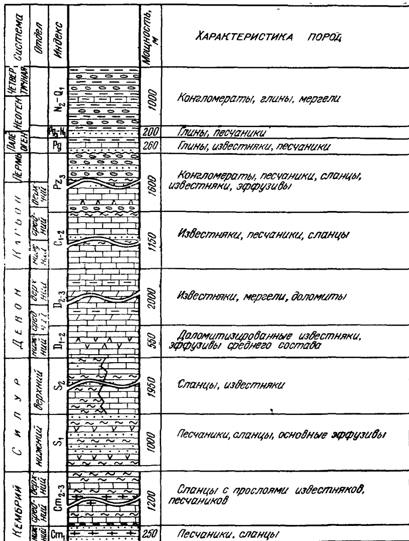
Рис. 14. Сводная стратиграфическая колонка пород Туркестано-Алайской подзоны
