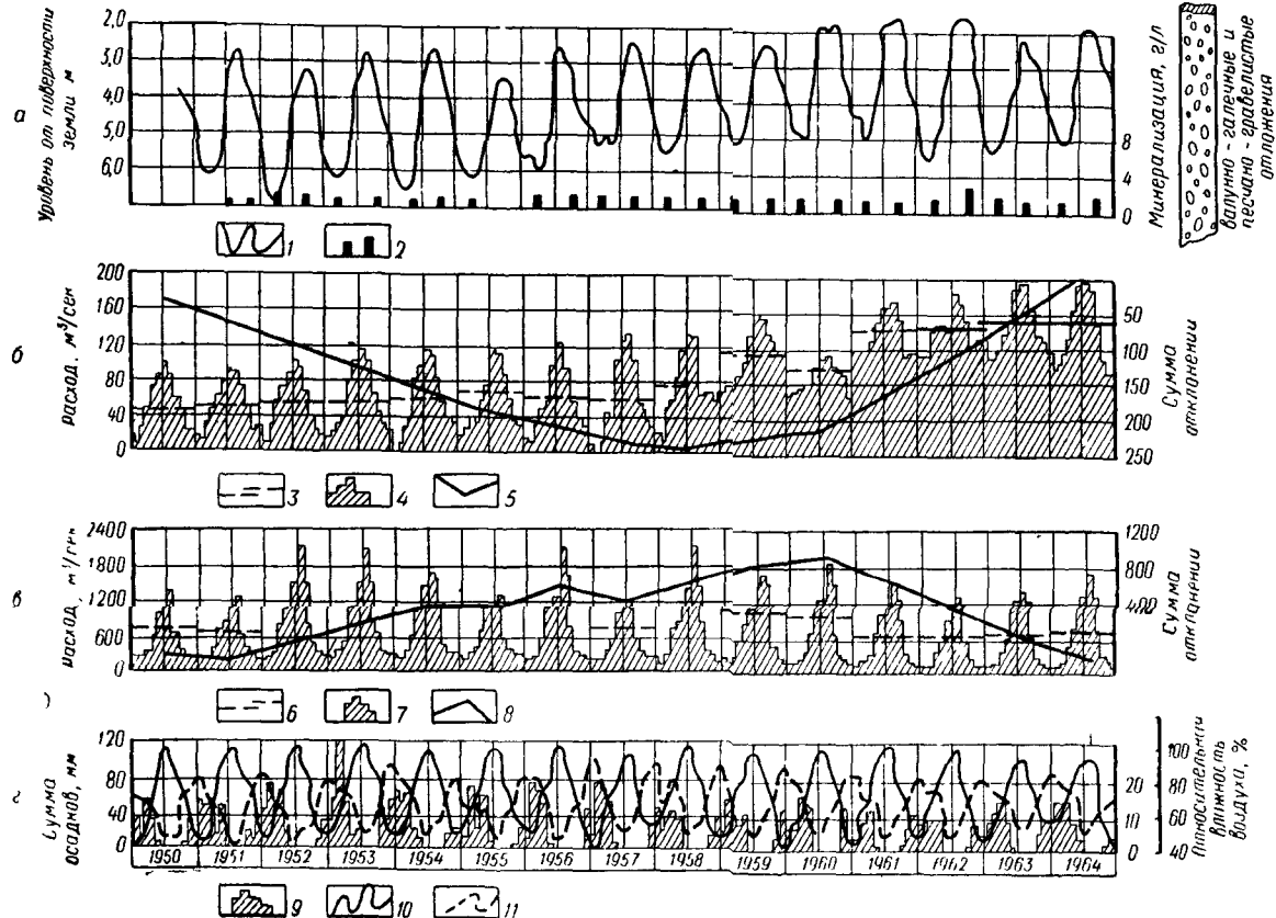
Рис. 77. Режим уровня грунтовых вод и изменение их минерализации на конусе выноса в сопоставлении с водоносностью р. Вахш, водоподачей на орошение и климатическими факторами:
