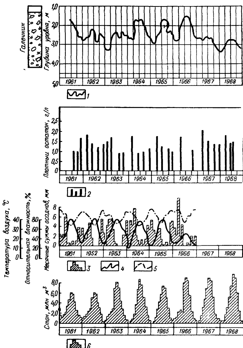
Рис 71 Режим уровня и изменение минерализации грунтовых вод южной части Нау-Костакозской впадины (скв 20 с) в сопоставлении с климатическими факторами и водоподачей на орошение
