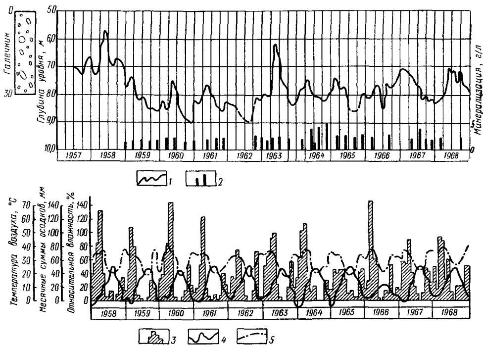
Рис. 74. Режим уровня и изменение минерализации грунтовых вод северной части Шахрнстанской впадины (скв. 8-кб) в сопоставлении с климатическими факторами (метеостанция Ура-Тюбе): 1 — уровень от поверхности земли, м, 2 — минерализация грунтовых вод, г/л, 3 — осадки мм, 4 — температура воздуха, °С, 5 — относительная влажность %
