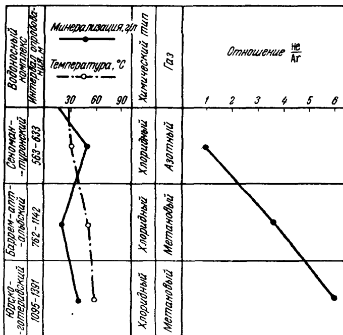
Рис. 49. Характеристика пластовых вод структуры Андыген
