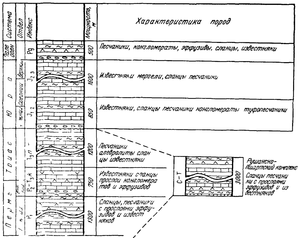
Рис 21 Сводная стратиграфическая колонка пород зоны Юго-Восточного Памира
