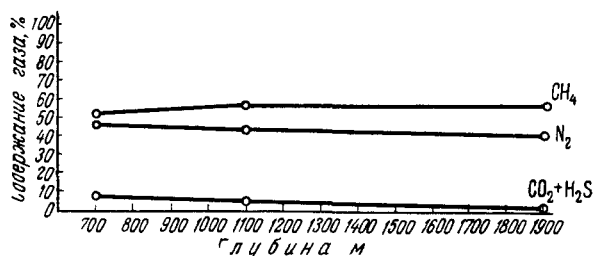
Рис. 63. Изменение газового состава подземных вод Вахшского артезианского бассейна (за исключением газонефте-носных горизонтов) с глубиной
