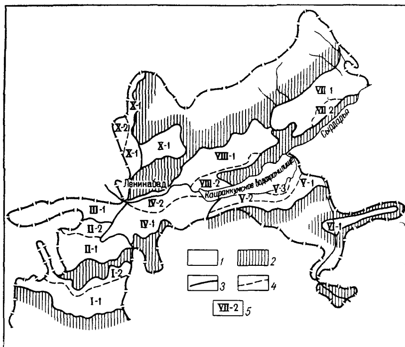
Рис. 81. Схема гидрогеолого-мелиоративного районирования орошаемых земель Северного Таджикистана:
