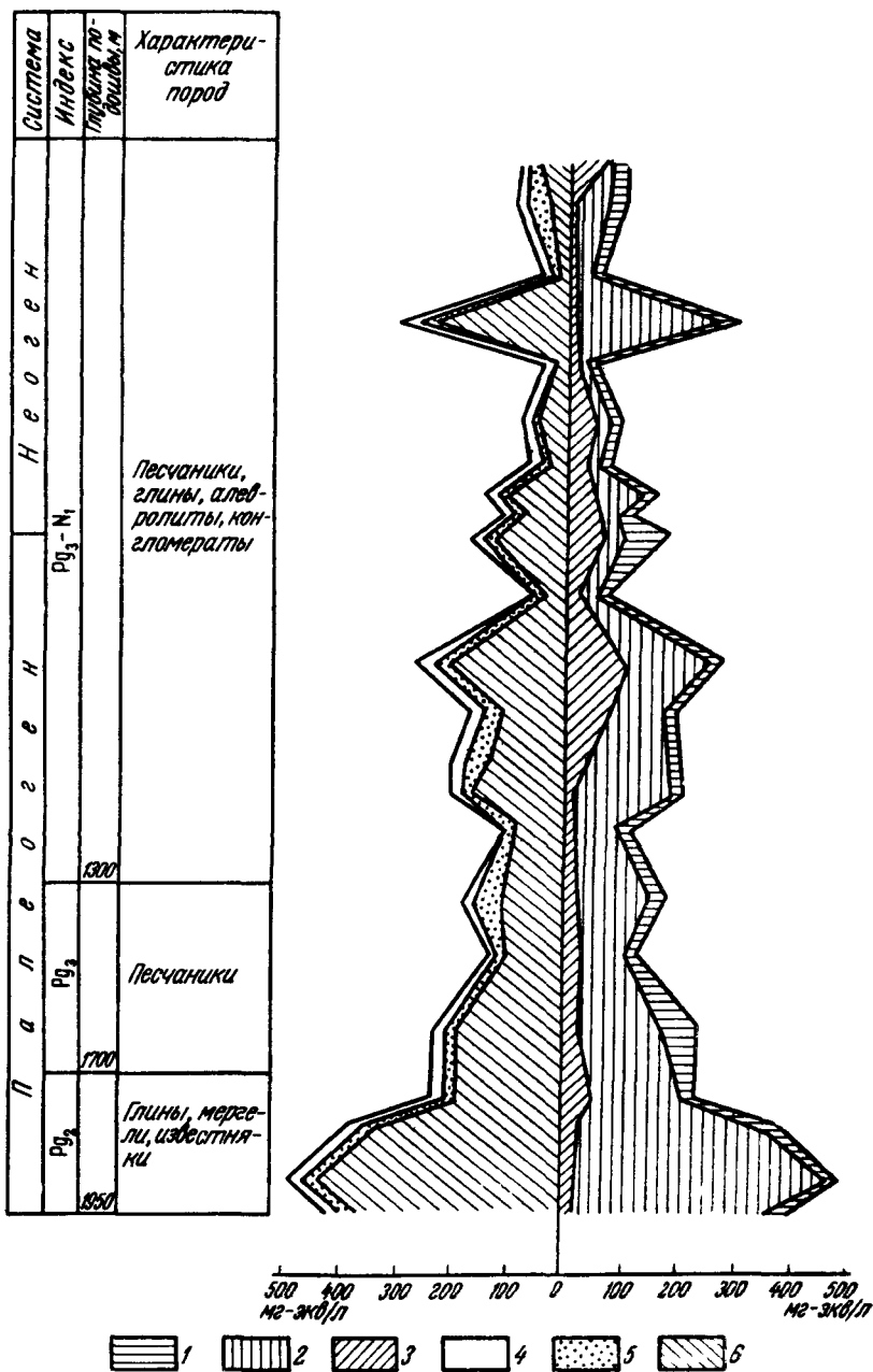
Рис. 55. Эпюры химического состава поровых растворов по скв. 2 структуры Каратаг
