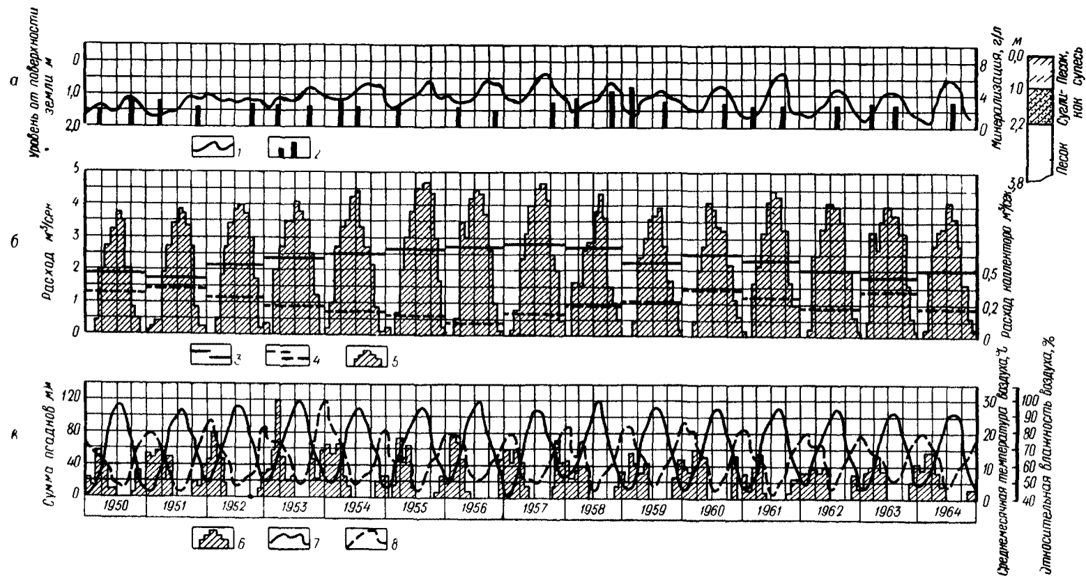
Рис 78 Режим уровня грунтовых вод и изменение их минерализации для естественно слабодренированных площадей третьей террасы р Вахш в сопоставлении с водоподачей на орошение и климатическими факторами а — орошаемые земли левобережья в 250 м от коллектора В Д II и в 250 м от канала «Ветка переключения» (скв 56) б — канал «Ветка переключения» в метеорологические данные 1 — уровень от поверхности земли, м 2 — минерализация грунтовых вод, г/л 3 — кривая среднеговегационного расхода канала «Ветка переключения», м³/сек 4 — кривая среднегодового расхода коллектора В Д II, м³/сек 5 — водоподача на орошение, м³/сек 6 — осадки, мм 7 — температура воздуха, °C 8 — относительная влажность воздуха, %
