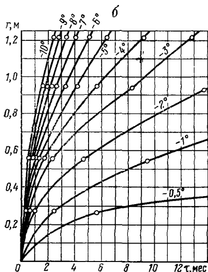
Рис. 80. Продолжительность промерзания ( \tau , месяцы) затрубных таликов различного радиуса ( r , метры), в зависимости от состава и температуры ( t , градусы) пород. а — влажность пород t_0 W = 200 кг/м 3 , теплопроводность \lambda_m = 2,2 ккал/м · час · град, температуропроводность a = 0,003 м 2 /час. б — влажность пород t_0 W = 600 кг/м 3 , теплопроводность \lambda_m = 1,8 ккал/м · час · град, температуропроводность a = 0,002 м 2 /час
