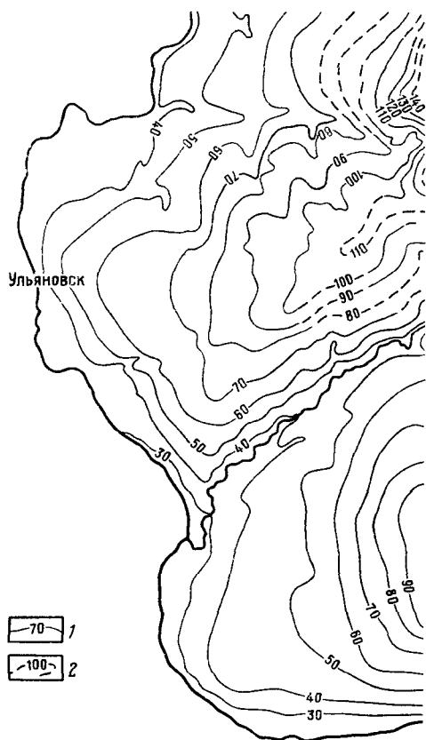
Рис. 31. Схема гидроизогипс левобережья р. Волги на переподмежи до создания Куйбышевского водохранилища (по М. А. Везировой).
