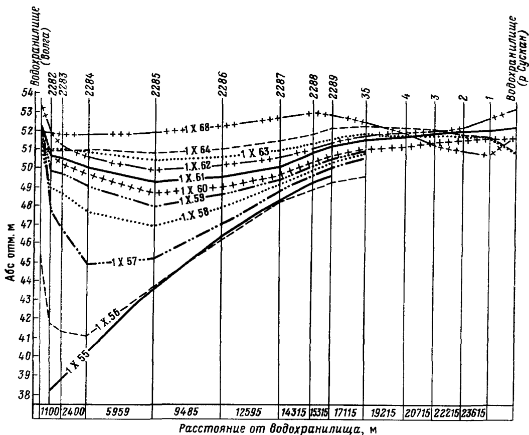
Рис. 34. Формирование подпора грунтовых вод на Волго-Сусанском водсразделе (разрез по линии А—А, см. рис. 35).
