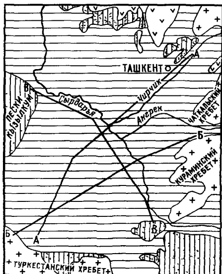
Рис. 59. Схема Приташкентско-Голодно-степской впадины.
