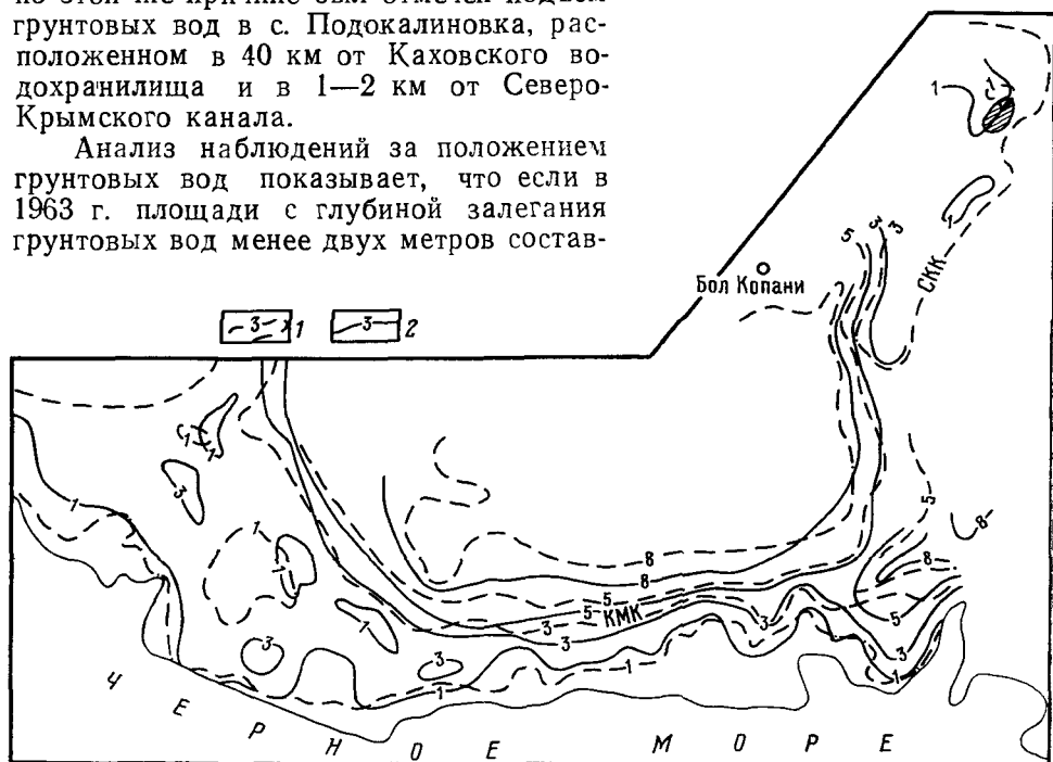
Рис. 50. Схема глубин залегания грунтовых вод Краснознаменского орошаемого массива.
