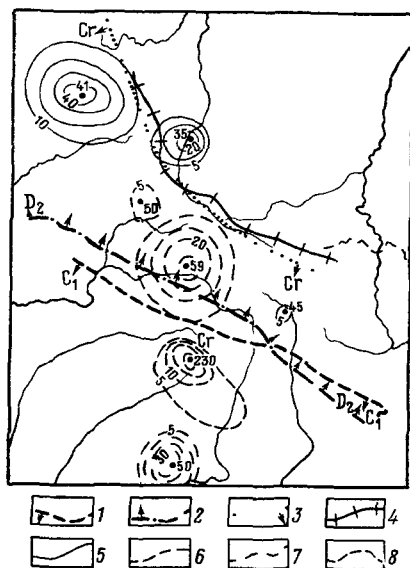
Рис. 19. Существовавшие воронки депрессии на территории Курской магнитной аномалии.
