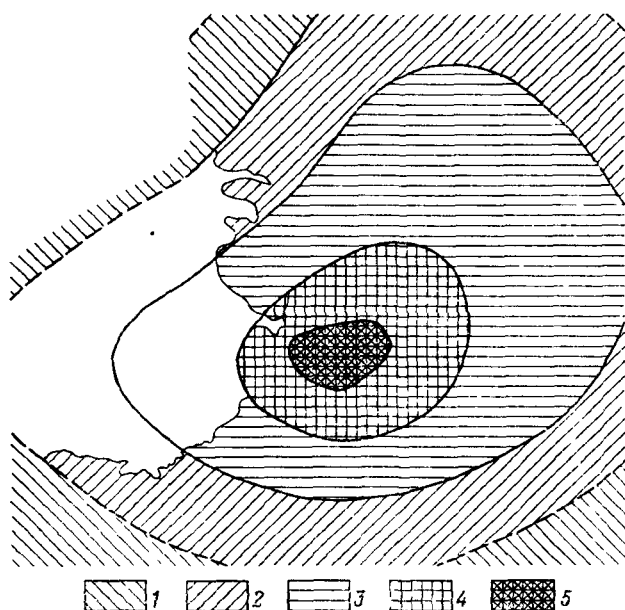
Рис. 4. Схема понижения уровня подземных вод гдовского горизонта за период с 1944 по 1963 г. (по М. П. Гасс). 1 — от 40 до 45; 2 — от 45 до 50; 3 — от 50 до 55; 4 — от 55 до 60; 5 — более 60 м
