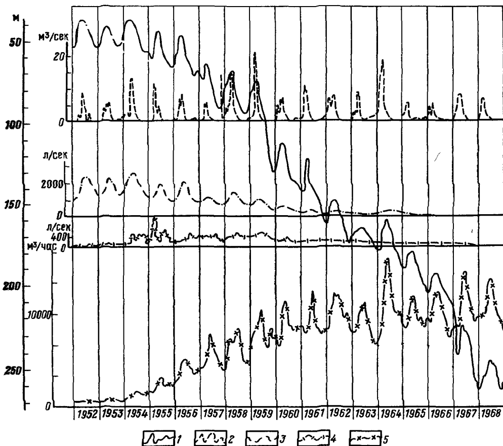
Рис. 17. Сводный график режима подземных и поверхностных вод района Миргалымсайского месторождения (по П. А. Серому и В. П. Горбаню).
