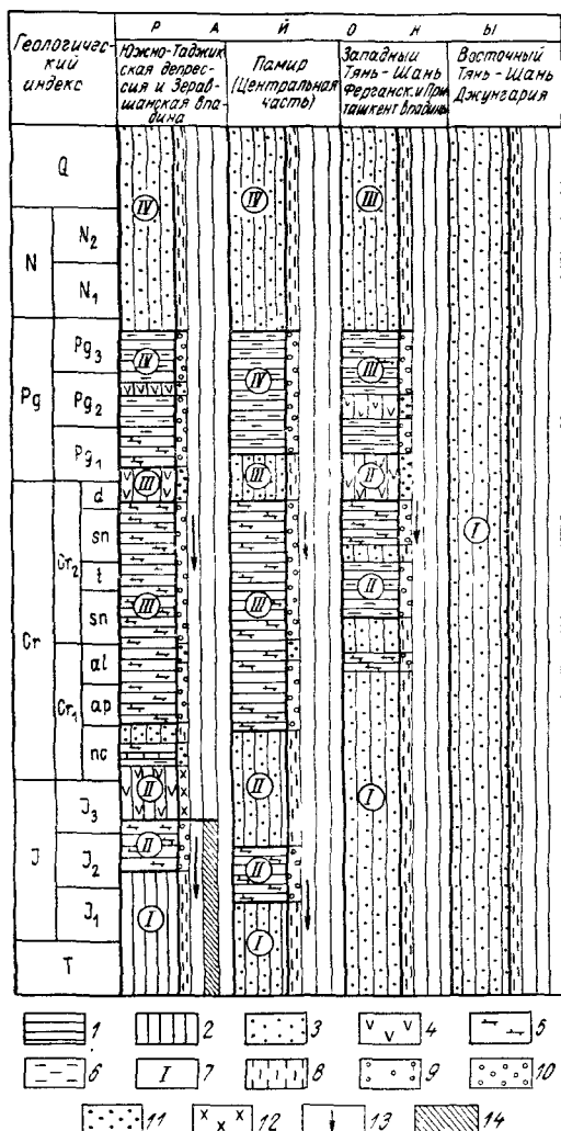
Рис. 73. График гидрогеологической цикличности в мезозое и кайнозое. По Б. Е. Аитыпко.
