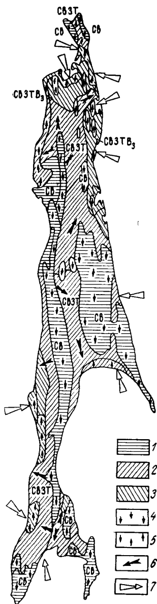
Рис. 60. Схема гидродинамической зональности (О. В. Равдоникас, 1967).
