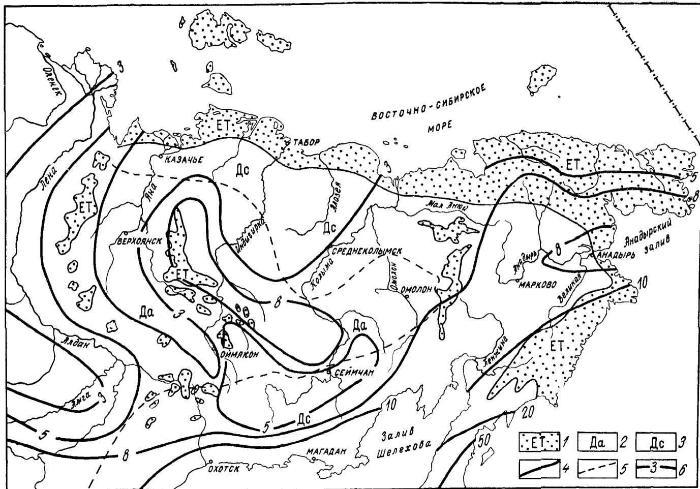
Рис. 51. Схематическая карта климатического районирования и подземного стока Северо-Востока СССР (по материалам Н. К. Ключкина, 1960 и В. И. Куделина, 1966).
