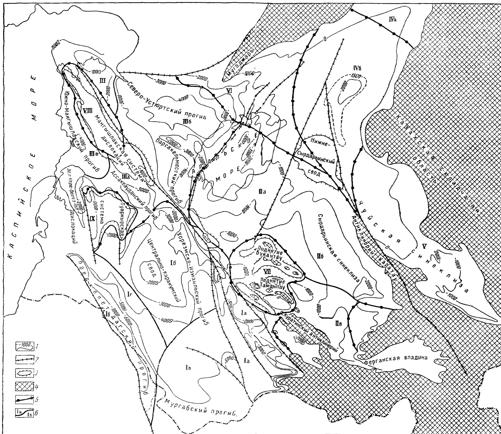
Рис. 23. Схема гидрогеологического районирования Туранской плиты с элементами тектоники. По материалам Л. А. Островского, А. П. Янишина, А. Б. Бабаева, Г. Х. Дикенштейна.
