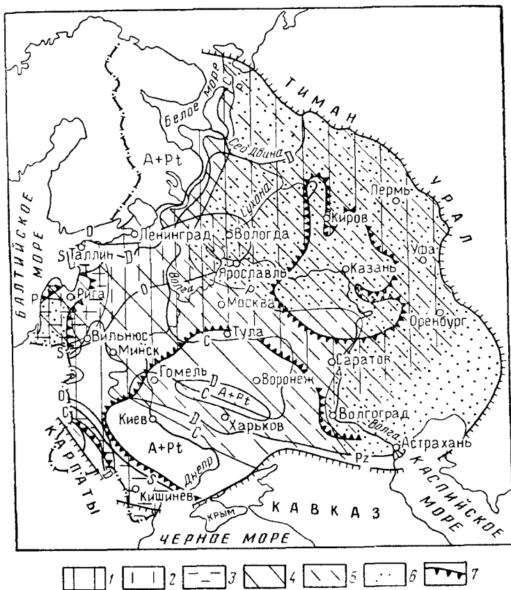
Рис. 11. Схема распространения докембрийских отложений. По Б. Н. Архангельскому, 1967.
