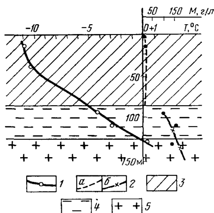
Рис. 36. Изменение температуры и минерализации подземных вод с глубиной в нижнемеловых отложениях архипелага Земли Франца-Иосифа
