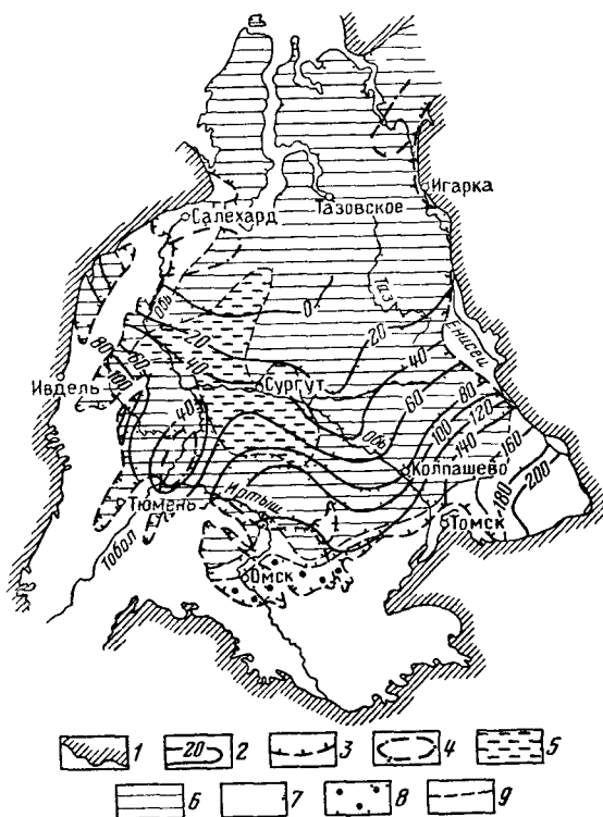
Рис. 20. Схема пьезометрической поверхности и песчаности отложений пятого гидрогеологического комплекса. По А. Д. Резникову и И. И. Нестерову, 1967. 1 — современная граница артезианского бассейна; 2 — пьезозогины; 3 — граница распространения комплекса; 4 — участки гидродинамических аномалий. Содержание песчаных (проницаемых) пород, % от общей мощности толщи: 5 — 20—40; 6 — 40—60; 7 — 60—80; 8 — 80—100; 9 — граница распространения песчаных (проницаемых) пород различной мощности.
