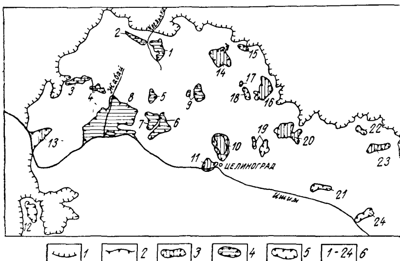
Рис. 78. Схема размещения девон-карбоновых мульд разного типа:
