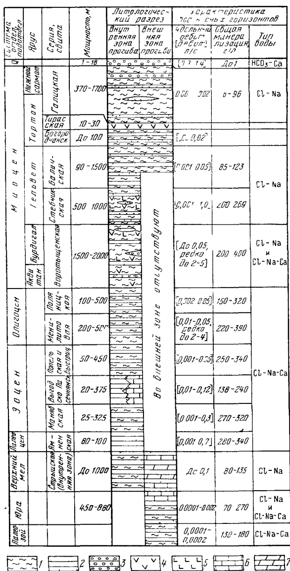
Рис. 38. Гидрогеологическая колонка Предкарпатского артезианского бассейна. Составил И. Г. Киссин по материалам О. С. Вялова, Г. Н. Доленко, А. Ф. Романюка и др.
