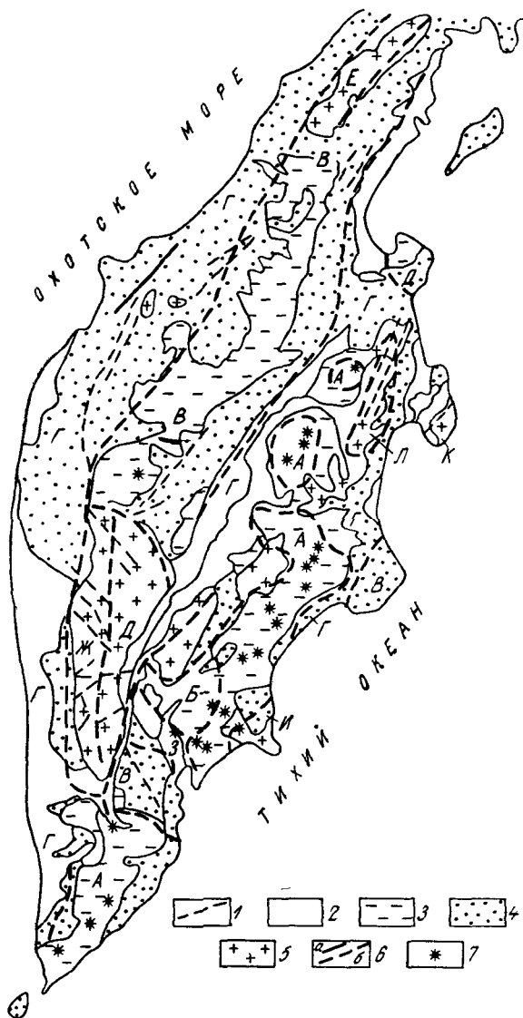
Рис. 50. Схема распространения минеральных вод Камчатки. По В. В. Иванову, В. Н. Дислеру, 1967.
