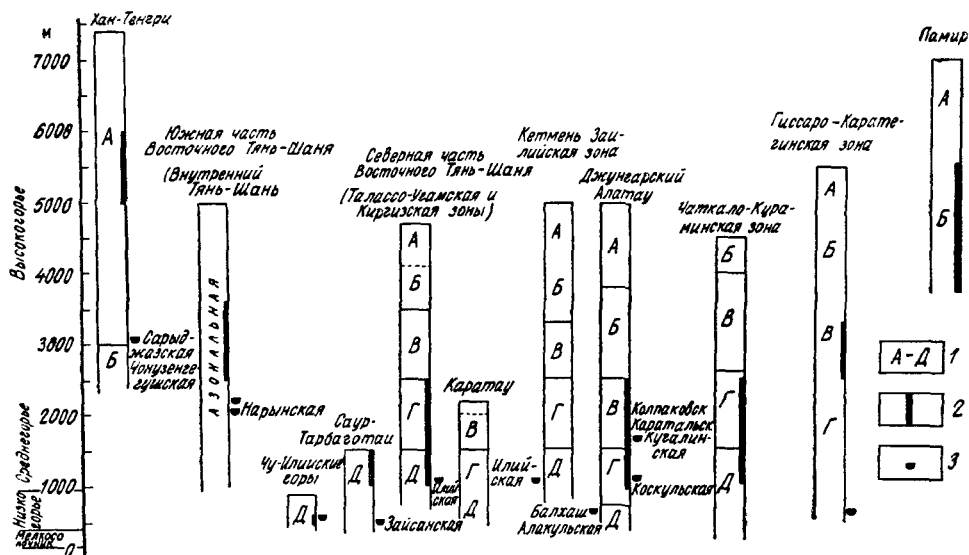
Рис. 69. Схема поясной зональности Тянь-Шаньско-Джунгаро-Памирской складчатой области. По Б. Е. Антыпко.
