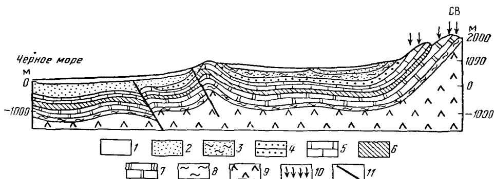
Рис. 47. Схематический гидрогеологический разрез Колхидской низменности. Составил И. М. Буачидзе.
