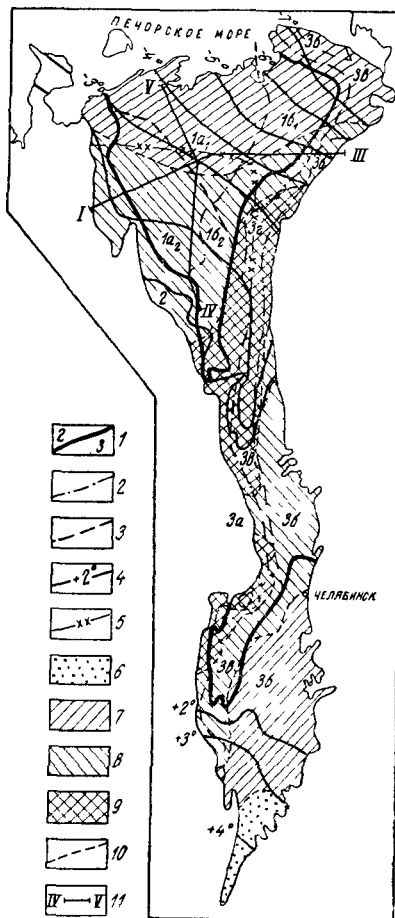
Рис. 62. Схема гидрогеологического районирования (с элементами климата) Уральской складчатой области (VII)
