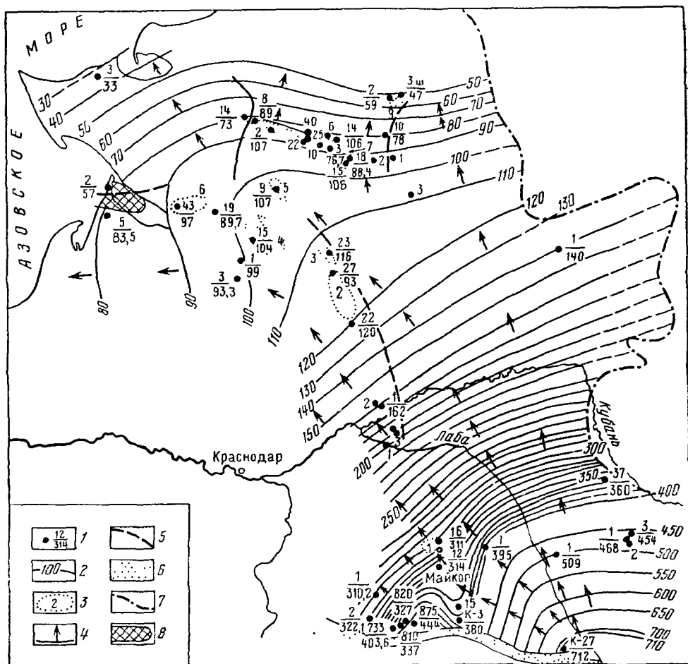
Рис. 40. Схема приведенных напоров нижнемелового водоносного комплекса Западного Предкавказья. По Д. И. Рогожину, 1964.
