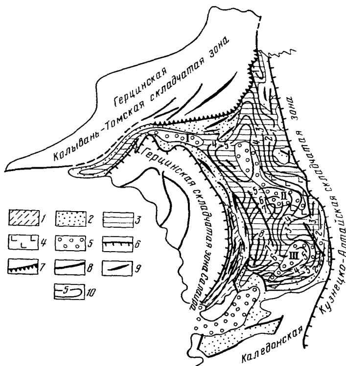
Рис. 83. Тектоническая схема Кузнецкого прогиба (по Н. С. Зайцеву, 1963 г., с упрощениями)
