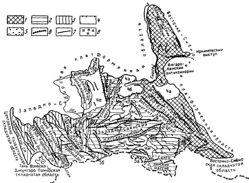
Рис. 82. Тектоническая схема Саяно-Алтайско-Енисейской гидрогеологической области (по Тектонической карте Евразии м-ба 1:5 000 000, 1966, и данным Э. Н. Янова и др.)
