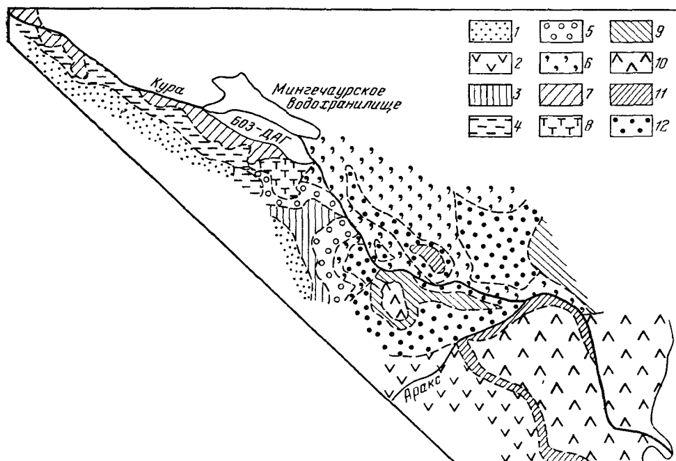
Рис. 45. Схематическая карта химического состава и минерализации грунтовых вод Куринской депрессии («Гидрогеология СССР», т. 12, М., «Недра», 1969).
