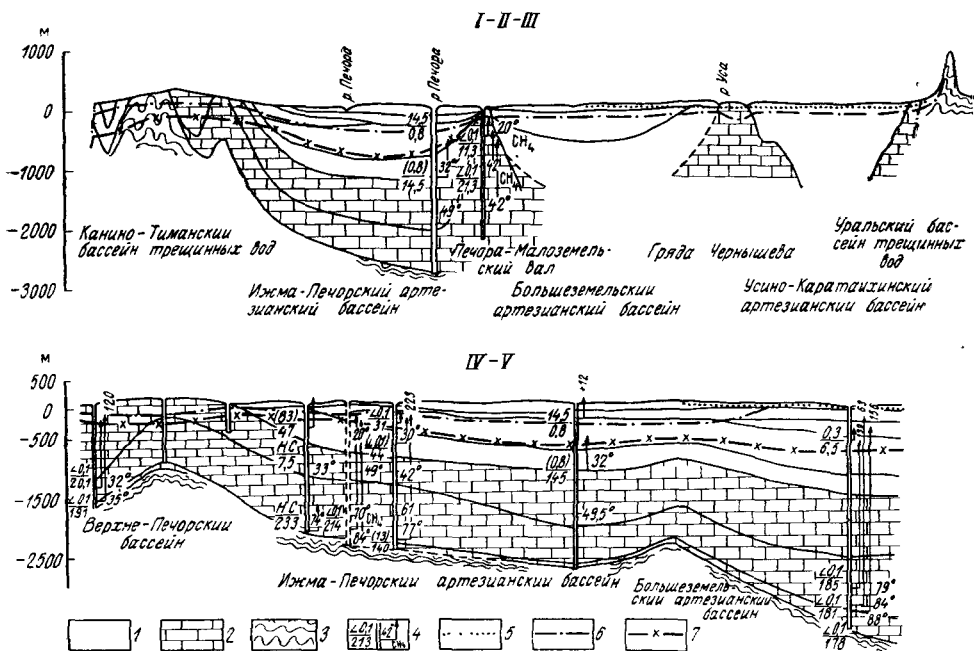
Рис. 63. Схематические разрезы Печорской системы артезианских бассейнов.
