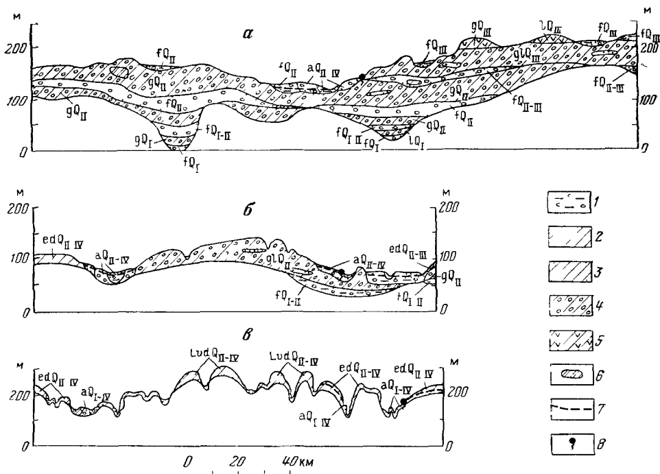
Рис. 4. Типовые разрезы четвертичных отложений:
