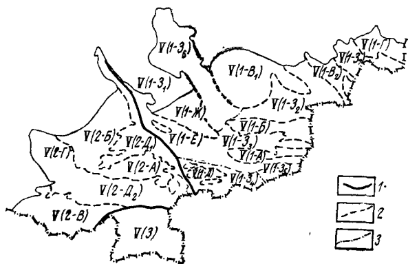
Рис. 71. Схема гидрогеологического районирования Тянь-Шаньско-Джунгаро-Памирской складчатой области. По Б. Е. Антыпко, Е. И. Лагутину, В. С. Самаринной. Границы и индексы гидрогеологических районов: 1 — первого порядка; 2 — второго порядка; 3 — третьего порядка (цифры на схеме): V(1) — Восточный Тянь-Шань и Джунгарский Алатау. Межгорные артезианские бассейны: V(1-А) — Иссыккульский; V(1-Б) — Илийский; V(1-В) — сложный Балхаш-Алакульский (в нем выделены: V(1-В₁) — Прибалхашский, V(1-В₂) — Алакульский); V(1-Г) — Зайсанский; V(1-Д) — Нарынский; V(1-Е) — Таласский; V(1-Ж) — Чуйский; V(1-З) — складчато-глыбовые зоны Восточного Тянь-Шаня и Джунгарского Алатау (в том числе: V(1-З₁) — Каратауская; V(1-З₂) — Джунгаро-Алатауская; V(1-З₃) — северная часть Восточного Тянь-Шаня; V(1-З₄) — южная часть Восточного Тянь-Шаня; V(1-З₅) — Хан-Тенгри; V(1-З₆) — Чу-Илийская; V(1-З₇) — Саур-Тарбагатайская); V(2) — Западный Тянь-Шань. Межгорные и предгорные артезианские бассейны: V(2-А) — сложный Ферганский; V(2-Б) — Приташкентский; V(2-В) — сложный Южно-Таджикский; V(2-Г) — Зеравшанский; V(2-Д) — сложная глыбовая зона Западного Тянь-Шаня (в том числе: V(2-Д₁) — Чаткало-Курамнянский; V(2-Д₂) — Гиссаро-Алайский); V(3) — Памир, складчато-глыбовая зона
