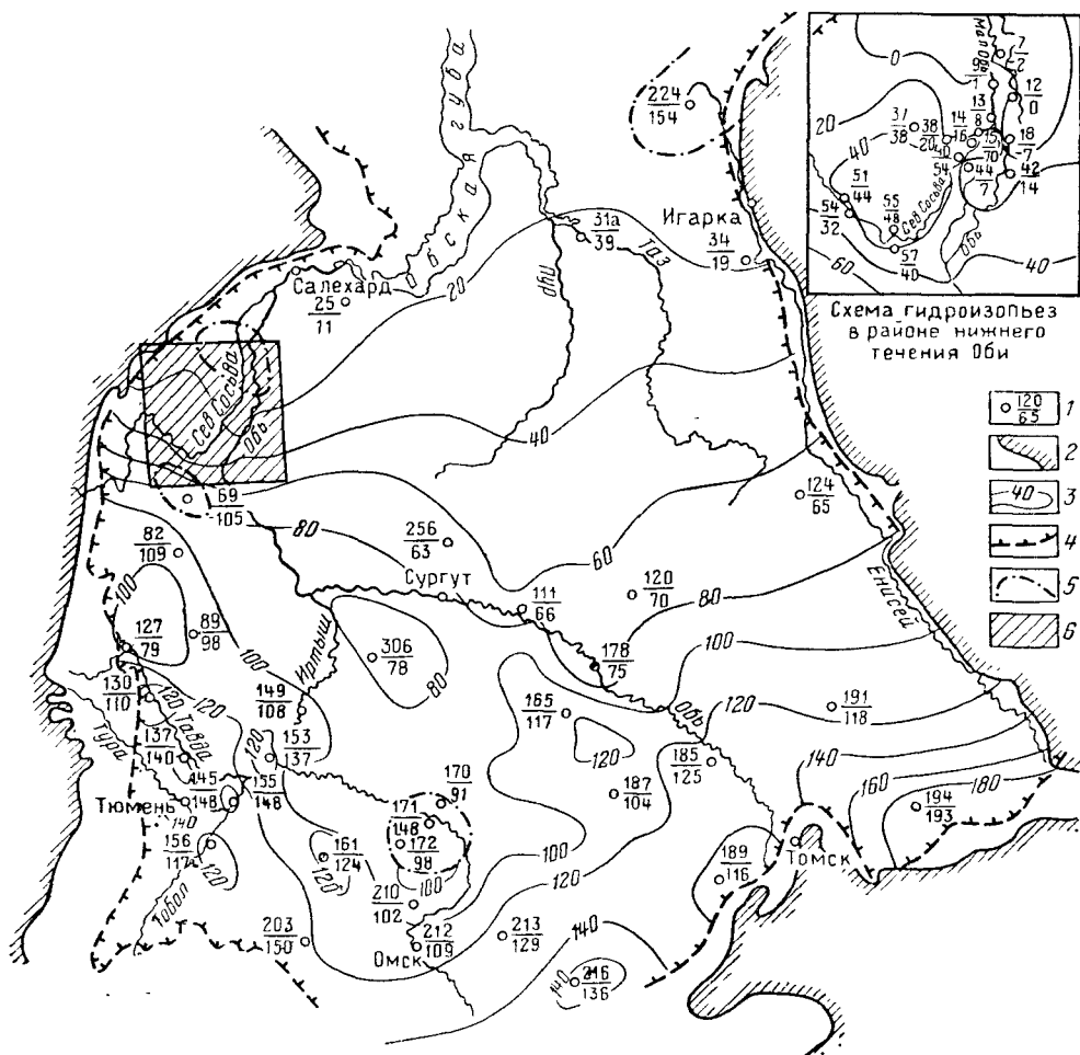
Рис. 19. Схема пьезометрической поверхности четвертого гидрогеологического комплекса. По А. Д. Резникову, 1967.
