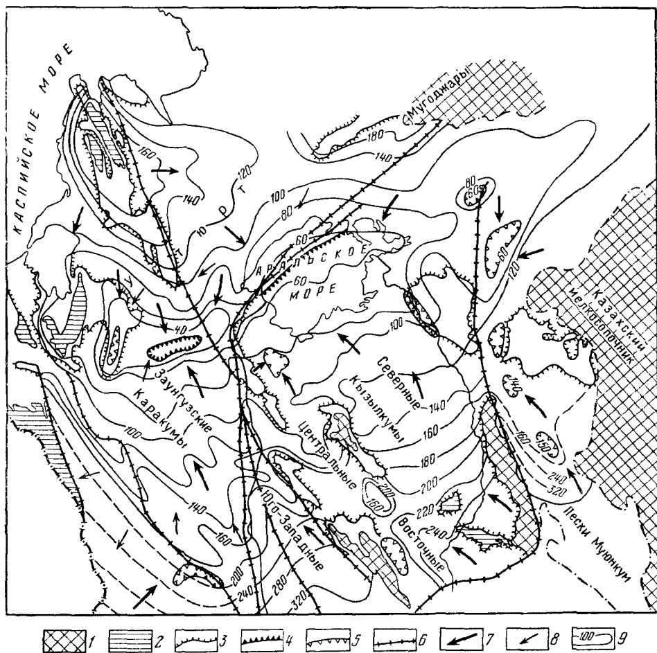
Рис. 25. Гидродинамическая схема верхней части среднего гидрогеологического этажа (зоценового, палеозенового — зоценового и верхнемелового — зоценового и верхнемелового водоносных комплексов). По Л. А. Островскому и В. М. Фомину.
