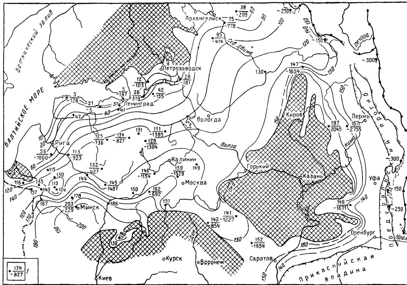
Рис. 8. Схема пьезометрической поверхности вод верхнепермско-нижепермского водопосного комплекса. По Г. П. Якобсон. 1 — буровая скважина; цифры обозначают: в числителе — величина приведенного статического уровня, м абс. отм., в знаменателе — глубина опробования, м. Другие условные обозначения см. на рис. 7
