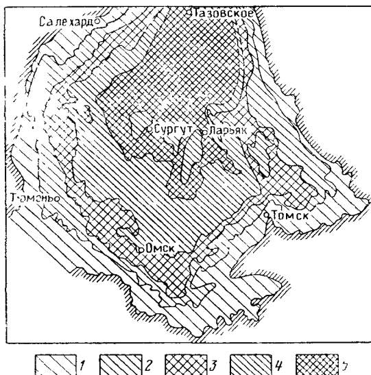
Рис. 21. Схема дифференциации температур по поверхности фундамента. По Ю. К. Махневу и А. А. Розину.
