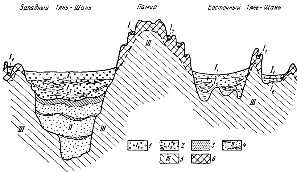
Рис. 68. Схема гидрогеологической этажности. По Б. Е. Антыпко и Е. И. Лагутину.
