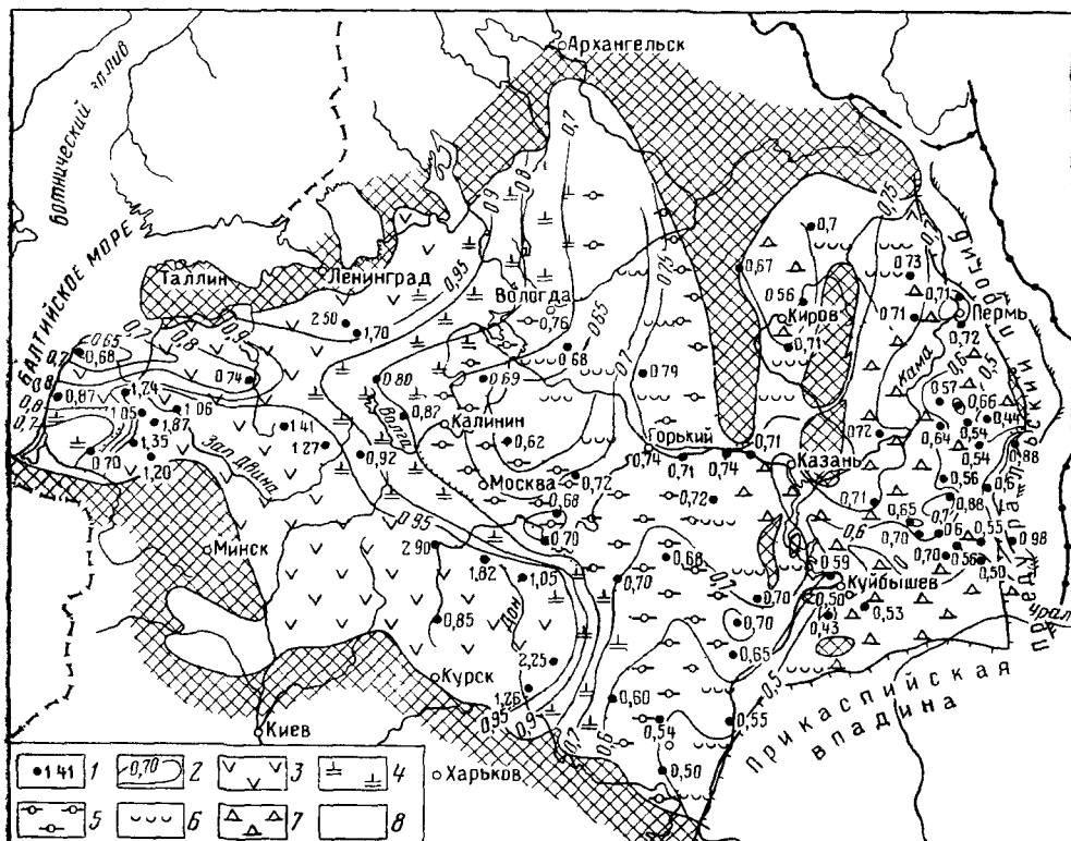
Рис. 5. Схема метаморфизации по Na/Cl и минерализации вод средне-верхнедевонского водоносного комплекса. По Г. П. Яковсон.
