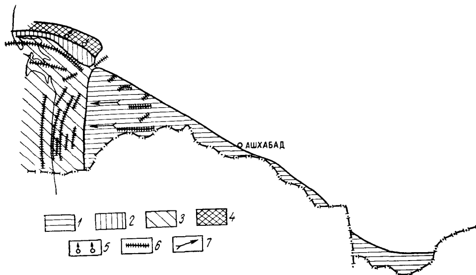
Рис. 48 Схема гидрогеологического районирования Копетдагско-Большебалханской складчатой области:
