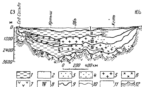
Рис. 15. Схематический гидрохимический разрез Западно-Сибирского артезианского бассейна. По А. Д. Лобачеву, Ю. В. Махневу, А. А. Розину, Б. П. Ставицкому, Ю. К. Смоленцеву.
