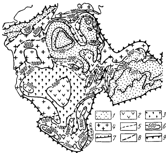
Рис. 32. Схема гидрогеотермической зональности.
