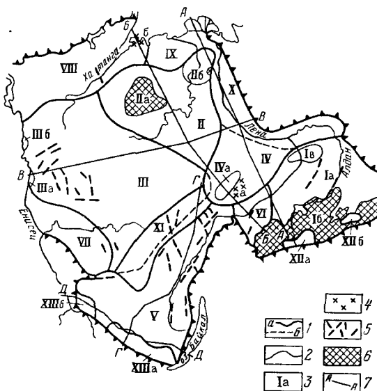
Рис. 27. Схема расположения основных тектонических структур Сибирской платформы (по Т. И. Спизарскому, 1961, И. И. Краснову и др., 1966) и местоположение гидрогеологических профилей.
