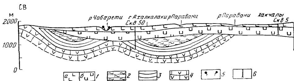
Рис. 44. Схематический гидрогеологический разрез Ахалкалакского лавового нагорья. Составил Т. П. Лазарашвили.
