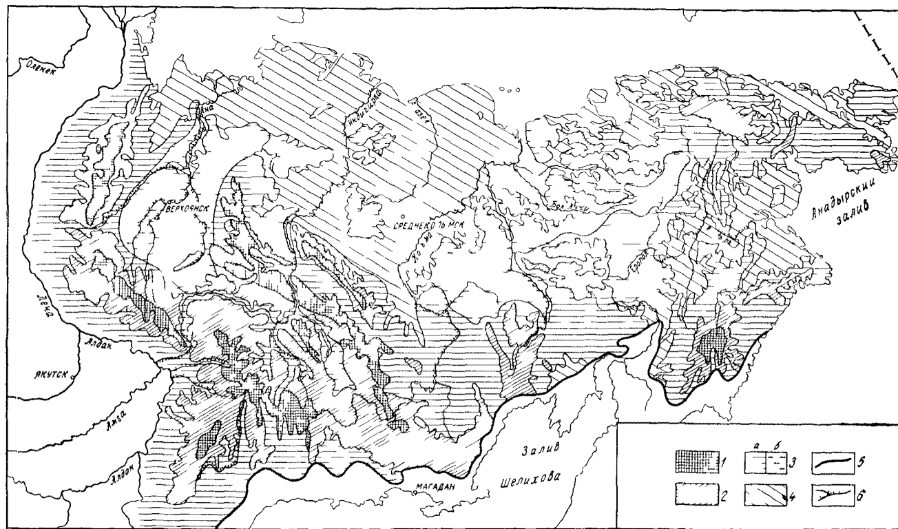
Рис. 55. Схема вертикальной поясности порово-пластовых вод в рыхлых четвертичных отложениях в области сплошного распространения мерзлой зоны Составила Н И Индолева по материалам А А Зеленкевича
