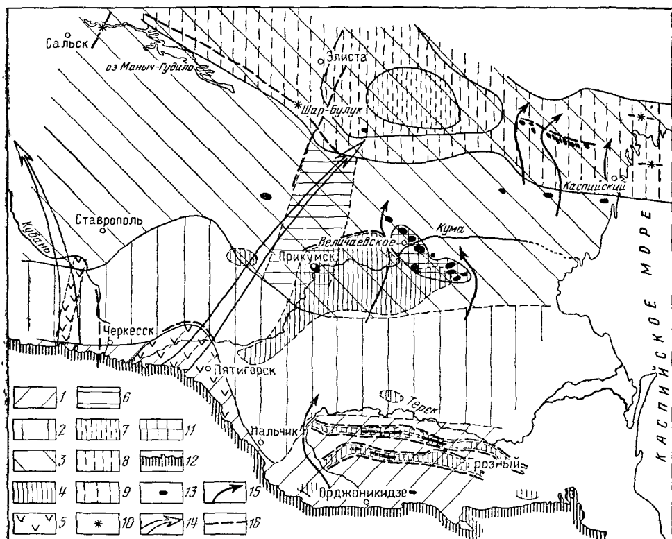
Рис. 42. Гидродинамическая схема мезозойских водоносных комплексов Восточно-Предкавказского бассейна. По И. Г. Киссину, 1964.
