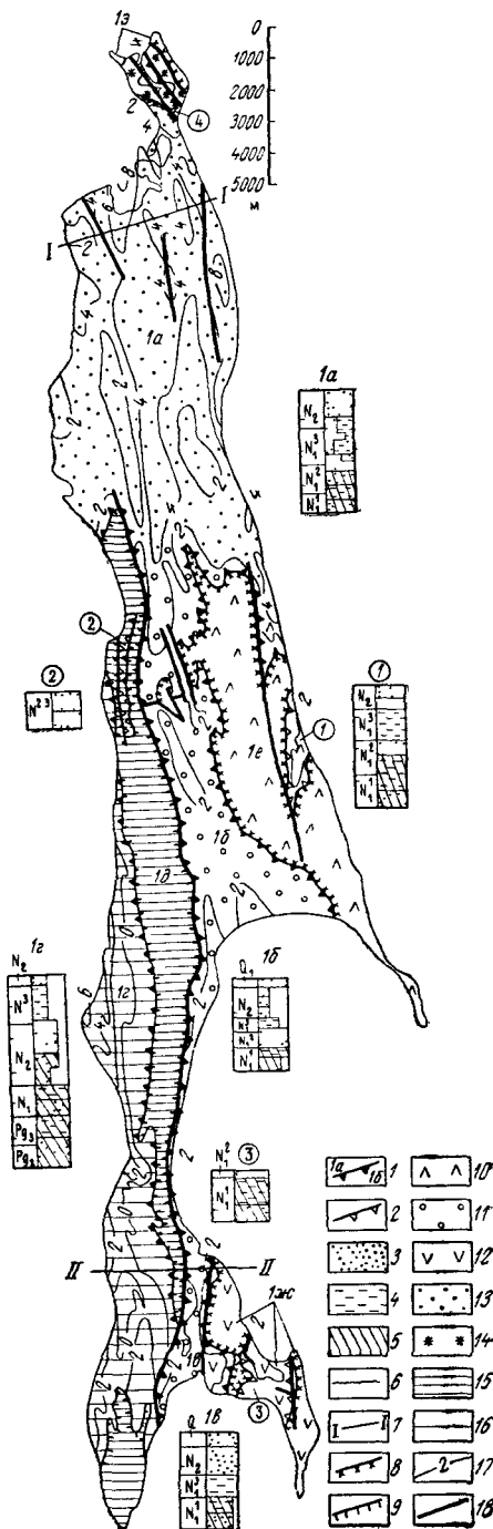
Рис. 57. Схема гидрогеологического районирования Сахалина (по О. В. Равдоникас) с элементами тектонического строения (по Ю. М. Пушаровскому)
