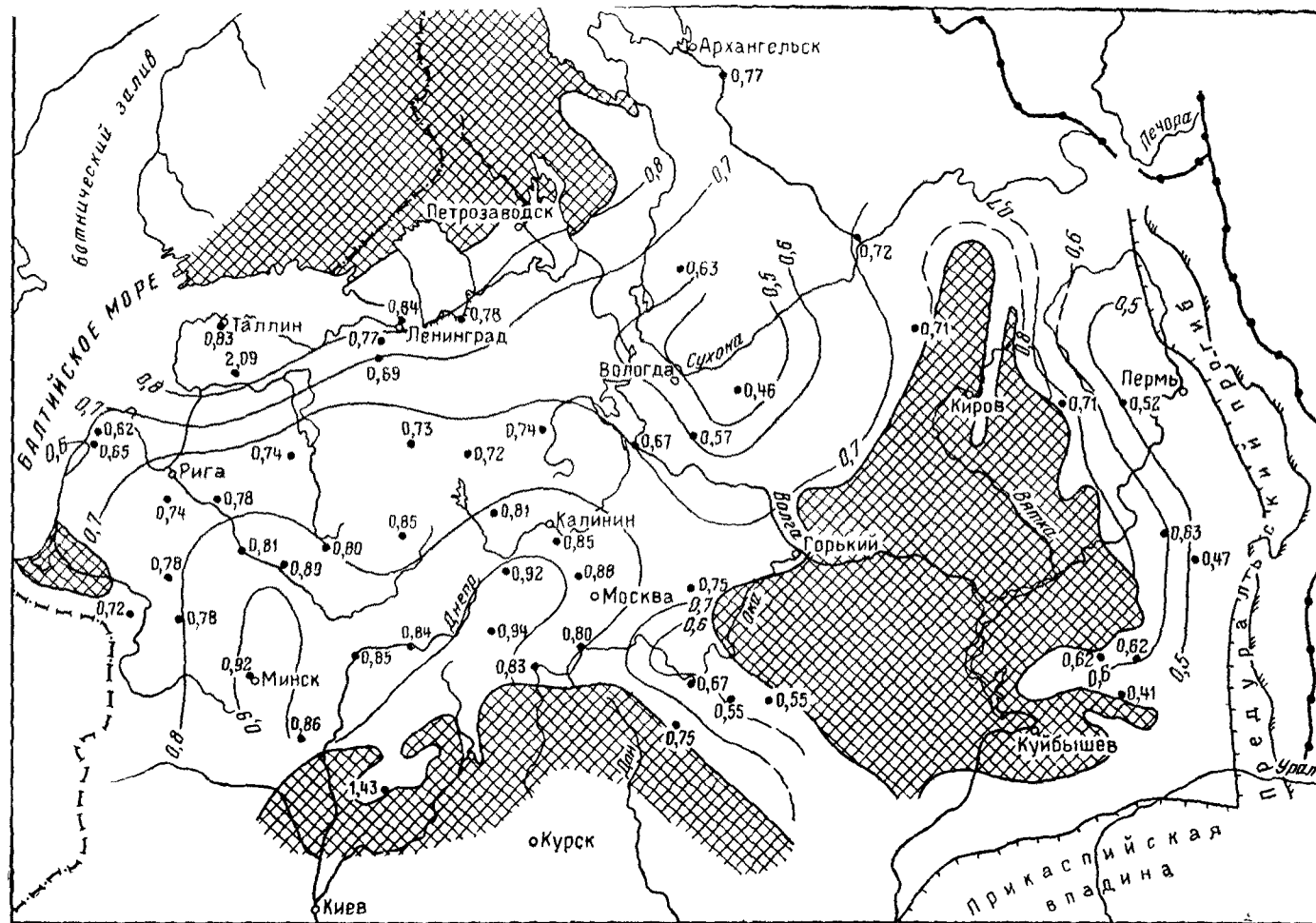
Рис. 6. Схема метаморфизации вод по Na/Cl верхнерифейско-вендско-нижнекембрийского водоносного комплекса. По Г. П. Якобсон. Условные обозначения см на рис. 5
