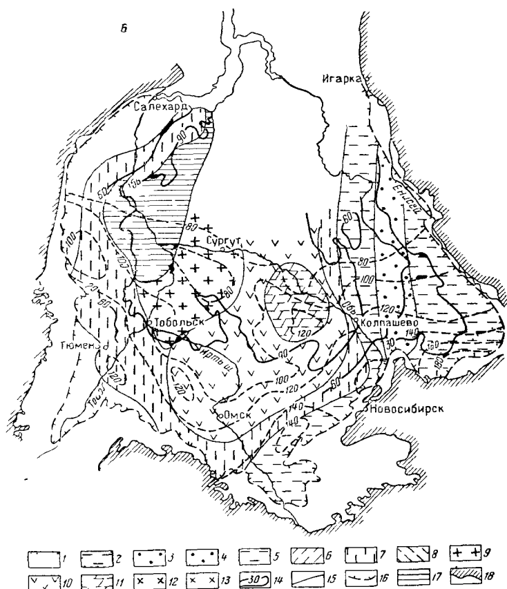
Рис. 17. Гидрохимические схемы водоносных комплексов. По Г. М. Богомякову, Ю. В. Махневу, В. В. Нелюбину, В. А. Нуднер, А. А. Розину, Б. П. Ставицкому, 1966.
