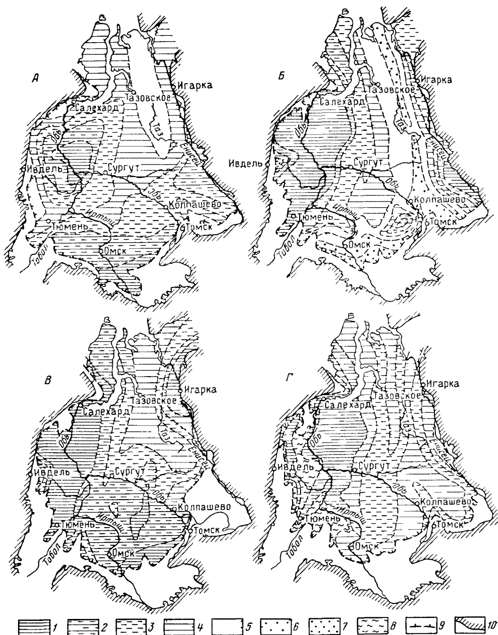
Рис 18. Схема песчанистости отложений четвертого гидрогеологического комплекса. Возраст толщ А — готерив — баррем, Б — верхний валанжин, В — средний и нижний валанжин, Г — верхняя юра. Содержание песчаных (проницаемых) пород в % от общей мощности толщи (по И. И. Несторову) 1 — 0, 2 — 0—20, 3 — 20—40, 4 — 20—60, 5 — 60—80, 6 — 80—100, 7 — 100, 8 — область локального распространения песчаных пород верхнеюрской трансгрессии, относимых к пятому гидрогеологическому комплексу, 9 — граница распространения комплекса, 10 — граница артезианского бассейна
