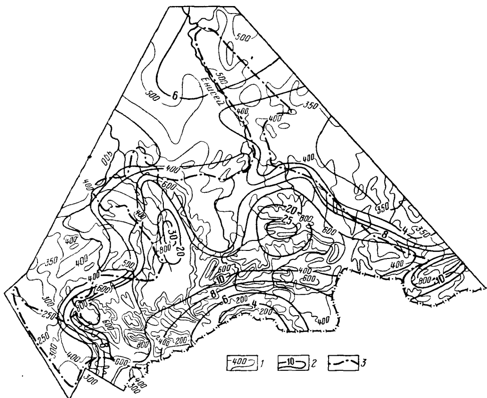
Рис. 81. Схематическая карта распределения годовых осадков (по материалам «Климатического атласа СССР», 1960) и среднегодового стока рек (К. П. Воскресенский, 1962 г.).
