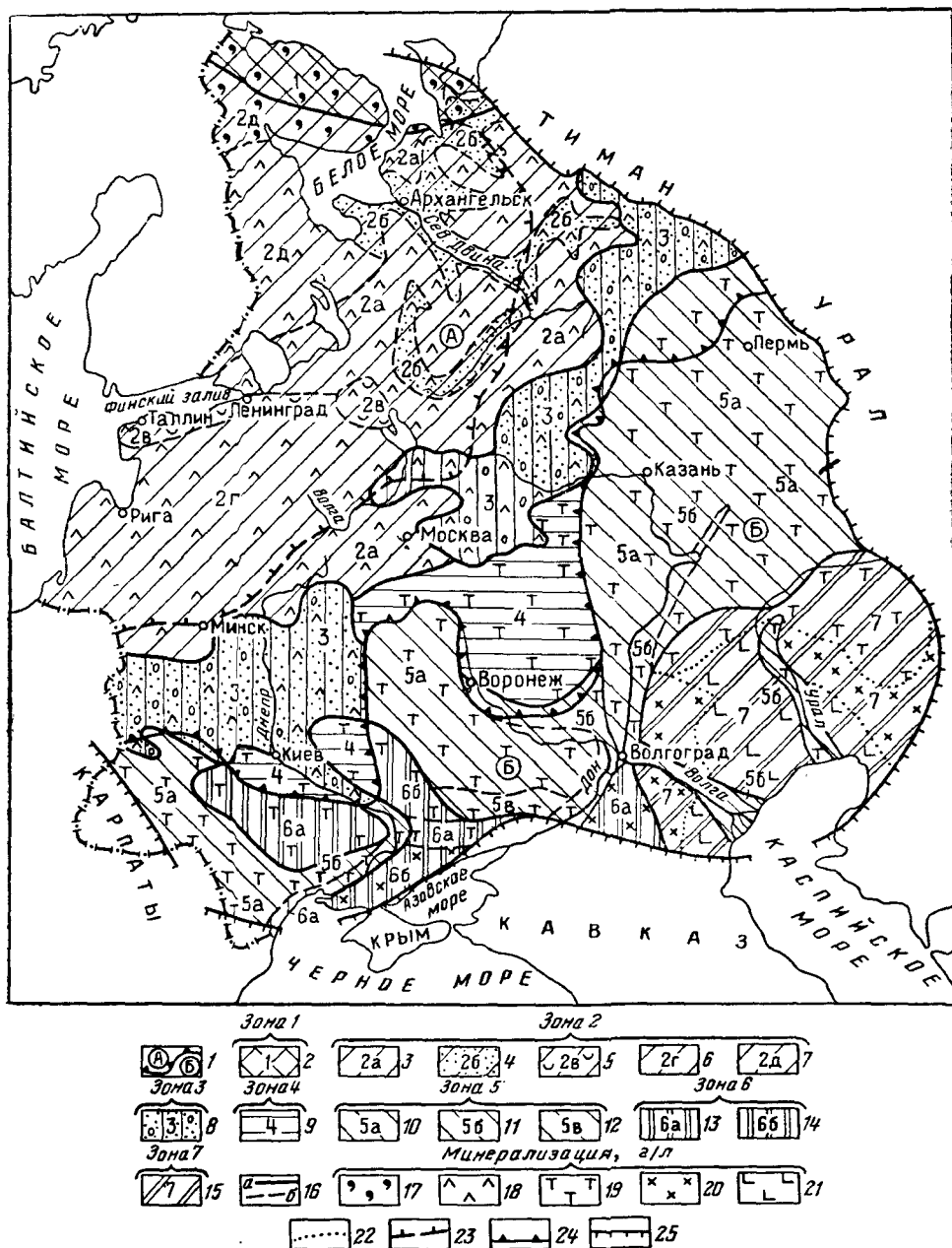
Рис. 9. Схема распространения грунтовых вод. По Я. А. Сыровашной.
