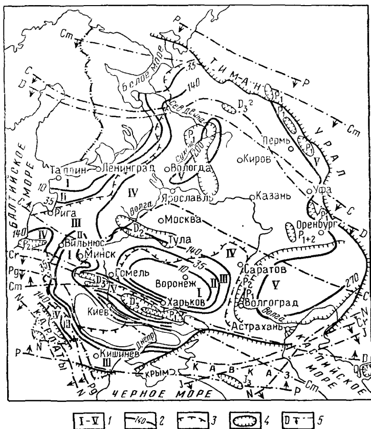
Рис. 10. Гидрохимическая карта. Составил Б. Н. Архангельский, 1967.
