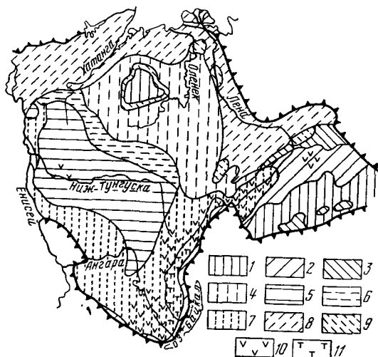
Рис. 31. Схема зональности газового состава подземных вод. Районы распространения подземных вод с растворенными газами:
