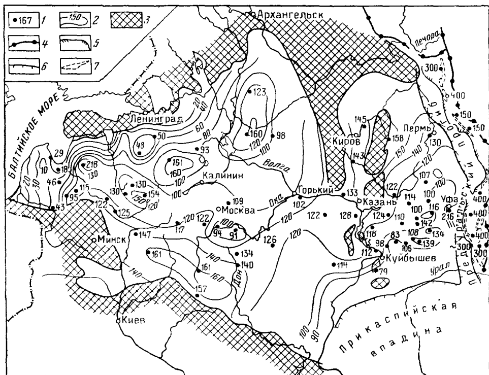
Рис. 7. Схема пьезометрической поверхности вод средне-верхнедевонского водоносного комплекса По Г. П. Яковсону
