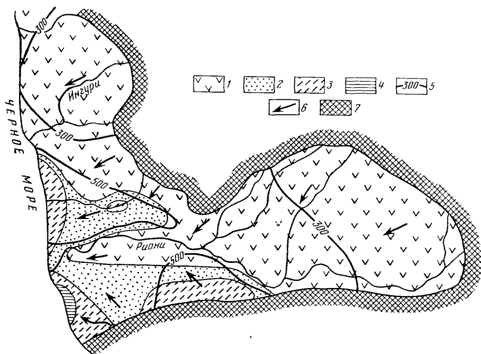
Рис. 46. Схематическая карта химического состава подземных вод четвертичных отложений Колхидской низменности. Составил Л. А. Харатишвили.
