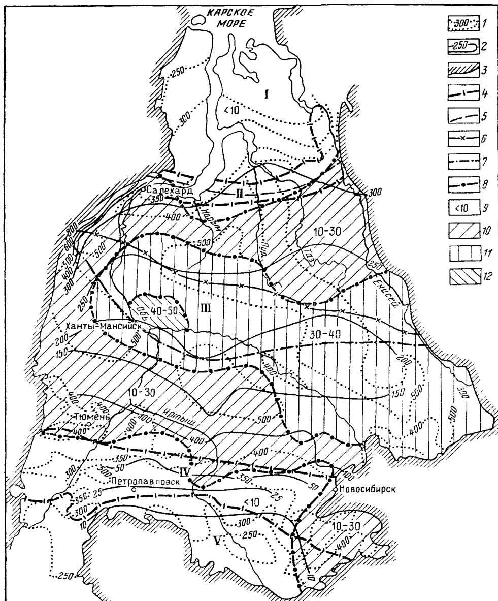
Рис. 14. Схема природных зон и элементы водного баланса.
