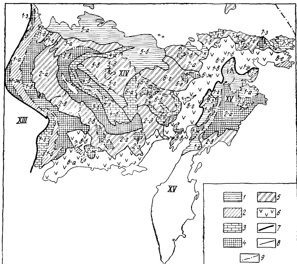
Рис. 54. Схема гидрогеологического районирования Верхояно-Чукотской мезозойской (XIV) и Корякской кайнозойской складчатых областей (XV):
