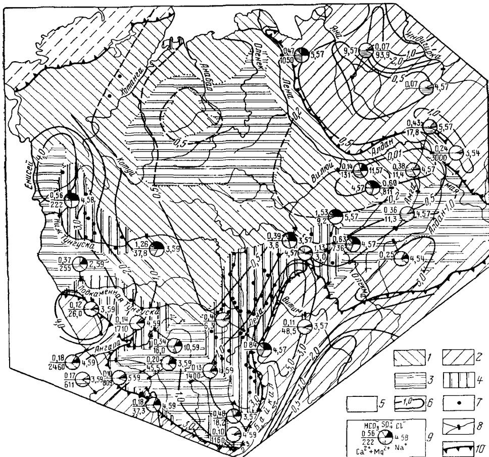
Рис. 33. Схема гидрохимической зональности подземного стока (в зимний период).
