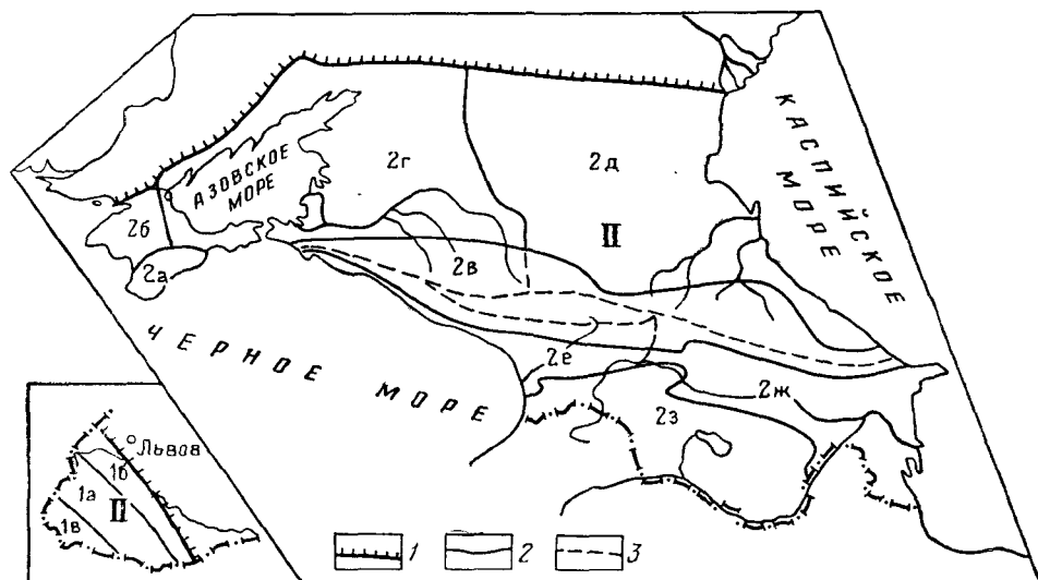
Рис. 37. Схема гидрогеологического районирования Карпатской и Крымско-Кавказской областей. 1 — граница гидрогеологических структур первого порядка; 2 — граница гидрогеологических структур второго порядка; 3 — границы внешних областей питания артезианских бассейнов. 1а — Горные Карпаты, 1б — Предкарпатский артезианский бассейн, 1в — Закарпатский артезианский бассейн; 2а — Горный Крым; 2б — Западно-Крымский артезианский бассейн; 2в — Большой Кавказ; 2г — Азово-Кубанский артезианский бассейн; 2д — Восточно-Предкавказский артезианский бассейн; 2е — Восточно-Черноморский артезианский бассейн; 2ж — Куринский артезианский бассейн; 2з — Малый Кавказ
