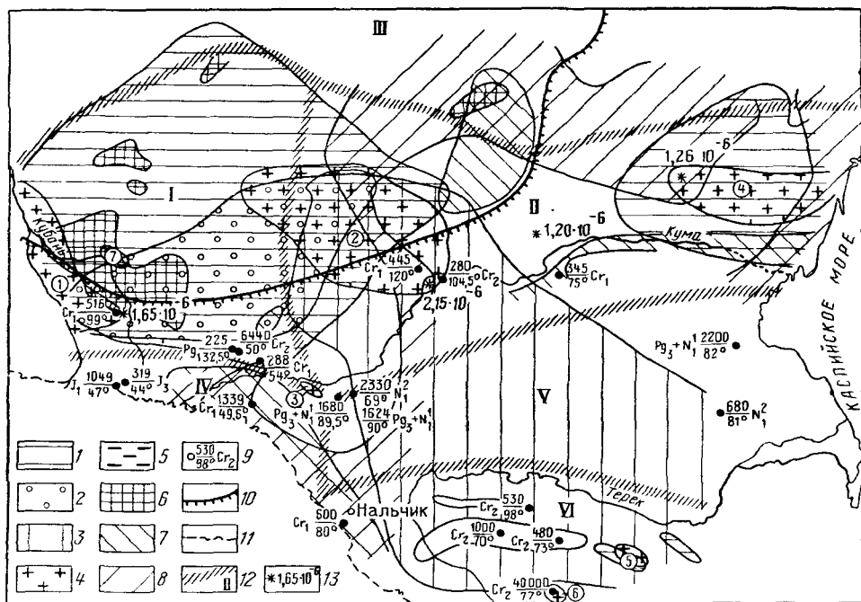
Рис. 43. Геотермическая карта Восточного и Центрального Предкавказья. Составили И. Г. Киссин и Е. А. Казинцев, 1962.
