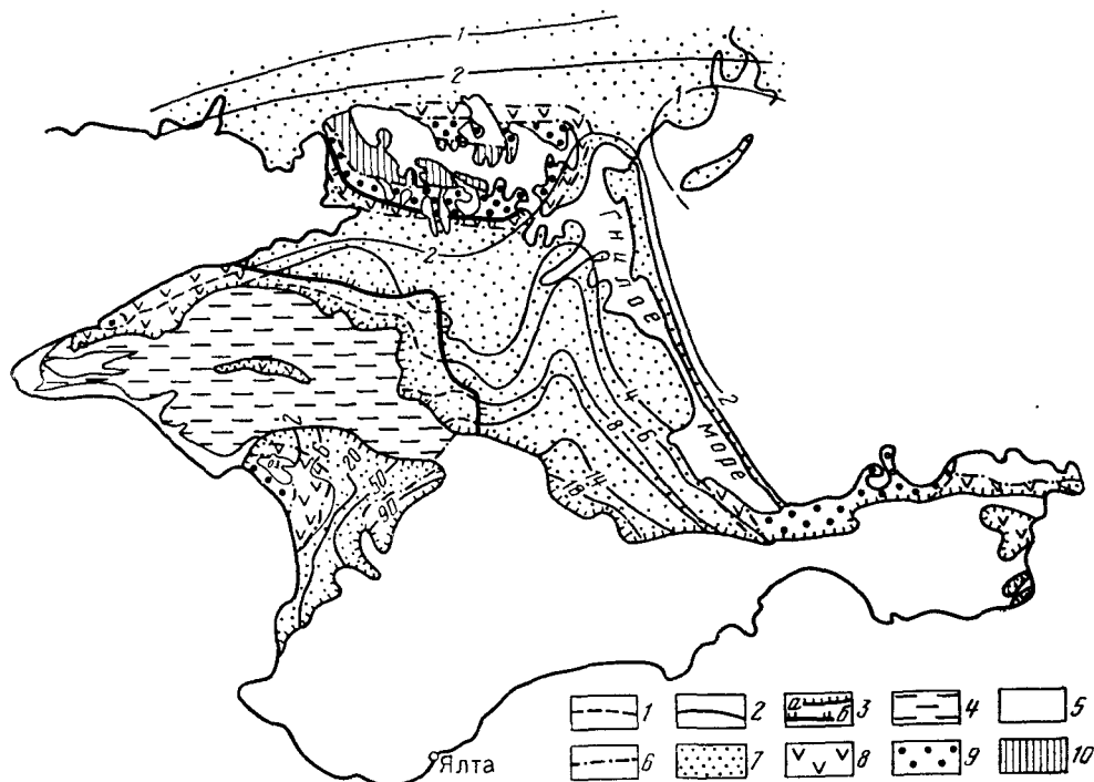
Рис. 39. Схема водноносности мзотических и понтических отложений Крыма По Е. А. Ришес и О. И. Сурдутович
