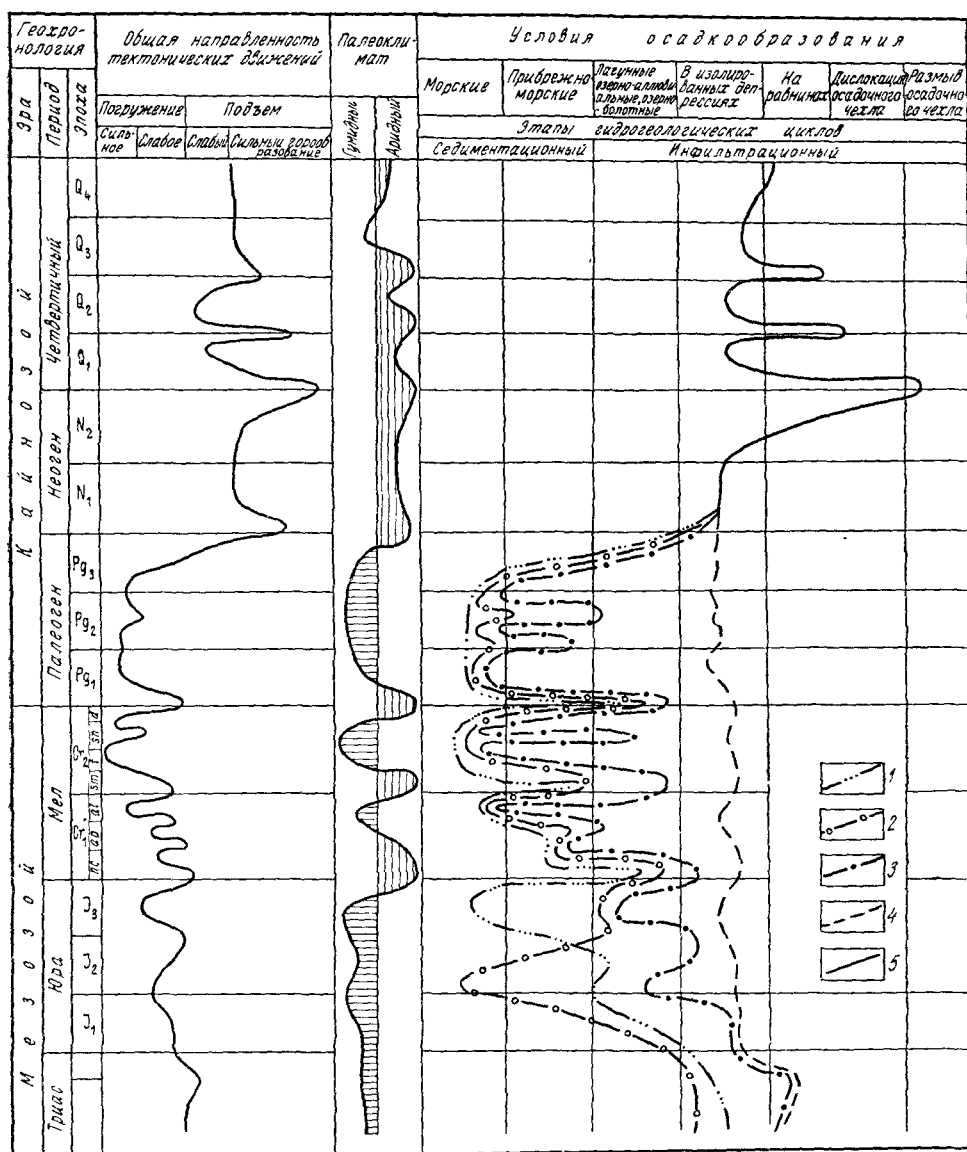
Рис. 72. График историко-геологического развития в мезозойскую и кайнозойскую эры. По Б. Е. Антыпко:
