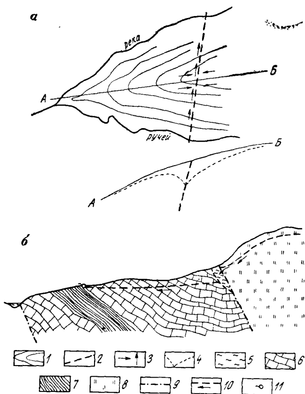
Рис. 64. Схема подземного стока:
