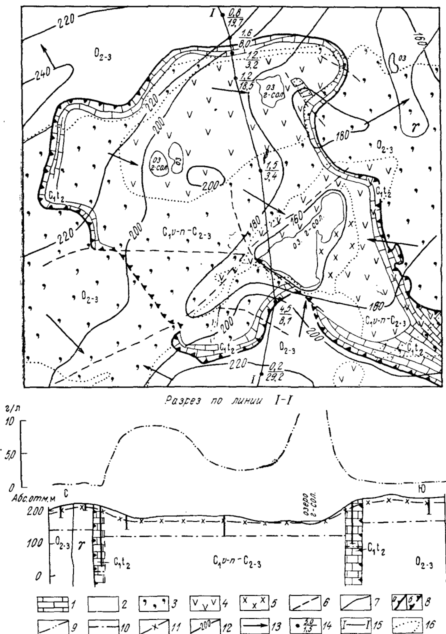
Рис. 79. Гидрогеологическая схема мульд первого типа:
