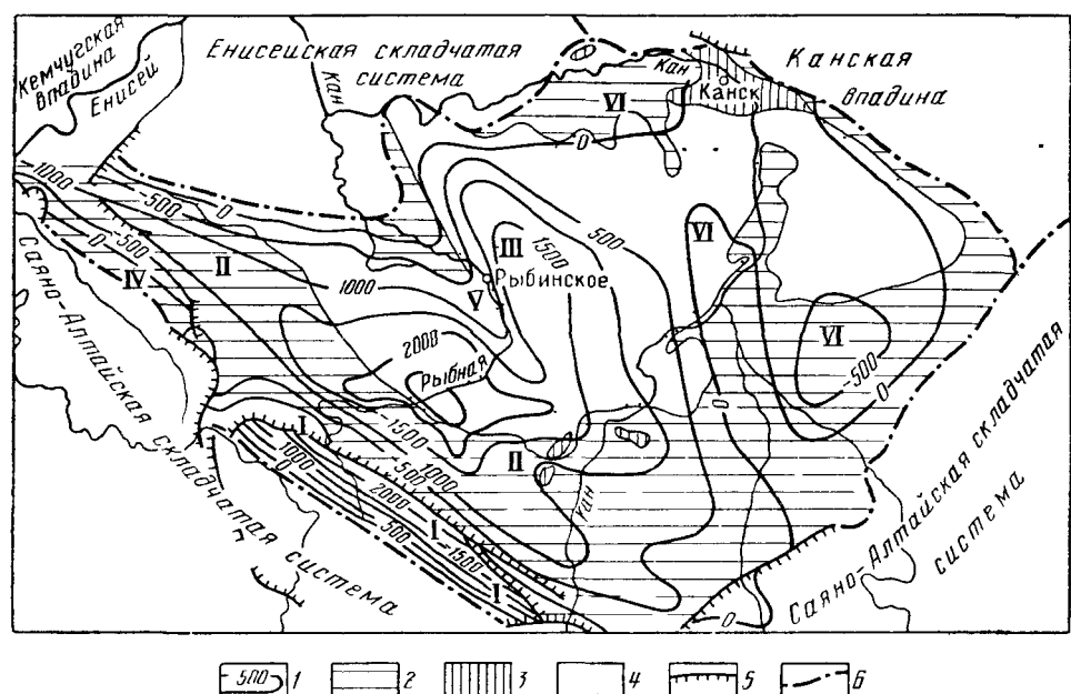
Рис 84 Тектоническая схема Рыбинской впадины (по Э. Н. Янову, 1957 г., с упрощениями). 1 — стратонизогипсы по кровле девонского фундамента (абс. отм. в м), 2—4 — отложения, заполняющие впадины (2 — девонские, 3 — каменноугольные, 4 — юрские), 5 — тектонические нарушения, 6 — граница Рыбинской впадины. Прогибы фундамента (I — Саяно-Партизанский, II — Балецкий, III — Бородинский). Поднятия фундамента (IV — Кияй Арбайское, V — Уярское, VI — Канское).
