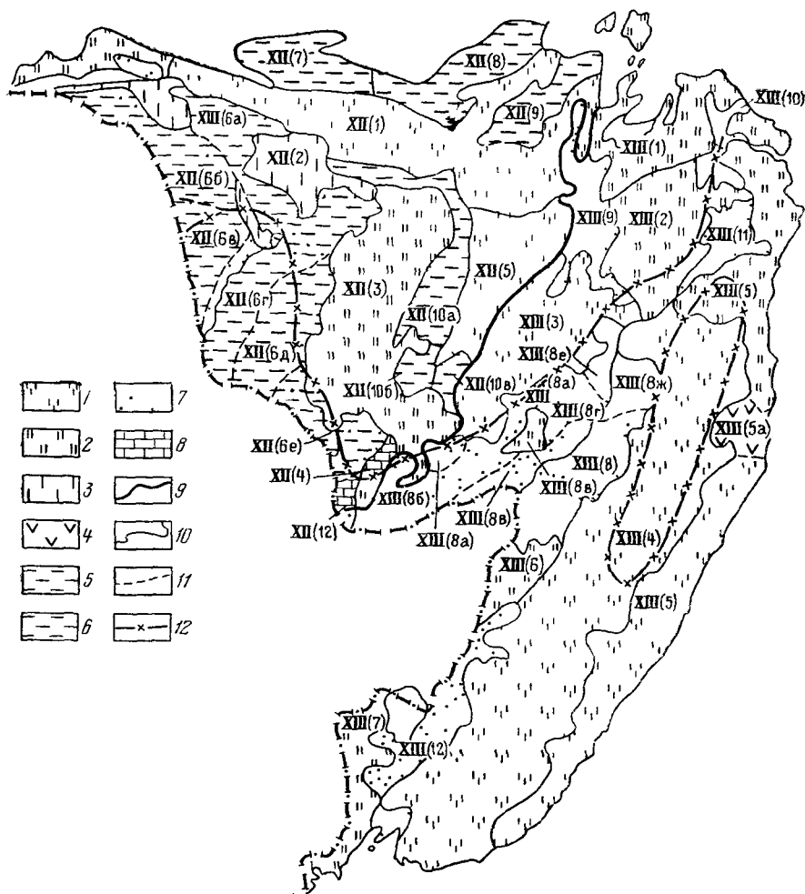
Рис 89. Схема гидрогеологического районирования
