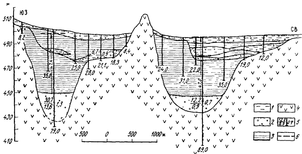
Рис. 77. Гидрогеологический разрез долины р. Джен на Жартасском участке. По В. А. Курдюкову. Водонасыщенные горизонты. 1 — аллювиальных нижнечетвертичных современных отложений (песка с галькой, гравием и прослоями глин); 2 — аллювиальных верхнеолигоценовых отложений (гравелистые глинистые пески с галькой и щебнем); 3 — водоупорные глинны; 4 — водоносный комплекс вулканогенных девонских отложений; 5 — скважина: слева в числителе — дебит (л/с), в знаменателе — понижение (м), справа — минерализация (г/л), внизу — глубина (м), 6 — пьезометрический уровень
