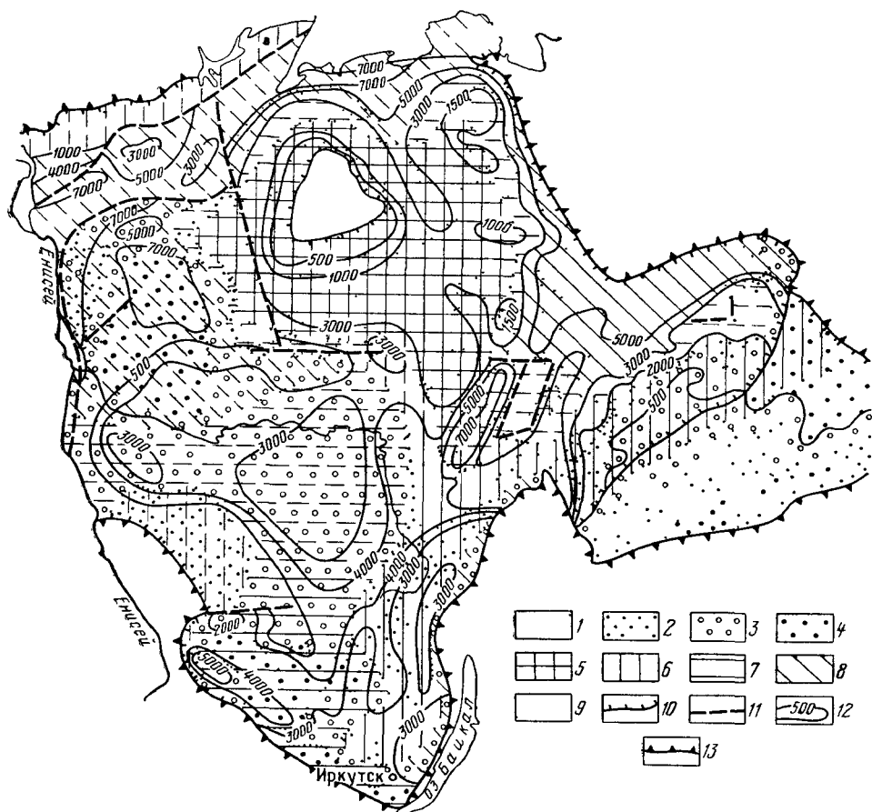
Рис 30 Схема распространения пресных и соленых подземных вод и их мощность
