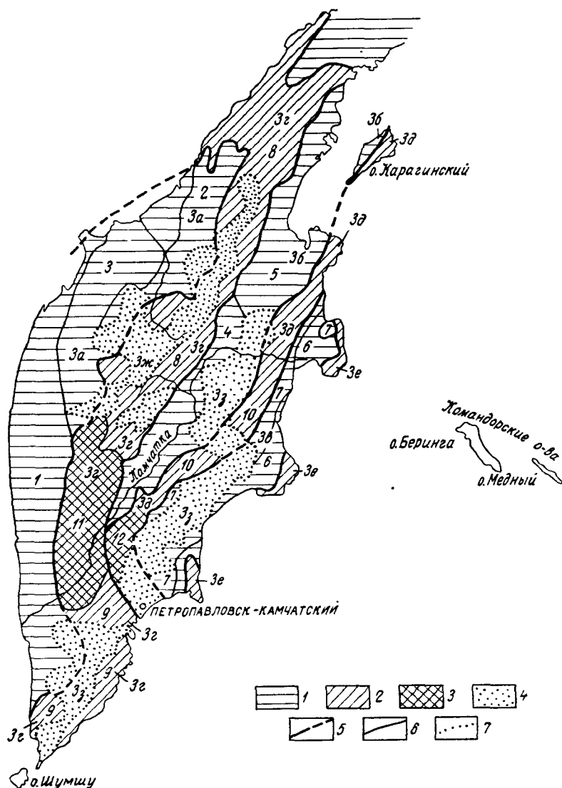
Рис. 49. Схема гидрогеологического районирования Камчатки (XV-3):
