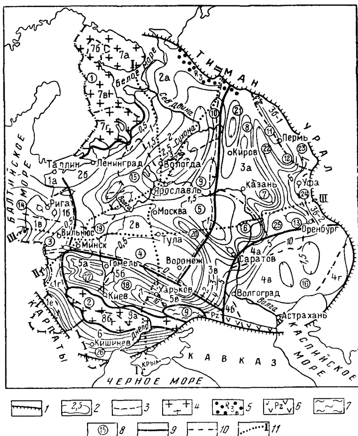
Рис 12 Схема рельефа и структур фундамента и гидрогеологического районирования По Б. Н. Архангельскому.
