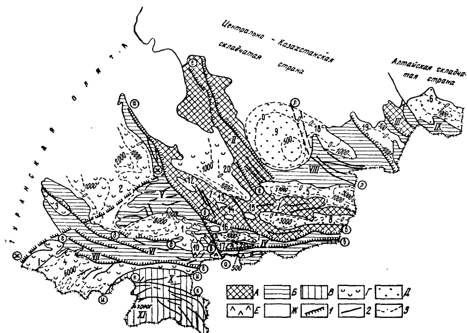
Рис. 67. Структурно-тектоническая схема Тянь-Шаньско-Джунгаро-Памирской складчатой области (по материалам тектонической карты Евразии масштаба 1:5 000 000, 1966 г. с дополнениями по новейшим данным Казахского и Узбекского гидрогеологических трестов и геологических управлений).
