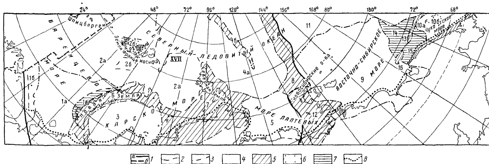
Рис. 35 Схема гидрогеологического районирования Арктического пояса (XVII) артезианских бассейнов По Н. Н. Толстихину, 1967
