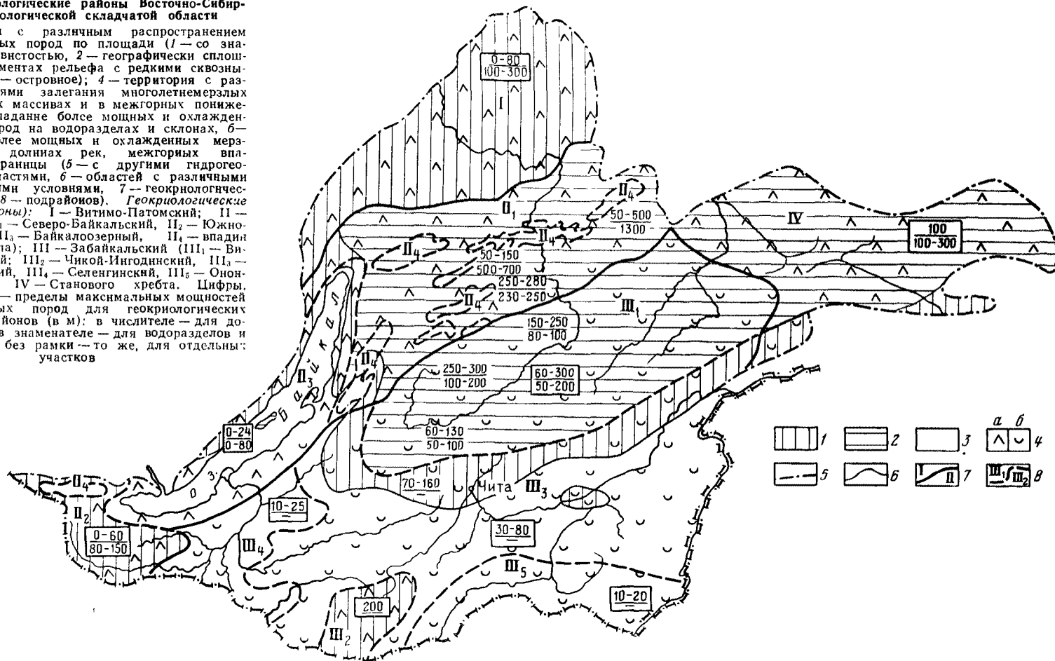
Рис. 87. Геокриологические районы Восточно-Сибирской гидрогеологической складчатой области
