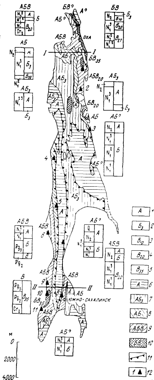
Рис. 61. Схема гидрохимической зональности. По О. В. Равдоникас, 1967.
