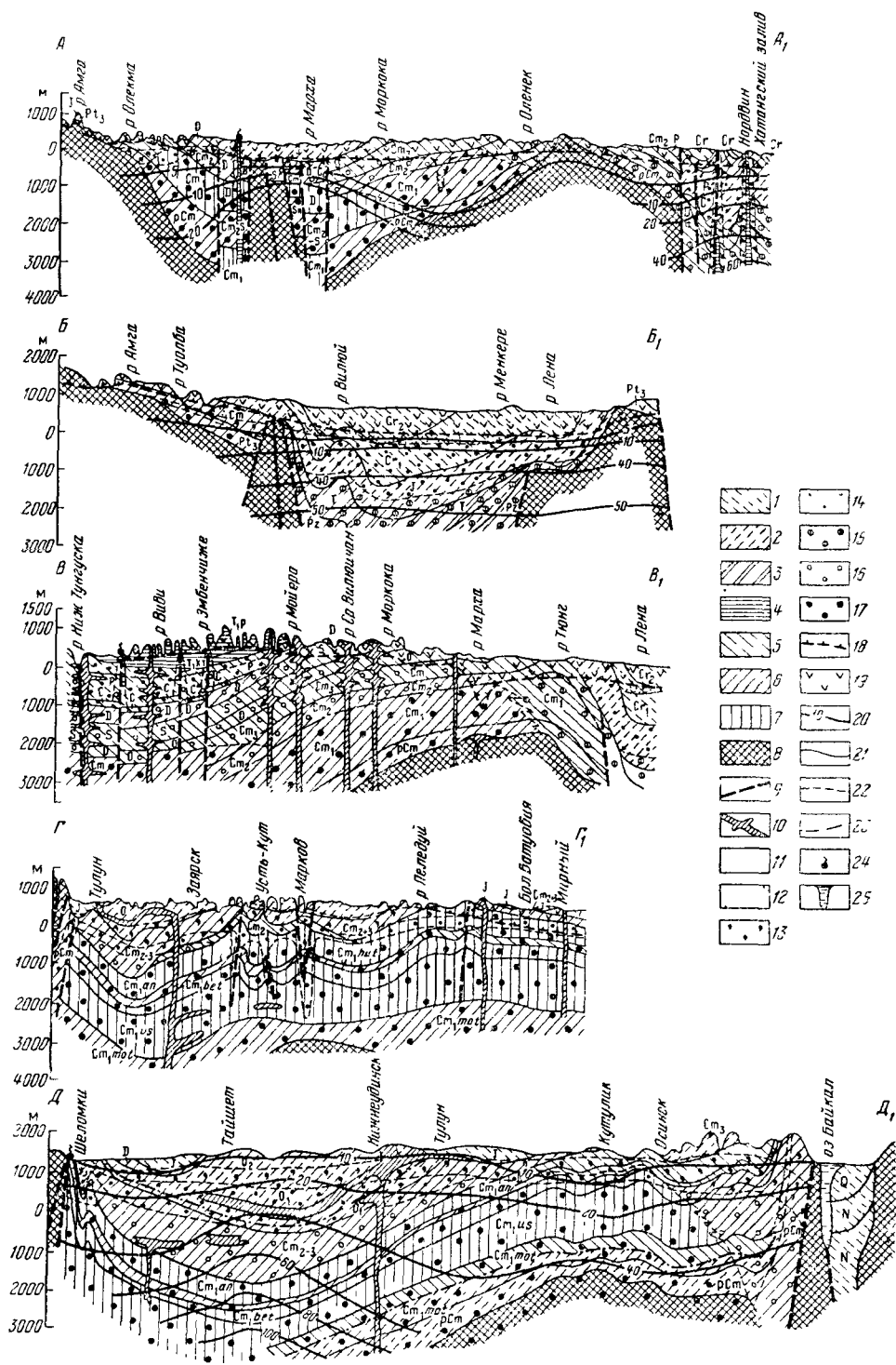
Рис. 28. Гидрогеологические профили по линиям А-А 1 , Б-Б 1 , В-В 1 , Г-Г 1 , Д-Д 1 (расположение профилей см. на рис. 27).
