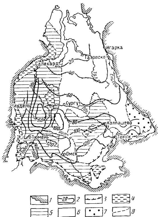
Рис. 16. Схема пьезометрической поверхности и песчаности отложений третьего гидрогеологического комплекса. По И. И. Нестерову, А. Д. Резникову, 1967
