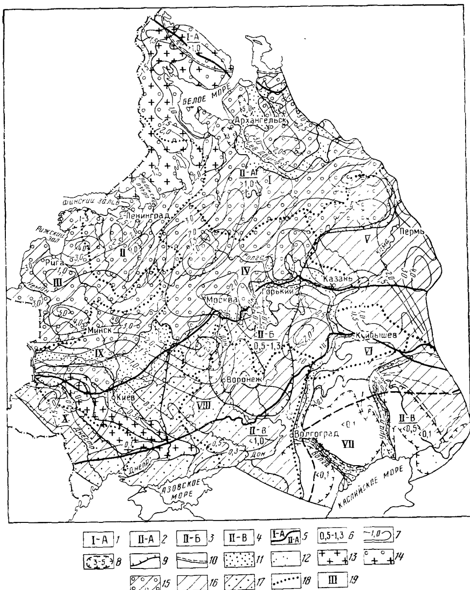
Рис. 2. Карта-схема подземного стока, зон увлажнения и бассейнов стока Восточно-Европейской (Русской) платформы. Составила Я. А. Сыровашкина.
