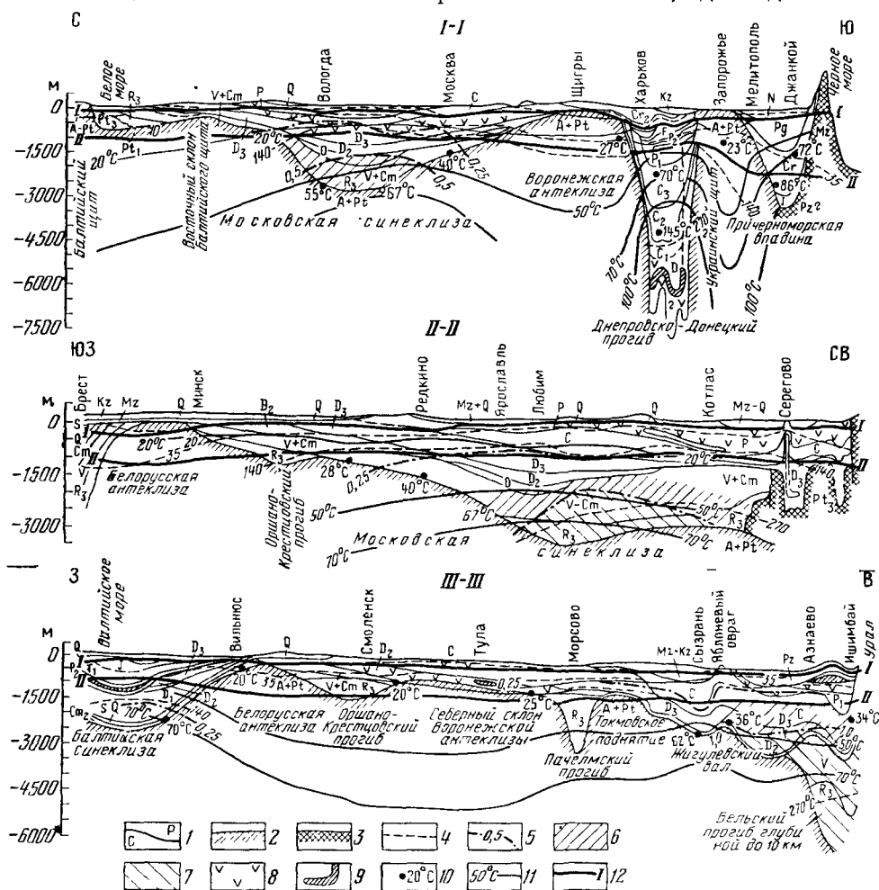
Рис. 3. Структурно-гидрогеологические разрезы (см. рис. 12). Составил Б. Н. Архангельский. 1 — стратиграфические границы укрупненных водоносных комплексов с индексами; 2 — поверхность кристаллического докембрийского фундамента (А-Рт-Рт 1 ); 3 — поверхность послерифейского фундамента Прикамья, палеозойского и мезозойского складчатого основания Причерноморья; 4 — изолинии минерализации подземных вод, г/кг (границы основных гидрохимических зон); 5 — изобромы, г/кг; 6 — рассолы хлоридные натриево-кальциевые; 7 — рассолы хлоридные кальциево-натриевые; 8 — гипс, ангидрит, заглинованные породы; 9 — каменная соль; 10 — температура подземных вод, °С; 11 — изотермы (20, 50, 70, 100 °С); 12 — нижние границы гидродинамических зон: I — свободного водообмена, II — затрудненного водообмена
