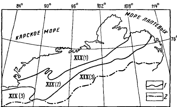
Рис. 91. Схема гидрогеологического районирования Таймырской складчатой области (XIX).
