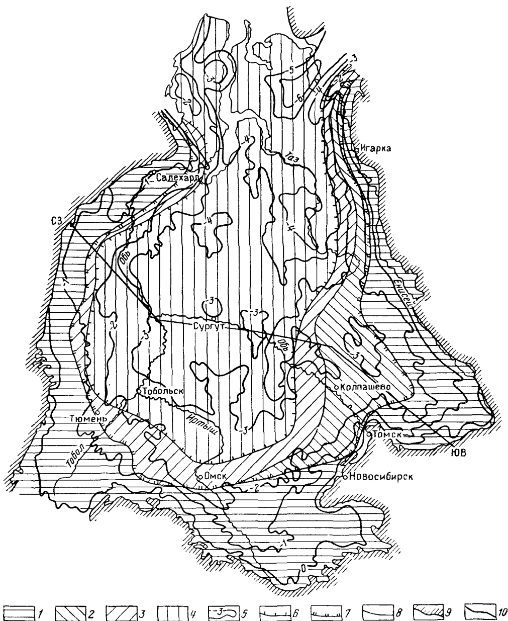
Рис. 22. Схема районирования нижнего гидрогеологического этажа.
