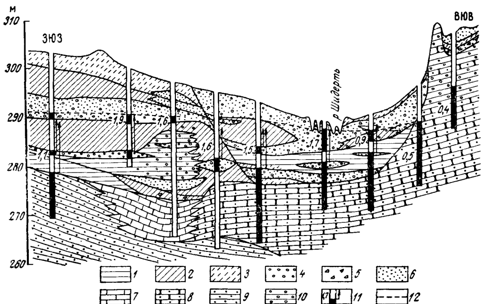
Рис. 76. Гидрогеологический разрез долины р. Шидерты ниже впадения р. Карасу. По З. Н. Рождественской и С. Г. Шапской.
