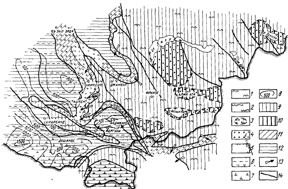
Рис 74. Палеогидрогеологическая схема эпохи максимальной верхнемеловой (сенон) трансгрессии По Б. Е. Антыпко и И. Е. Лагутину.
