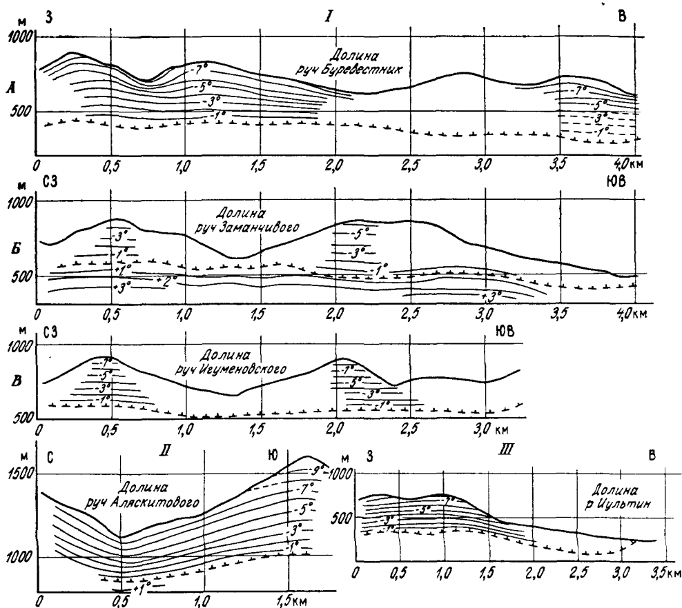
Рис. 52. Геотермические разрезы:
