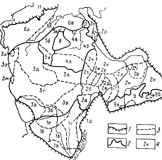
Рис. 29. Схема гидрогеологического районирования Восточно-Сибирской артезианской области.
