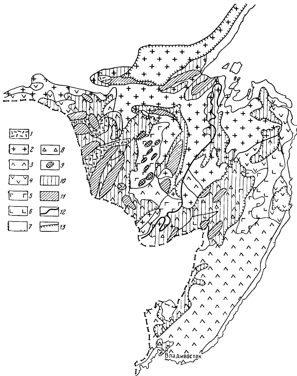
Рис 90. Гидрогеохимическая схема.
