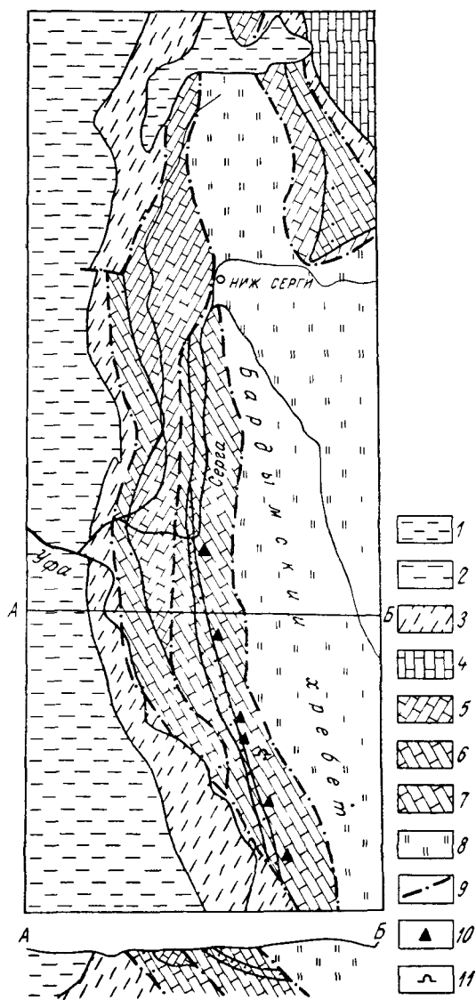
Рис. 65. Гидрогеологическая схема Нижне-Сергинской синклинали. Составил В. И. Антипин.
