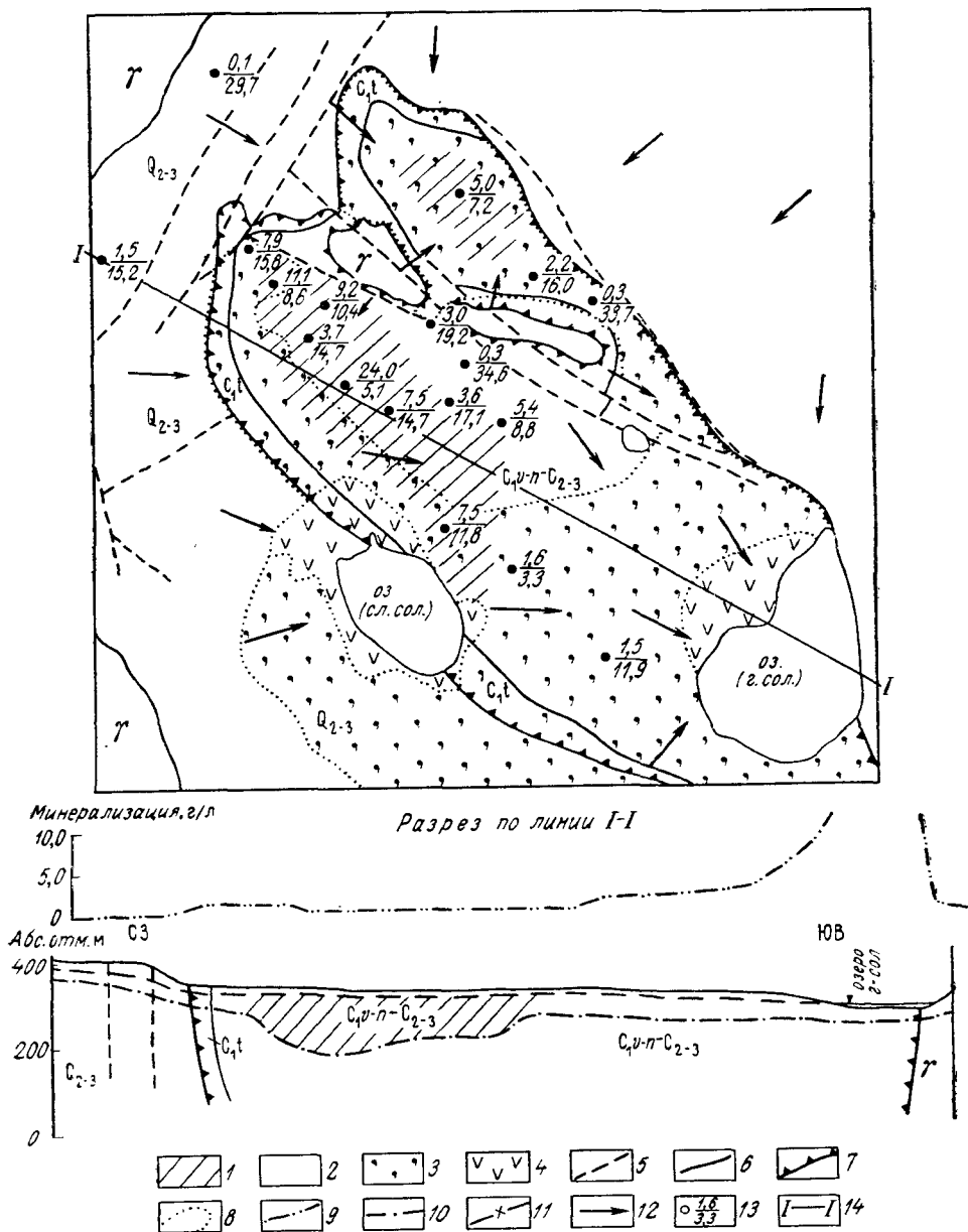
Рис. 80. Гидрогеологическая схема мульд второго типа:
