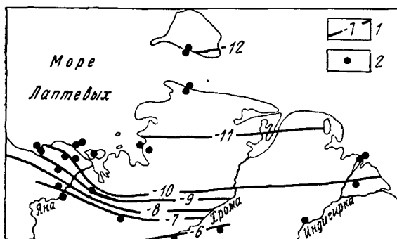
Рис. 53. Изменение температуры многолетнемерзлых пород у подошвы слоя с ее годовыми колебаниями. По Н. Ф. Григорьеву, 1966. 1 — изотермы; 2 — геотермические скважины
