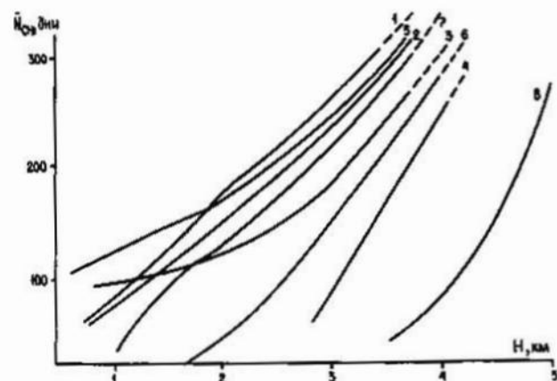
Рис.4.17. Изменение с высотой H среднего числа дней со снежным покровом \bar{N}_{CH} на Тянь-Шане (1-5) и Памиро-Алае (6-8). Бассейны рек: 1 - Пскем, 2 - Кугарт, Яс-си, 3 - Нарын (среднее течение), 4 - Б.Нарын, 6 - Зеравшан. Участки горной системы: 5 - северный склон Заилийского Алатау, 7 - южный склон Гиссарского хребта, 8 - Восточный Памир
