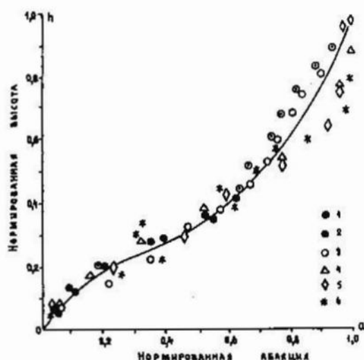
Рис.7.3. Распределение абляции на ледниках с высотой: 1 - Марухский, 2 - Джанкуат, 3 - Абрамова, 4 - Центральный Туюкский, 5 - Малый Актру, 6 - № 31, \bar{h} = (\bar{h}_i - \bar{h}_0) / (\bar{h}_s - \bar{h}_0) , где \bar{h}_i - средняя высота i -ой зоны между наивысшей точкой бассейна и концом ледника, \bar{h}_0 - средняя высота самой нижней высотной зоны ледника, \bar{h}_s - средняя высота самой верхней высотной зоны ледникового бассейна; a = (a_i - a_0) / (a_{max} - a_0) , где a_i - абляция в i -ой высотной зоне, a_0 - минимальная абляция (в верхней высотной зоне), a_{max} - наибольшая из величин абляции по высотным зонам
