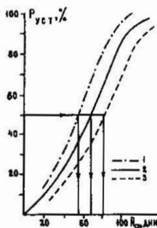
Рис. 4.21. Вероятность образования устойчивого снежного покрова P_{\text{уст}} в зависимости от среднего числа дней со снежным покровом \bar{N}_{\text{сн}} в многоснежных (1), среднеснежных (2) и экстремально малоснежных (3) горных районах
