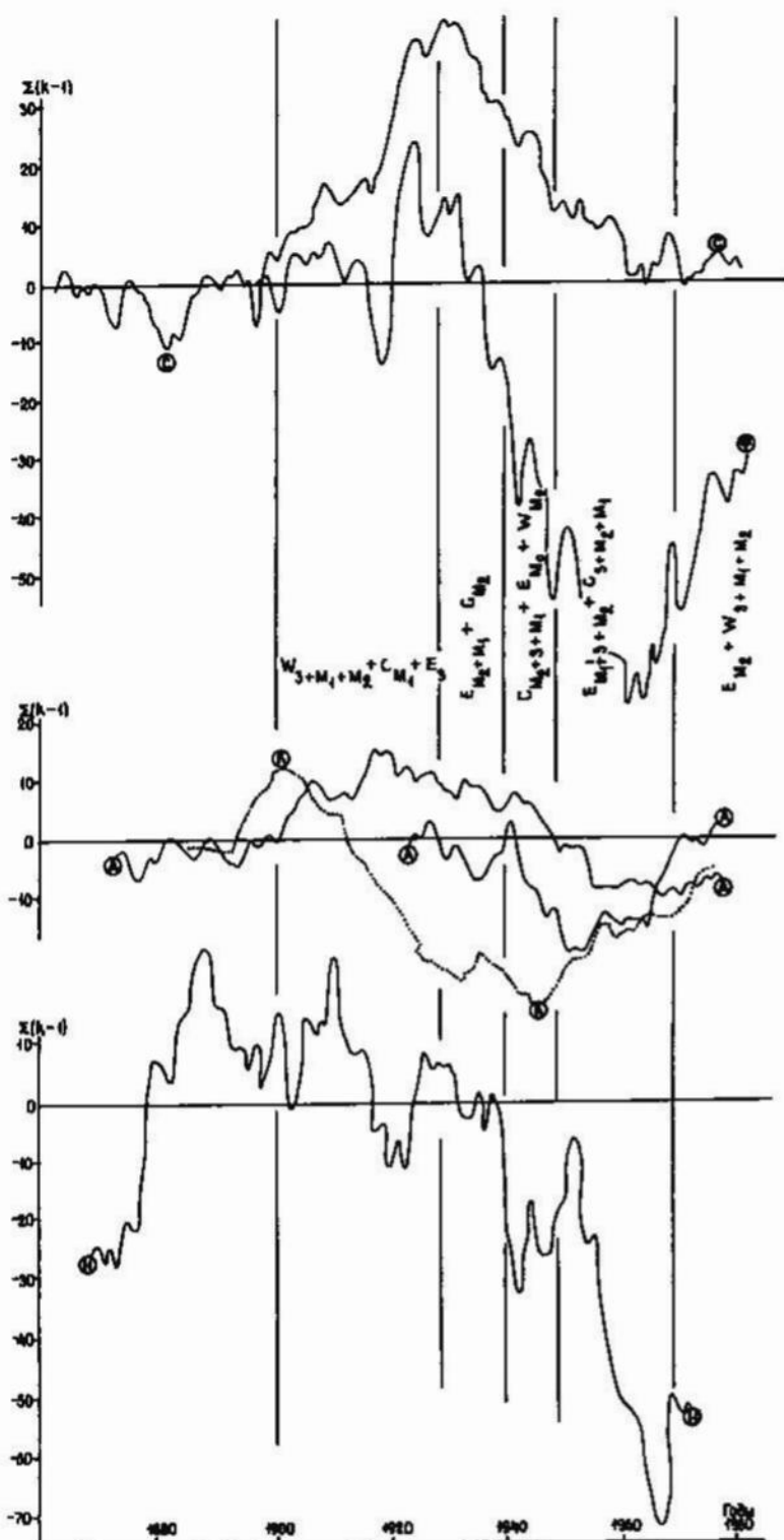
Рис. 7.13. Тенденция и колебания баланса массы ледников, представленные в виде интегральных разностных кривых. Буквенные обозначения - названия ледников: С - Стурбреэн, Ф - Фольгфонни, А - Большой Алецкий, Д - Джанкуат, К - Южный Каскадный, И - ИГАН, Индексы атмосферных циркуляционных эпох по А.А.Гирсу (1971)
