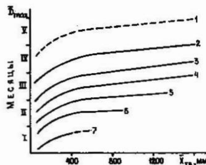
Рис.4.7. Зависимость средних дат накопления максимальных снегозапасов \bar{D}_{max} от годового количества твердых осадков X_{TB} и продолжительности холодного периода N_{TL0} : 1 - 300, 2 - 250, 3 - 200, 4 - 150, 5 - 100, 6 - 50, 7 - 0 дней
