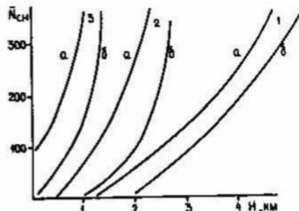
Рис.4.18. Изменение с высотой H среднего числа дней со снежным покровом \bar{N}_{CH} в Кордильерах Южной Америки: 1 - 33° ю.ш., 2 - 40° ю.ш., 3 - 50° ю.ш.; а - восточные, б - западные склоны гор. По Т.Г.Кадошцевой (1987). Зависимости получены в результате косвенных расчетов
