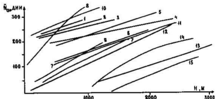
Рис.4.16. Изменение с высотой H среднего числа дней со снежным покровом \bar{N}_{\text{сн}} : 1 - плато Путорана, 69^{\circ} с.ш.; 2 - Скандинавские горы, 66-70^{\circ} с.ш.; 3 - горы Брукса, 68-69^{\circ} с.ш.; 4 - Верхоянский хребет, 66-68^{\circ} с.ш.; 5 - Северное Забайкалье, 55-57^{\circ} с.ш.; 6 - Южное Забайкалье, 50-52^{\circ} с.ш.; 7 - Скалистые горы, 51-52^{\circ} с.ш.; 8 - Исландия, 64^{\circ} с.ш.; 9 - Скандинавские горы, 58-59^{\circ} с.ш.; 10 - Камчатка, южный район и Кроноцкий п-ов; 11 - Каскадные горы, западные склоны, 43-45^{\circ} с.ш.; 12 - Западный Кавказ, южный склон западной части Кавказского хребта; 13 - Восточный Кавказ, северный склон Кавказского хребта в пределах Дагестана; 14 - Сьерра-Невада, западные склоны, 36-40^{\circ} с.ш.; 15 - Сьерра-Невада, восточные склоны, 38-39^{\circ} с.ш. Зависимости 12, 13 по Цоям (1988)
