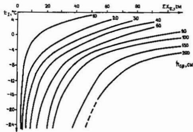
Рис.5.2. Зависимость максимальной декадной толщины снежного покрова h_{cp} , см от суммы осадков холодного периода \Sigma X_{t_1-t_2} и средней температуры января t_I
