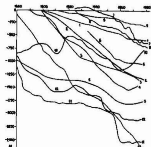
Рис. 7.17. Кумулятивные кривые изменения фронта ледников с конца прошлого века. Западный Кавказ: 1 - Большой Кичкинекол, 2 - Даут, 3 - Цаннер, 4 - Кибиса; Восточный Кавказ: 5 - Тихицар, 6 - Юго-восточный; Кунгей Алатау: 7 - Аксу Восточный; Заилийский Алатау: 8 - Центральный Туусульский; Алтай: 9 - Малый Актру; Альпы: 10 - Верхний Гриндельвальд, 11 - Хоффири, 12 - Ронский, 13 - Большой Алевский
