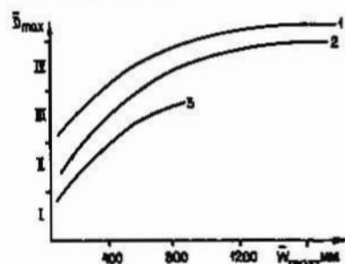
Рис.4.8. Зависимость средних дат накопления максимальных снегозапасов \bar{D}_{max} от их нормы W_{max} и широты местности на территории Западной Европы. 1 - 56-70°, 2 - 46-55°, 3 - 40-45° ш. По Е.М.Локтионовой (1987)
