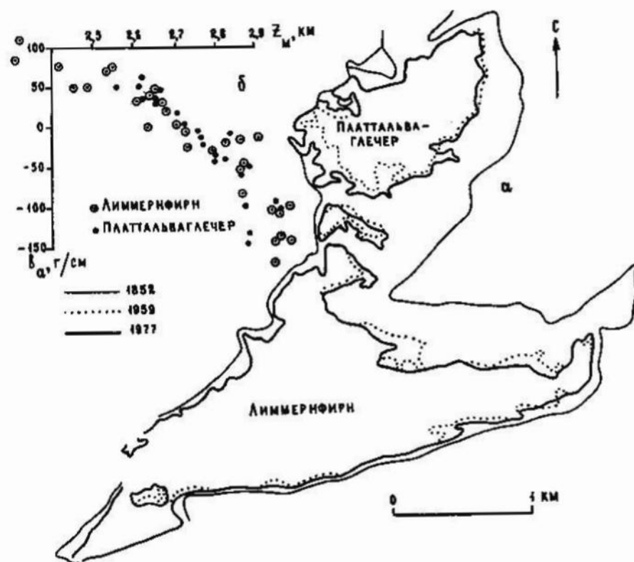
Рис.7.15. Изменение контуров (а) и характер зависимости баланса массы от высоты границы питания (б) на ледниках Лиммернфирн и Платтальяваглетчер в Альпах (Les Variations..., 1983)
