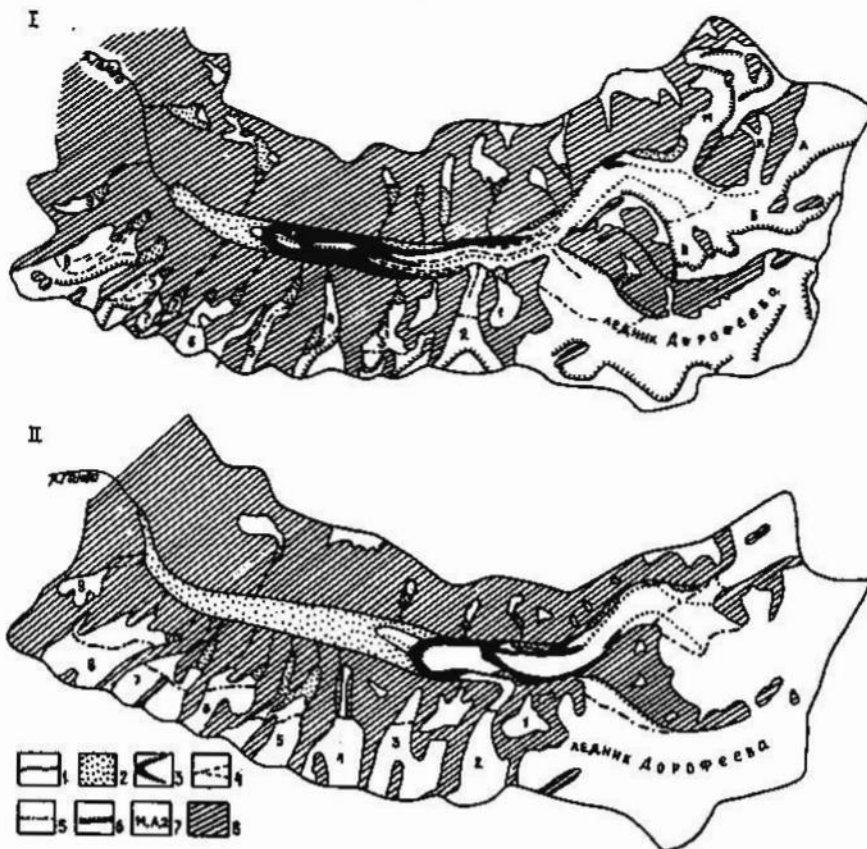
Рис.2.5. Схемы опеденения долины р.Гандо. I. По наблюдениям в 1948 г. (Тимашев, 1949). II. По результатам дешифрирования космического снимка 1973 г. 1 - водоразделы, 2 - моренный покров ледника, 3 - валы поверхностных морен, 4 - ледниковые ручьи, 5 - фирновая граница, 6 - основные бергшруды, 7 - обозначения отдельных ветвей ледника Гандо и ледников левого склона долины, 8 - склоны, свободные от снега и льда
