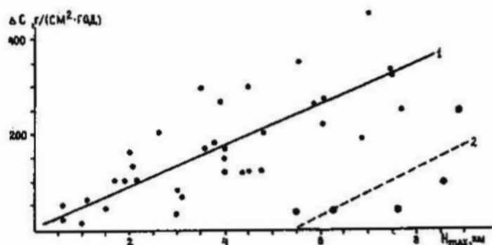
Рис. 7.9. Зависимость различий в интенсивности питания \Delta C наветренных и подветренных краев ледниковых систем от высоты горных массивов H_{max} : 1 - ледниковые системы на архипелагах островов и в горных массивах на побережьях и над равнинами; 2 - ледниковые системы в горных массивах над Центрально-Азиатским нагорьем
