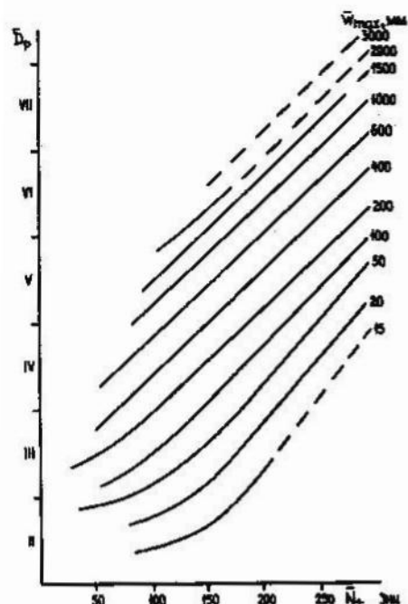
Рис. 4.20. Зависимость средних дат разрушения устойчивого снежного покрова \bar{D}_p от продолжительности холодного периода N_{\text{хл}} и норм максимальных снегозапасов W_{\text{max}} : 1 - 15 мм, 2 - 20 мм, 3 - 50 мм, 4 - 100 мм, 5 - 200 мм, 6 - 400 мм, 7 - 600 мм, 8 - 1000 мм, 9 - 1500 мм, 10 - 2000 мм, 11 - 3000 мм
