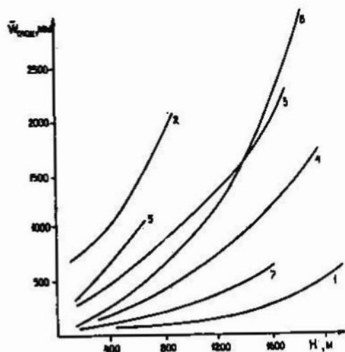
Рис.4.1. Изменение с высотой H_{сн} средних максимальных снегозапасов \bar{W}_{зак} в горах субарктического и севера умеренного поясов. Аляска: 1 - горы Брукса; 2 - горы Св.Ильи, западные наветренные склоны, 3 - горы Чугач, южные наветренные склоны, 4 - горы Чугач, северные подветренные склоны; Скандинавские горы: 5 - северные наветренные склоны, 6 - юго-западные наветренные склоны, 7 - южные склоны. Зависимости 5-7 по (Э.И.Локтионовой, 1987).
