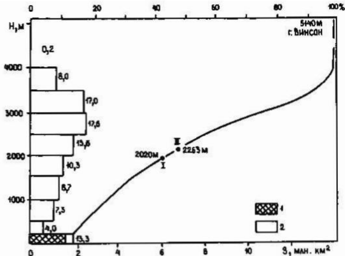
Рис.6.1. Гипсографическая кривая поверхности Антарктического покрова (Винник и др., 1976): 1 - шельфовые ледники, 2 - диаграмма процентного соотношения площадей высотных ступеней; I - средняя высота поверхности всего ледникового покрова, II - то же наземного ледникового покрова
