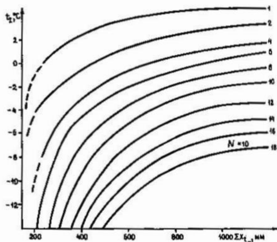
Рис.5.3. Зависимость числа дней с твердыми осадками более 10 мм/сут N_{10} от суммы осадков холодного периода \Sigma X_{t_1-t_2} и средней температуры января t_I
