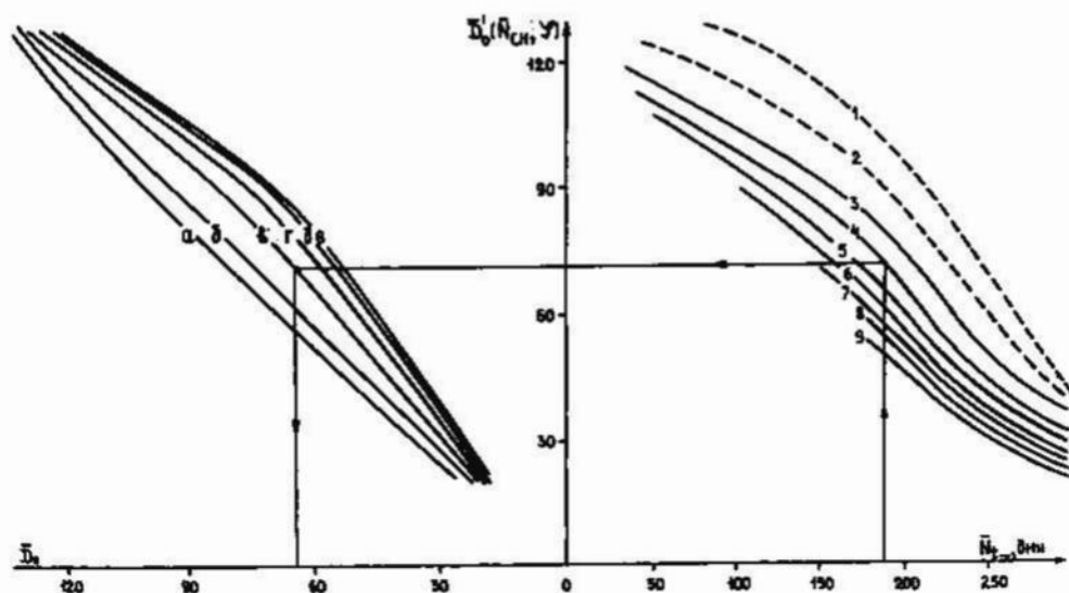
Рис.4.19. Зависимость средних дат образования устойчивого снежного покрова \bar{D}_o от продолжительности холодного периода N_{холод} , нормы максимальных снегозапасов W_{max} и широты \varphi : 1-30°, 2 - 35°, 3 - 40°, 4 - 45°, 5 - 50°, 6 - 55°, 7 - 60°, 8 - 65°, 9 - 70° с.ш. W_{max} , мм: а - 20, б - 50, в - 200, г - 600, д - 1000, е - 2000. \bar{D}_o(N_{CH}, \varphi) - расчетные даты образования устойчивого снежного покрова при фиксированной величине W_{max} . \bar{D}_o , \bar{D}_o(N_{CH}, \varphi) - в днях от 1 сентября
