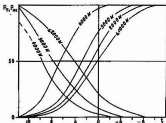
Рис.3.1. Система кривых, определяющих зависимость месячной доли твердых ( P_T, \% ) и жидких ( P_{ж}, \% ) осадков в горах от температуры воздуха ( t, ^\circ C ) и высоты местности
