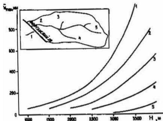
Рис. 4.4. Эффект "массивности" гор на Тянь-Шане. Изменение с высотой H средних максимальных снегозапасов W_{\text{дв}} в долине р. Нарын. Бассейны рек: 1 — Яссы (наветренный склон Ферганского хребта), 2 — Сусамыр (85 км), 3 — Западный Каракол (120 км), 4 — Атбаш (290 км), 5 — Б.Нарын (450 км). В скобках указано расстояние на восток от "экрана" (Ферганского хребта)
