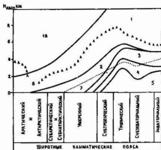
Рис. 5.10. Обобщенная схема высотных поясов лавинообразования. Пояса: 1 - вечных снегов, в том числе 1а - область холодной горной пустыни, 2 - устойчивого зимнего снежного покрова, 3 - неустойчивого зимнего снежного покрова, 4 - редких снегопадов, 5 - бесснежные территории, 6 - обобщенный уровень горных вершин, 7 - верхняя граница лесов
