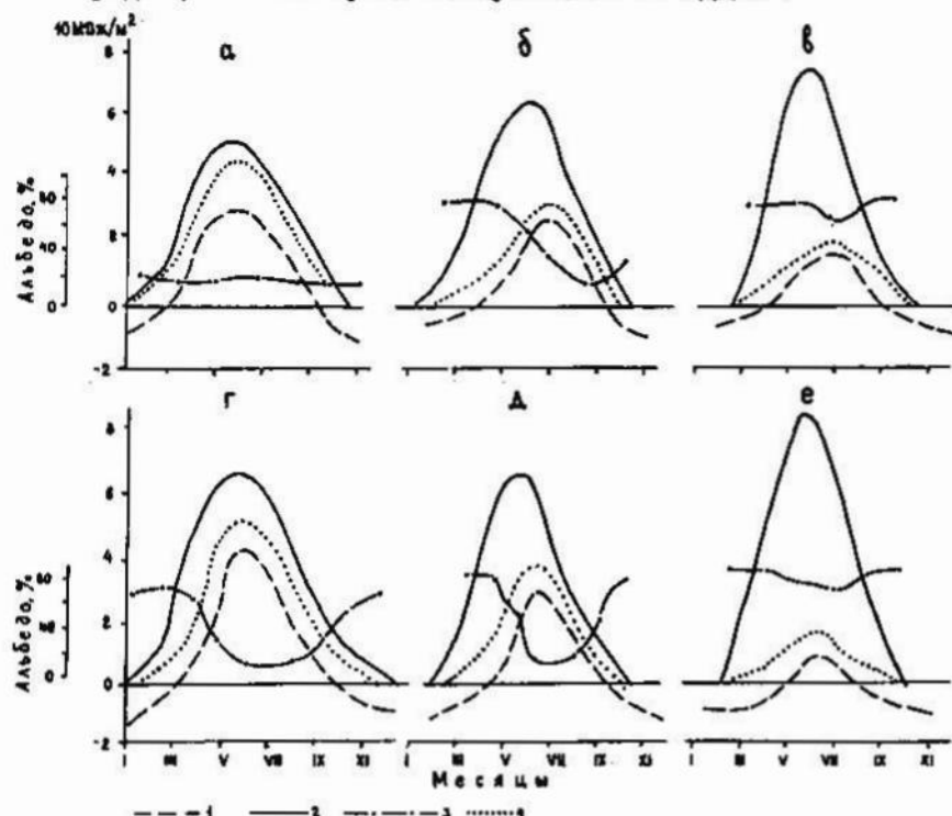
Рис.3.7. Годовой ход радиационного баланса и его составляющих в Арктике: а - открытое море, б - море с сезонными изменениями ледовитости, в - паковый лед, г - побережье арктических морей южнее 70°с.ш., д - побережье арктических морей севернее 70°с.ш., е - ледники. 1 - радиационный баланс; 2 - альbedo, 3 - суммарная радиация, 4 - поглощенная радиация
