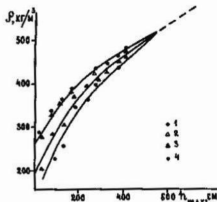
Рис.4.11. Зависимость средней плотности снежного покрова P от максимальной его толщины h в горных районах Северной Америки. Диапазоны широт: 1 - 30-39^\circ ; 2 - 40-49^\circ ; 3 - 50-59^\circ ; 4 - 60-69^\circ \text{с.ш.}
