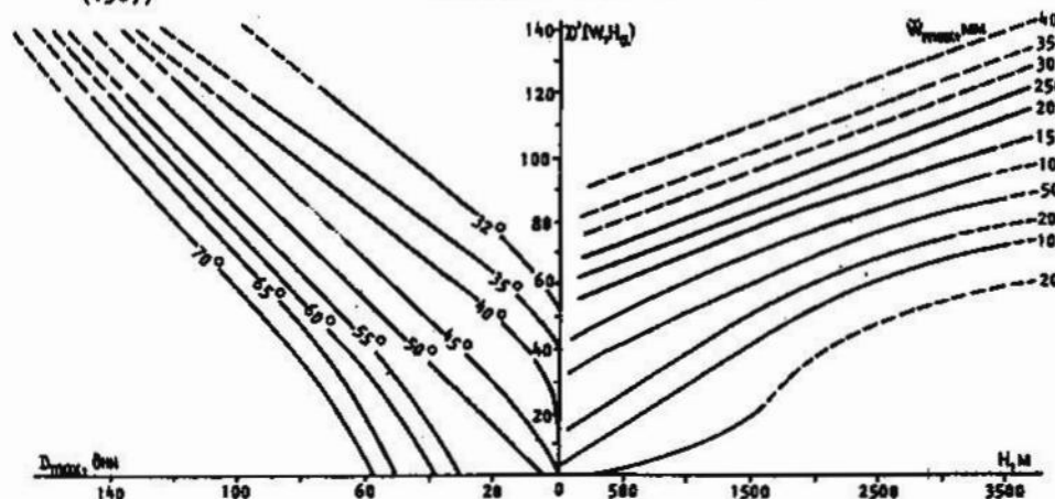
Рис.4.9. Зависимость средних дат накопления максимальных снегозапасов \bar{D}_{max} от их нормы W_{max} , высоты H и широты местности в Кордильерах Северной Америки. \bar{D}(W, H) - расчетные даты накопления максимальных снегозапасов на широте 48°. \bar{D}_{max} - в днях от 1 февраля
