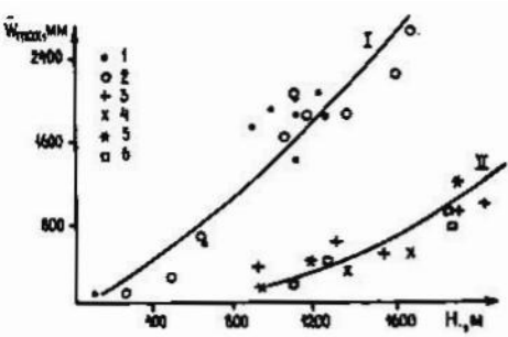
Рис. 4.2. Изменение с высотой H средних максимальных снегозапасов \bar{W}_{max} на наветренных прибрежных (I - Каскадные горы, береговой хребт Канады) и континентальных (II - Колумбийские, Скалистые горы) склонах Кордильер в диапазоне 49-50° с.ш. Бассейны: 1 - Тихого океана; 2, 3, 4, 5, 6 - рек Бейкер, Зап.Кутени, Кетл, Ю.Томпсон, Колумбия, соответственно
