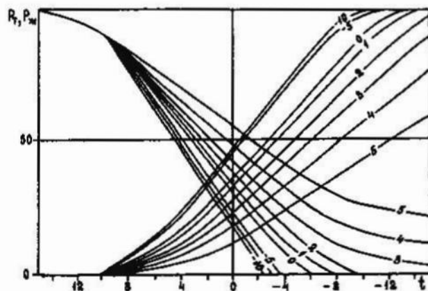
Рис.3.2. Система кривых, определяющих зависимость месячной доли твердых ( P_T, \% ) и жидких ( P_{ж}, \% ) осадков на равнине от температуры воздуха ( t, ^\circ C ) и параметра континентальности (цифры на кривых)
