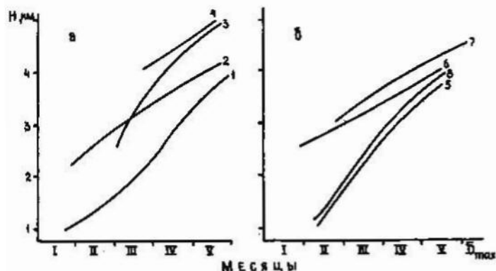
Рис.4.10. Изменение с высотой средних дат накопления максимальных снеготрезоров на Тянь-Шане (а) и Памиро-Алае (б): 1 - южный склон Гиссарского хребта, 2 - бассейн р.Зеравшан, 3 - бассейн р.Муксу, 4 - Восточный Памир, 5 - бассейн р.Пскем, 6 - верховья бассейна р.Чу, 7 - бассейн р.Сарыджаз, 8 - северный склон Заилийского Алатау
