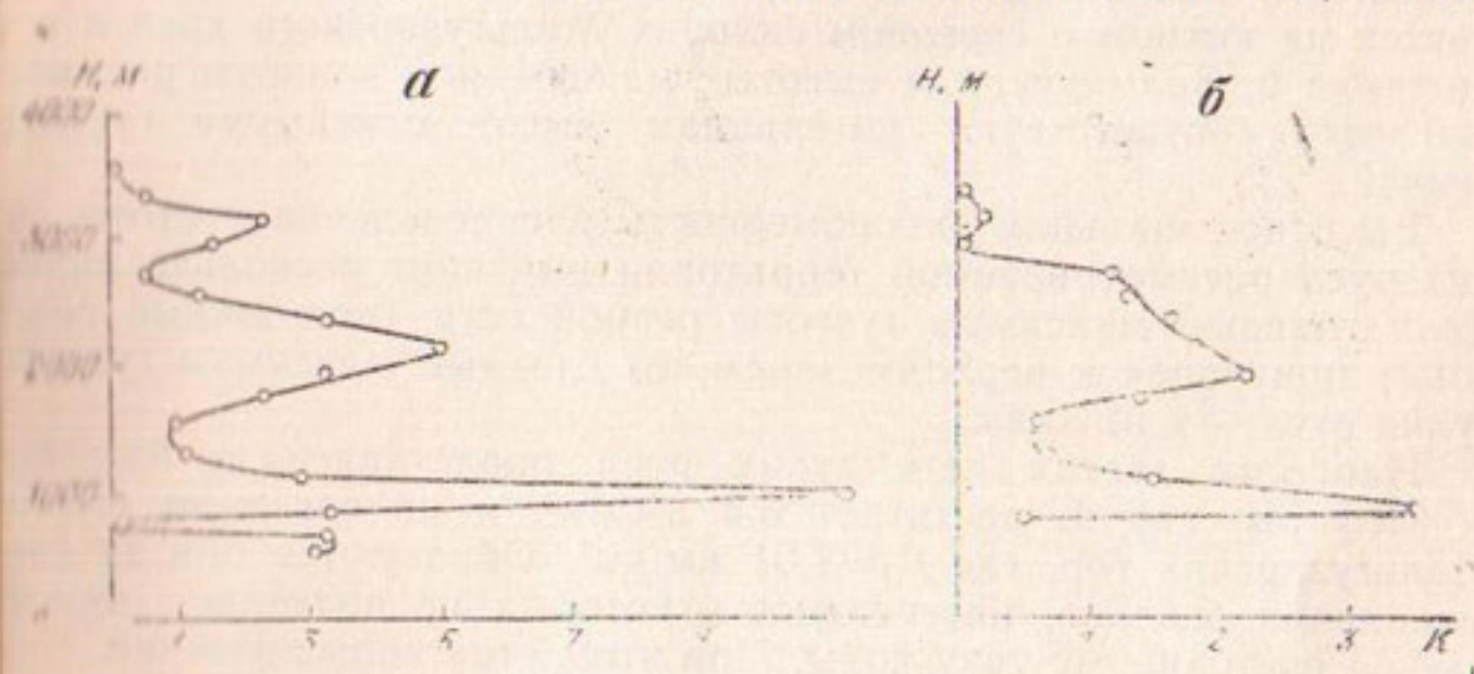
Рис. 14. Распределение показателя полноты родниковой сети по высоте.
