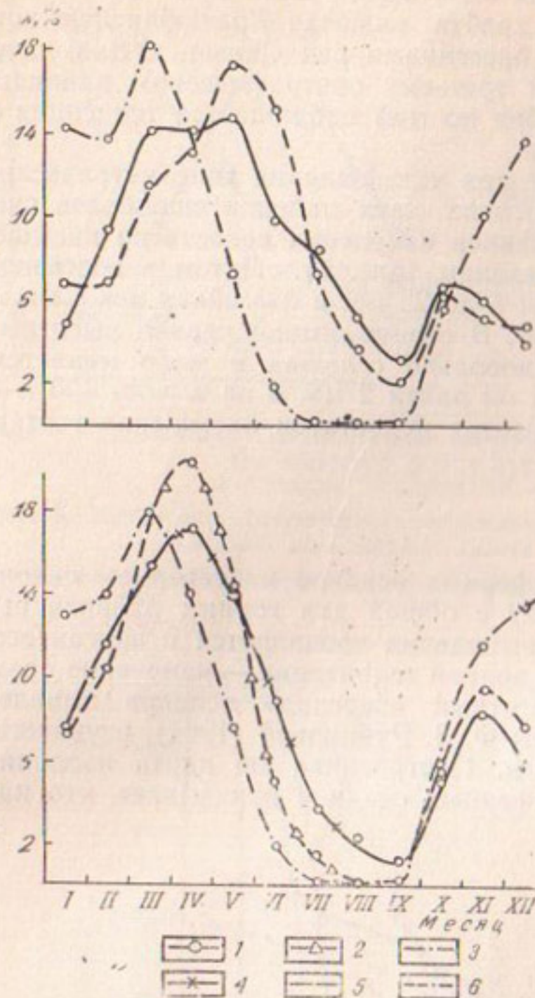
Рис. 9. Внутригодовое распределение атмосферных осадков на северном склоне Туркестанского хребта по характерным станциям:
