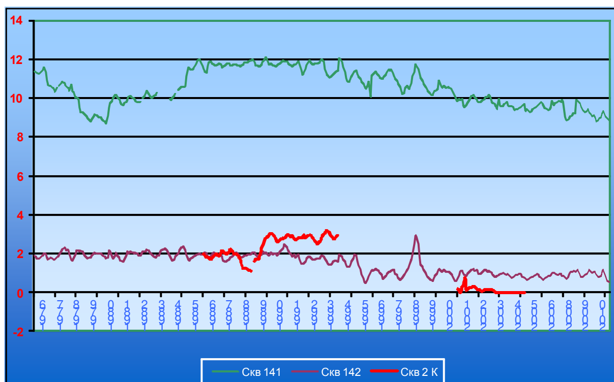
Рис. 1.4. Изменение уровня грунтовых вод в районе Айдаро-Арнасайской системы озер
