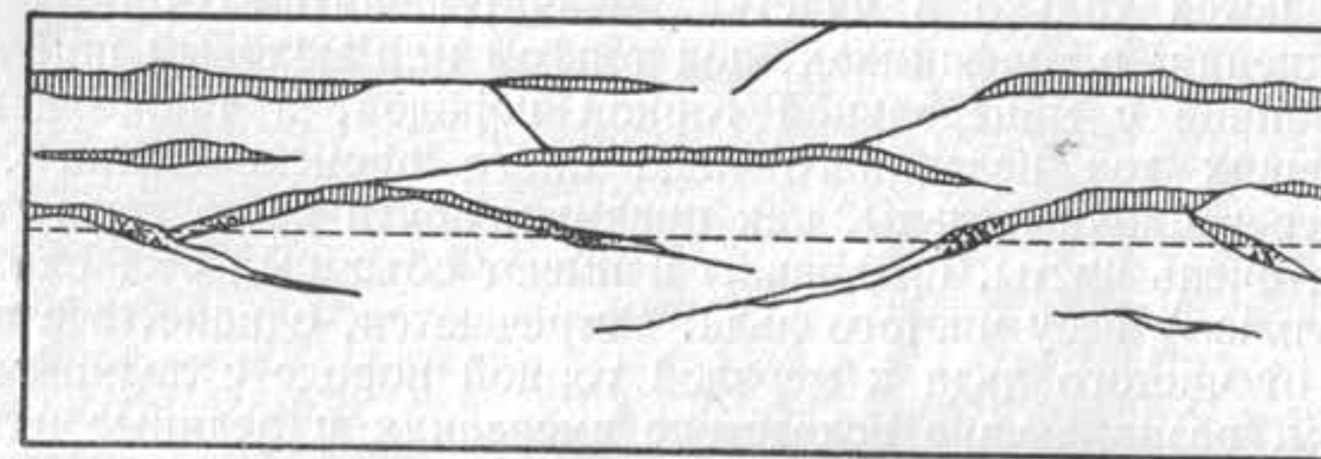
Фиг. 67. Поперечный разрез границы зоны промерзания в глине.
