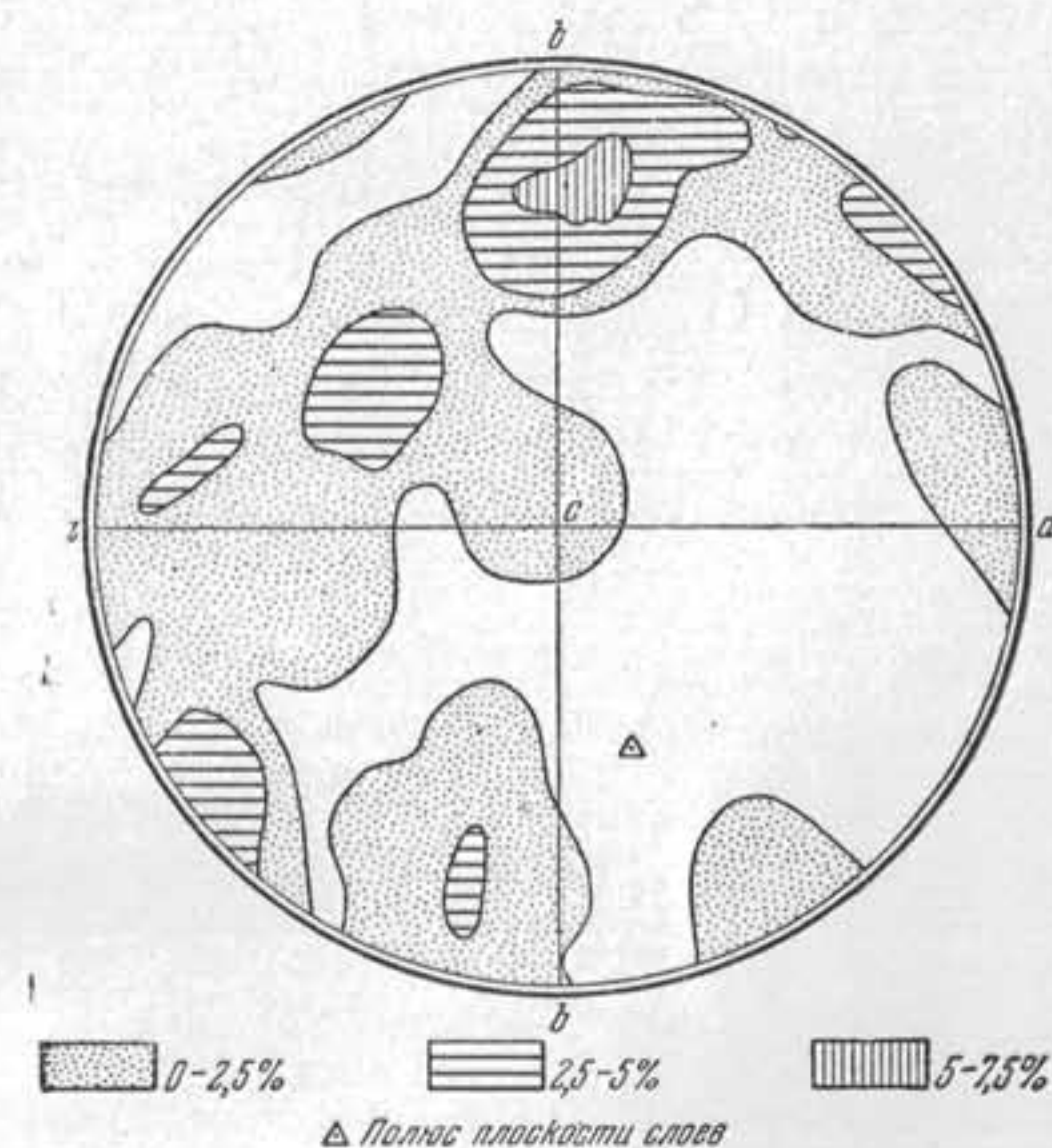
Фиг. 117. Стереограмма кристаллографической ориентировки льда, вмещающего голубую ленту, показанную на фиг. 115 и 116.
