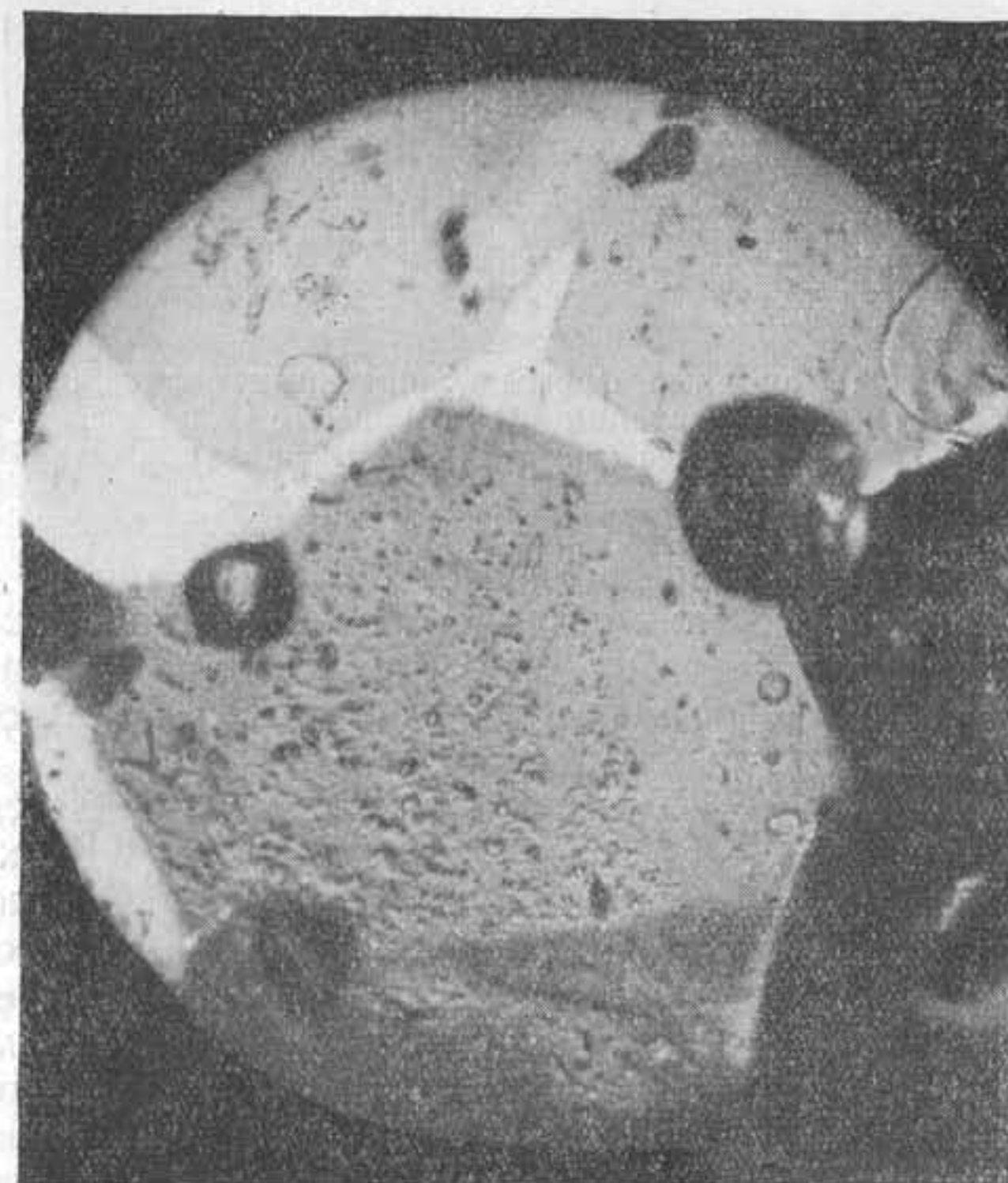
Фиг. 42. Интерсертальные воздушные включения (темные) в конжеляционном льду. \times 3 .
