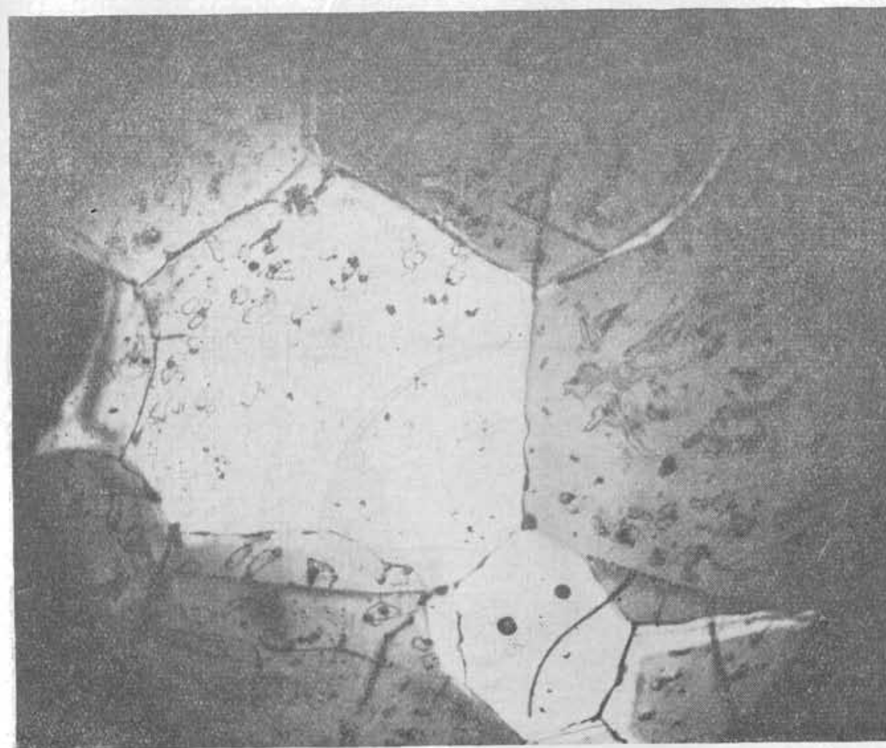
Фиг. 61. Гипидиоморфно-зернистая структура повторно-жильного льда. \times 16,5 .
