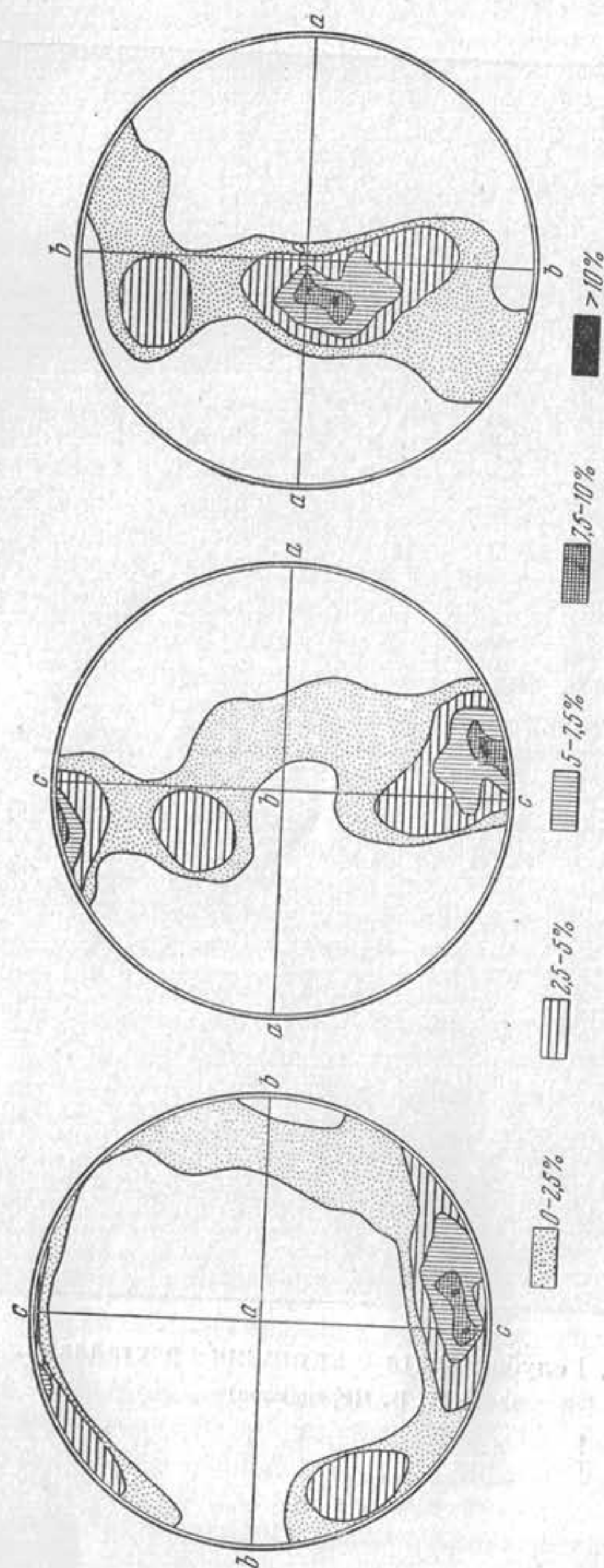
Фиг. 116. Стереограмма кристаллографической ориентировки льда голубой ленты, изображенной на фиг. 115.
