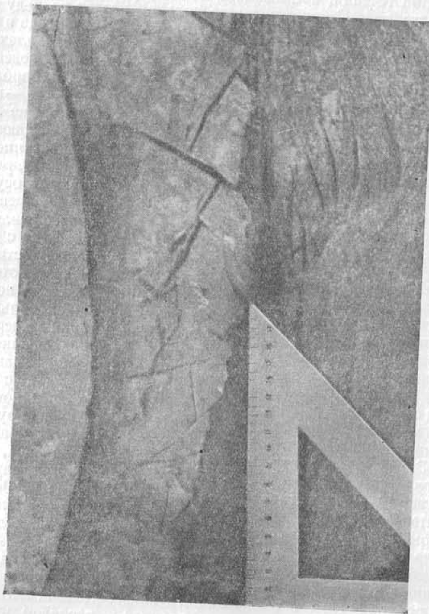
Фиг. 105. Вертикальное сечение контакта повторной ледяной жилы с вмещающей мерзлой породой. Темное—лед, светлое—мерзлая порода. Серия поперечных сросов между главным телом жилы и апофизой. (Фото Б. И. Втюрина)
