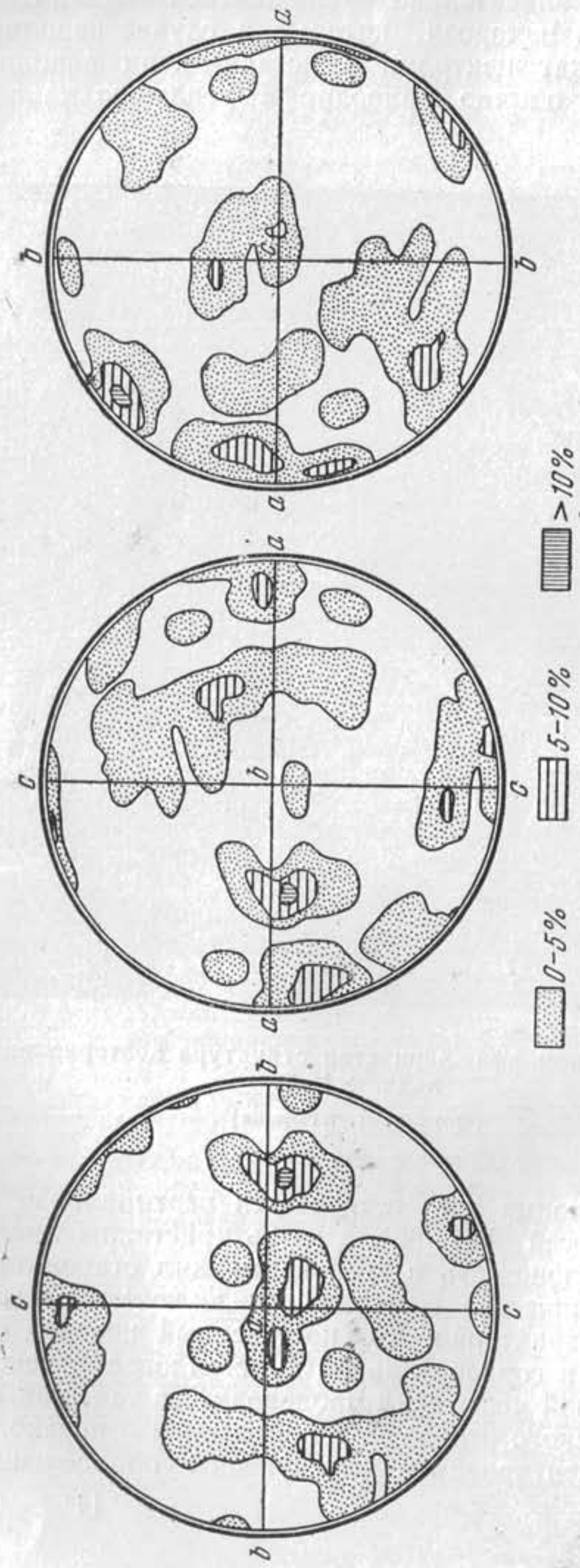
Фиг. 62. Стереогрaмма кристаллографической ориентировки повторно-жидкого льда. Хаотическая ориентировка главных осей.
