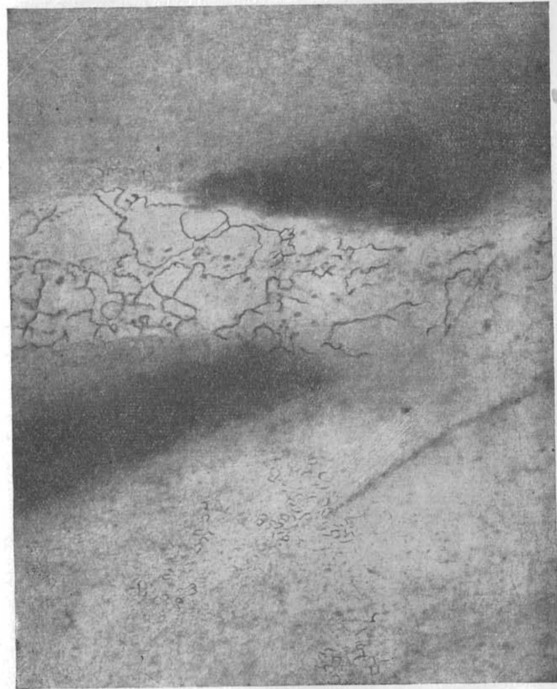
Фиг. 114. Голубая лента, пересекающая слой морены в мелкозернистом вторично-рекристаллизационном льду.
