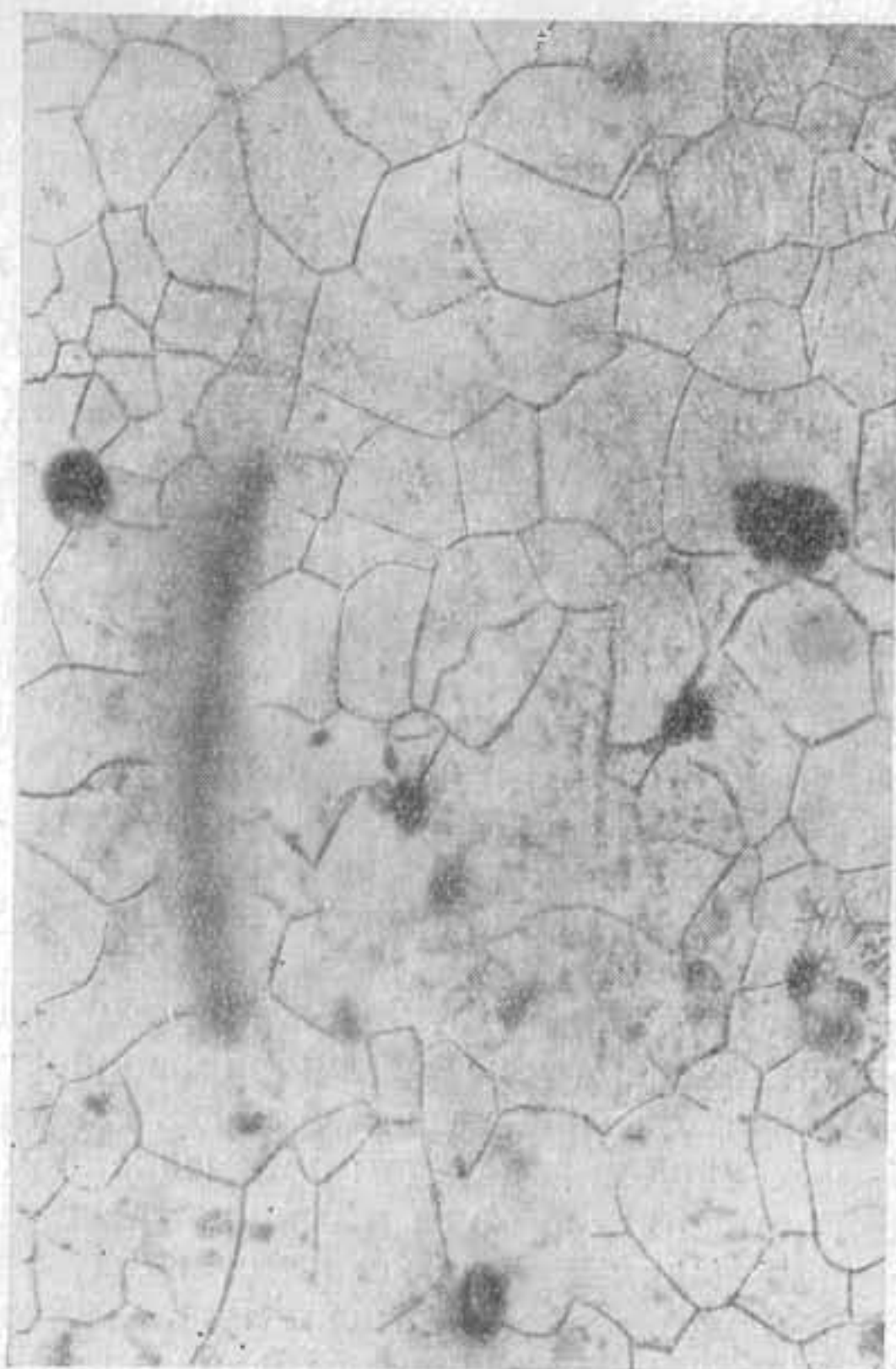
Фиг. 46. Полость по оси вертикальной жилы в ледниковом льду. По структуре жильный лед не отличается от вмещающего. Овальные темные пятна — пузырьки воздуха в ледниковом льду.
