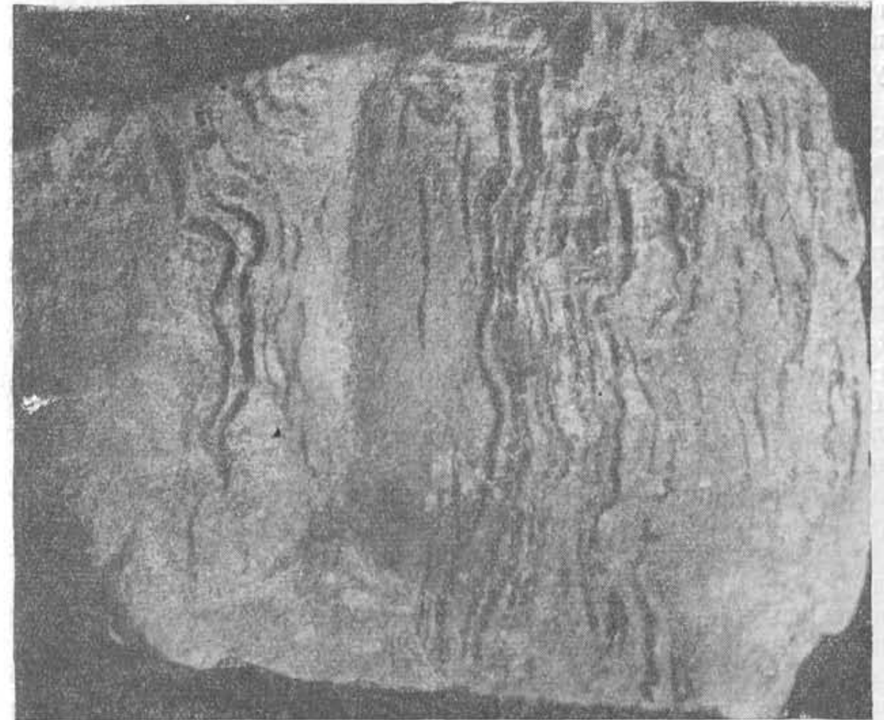
Фиг. 66. Шлыры сегрегационного льда в супеси. \times 0,5 .
