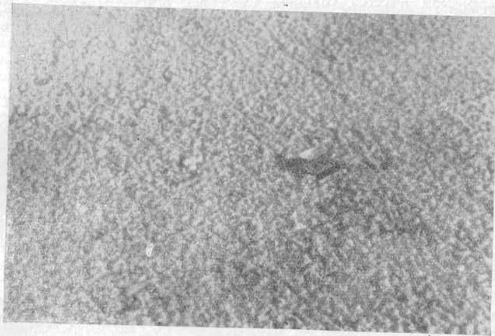
Фиг. 71. Слой тяжелой изморози на поверхности снежного покрова.
