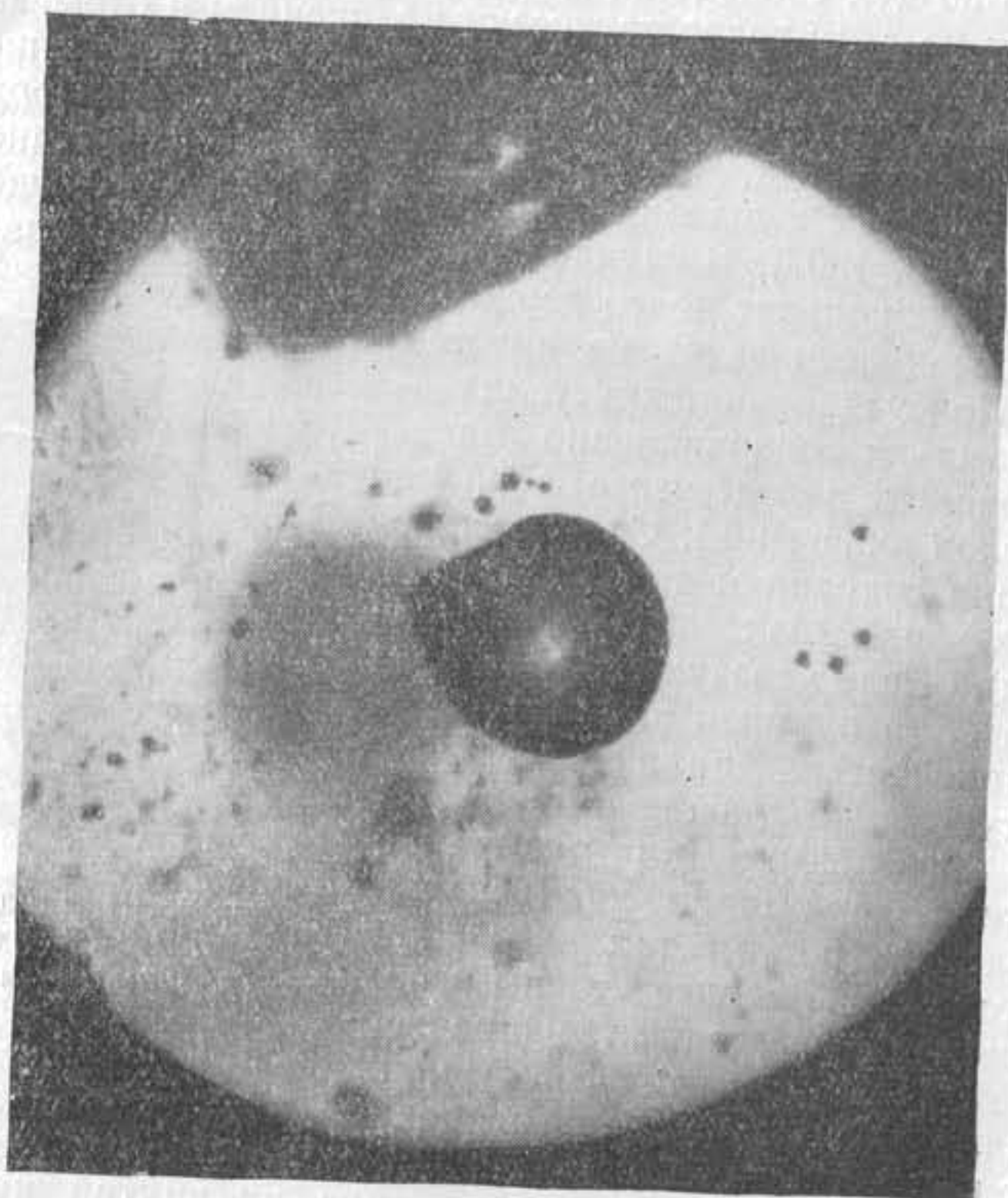
Фиг. 41. Грушевидный пузырек воздуха в конжеляционном льду. \times 10 .
