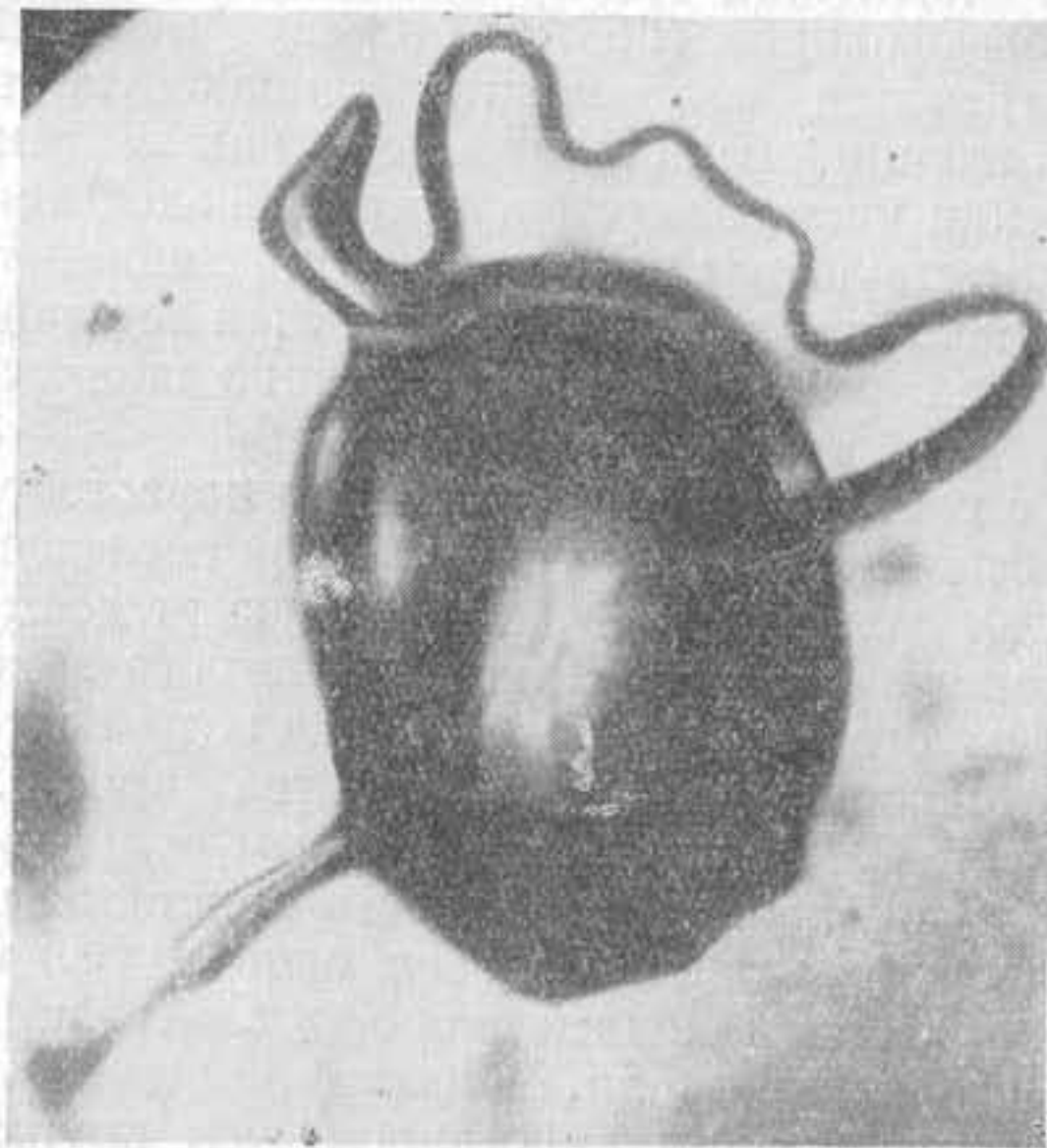
Фиг. 39. Протаивание льда вокруг воздушного пузырька вследствие наличия солей. \times 52 .
