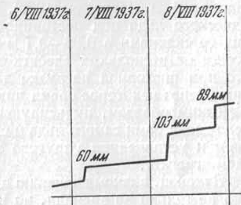
Фиг. 91. Часть автоматической записи движения поверхности ледника Шайглетчер (на Шпицбергене) в 200 м от конца ледника.
