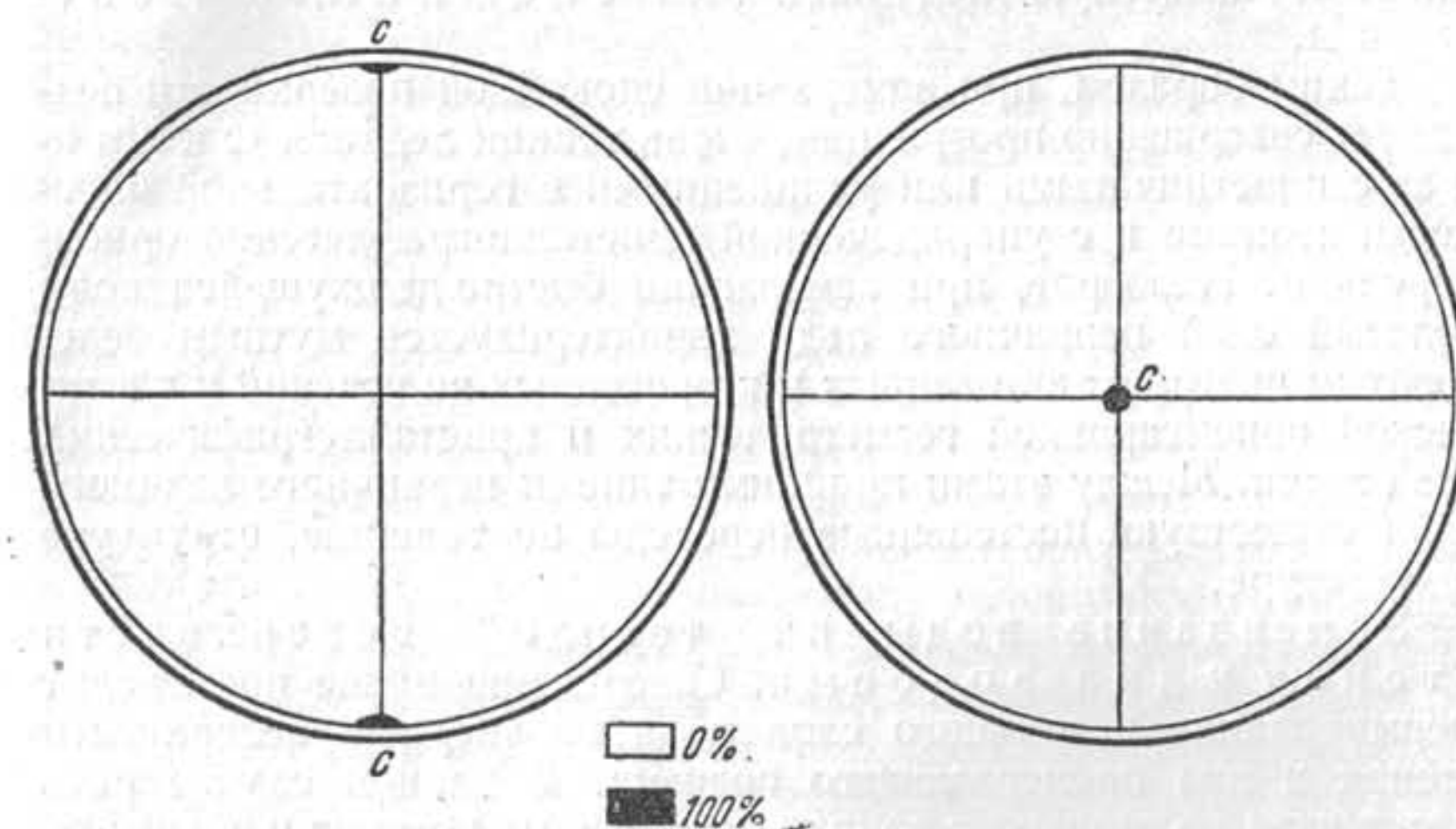
Фиг. 32. Стереогрaмма кристаллографической ориентировки первичного слоя конжеляционного льда на поверхности спокойной воды (очень медленное замерзание).
