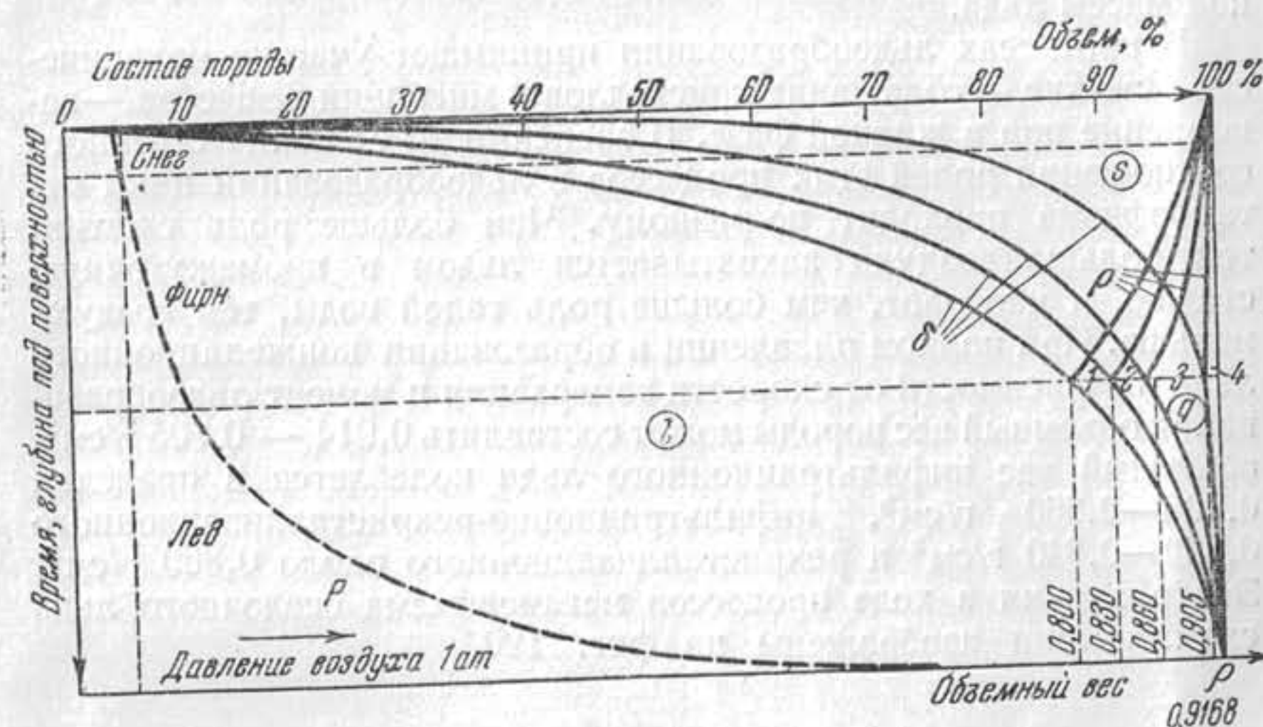
Фиг. 120. Схема циклов метаморфизма осадочного льда.
